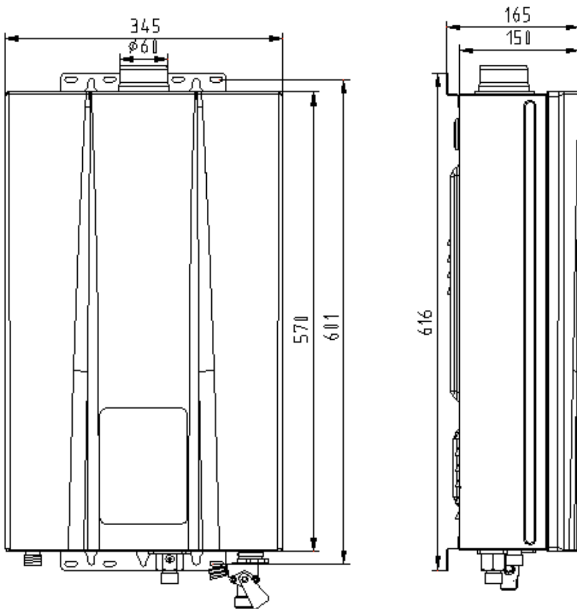
Fig. 2 (Unità di misura: mm) (I dati dimensionali sono solo indicativi. Fare riferimento al prodotto effettivo.)
