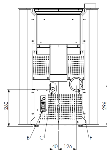
Dimensions du poêle à granulés VISION ERMETICA
