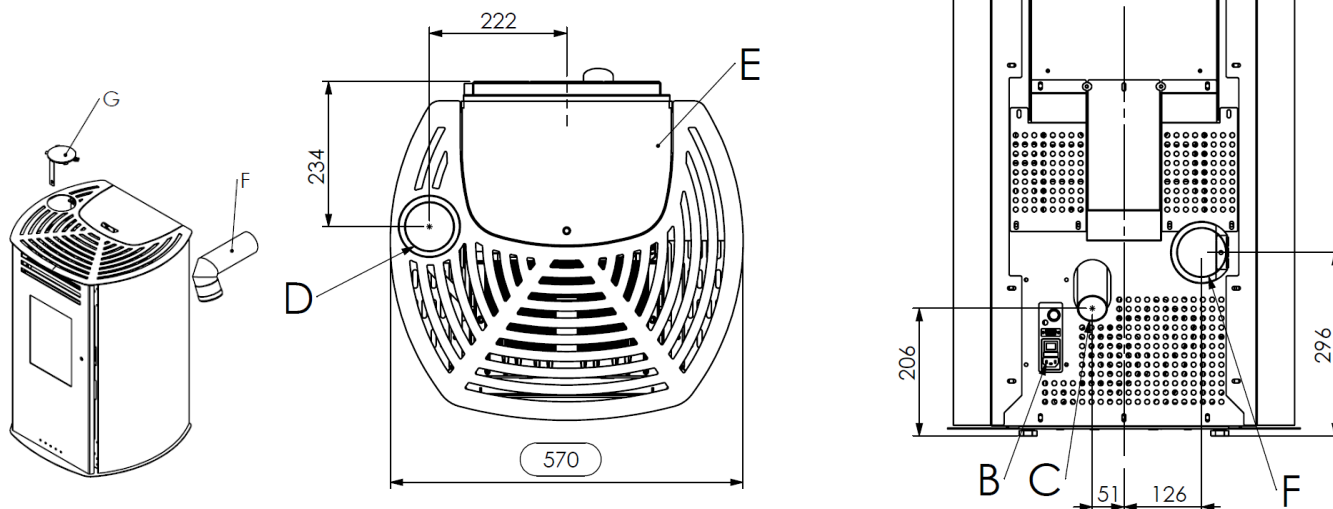
Ingombri stufa pellet VISION ERMETICA
