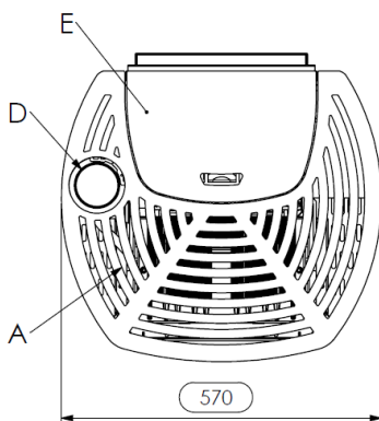
Dimensions du poêle à granulés VISION ERMETICA
