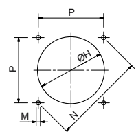
Foratura caldaia consigliata
