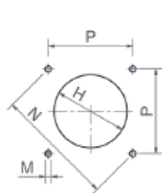
Foratura caldaia consigliata
