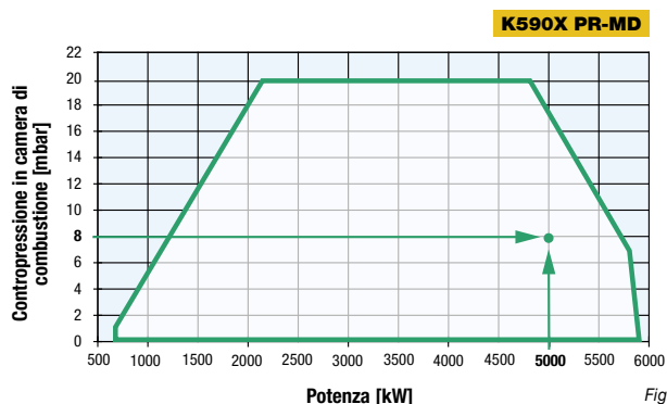
CURVA DI LAVORO DEL BRUCIATORE
