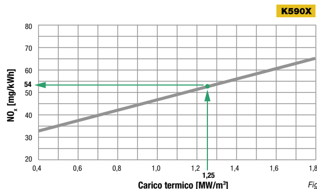
DIAGRAMMA NO x IN RIFERIMENTO AL CARICO TERMICO DELLA CALDAIA
