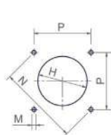
Foratura caldaia consigliata
