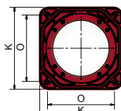
Flangia bruciatore
