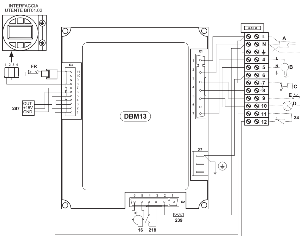
fig. 14 - Schema elettrico
