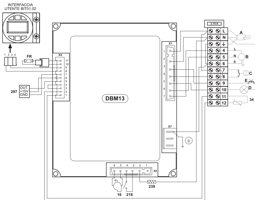
obr. 14 - Elektrické schéma
