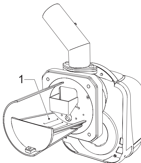
obr. 10 - Rošt hořáku
