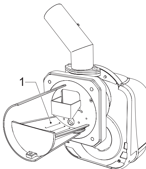
рис. 10 - Решетка горелки
