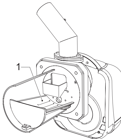
fig. 10 - Burner grille
