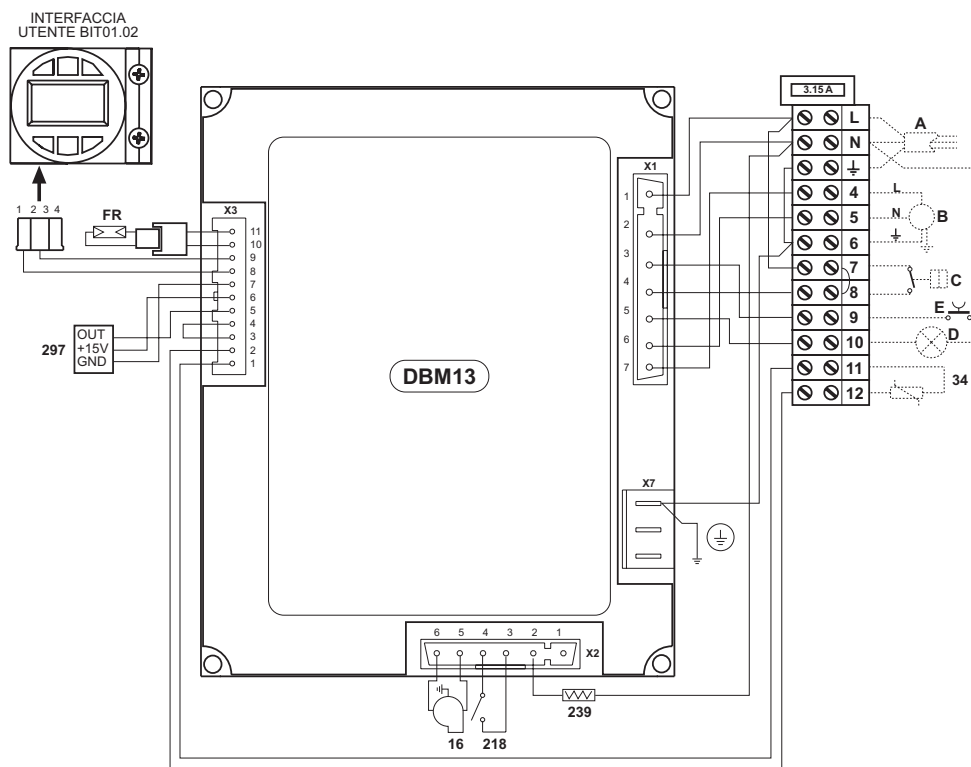
рис. 14 - Электрическая схема
