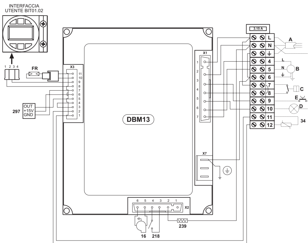
fig. 14 - Wiring diagram
