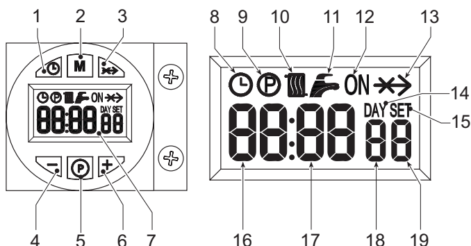
obr. 1 - Ovládací panel
