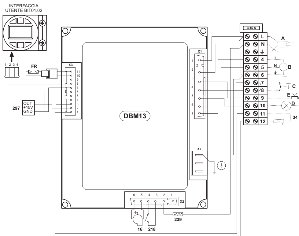
obr. 14 - Elektrická schéma
