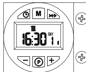
рис. 2 - Индикация во время работы горелки
