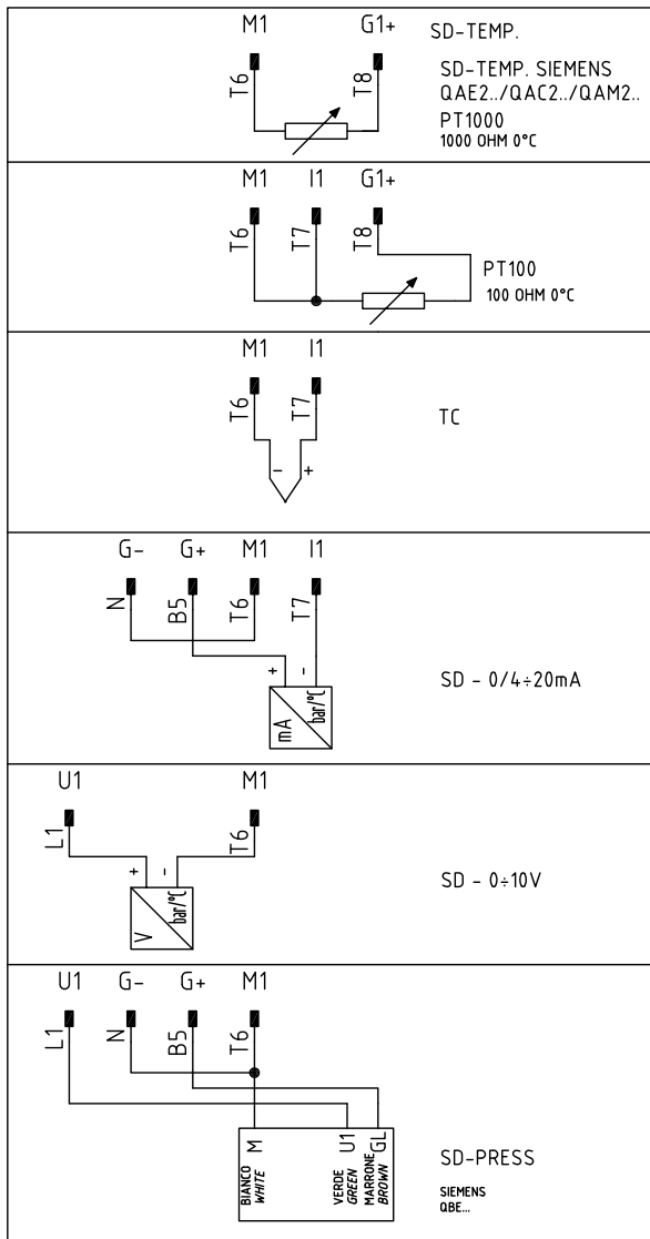
Fig. 29 - Collegamento sonde
