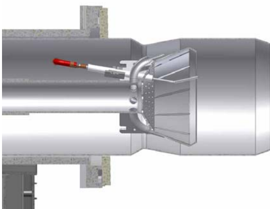
Fig. 36 - Testa tutta in avanti
