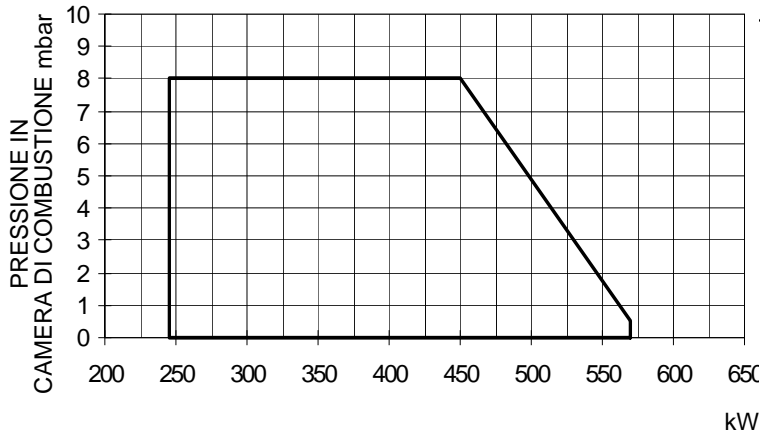
EM49 LN Bruciatore Low NOx
