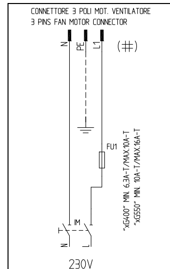
Fig. 28 - Connettore 3 poli per motore elettrico
