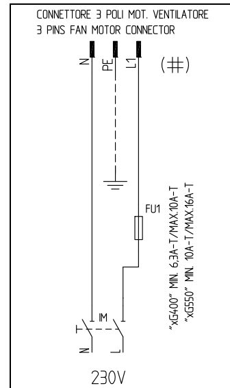
Fig. 26 - Connettore 3 poli motore elettrico
