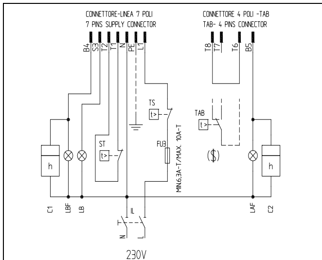
Fig. 27 - Connettori a 7 e a 4 poli
