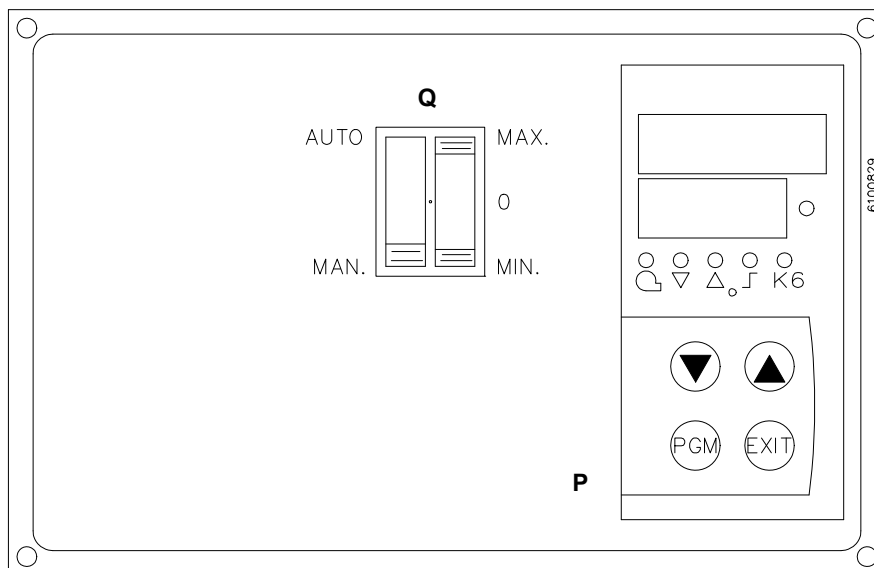
Fig. 40 - Solo bruciatori modulanti
