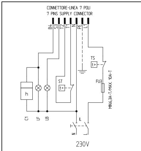
Fig. 25 - Connettore 7 poli
