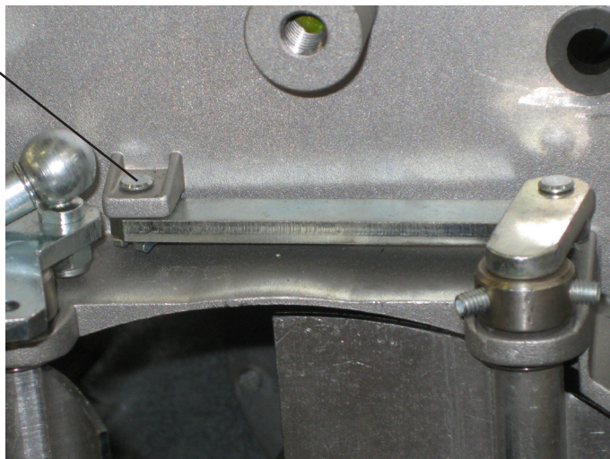
F Vista della serranda destra bloccata
