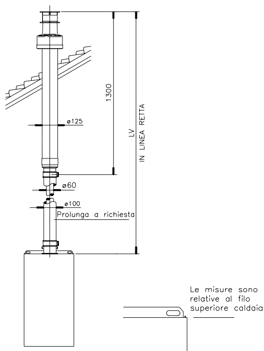
SISTEMA COASSIALE VERTICALE
