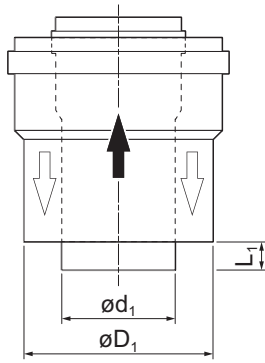
Fig.14 Dimensioni del collegamento concentrico
