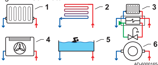
Fig.21 Utilizzatori
