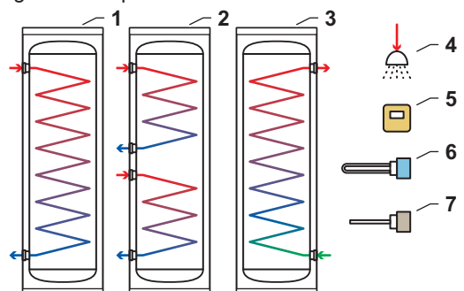
Fig.22 Acqua calda sanitaria
