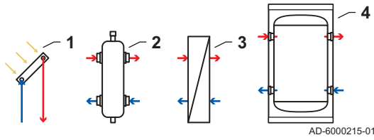
Fig.23 Separatore idraulico
