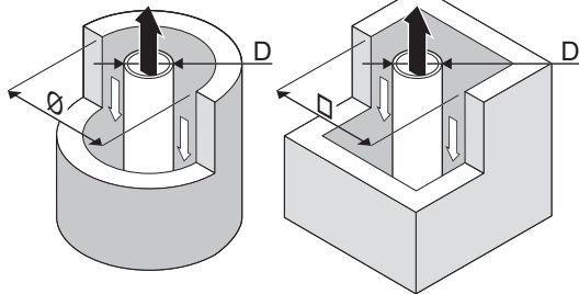
Fig.10 Dimensioni minime della canna fumaria o del condotto C 93
