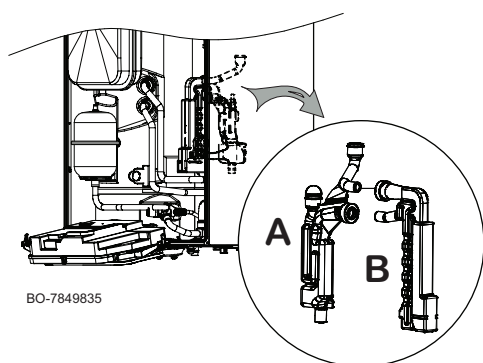
Fig.70 Smontaggio del sifone
