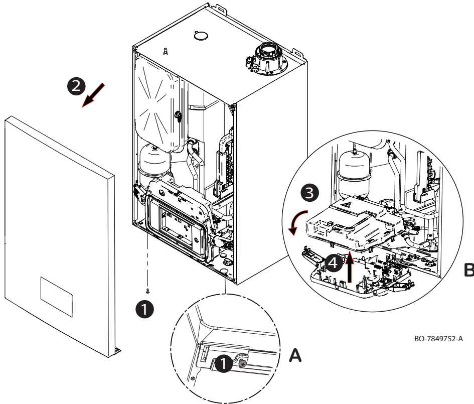
Fig.48 Accesso ai collegamenti elettrici
