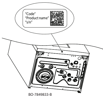
Fig.33 Etichetta Service
