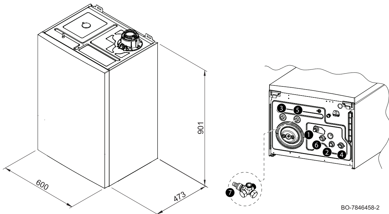
Fig.25 Dimensioni e collegamenti
