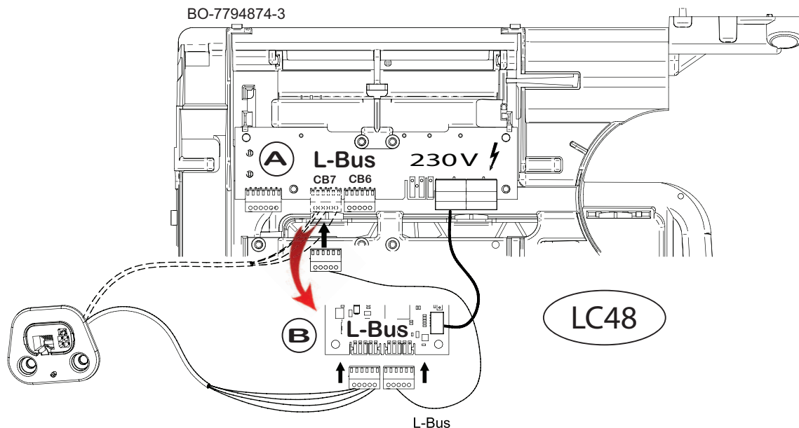
Fig.52 Collegamento scheda accessoria in caldaia
