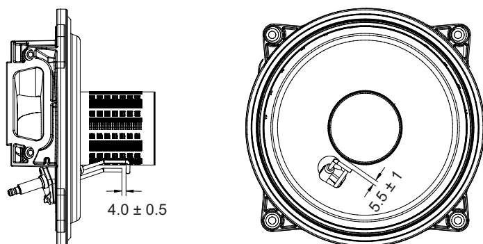
Fig.71 Distanze elettrodo
