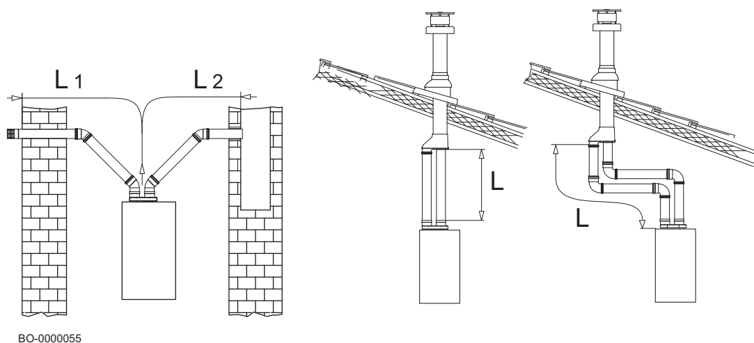
Fig.47 Esempi installazioni condotti separati
