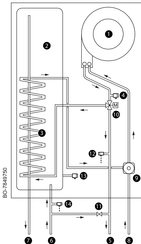
Fig.28 Schema di principio
