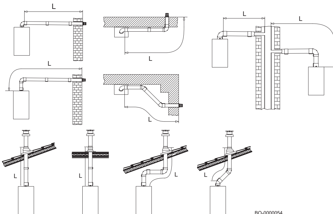
Fig.44 Esempi installazioni condotti coassiali
