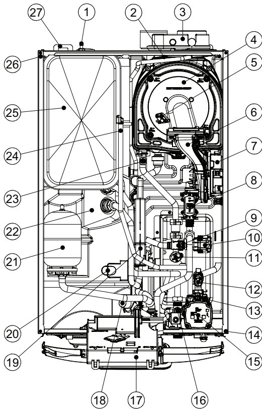
Fig.29 Descrizione componenti
