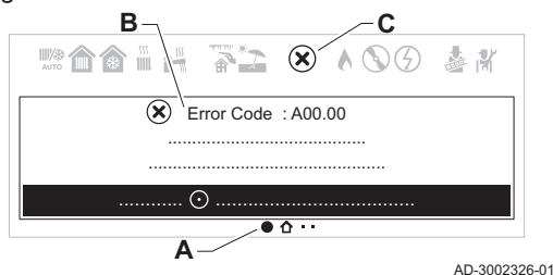
Fig.73 Visualizzazione codice di anomalia
