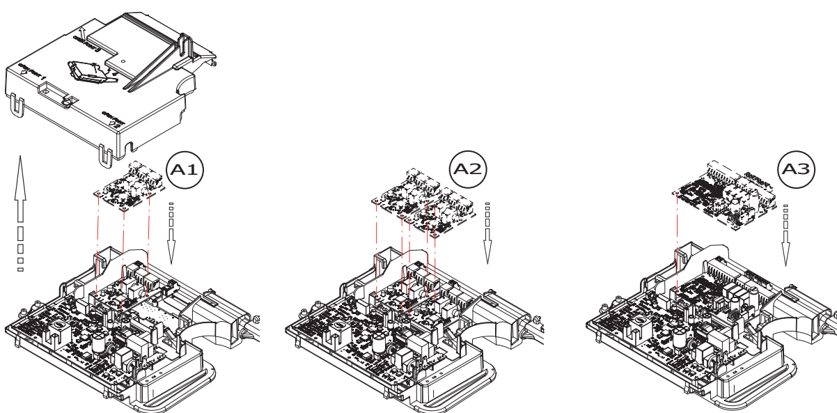
Fig.51 Posizionamento e fissaggio schede accessorie in caldaia
