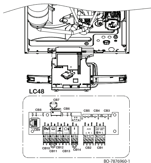
Fig.49 Collegamenti scheda di caldaia
