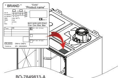
Fig.32 Targa matricola
