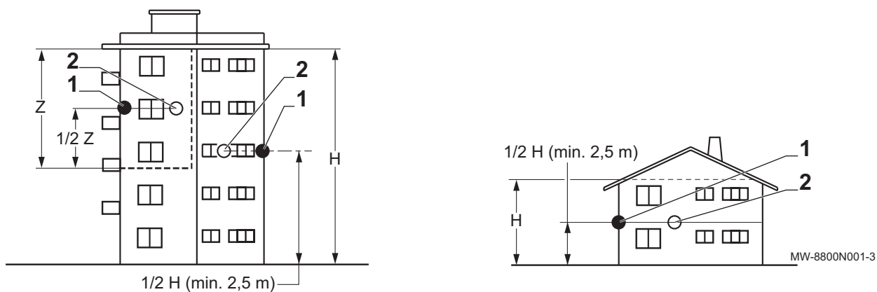
Fig.36 Ubicazioni consigliate A
