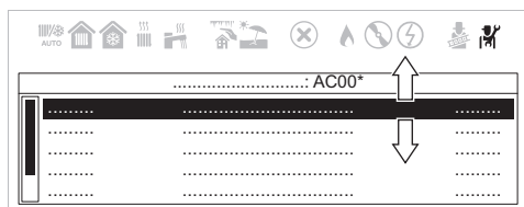
Fig.61 Risultati della ricerca di punti dati
