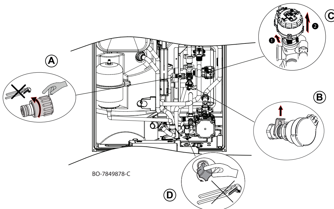
Fig.72 Componenti principale gruppo idraulico
