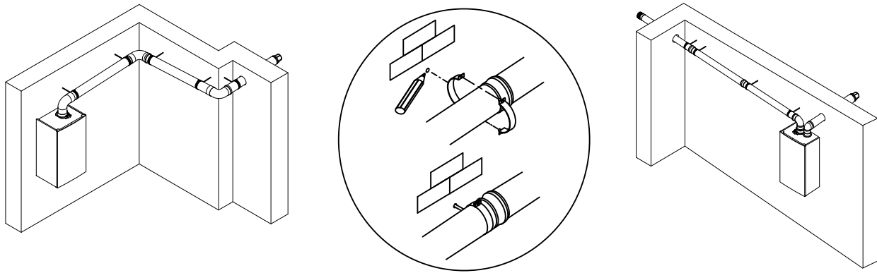
Fig.39 Modalità di fissaggio a muro dei condotti
