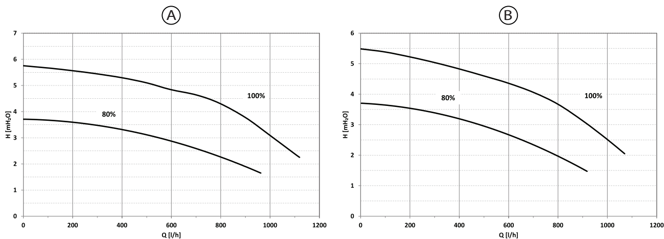
Fig.30 Grafico portata/prevalenza alla placca
