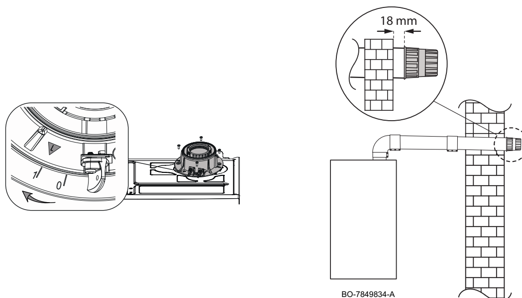
Fig.41 Installazione raccordo coassiale
