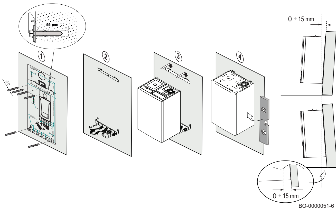
Fig.35 Installazione a parete dell'accessorio
