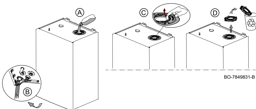
Fig.38 Modalità di riempimento del sifone
