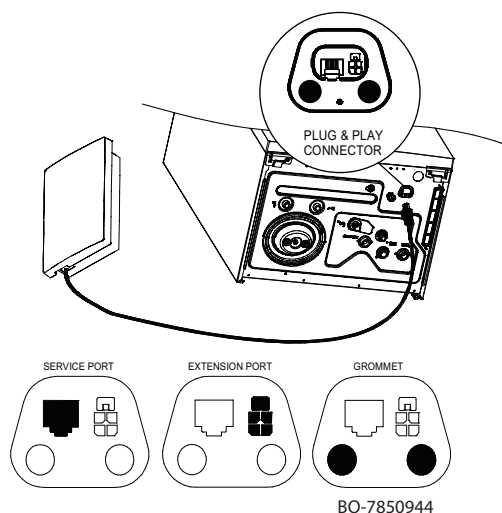
Fig.50 Posizione del connettore
