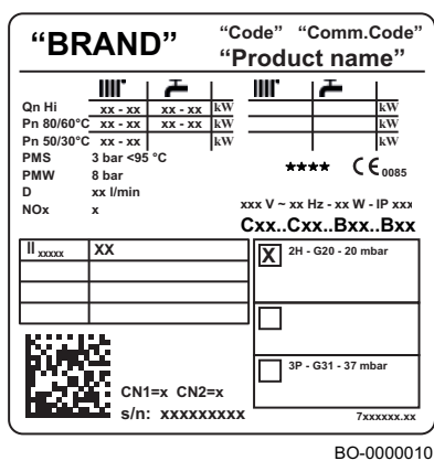
Fig.32 Targa matricola
