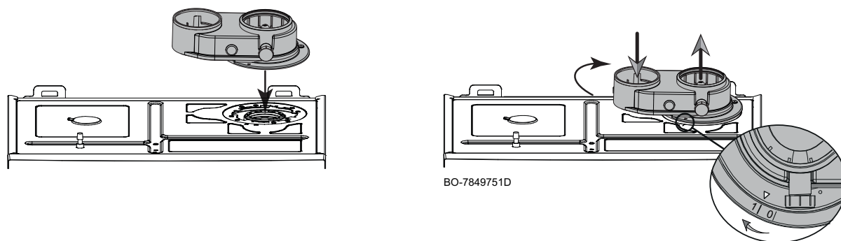
Fig.46 Installazione raccordo per condotti separati
