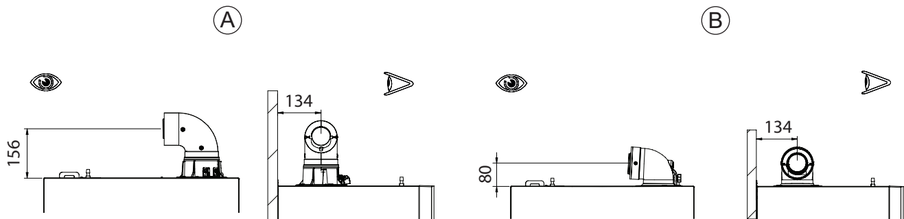
Fig.42 Tipo di scarico-aspirazione coassiale
