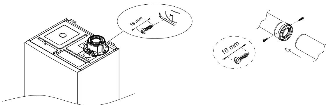
Fig.43 Fissaggio torretta fumi coassiale
