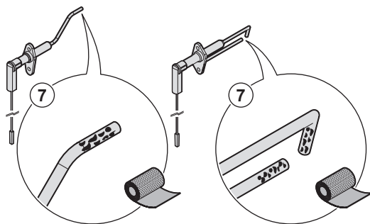
Fig.40 Pulizia degli elettrodi
