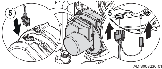
Fig.50 Montaggio dei connettori elettrici del ventilatore
