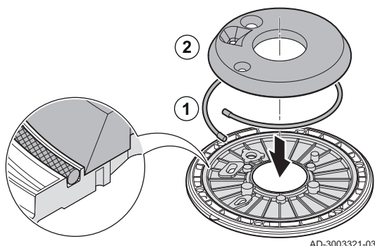
Fig.46 Posizionamento dell'isolamento del bruciatore e della guarnizione di tenuta a cavo in fibra di vetro
