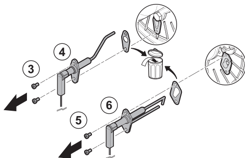
Fig.39 Rimozione degli elettrodi
