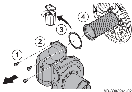
Fig.42 Rimozione del bruciatore nei tipi di caldaia 1.35 - 1.50 - 1.60 - 1.70.
