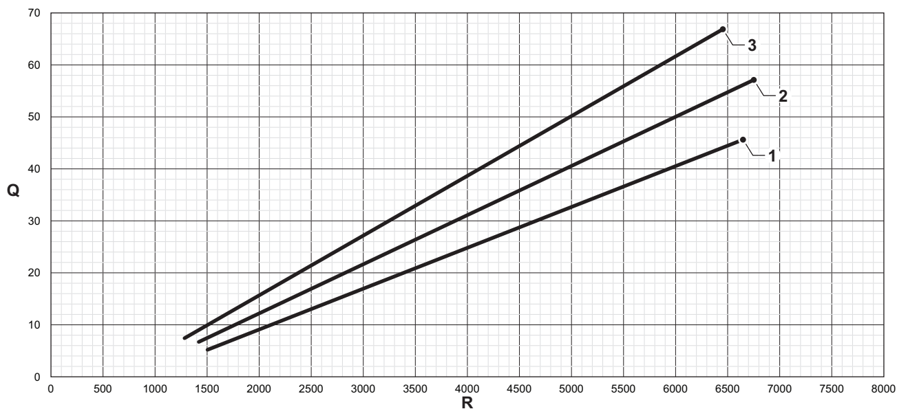
Fig.15 Potenza massima per riscaldamento
