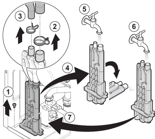
Fig.30 Pulizia del sifone
