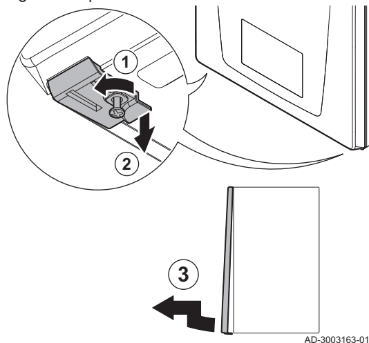
Fig.27 Apertura della caldaia
