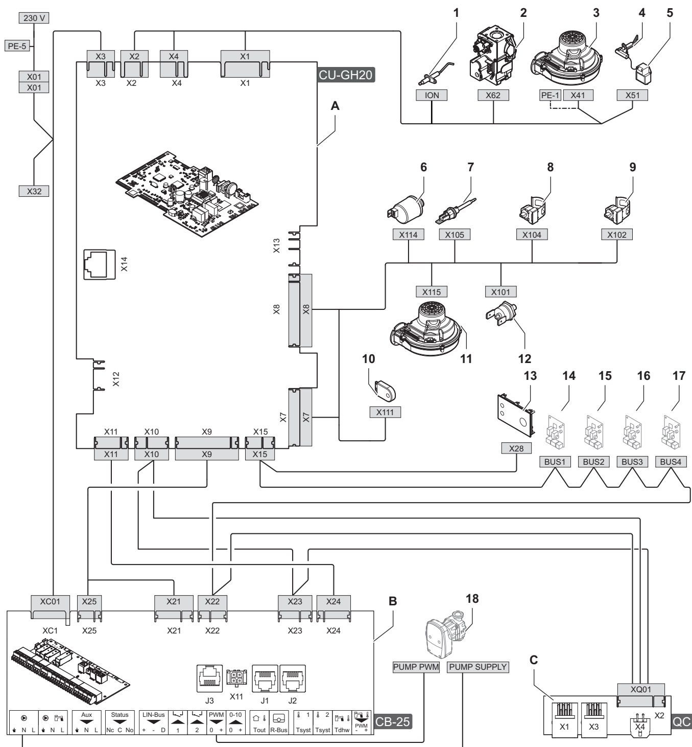
Fig.57 Schema elettrico per i tipi di caldaia 1.35 - 1.50 - 1.60 - 1.70
