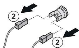
Fig.33 Rimozione del cavo di ionizzazione
