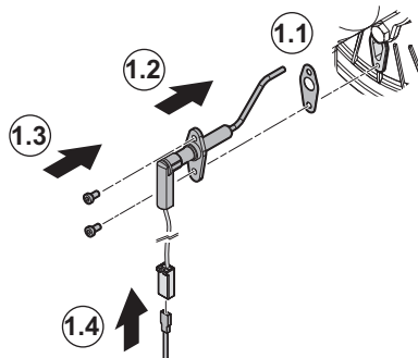
Fig.52 Montaggio dell'elettrodo di ionizzazione e accensione
