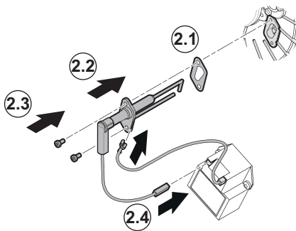
Fig.52 Montaggio dell'elettrodo di ionizzazione e accensione
