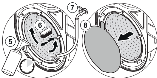
Fig.45 Pulizia dello scambiatore di calore
