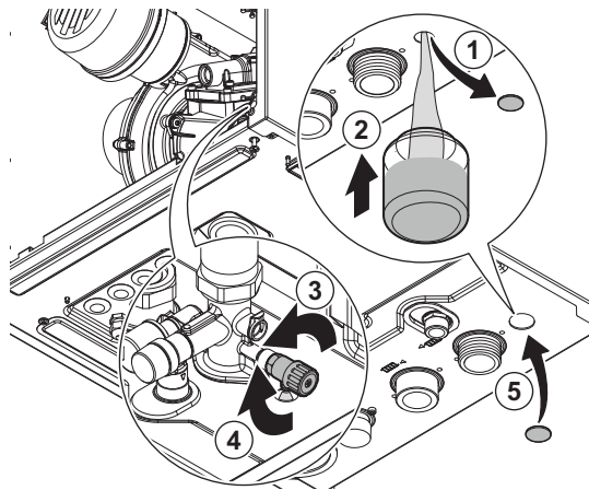
Fig.29 Aprire la valvola di scarico scambiatore di calore
