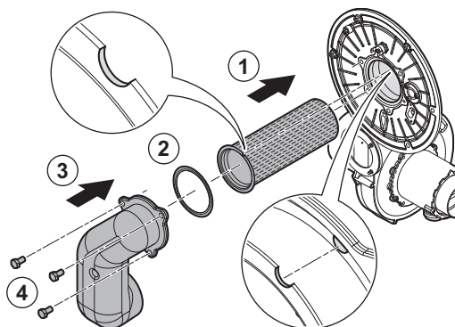
Fig.47 Montaggio del bruciatore nei tipi di caldaia 1.35 - 1.50 - 1.60 - 1.70.
