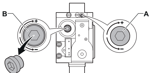
Fig.26 Valvola di controllo gas nei tipi di caldaia: 1.35 - 1.50 - 1.60 - 1.70
