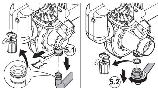
Fig.35 rimozione del tubo del gas dal Venturi
