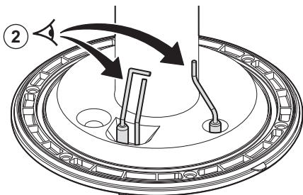
Fig.38 Controllo delle condizioni dell'elettrodo di ionizzazione e accensione
