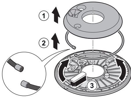
Fig.43 Rimozione dell'isolamento del bruciatore
