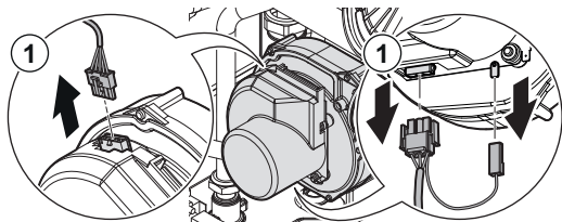
Fig.31 Rimozione dei connettori elettrici dal ventilatore
