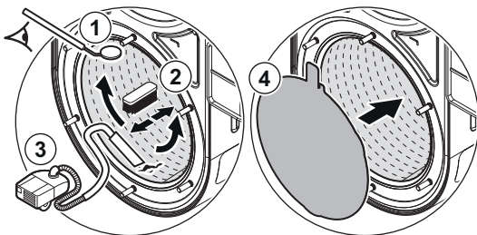
Fig.44 Pulizia con spazzolino e aspirapolvere dello scambiatore di calore
