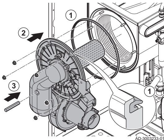
Fig.48 Montaggio dell'unità piastra anteriore
