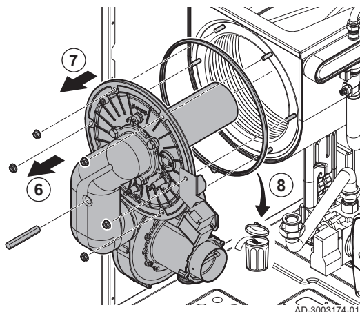
Fig.36 Rimozione dell'unità piastra anteriore
