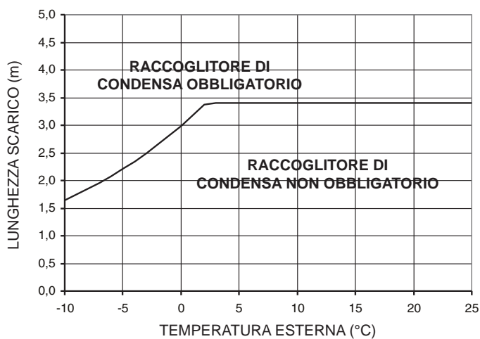
Lunghezza massima condotti coassiali ø 60-100 26 MICROMIX AR
