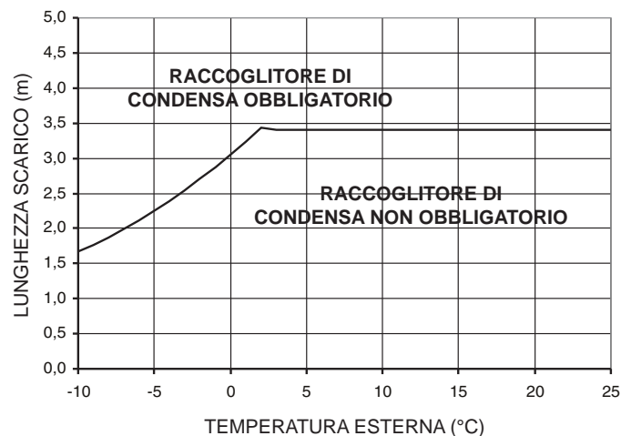
Lunghezza massima condotti coassiali ø 60-100 32 MICROMIX AR
