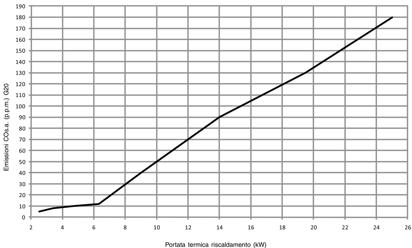
Curva portata termica - emissioni (Qnrisc) - 25 HE
