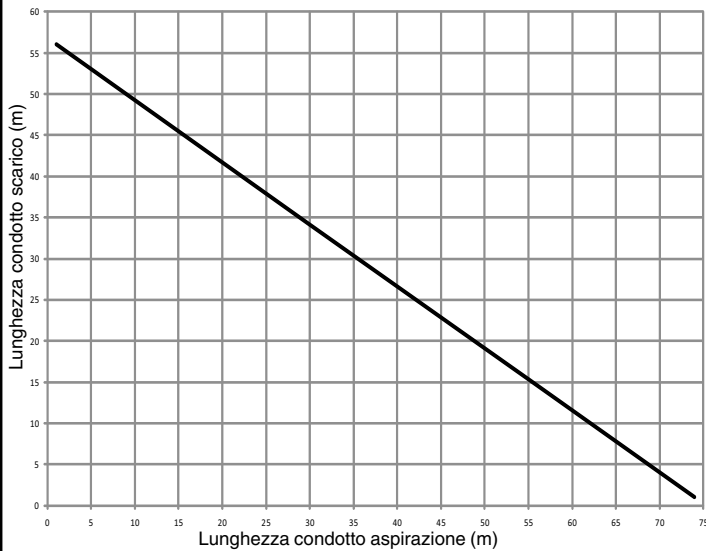
LUNGHEZZA MASSIMA TUBI Ø 80 - 25 HE
