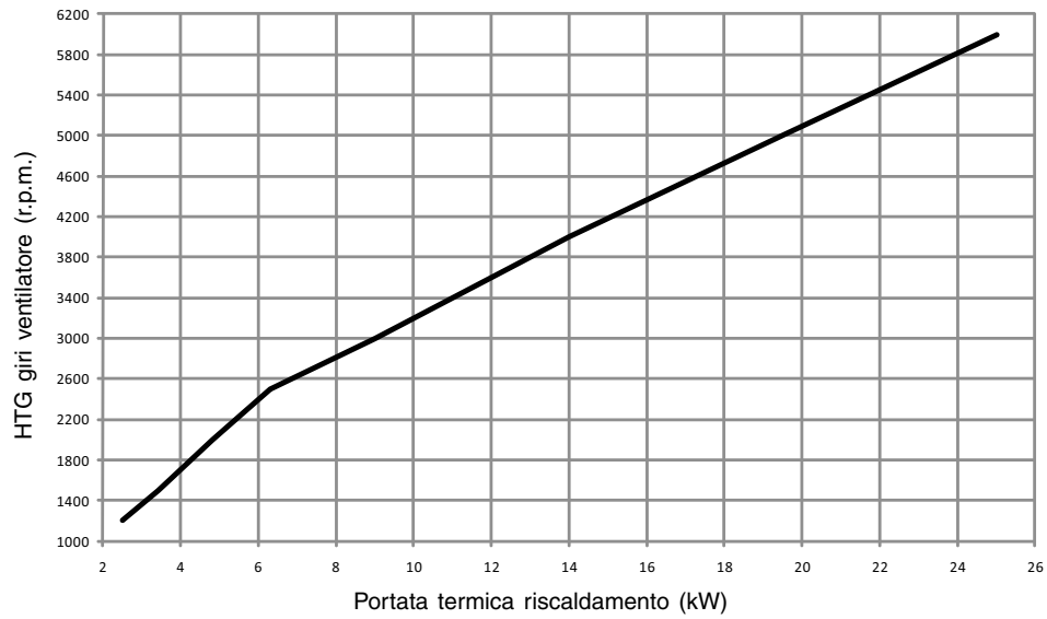
Curva portata termica - nr. giri ventilatore (Qnrisc) - 25 HE
