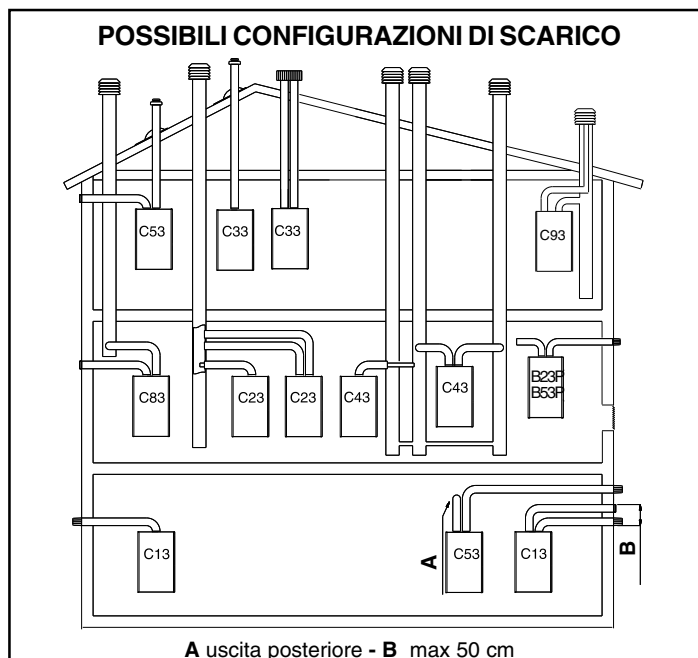
A uscita posteriore - B max 50 cm
