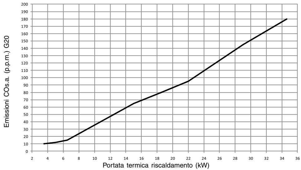
Curva portata termica - emissioni (Qnrisc) - 35 HE
