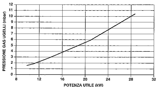
REGOLAZIONE POTENZA RISCALDAMENTO (G 20) Idra Exclusive turbo e s i 24
