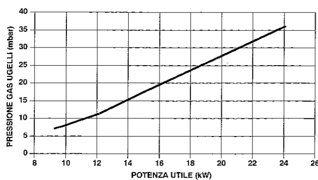
REGOLAZIONE POTENZA RISCALDAMENTO (G 31) Idra Exclusive turbo e s i 20
