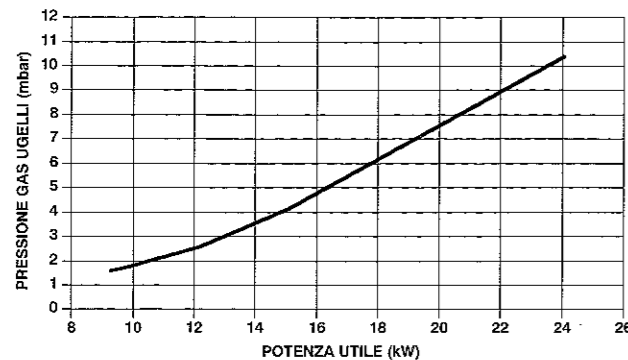
REGOLAZIONE POTENZA RISCALDAMENTO (G 20) Idra Exclusive turbo e s i 20
