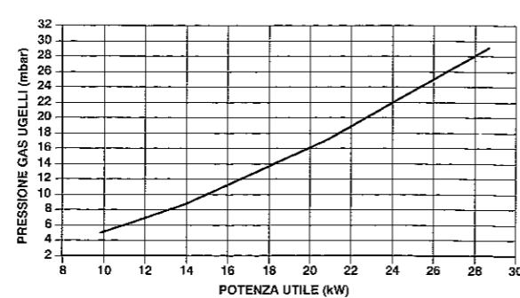
REGOLAZIONE POTENZA RISCALDAMENTO (G 31) Idra Exclusive turbo e s i 24
