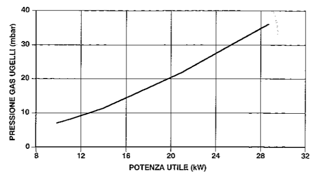
REGOLAZIONE POTENZA RISCALDAMENTO (G 31) Idra Exclusive turbo e s i 24
