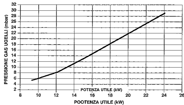
REGOLAZIONE POTENZA RISCALDAMENTO (G 30) Idra Exclusive turbo e s i 20
