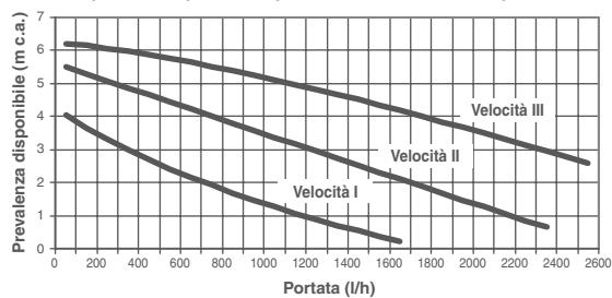
Gráfico prevalenza/portata disponibile circolatore ad alta prevalenza
