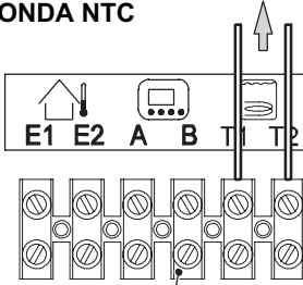
Morsettieria collegamento termostato bollitore / sonda NTC
