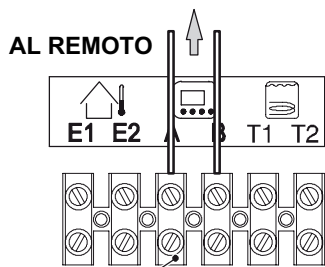
Morsettiera collegamento remoto
