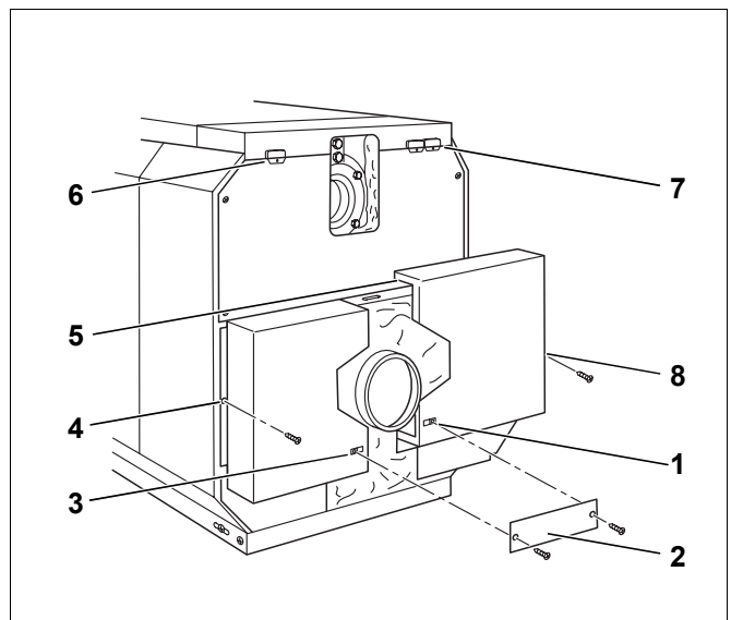
Fig. 56 Montaggio degli elementi del pannello posteriore
