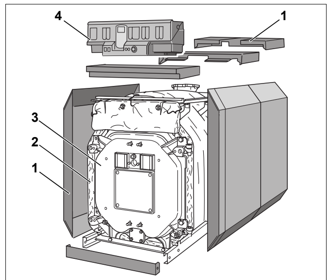
Fig. 1 Caldaia speciale a gasolio/gas Logano GE515
