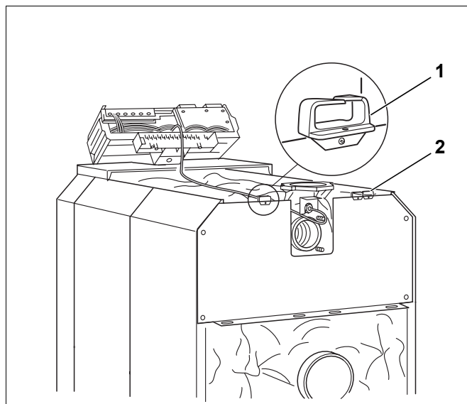
Fig. 63 Collegamenti elettrici
