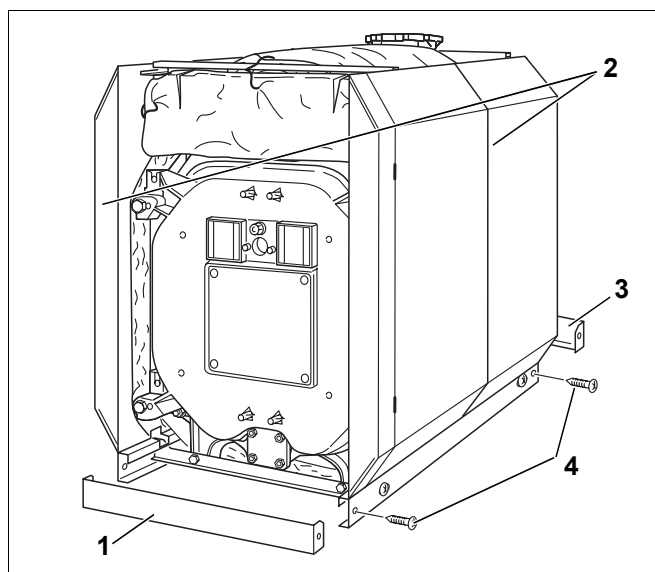
Fig. 51 Montaggio delle guide di zoccolo
