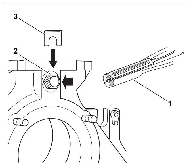
Fig. 62 Montaggio del pacchetto delle sonde di temperatura
