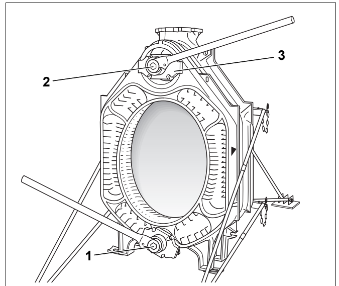
Fig. 19 Utilizzo degli strettoi di montaggio
