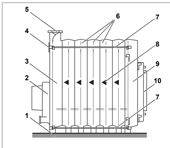
Fig. 8 Blocco caldaia
