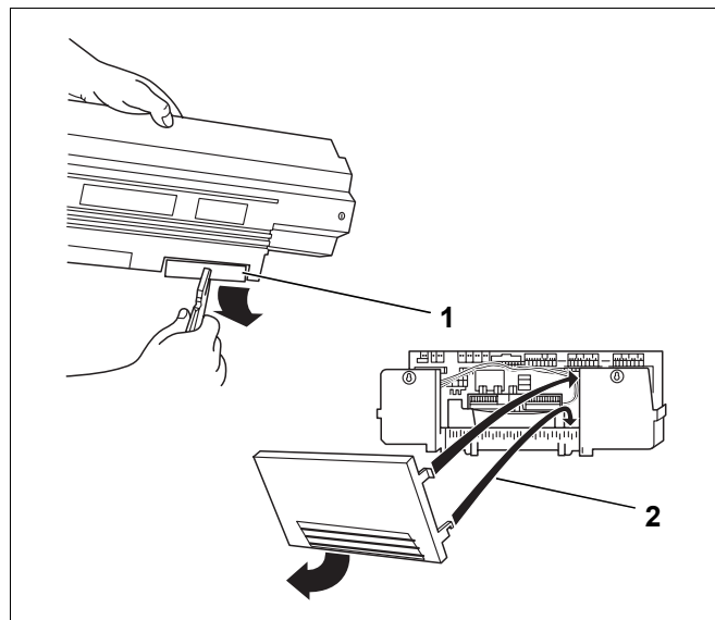
Fig. 61 Preparare il passaggio cavi
