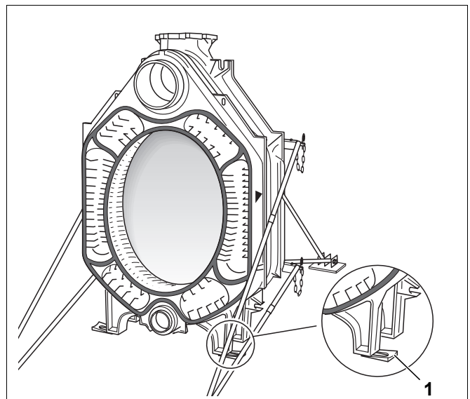
Fig. 21 Utilizzo di cunei di allineamento elementi caldaia
