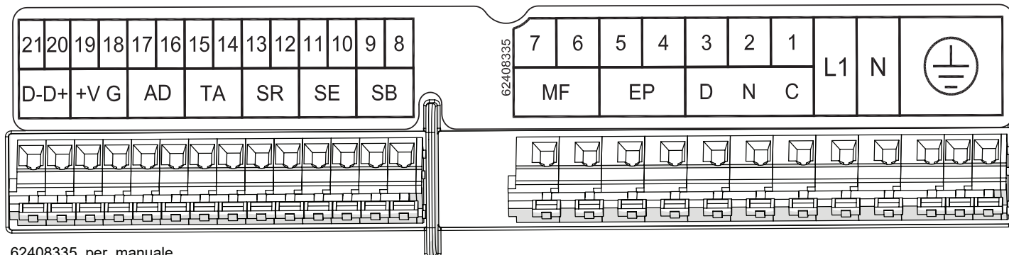
Figura 5-9 - Collegamenti elettrici
