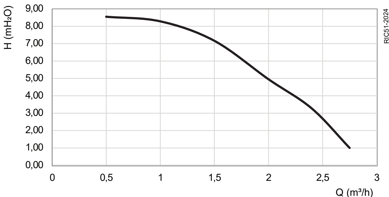
Figura 4-2 - Prevalenza residua
