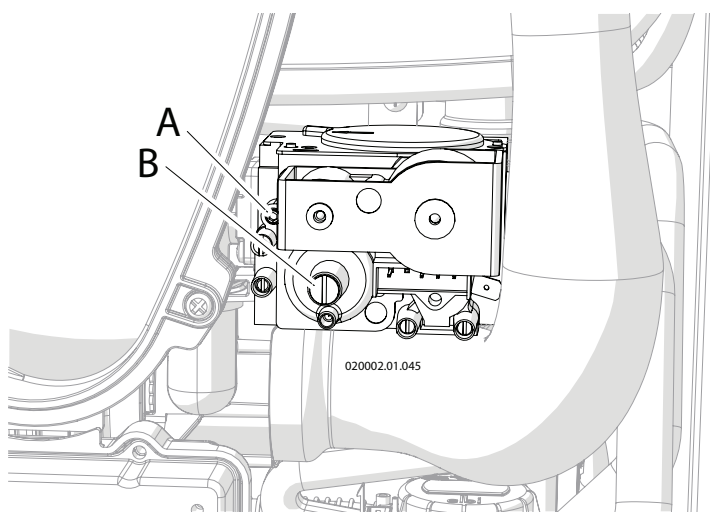
A - Vite di regolazione CO 2 alla massima potenza; B - Vite di regolazione CO 2 alla minima potenza;
