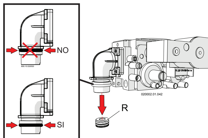
Figura 6-4 - Sostituzione ugello gas
