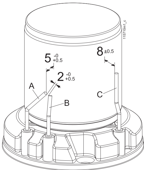
Figura 8-3 - posizionamento elettrodi sul bruciatore
