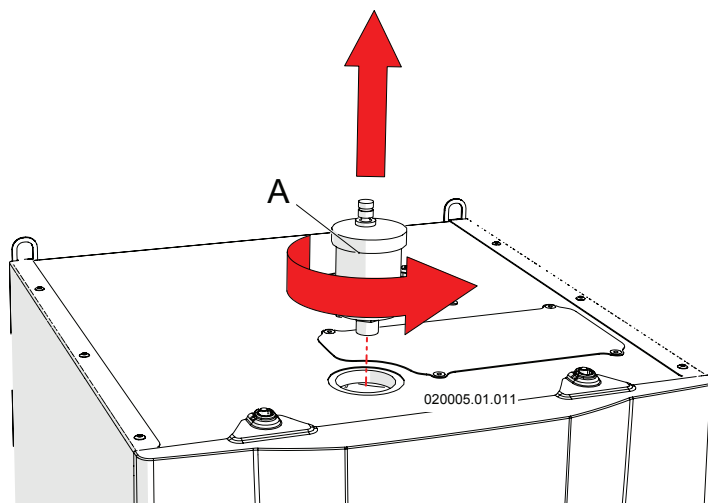
Figura 8-11 - Smontaggio della valvola di sfogo aria
