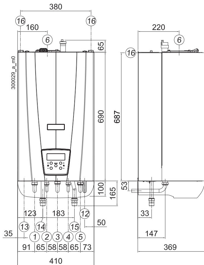
Figura 5-2 - Dimensioni e interassi attacchi
