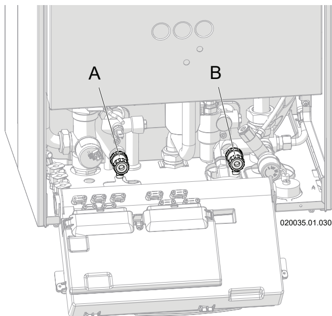
Figura 8-16 - Rubinetti di scarico circuito riscaldamento
