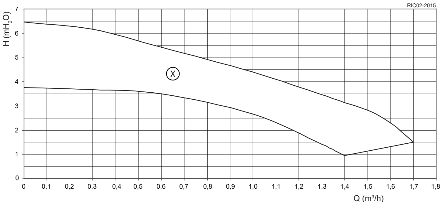
Figura 4-4 - Prevalenza residua con circolatore modulante (di serie)
