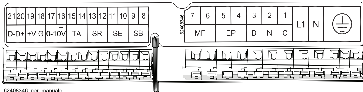
Figura 5-8 - Collegamenti elettrici
