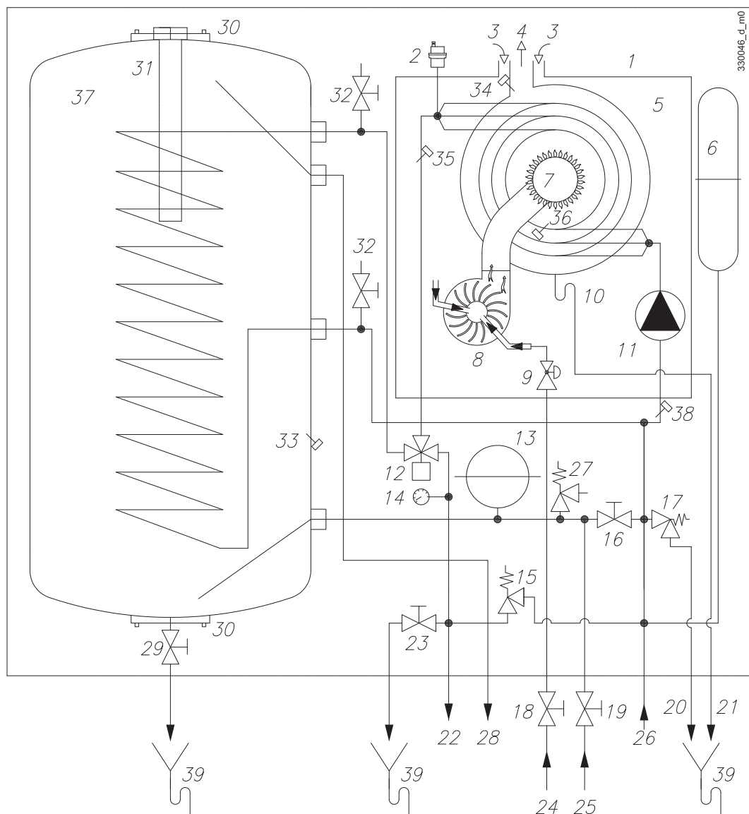
Figura 4-1 - Schema funzionale
