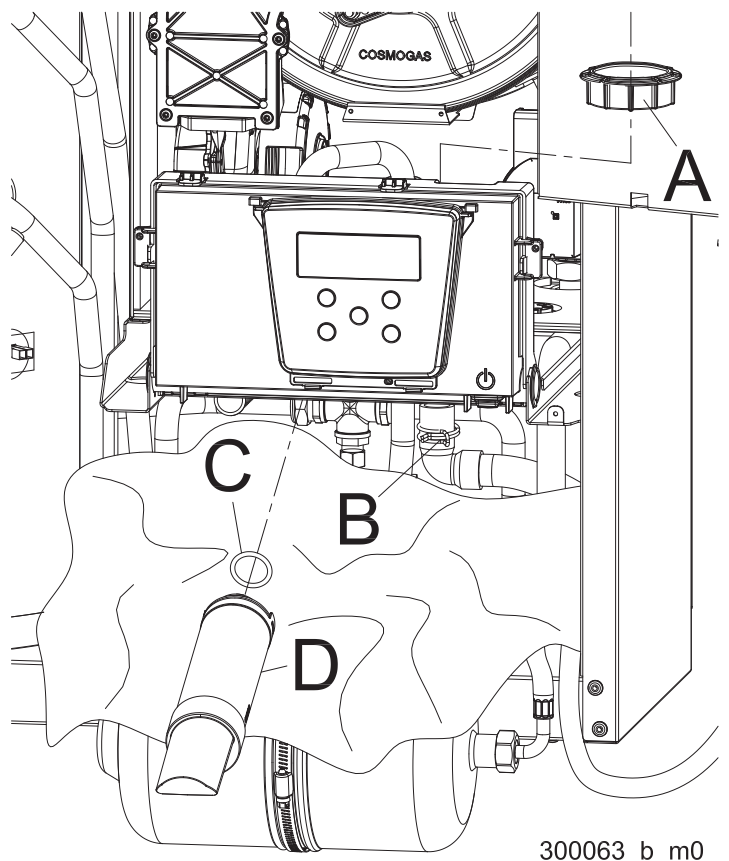
Figura 8-10 - Smontaggio sifone raccogli condensa
