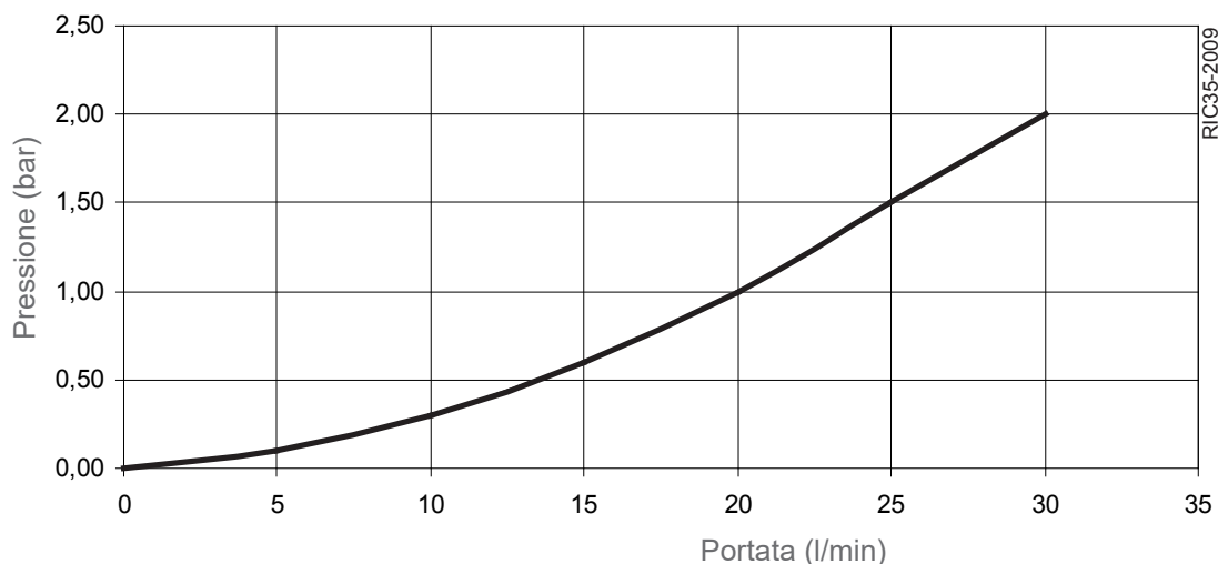
Figura 4-3 - Curva delle perdite del circuito sanitario
