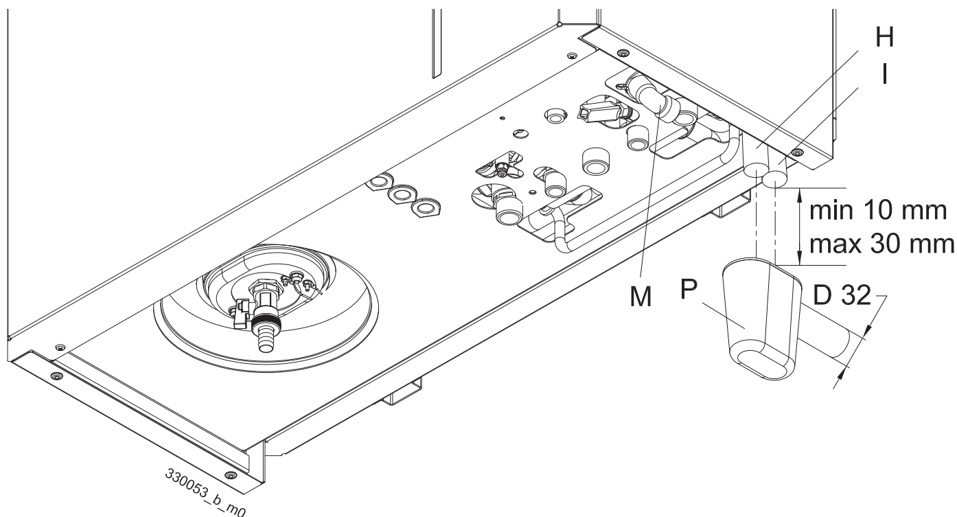
Figura 5-6 - Tubo di scarico condensa
