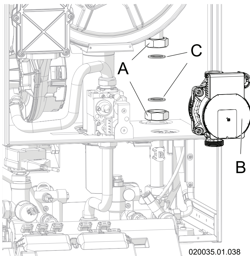
Figura 8-11 - Smontaggio del circolatore
