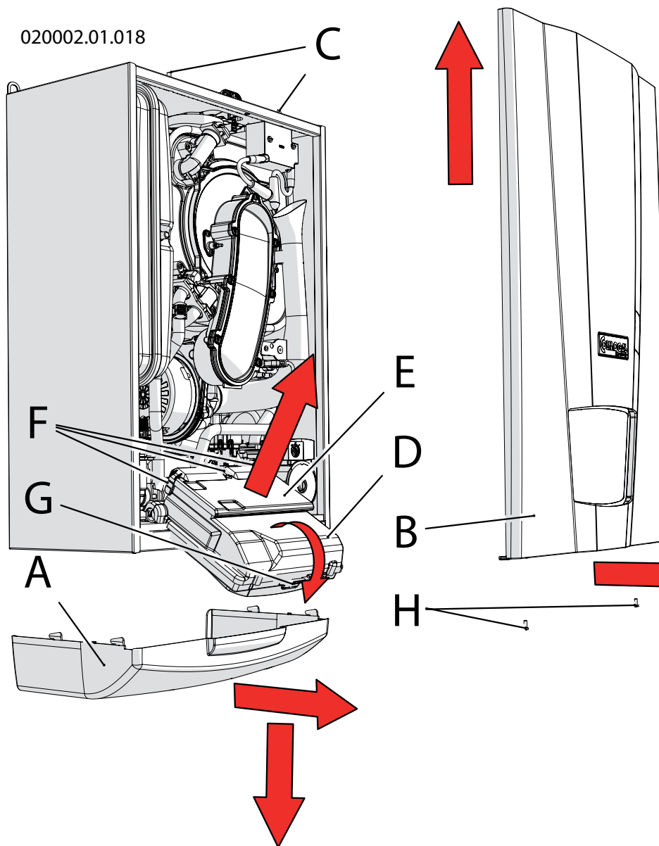
Figura 8.1 - smontaggio mantellatura e apertura quadro comandi
