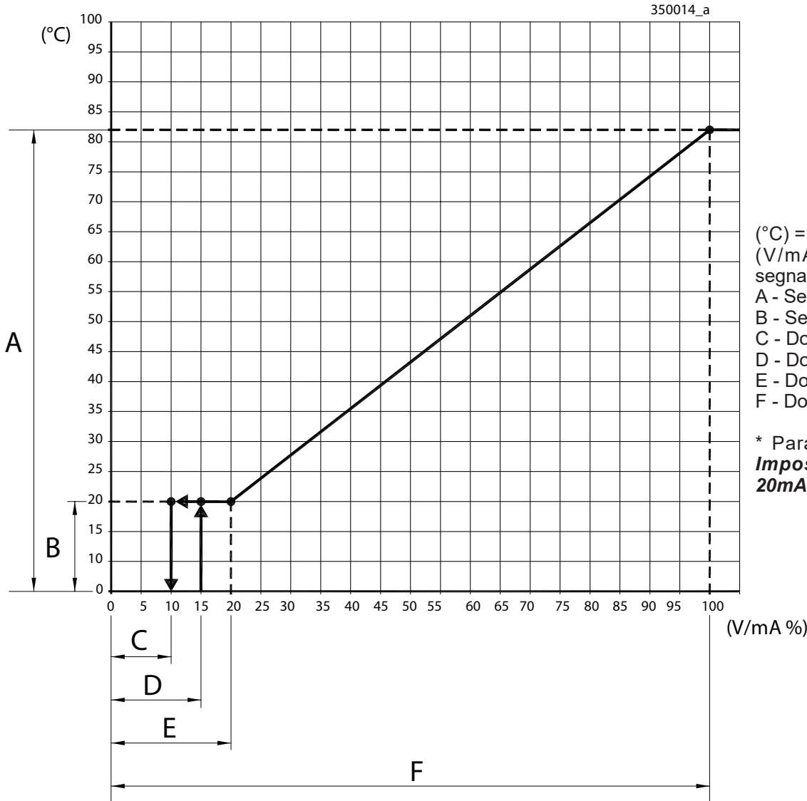
Figura 5-16 - Grafico del controllo della temperatura di setpoint in funzione del segnale 0-10Vdc o 4-20mA
