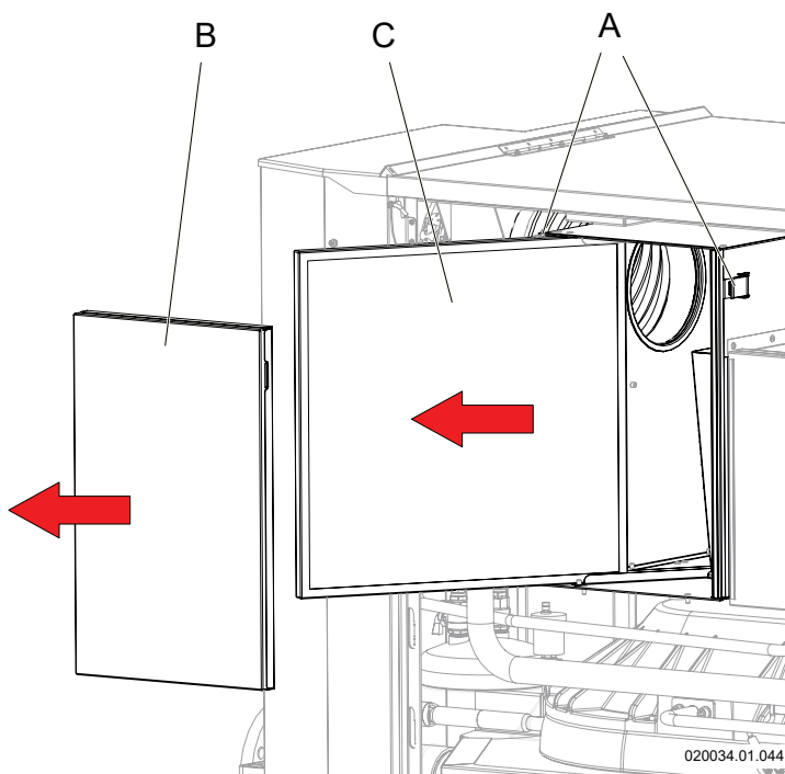
Figura 8-18 - Smontaggio filtro aspirazione aria
