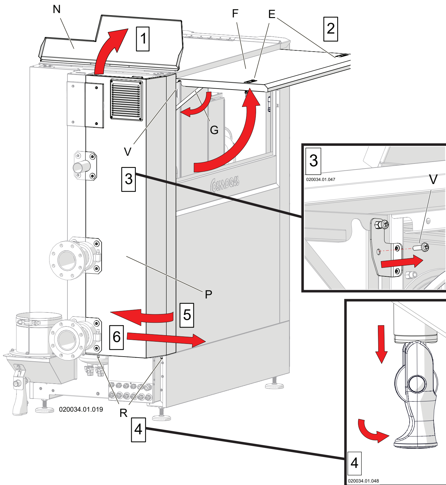
Figura 8-5 - Smontaggio mantello posteriore ed accesso ai componenti interni
