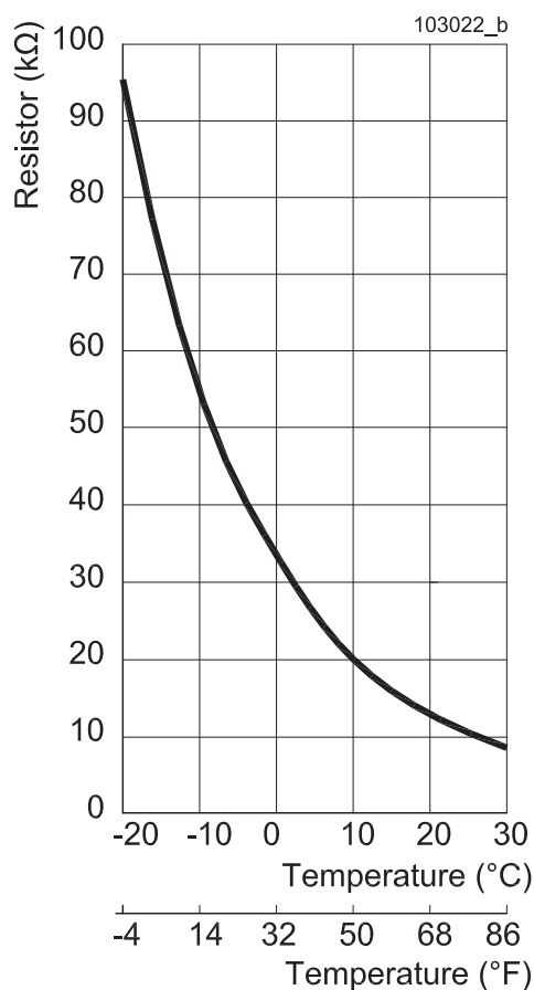
Figura 8-20 - Curva sensore di temperatura esterna
