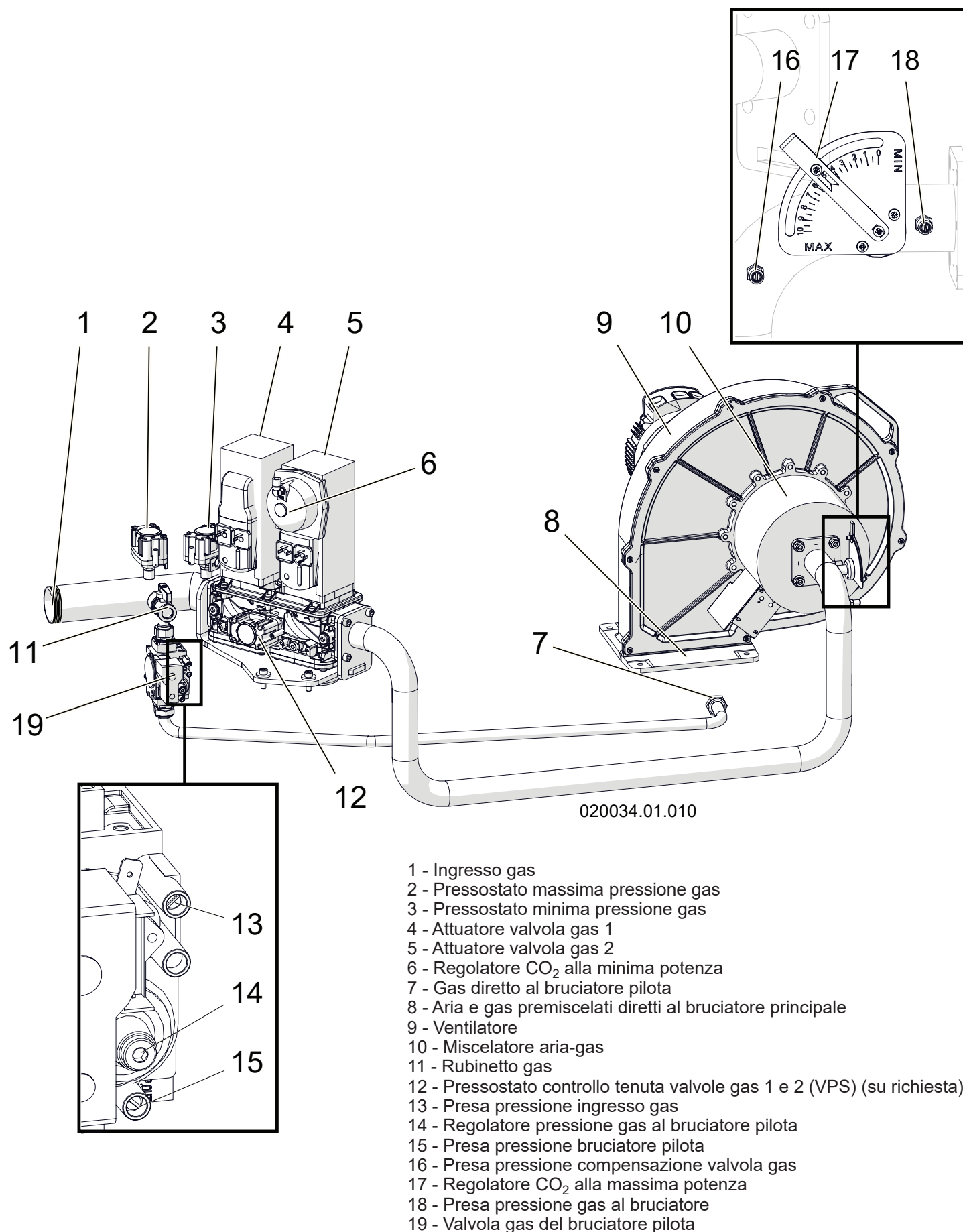
Figura 5-8 - Circuito gas
