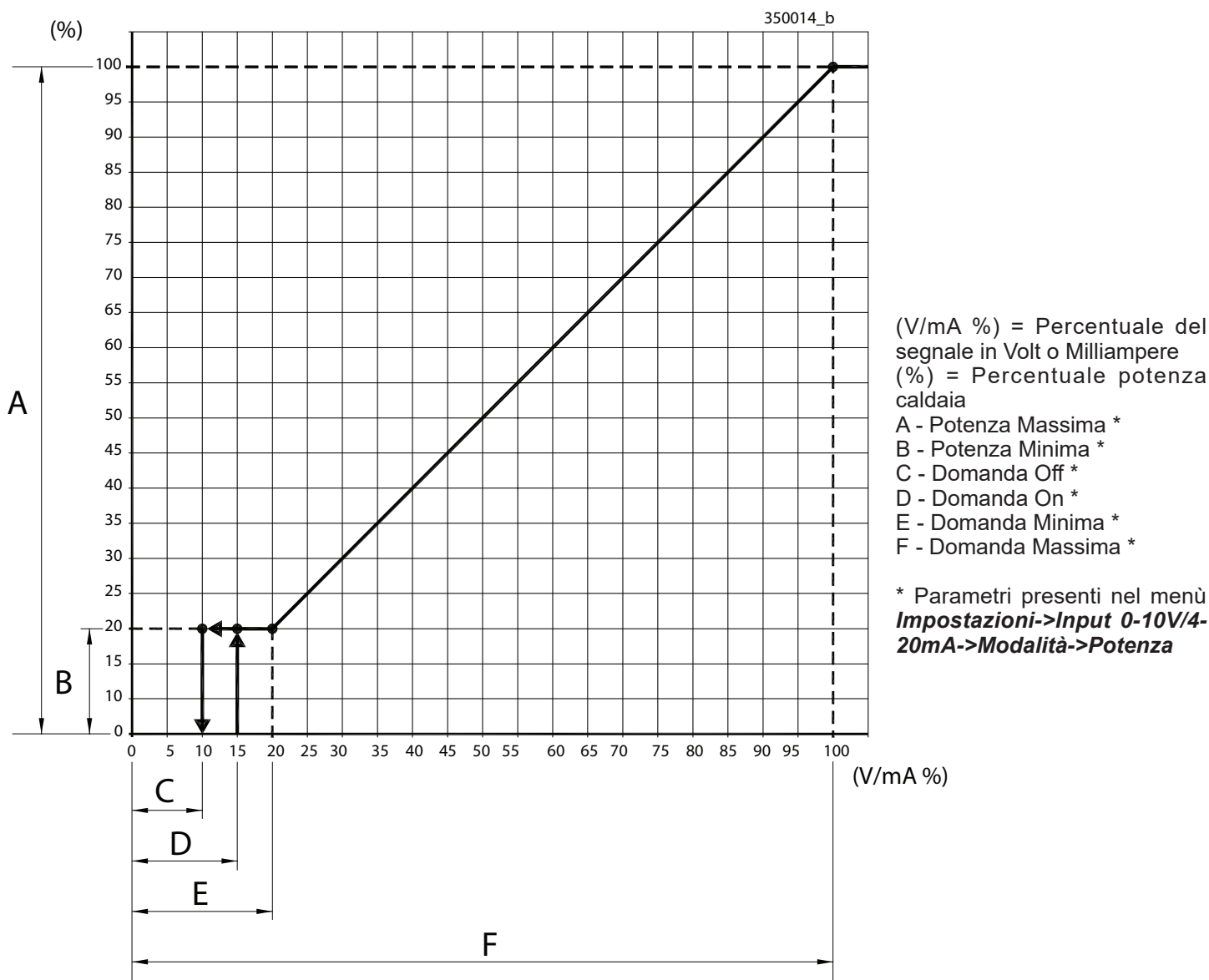
Figura 5-18 - Grafico del controllo della potenza del bruciatore in funzione del segnale 0-10Vdc o 4-20mA
