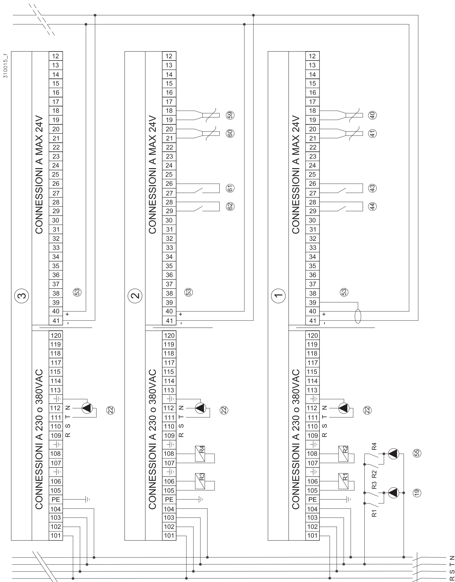
Figura 5-23 - Esempio di collegamento elettrico della cascata con due MASTER
