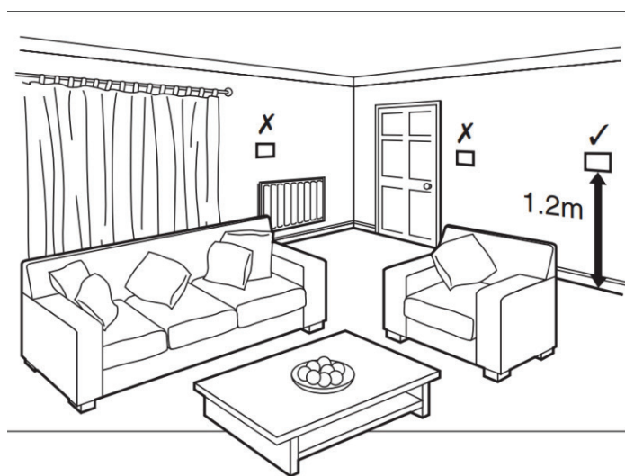
Figura 5-15 - Corretto posizionamento del termostato/cronotermostato
