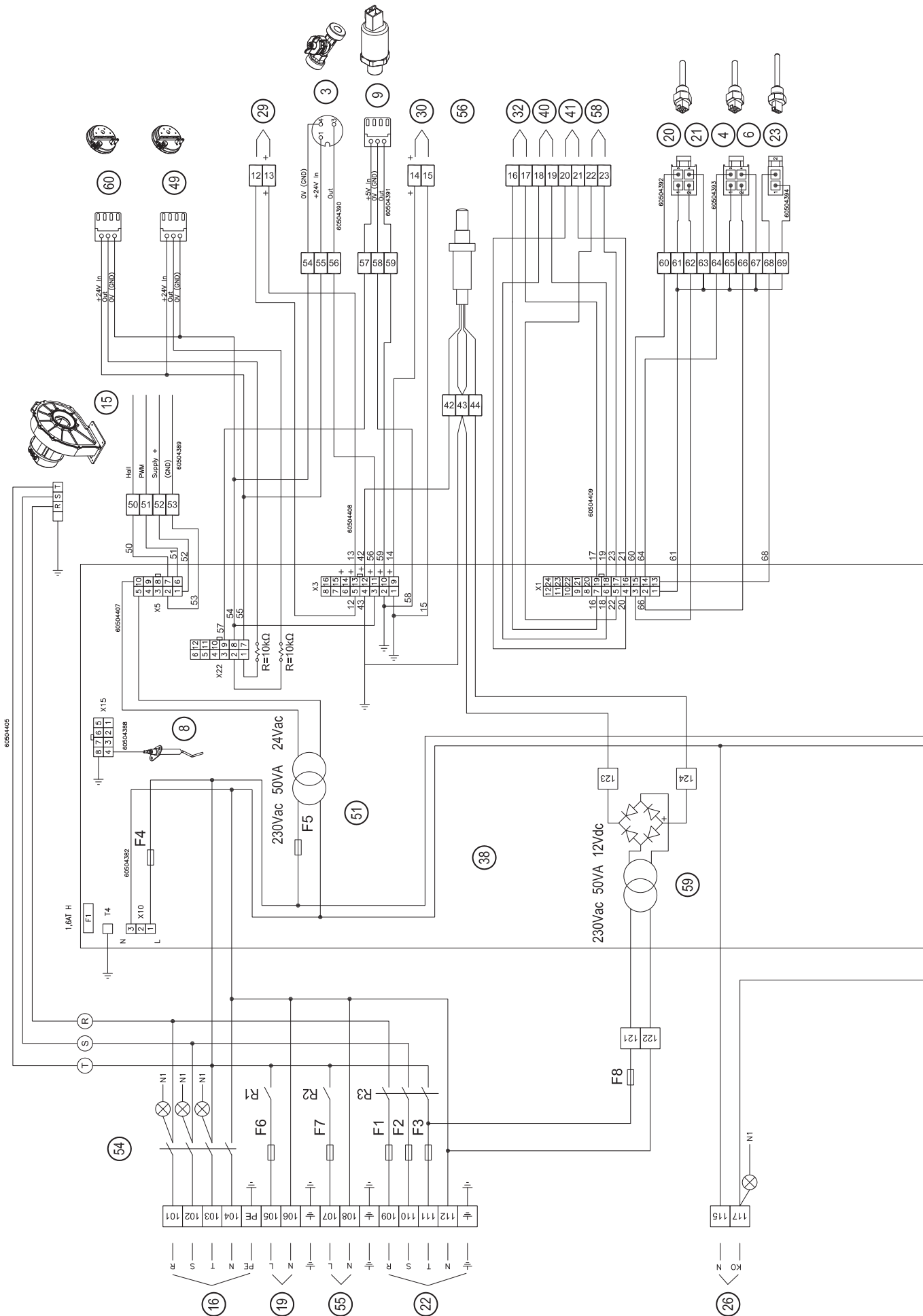
Figura 8-26 - Schema elettrico
