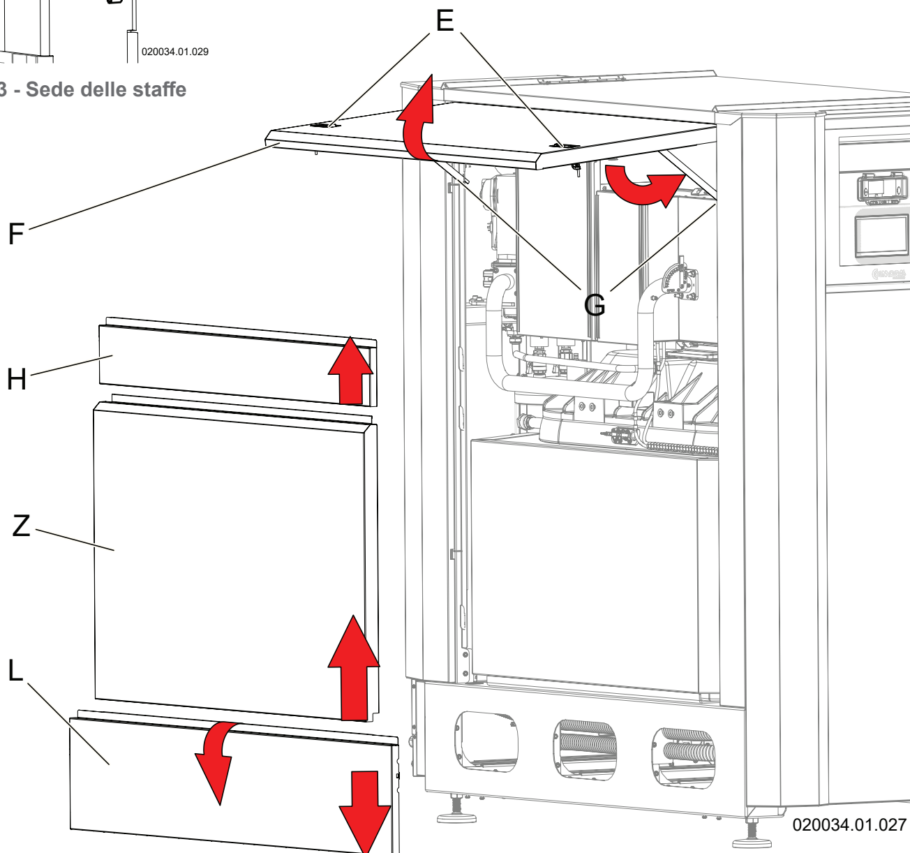
Figura 8-4 - Smontaggio mantello laterale ed accesso ai componenti interni
