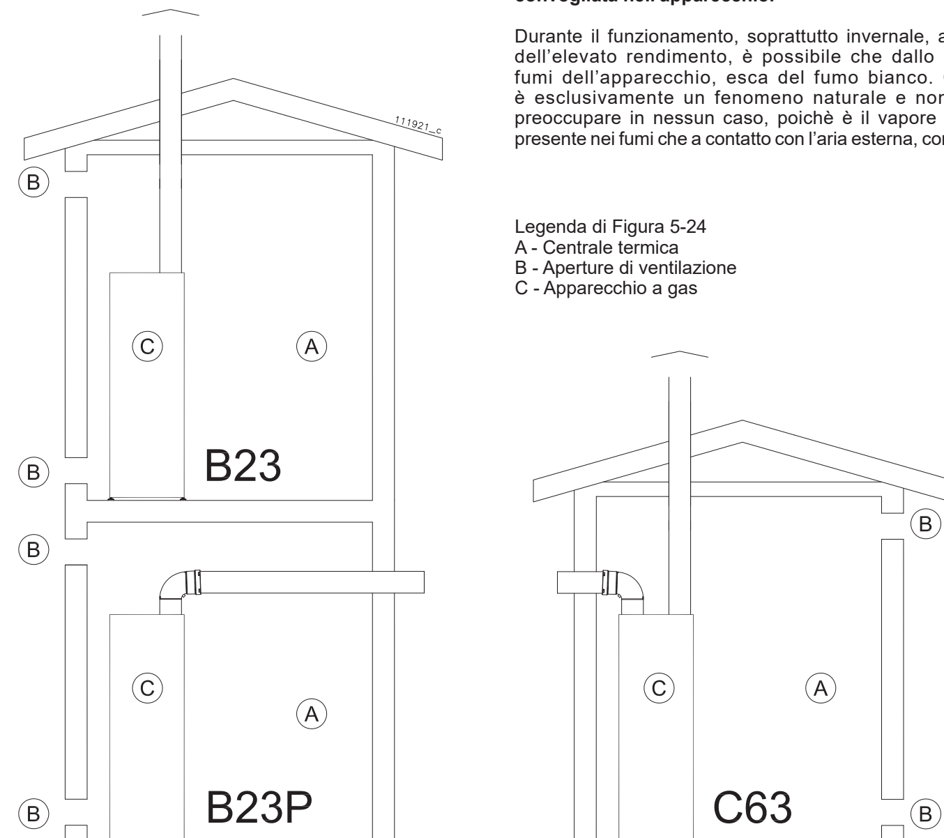
Figura 5-24 - Sistemi di aspirazione/scarico
