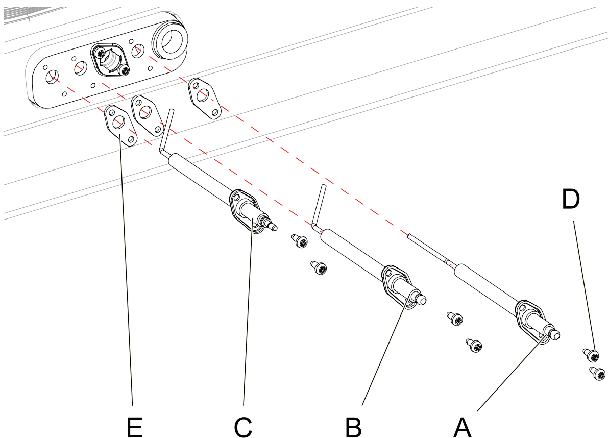
Figura 8-14 - Smontaggio elettrodi di accensione e rilevazione
