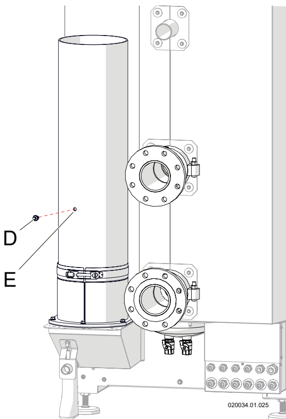
Figura 6-4 - Foro per analisi combustione
