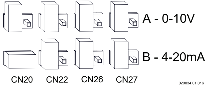
Figura 5-17 - Posizione jumper per segnale esterno 0-10V / 4-20mA (jumper nel quadro elettrico, Figura 3-4)
