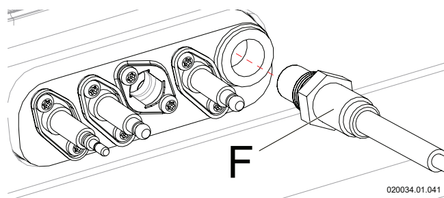
Figura 8-15 - Smontaggio sensore di O 2
