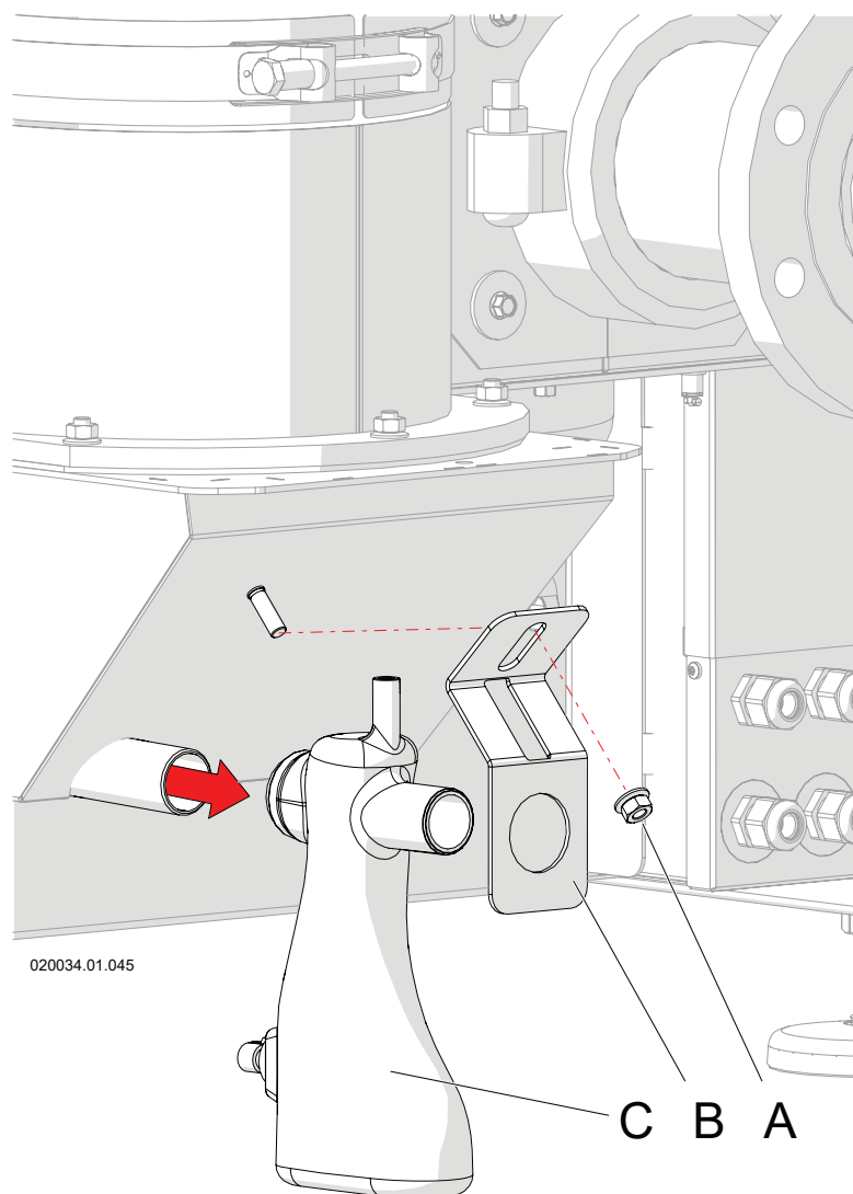
Figura 8-19 - Pulizia dello scarico della condensa
