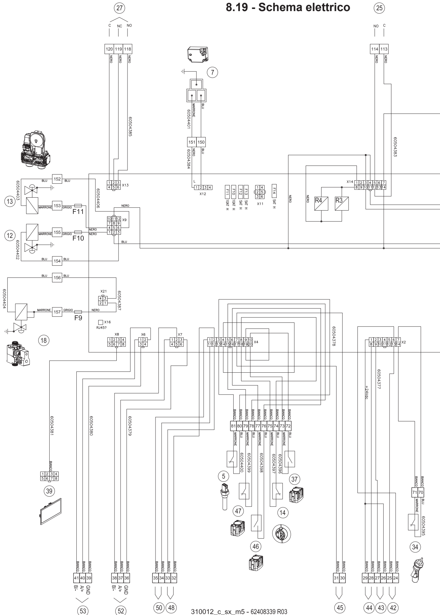
Figura 8-27 - Schema elettrico
