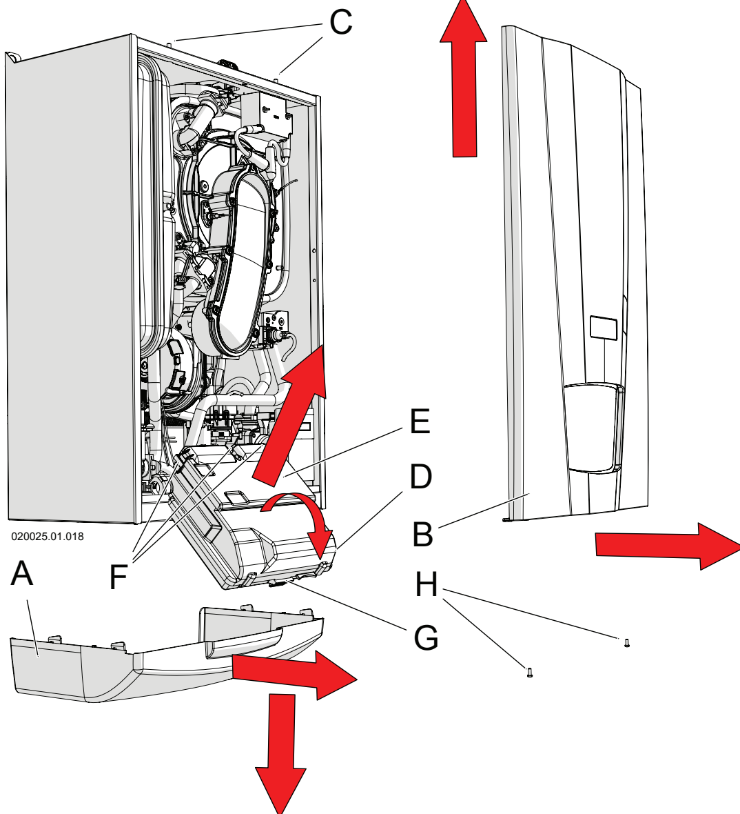
Figura 8-1 - smontaggio mantellatura e apertura quadro comandi
