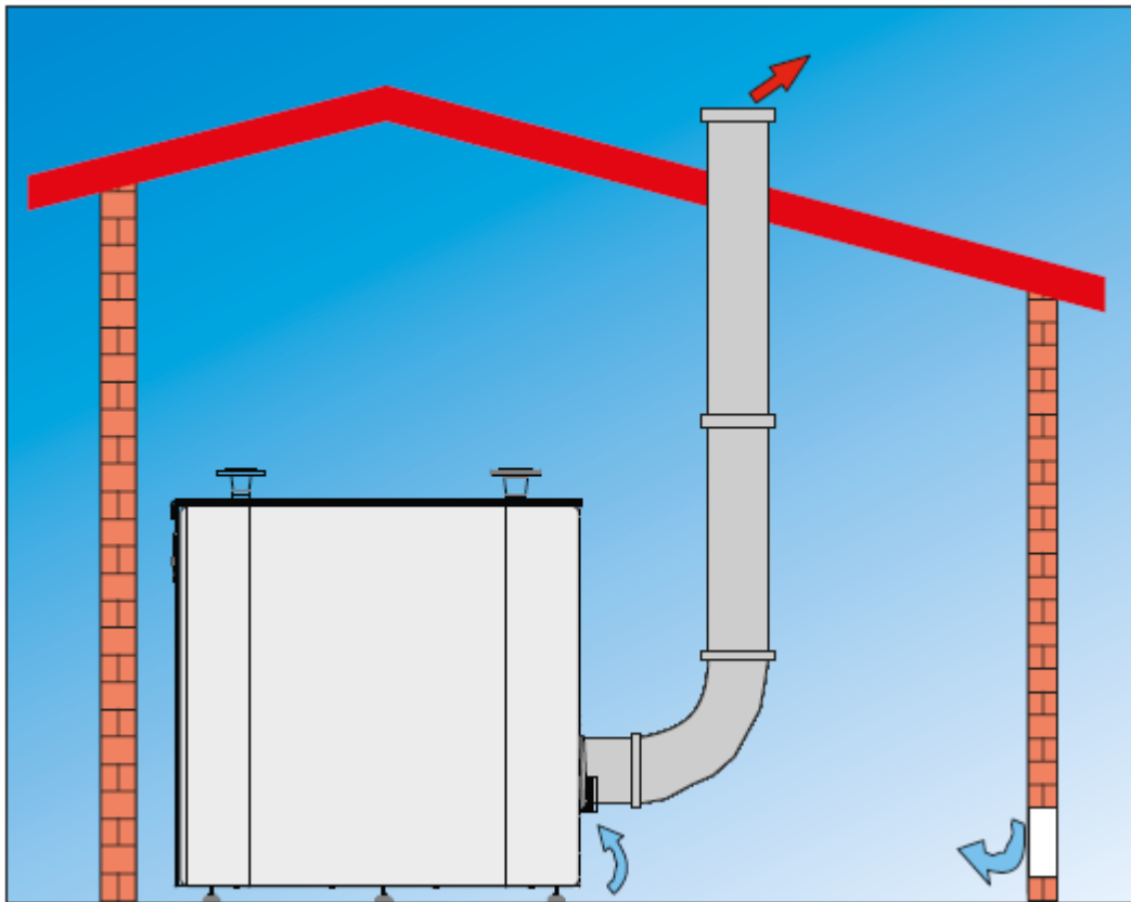
TIPO INSTALLAZIONE B23 – ATTACCO FUMI DIAM 250 mm
