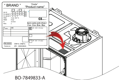
Fig.70 Placa de características
