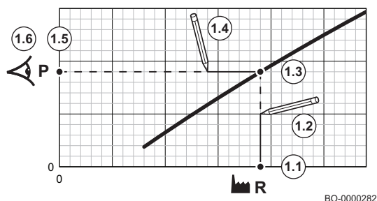
Fig.101 Ajuste de fábrica
