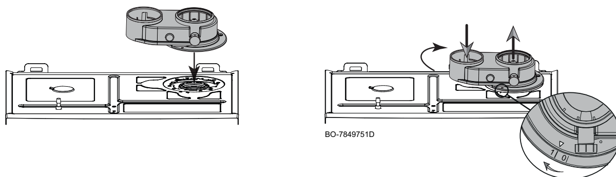
Fig.195 Instalação das condutas (condutas separadas)
