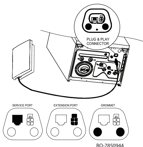
Fig.199 Posição do conector
