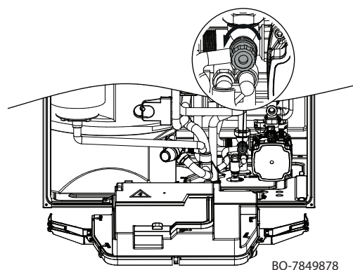
Fig.148 Scarico impianto
