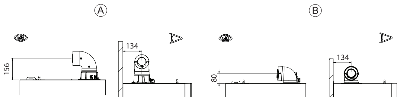
Obr.248 Koncentrický výfukový/prívodný typ
