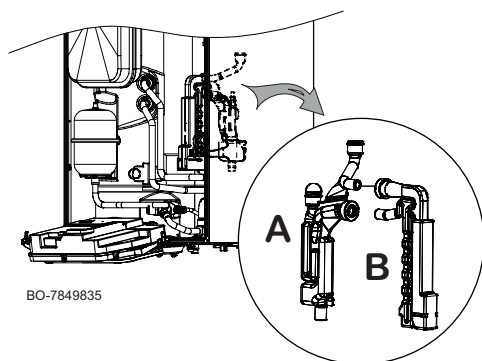
Fig.109 Desmontaje del sifón
