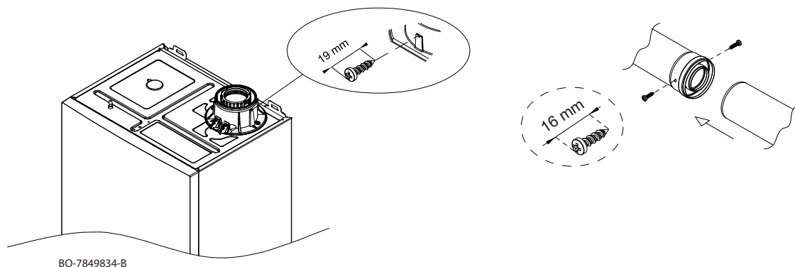
Fig.193 Fixação do adaptador coaxial dos gases da combustão
