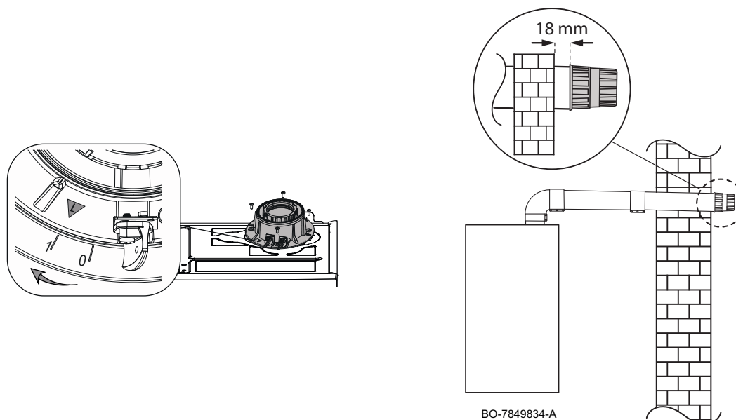
Fig.191 Instalar a ligação coaxial
