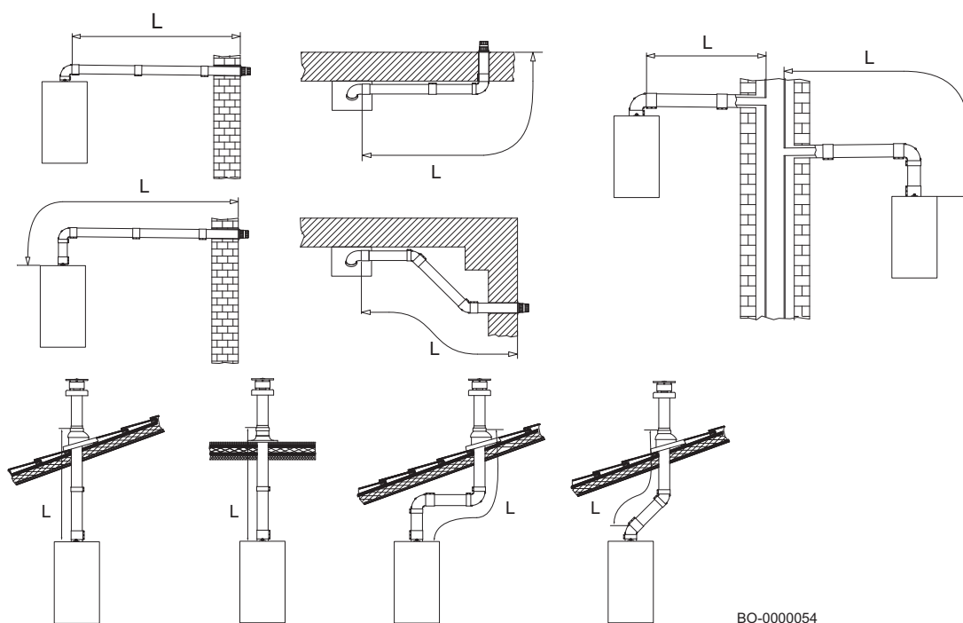
Fig.82 Ejemplos de instalación de tubo coaxial
