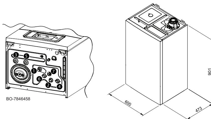
Fig.169 Dimensões e ligações
