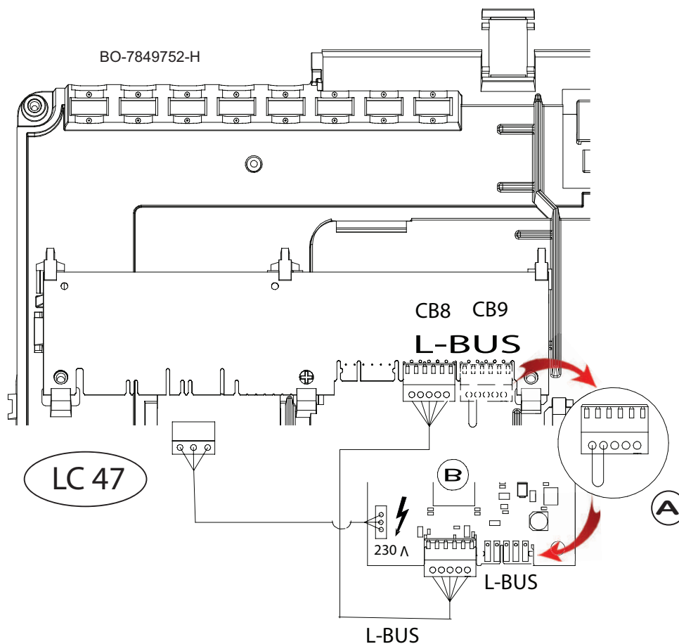
Obr.258 Pripojenie dosky príslušenstva v kotle
