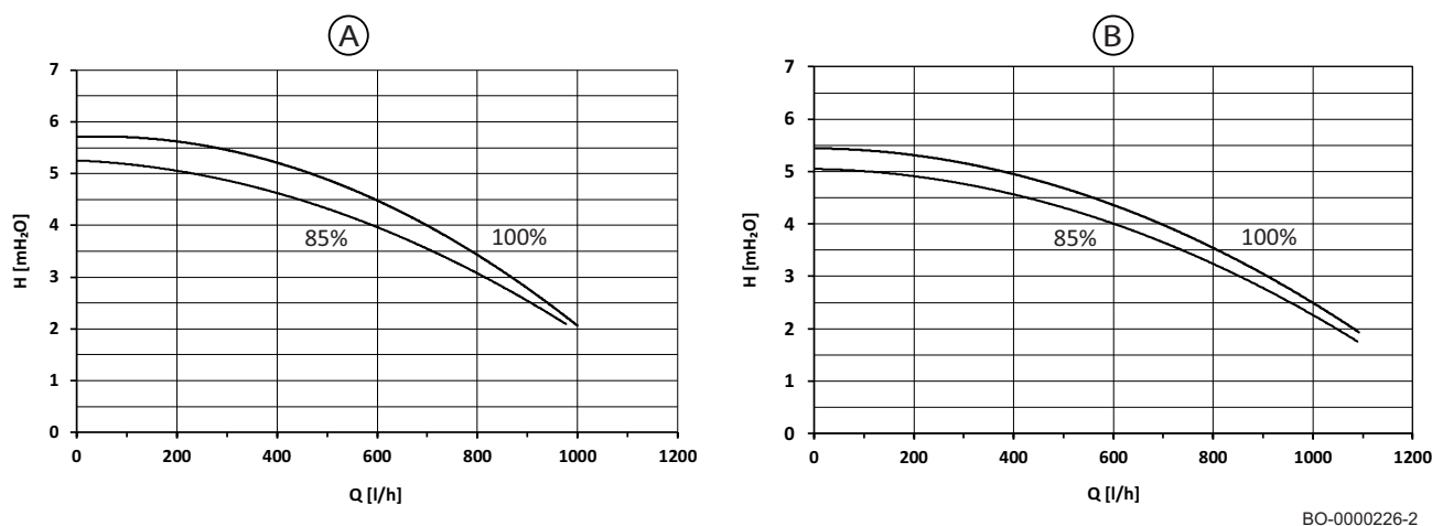
Obr.12 Graf průtoku/výšky na desce
