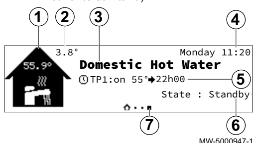
Fig.66 Pantalla de inicio de la página del agua caliente sanitaria (solo si está conectada la sonda del agua caliente sanitaria)
