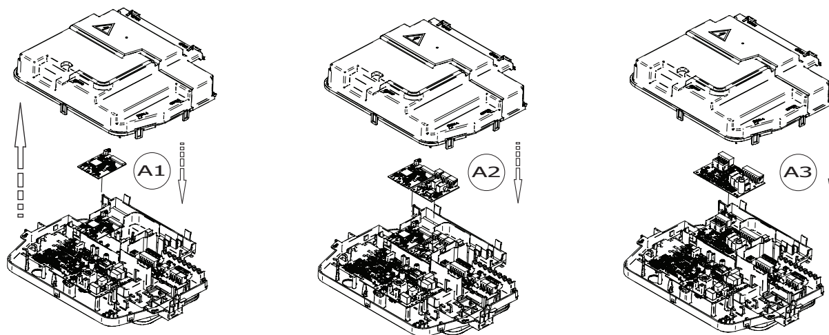
Fig.201 Posicionar e fixar placas adicionais na caldeira
