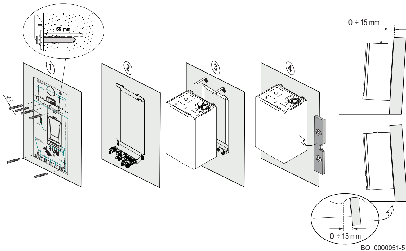
Fig.185 Montagem do acessório na parede
