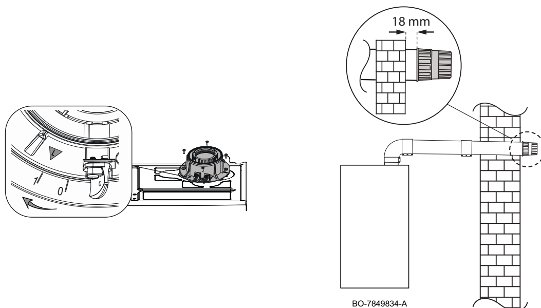
Obr.247 Inštalácia koaxiálnej prípojky
