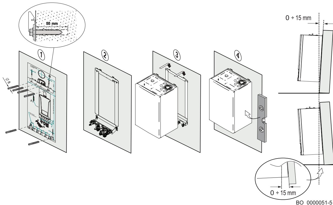
Fig.73 Montaje del accesorio en la pared
