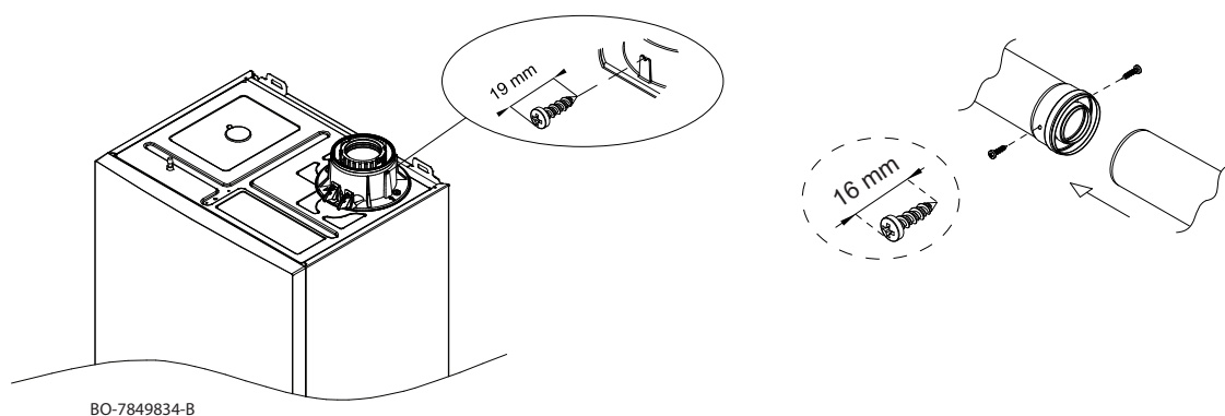
Obr.25 Upevnění věže koaxiálního odvodu spalín
