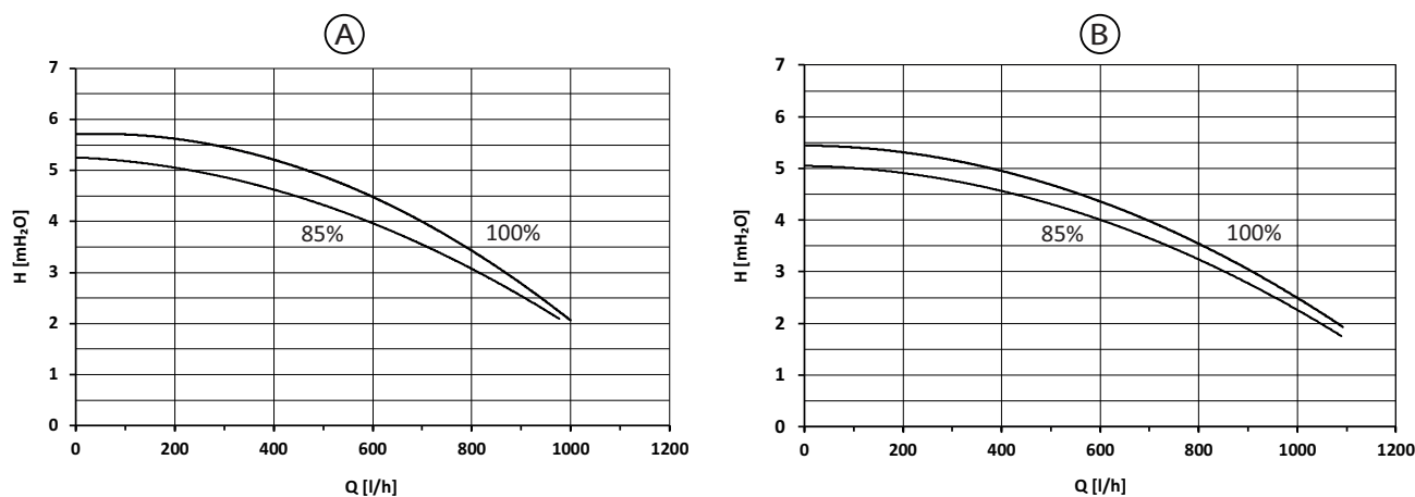
Fig.124 Grafico portata/prevalenza alla placca
