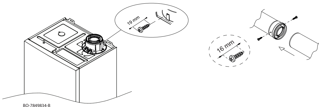
Fig.81 Fijación de la torre de gases de combustión
