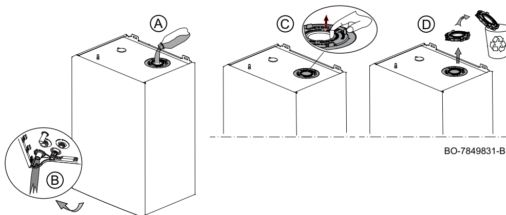
Fig.76 Método de llenado del sifón
