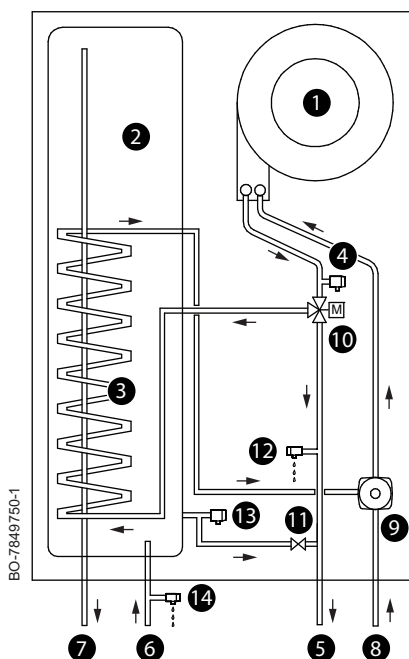
Fig.61 Esquema de principio
