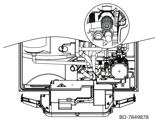
Fig.204 Drenar a instalação
