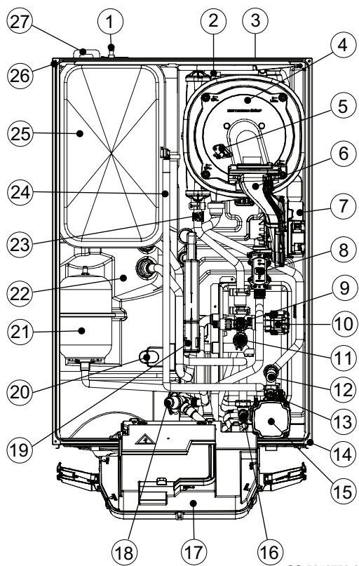
Obr.230 Opis komponentu
