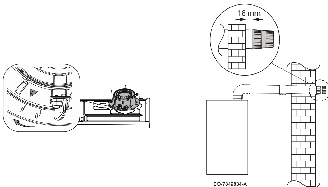
Obr.23 Instalace koaxiální přípojky
