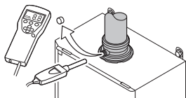
Fig.208 Exemplos de verificações da combustão
