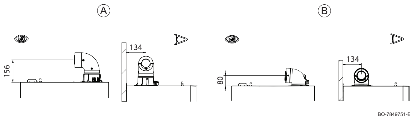
Fig.192 Tipo de evacuação/aspiração concêntrica
