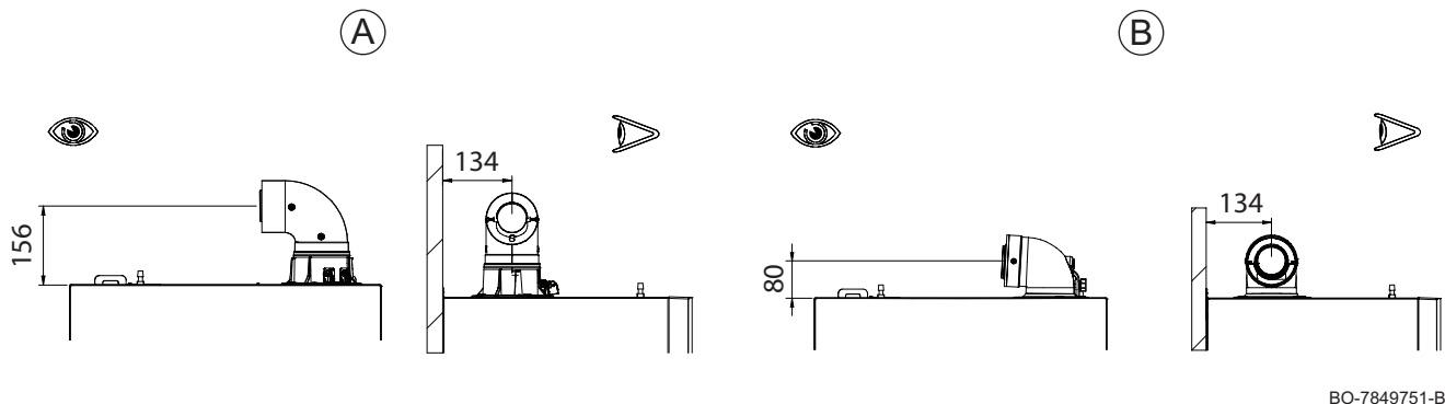
Fig.80 Tipo de aspiración/evacuación concéntrica
