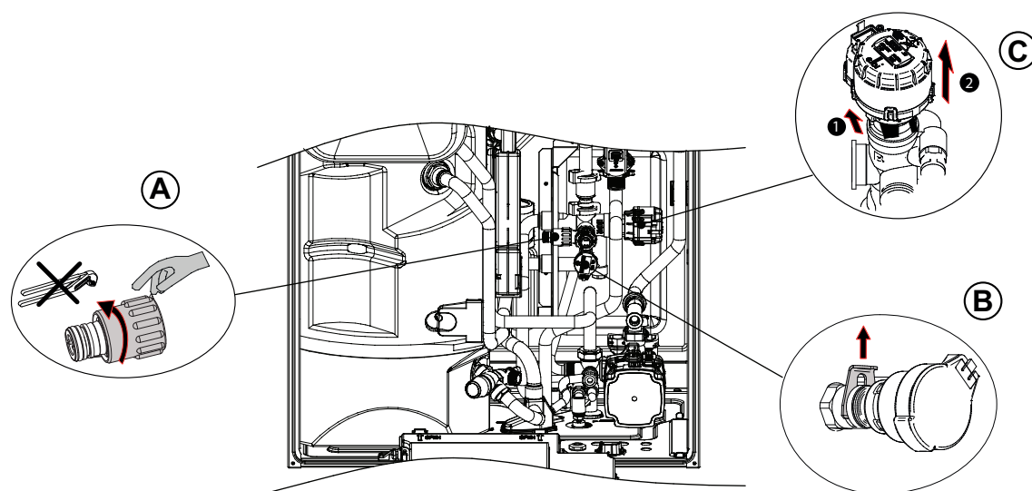
Fig.167 Componenti principale gruppo idraulico
