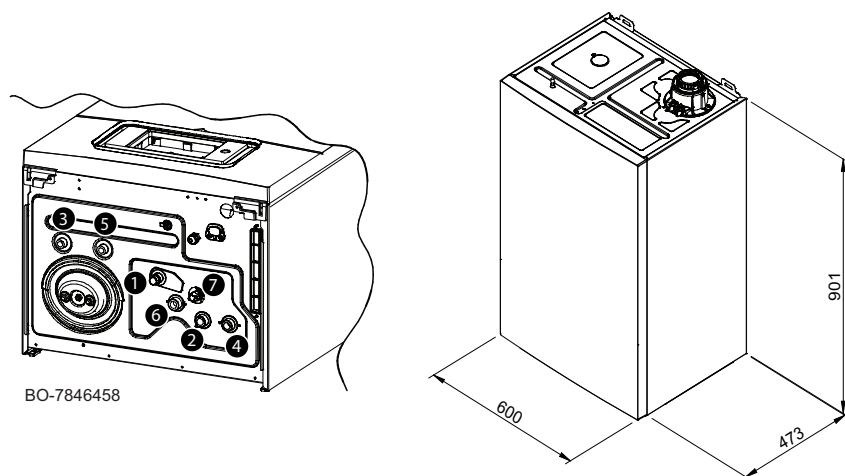
Obr.225 Rozmery a prípojky
