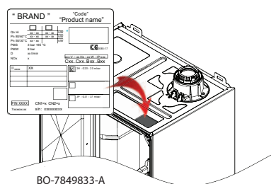
Obr.14 Výrobní štítek
