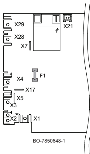
Obr.32 Poloha držáku pojistek
