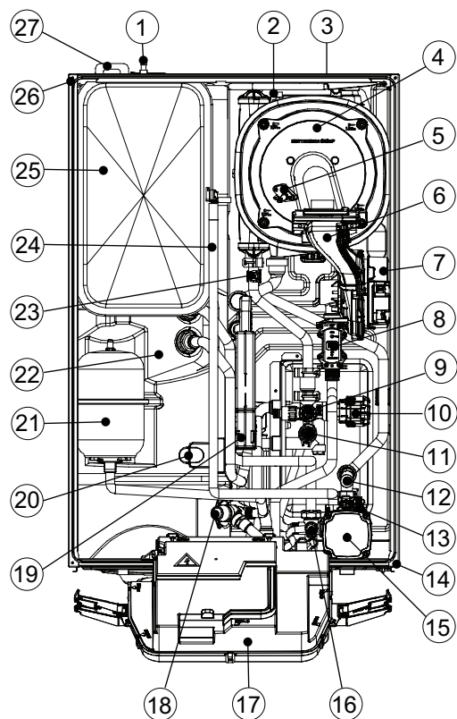
Fig.118 Descrizione componenti
