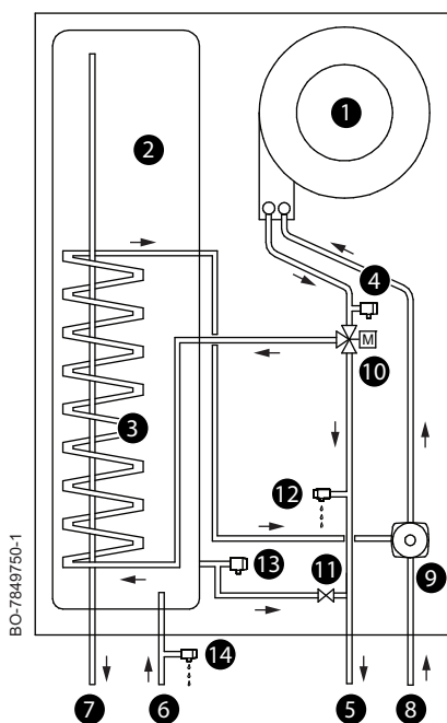
Fig.117 Schema di principio
