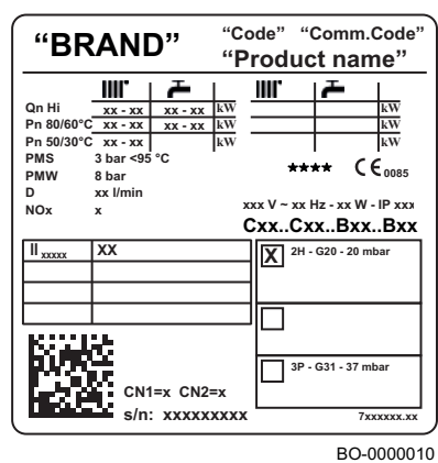
Fig.126 Targa matricola
