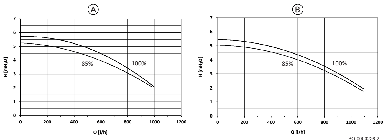
Fig.68 Gráfico de caudal/altura en la placa
