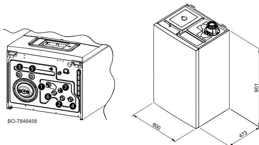
Fig.113 Dimensioni e collegamenti
