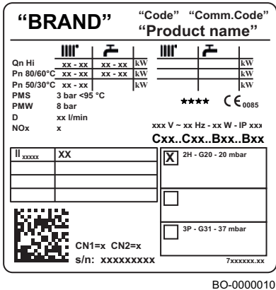
Fig.70 Placa de características
