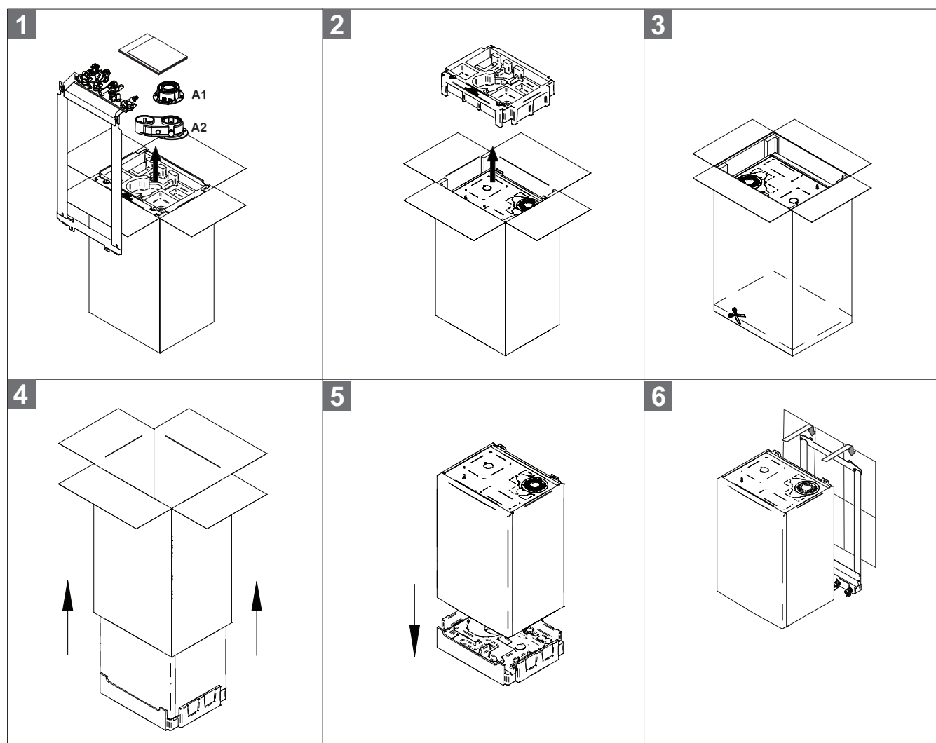
Fig.72 Proceso de desembalaje
