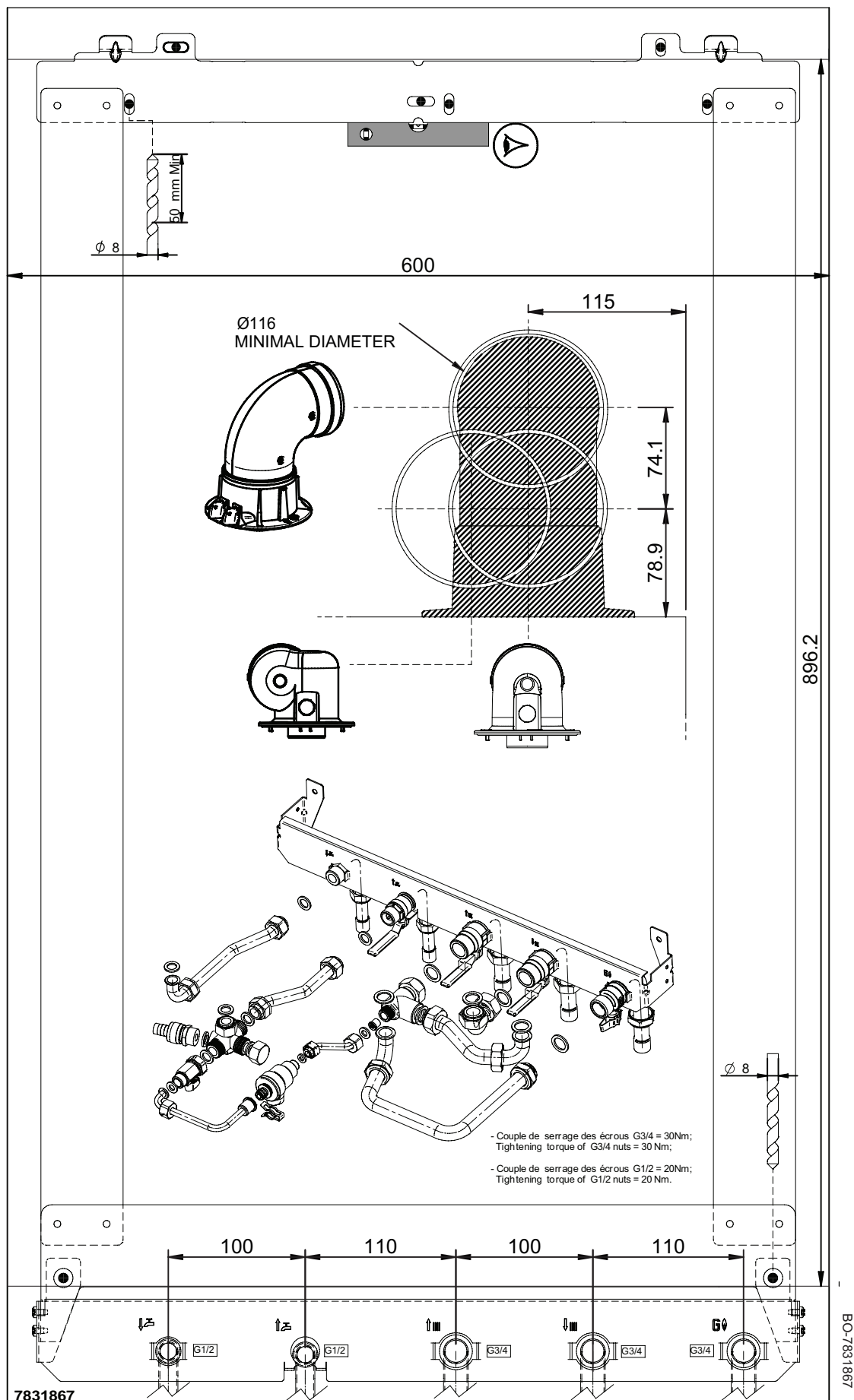
Fig.58 Plantilla de papel
