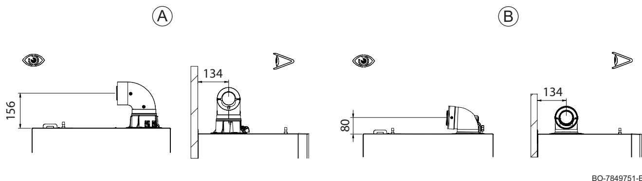
Obr.24 Typ koaxiálního sání – odvodu spalin
