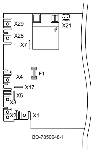
Fig.88 Posición del portafusibles
