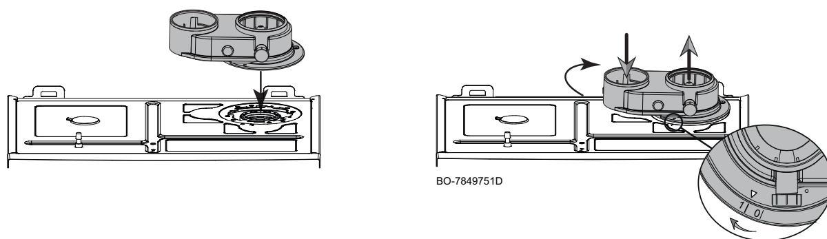
Fig.139 Installazione raccordo per condotti separati
