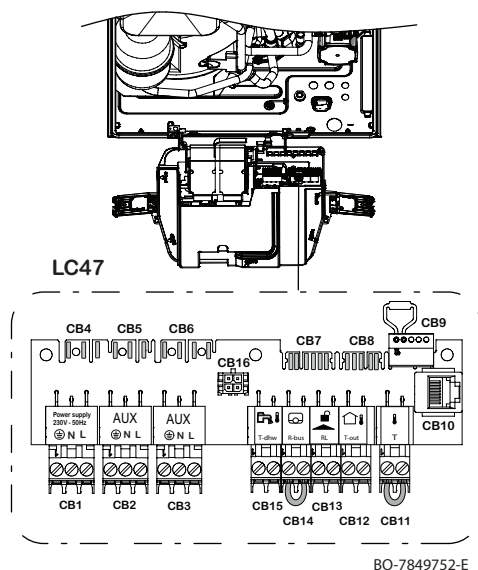
Obr.30 Připojení desky kotle
