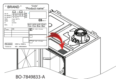
Obr.237 Umiestnenie typového štítka
