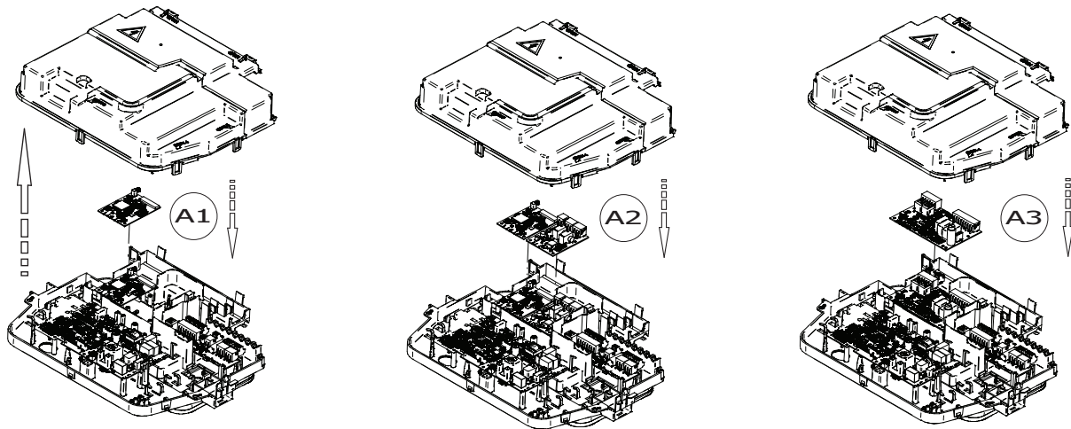
Obr.257 Umiestnenie a upevnenie dosiek príslušenstva v kotle
