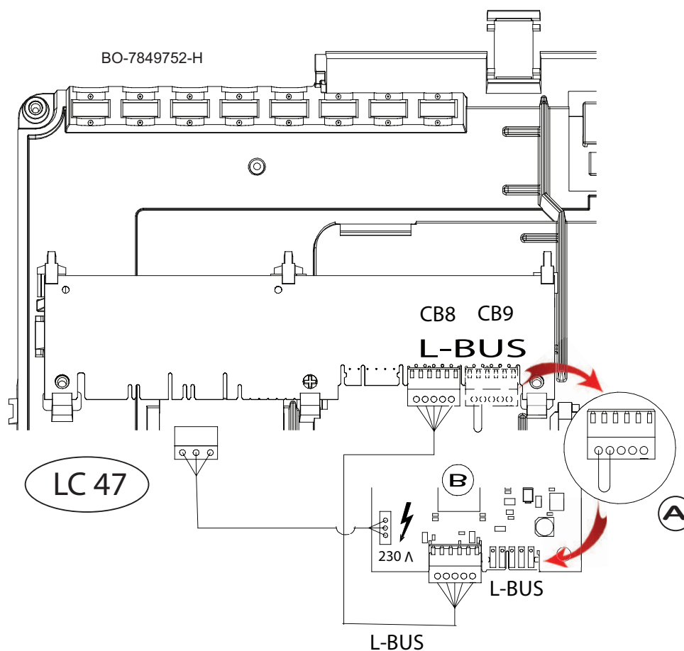
Fig.202 Ligação da placa adicional na caldeira
