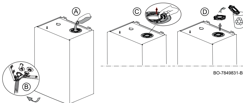
Fig.188 Método de enchimento do sifão
