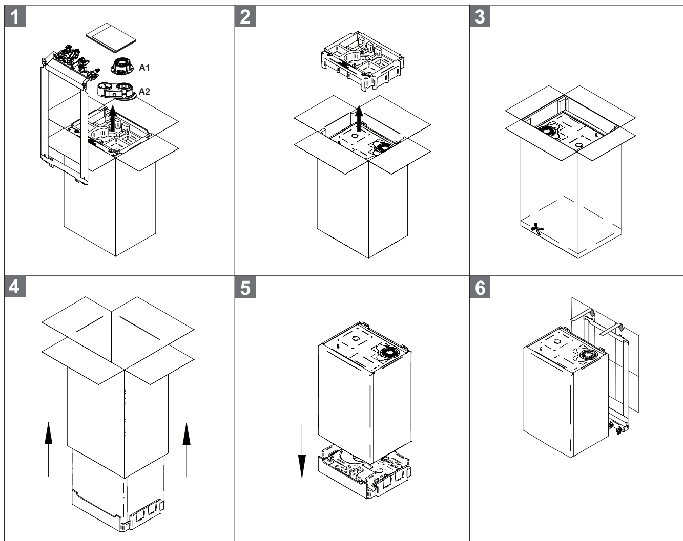
Obr.16 Postup při vybalování
