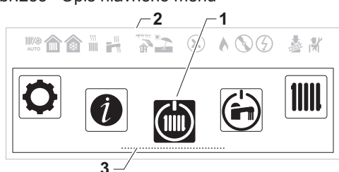
Obr.235 Opis hlavného menu
