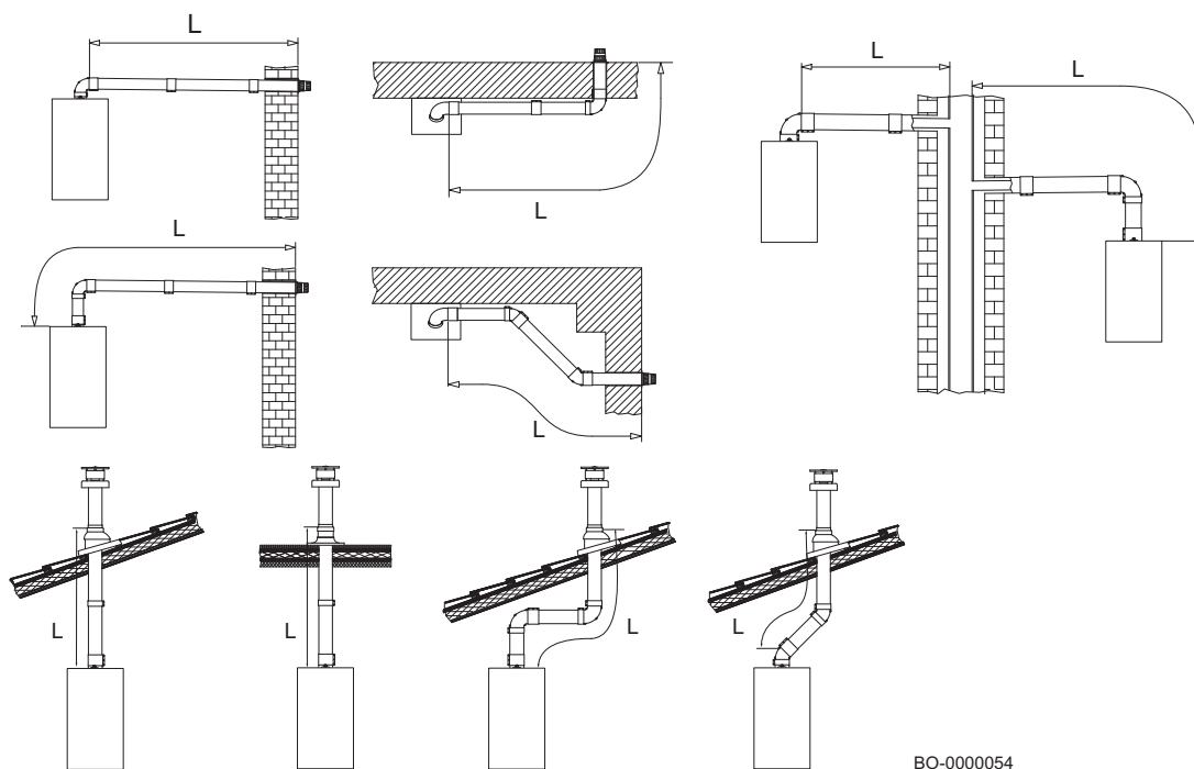
Obr.250 Príklady inštalácie koaxiálneho potrubia
