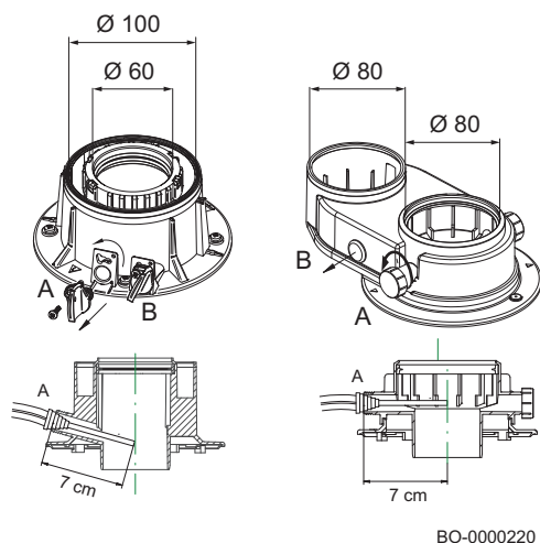
Fig.95 Punto de medición de los gases de combustión según accesorio de conexión a caldera
