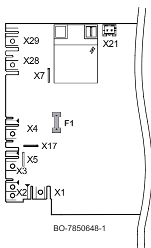
Fig.200 Posição do porta fusível
