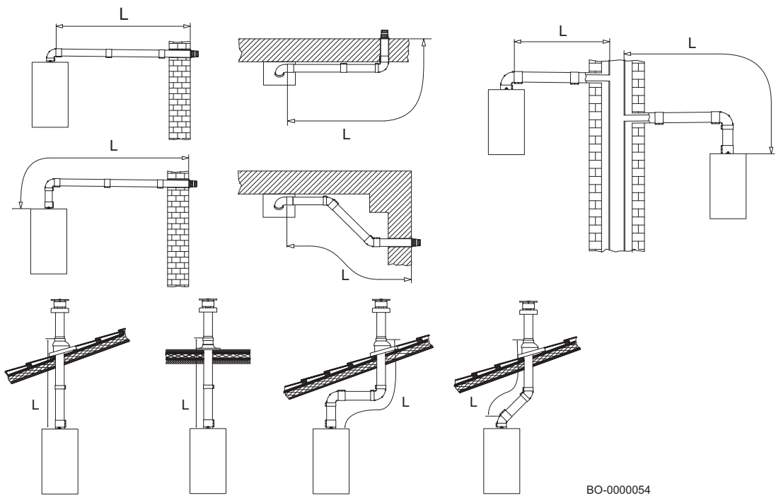
Fig.194 Exemplos de instalação do tubo coaxial
