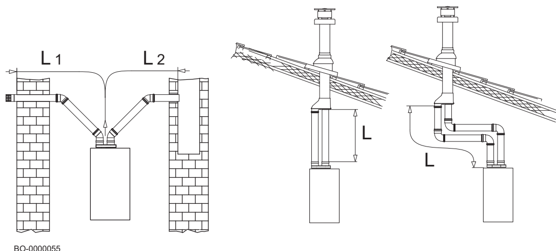
Obr.252 Príklady inštalácie oddeleného potrubia
