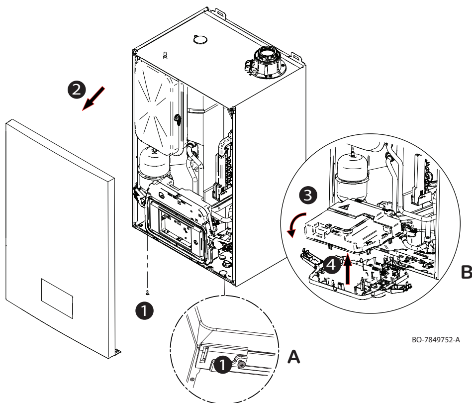
Obr.29 Přístup k elektrickým přípojkám
