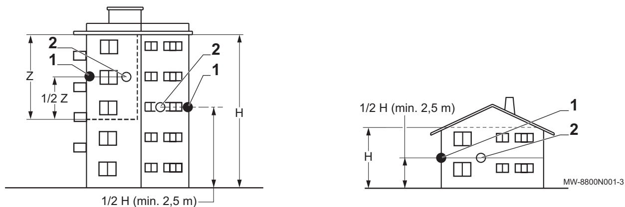
Obr.242 Odporúčané umiestnenia (A)
