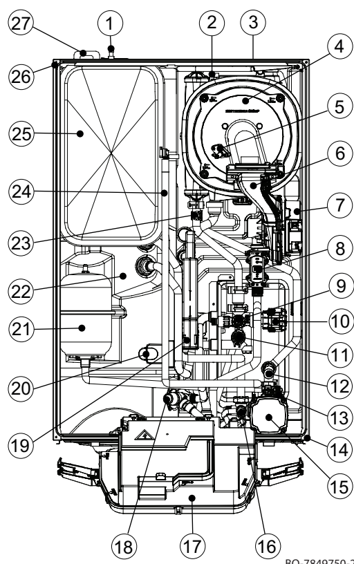
Fig.62 Descripción de componentes
