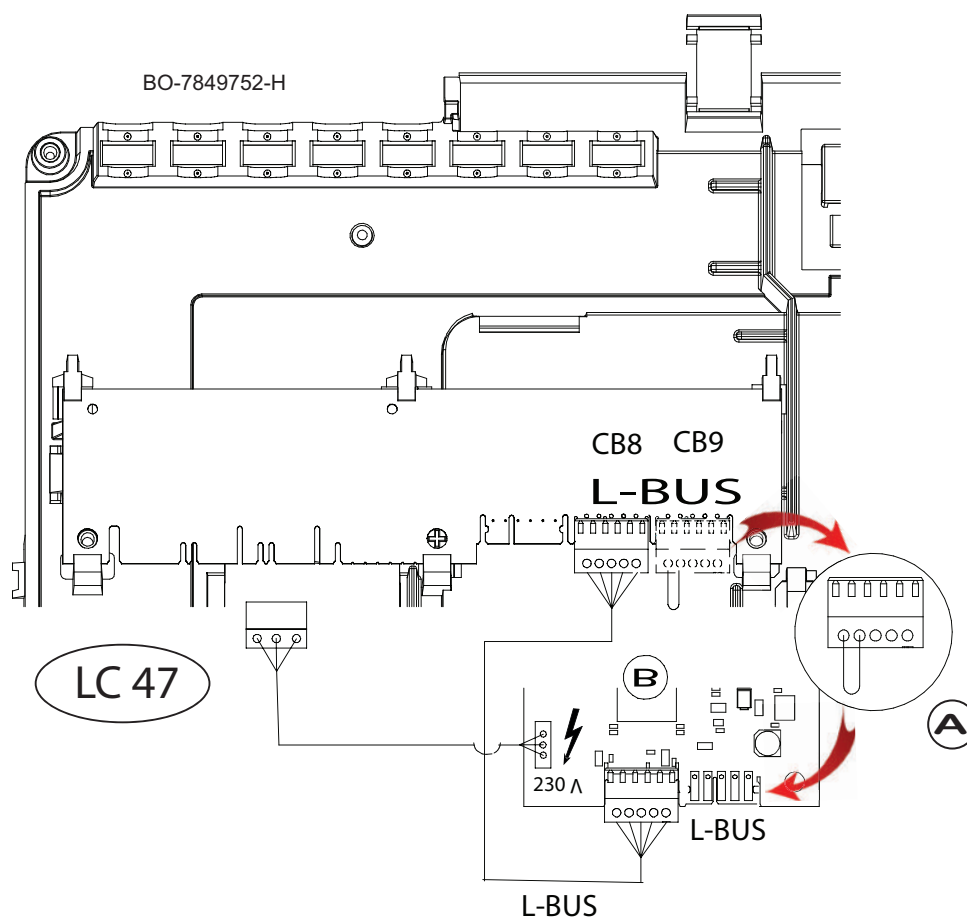
Fig.90 Conexión de la placa adicional a la caldera
