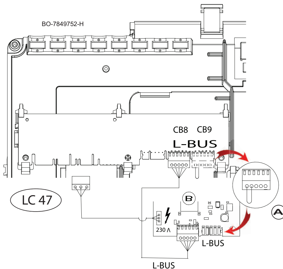
Obr.34 Připojení desky příslušenství v kotli
