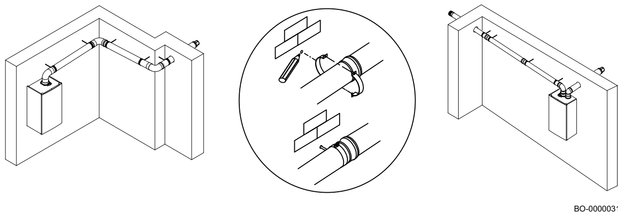
Fig.133 Modalità di fissaggio a muro dei condotti
