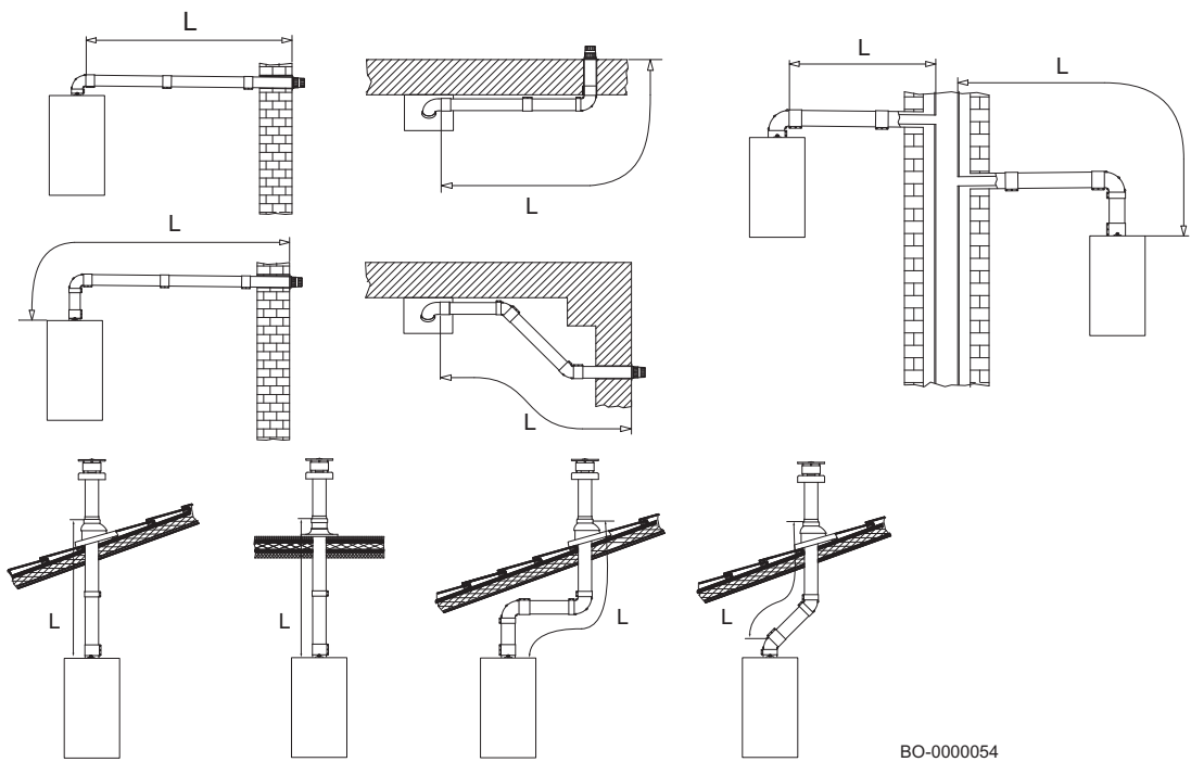
Fig.138 Esempi installazioni condotti coassiali
