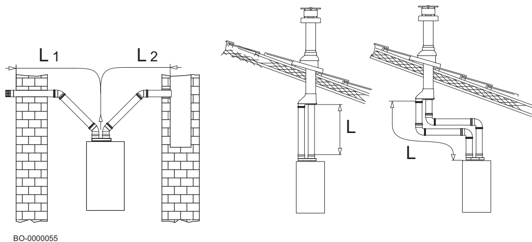
Obr.28 Příklady instalace samostatného potrubí
