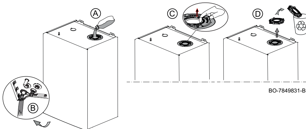
Obr.244 Spôsob plnenia sifónu
