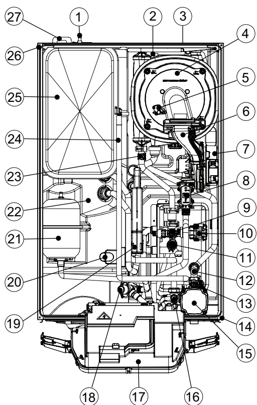
Obr.6 Popis komponenty
