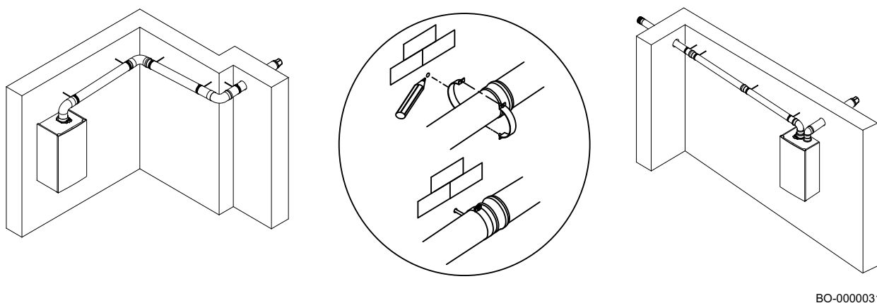
Obr.21 Způsob upevnění potrubí ke stěně
