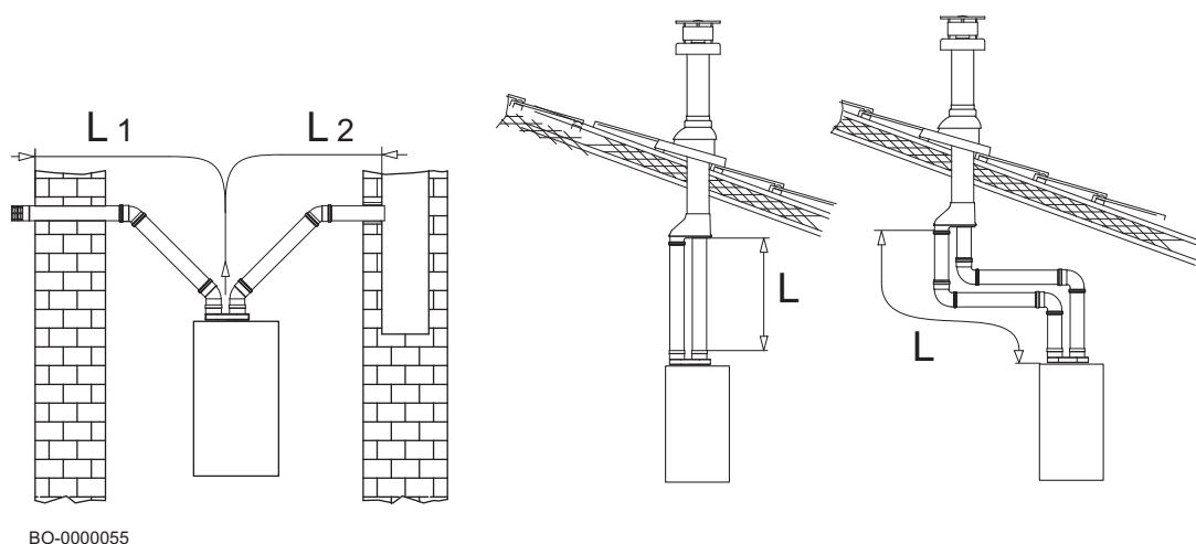
Fig.196 Exemplos de instalação de condutas separada
