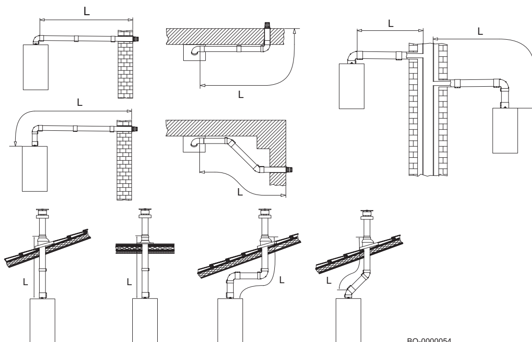
Obr.26 Příklady instalace koaxiálního potrubí
