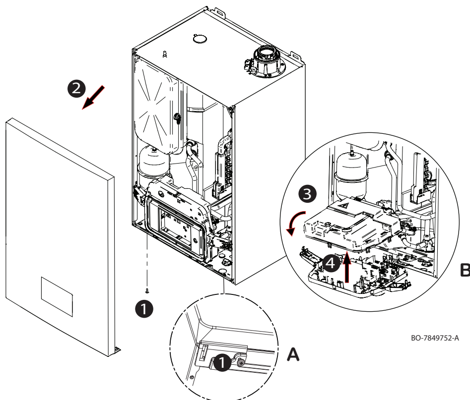
Obr.253 Prístup k elektrickým pripojeniam
