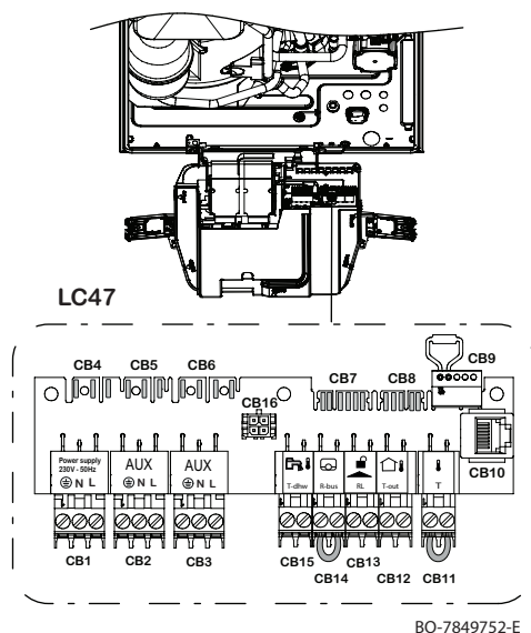
Fig.198 Ligações da placa da caldeira
