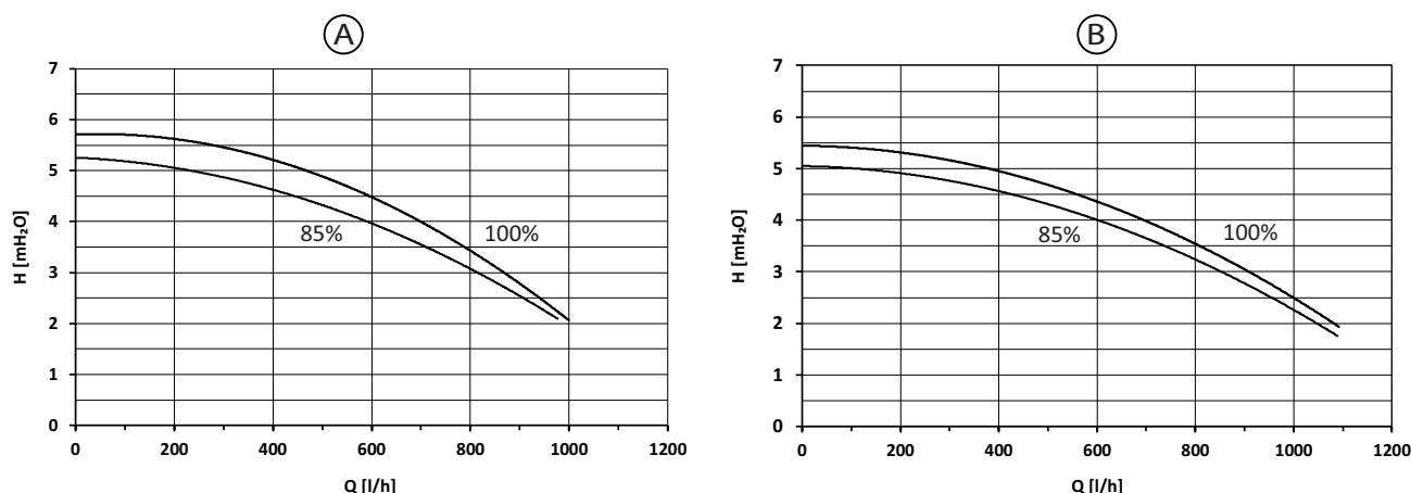
Fig.180 Gráfico de caudal/altura na placa
