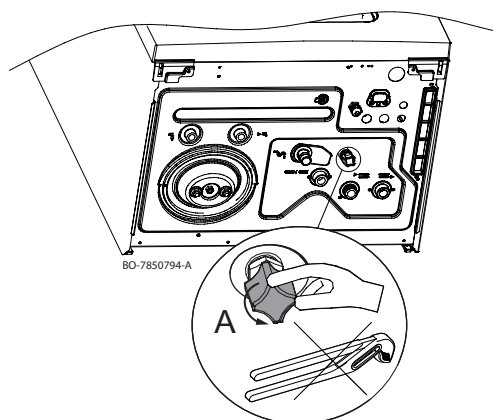
Fig.91 Llenado de la instalación
