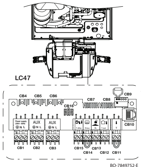
Obr.254 Pripojenia dosky kotla
