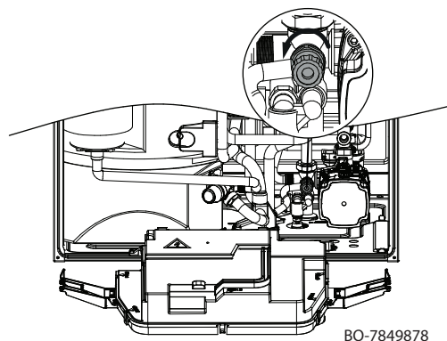
Obr.36 Vypuštění soustavy
