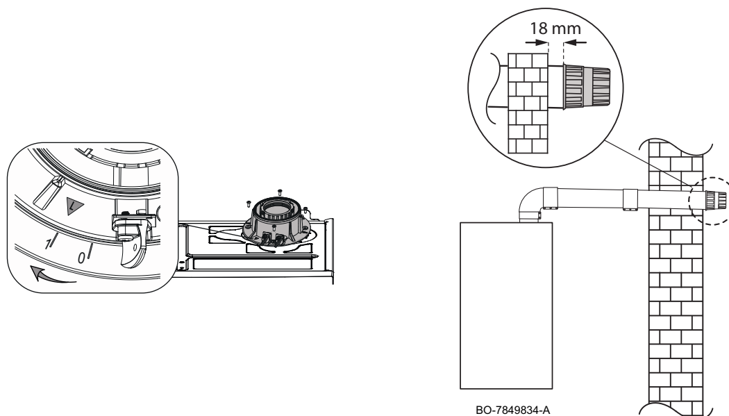
Fig.135 Installazione raccordo coassiale
