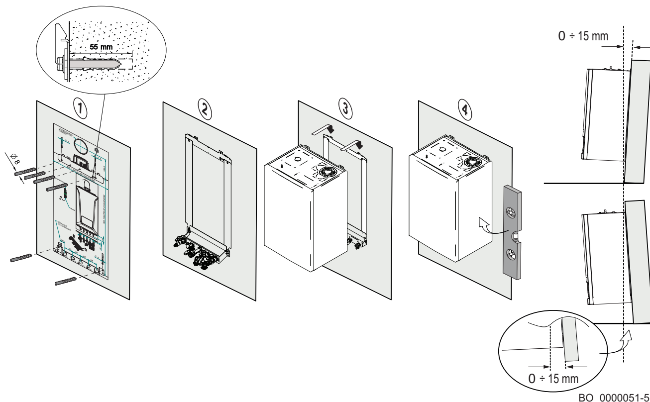
Fig.129 Installazione a parete dell'accessorio
