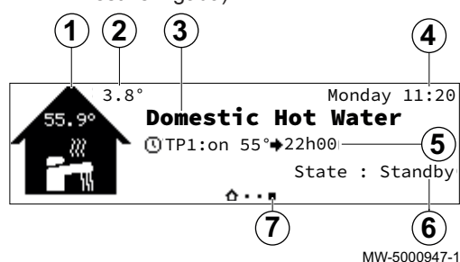
Fig.178 Ecrã inicial da página da água quente sanitária (apenas se a sonda de água quente sanitária estiver ligada)
