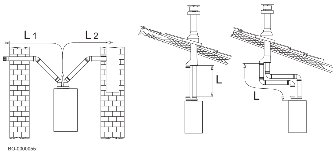
Fig.84 Ejemplos de instalación de conducto separado
