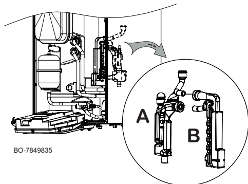
Fig.165 Smontaggio del sifone
