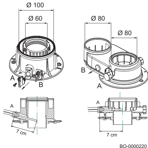
Fig.151 Tipologie di raccordi — punto di misurazione fumi
