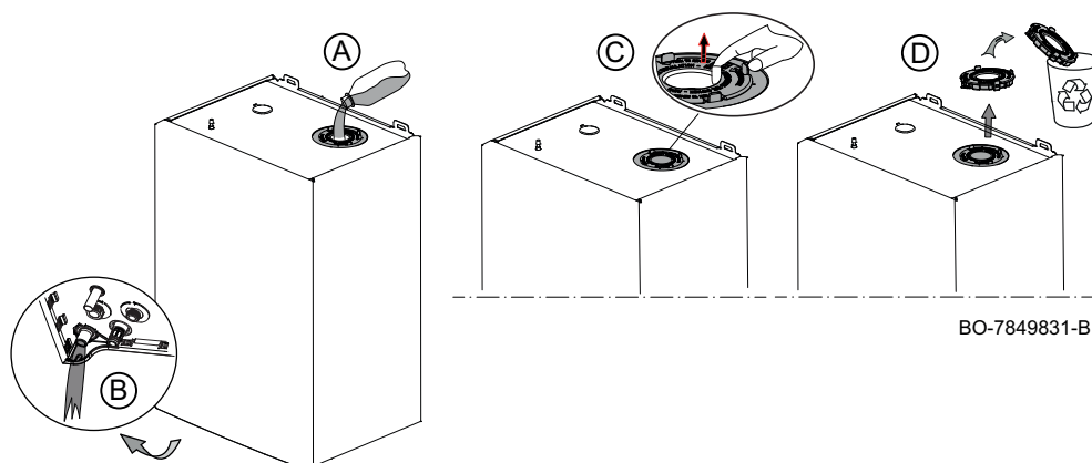
Obr.20 Způsob plnění sifonu
