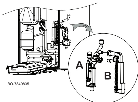
Fig.221 Desmontar o sifão
