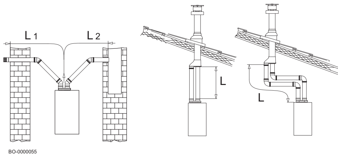
Fig.140 Esempi installazioni condotti separati
