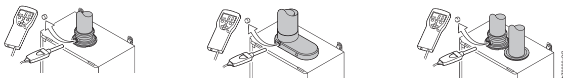
Fig.96 Ejemplos de comprobaciones de combustión
