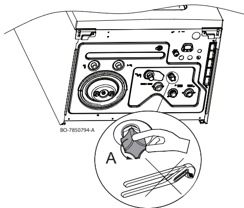
Obr.35 Plnění topného systému
