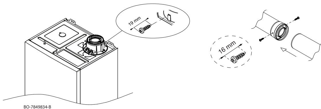
Obr.249 Upevnenie koaxiálneho odvodu spalín
