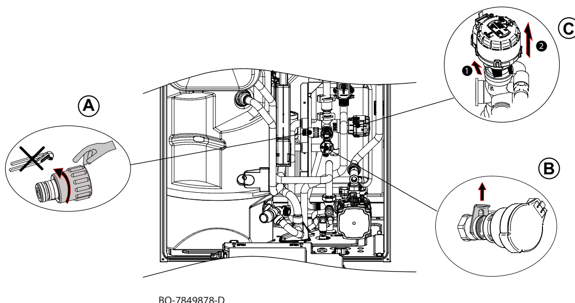
Fig.111 Principales componentes de la unidad hidráulica
