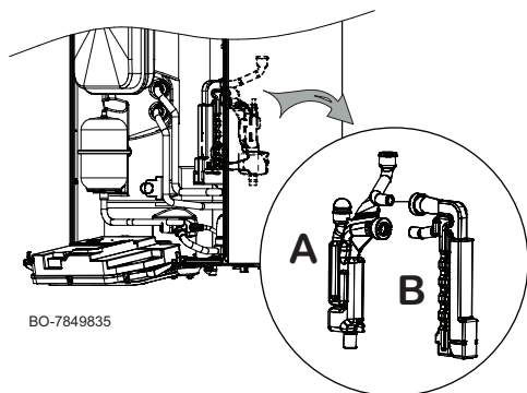
Obr.53 Demontáž sifonu
