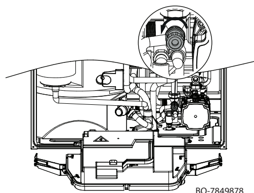
Fig.92 Vaciado de la instalación
