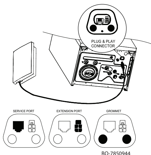
Fig.143 Posizione del connettore
