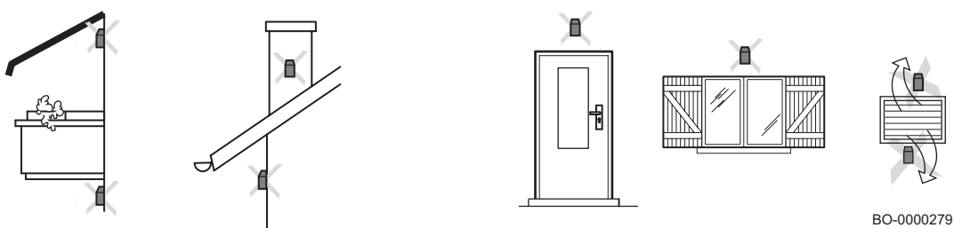
Fig.131 Ubicazioni sconsigliate B
