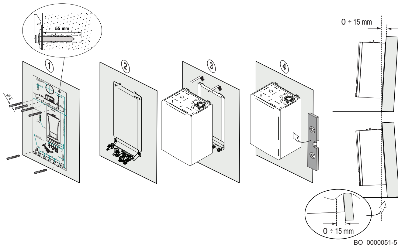
Obr.241 Upevnenie príslušenstva na stenu
