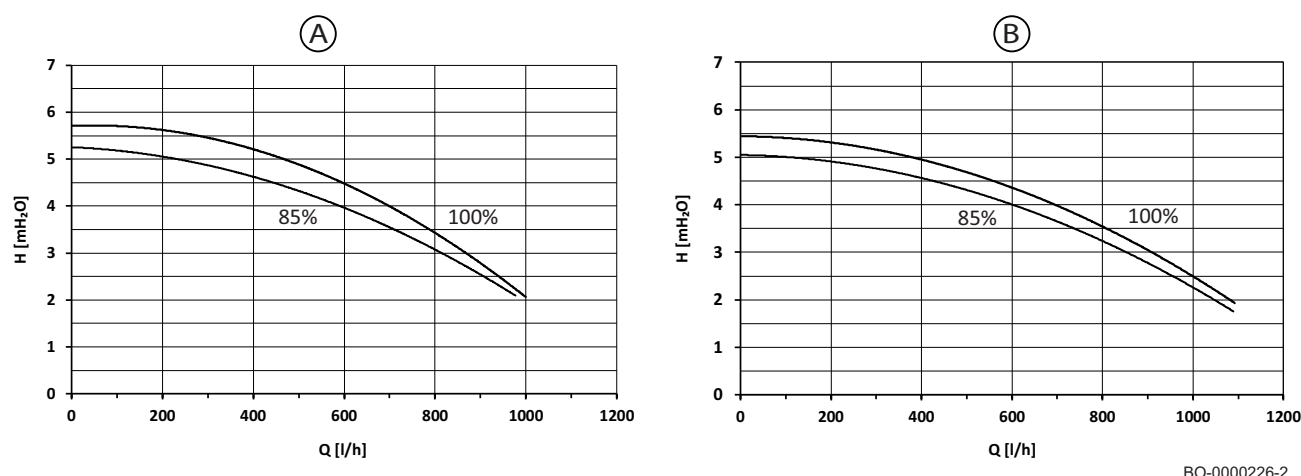
Obr.236 Graf prietoku/výšky na doske
