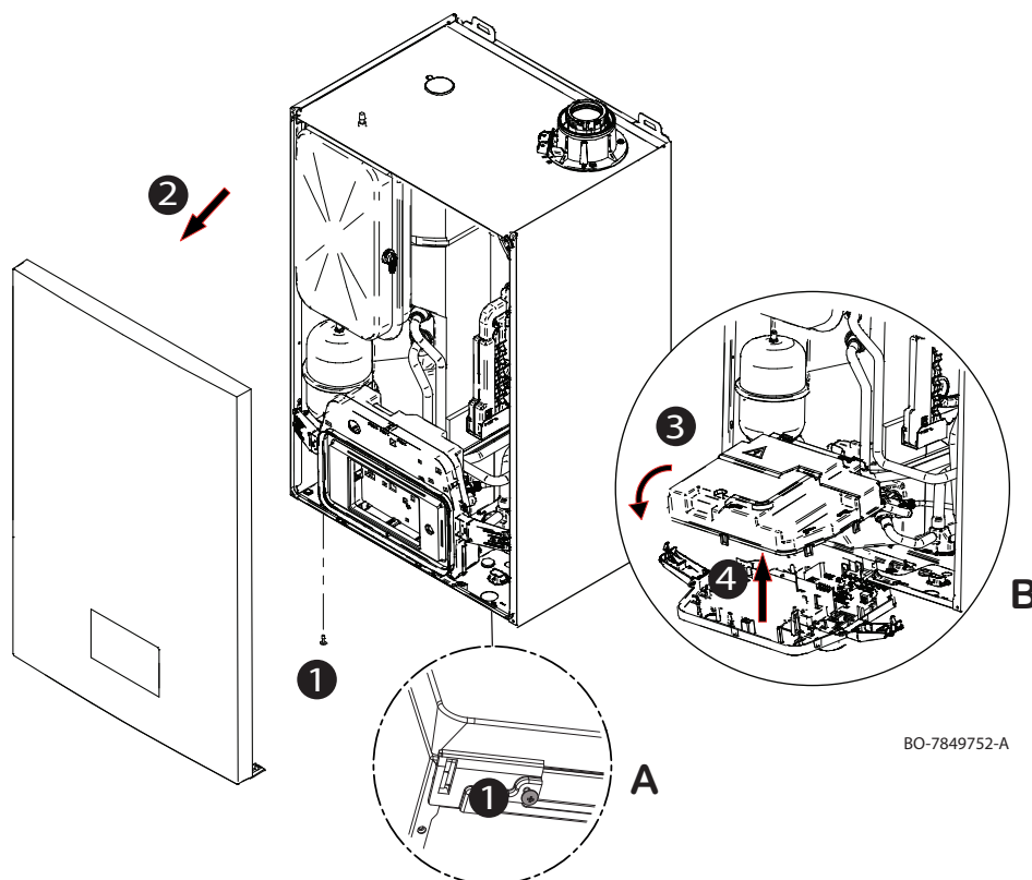
Fig.141 Accesso ai collegamenti elettrici
