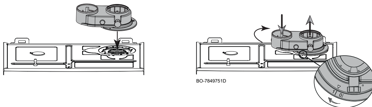
Fig.83 Instalación de conductos desdoblados
