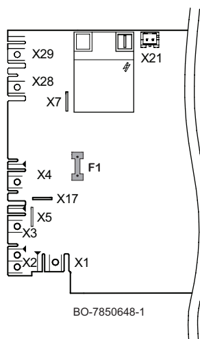
Obr.256 Poloha držiaka poistky
