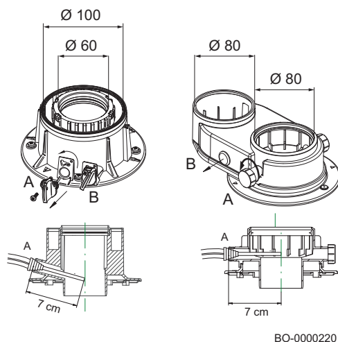
Obr.263 Typy prípojek – merací bod spalín
