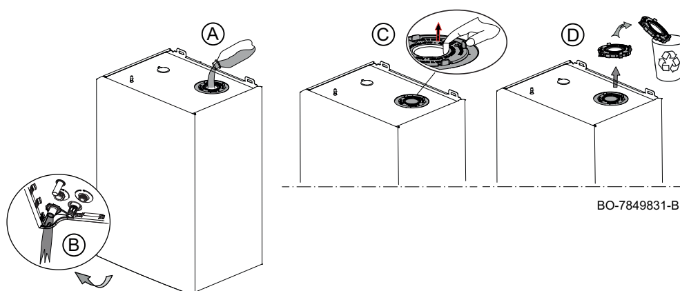
Fig.132 Modalità di riempimento del sifone
