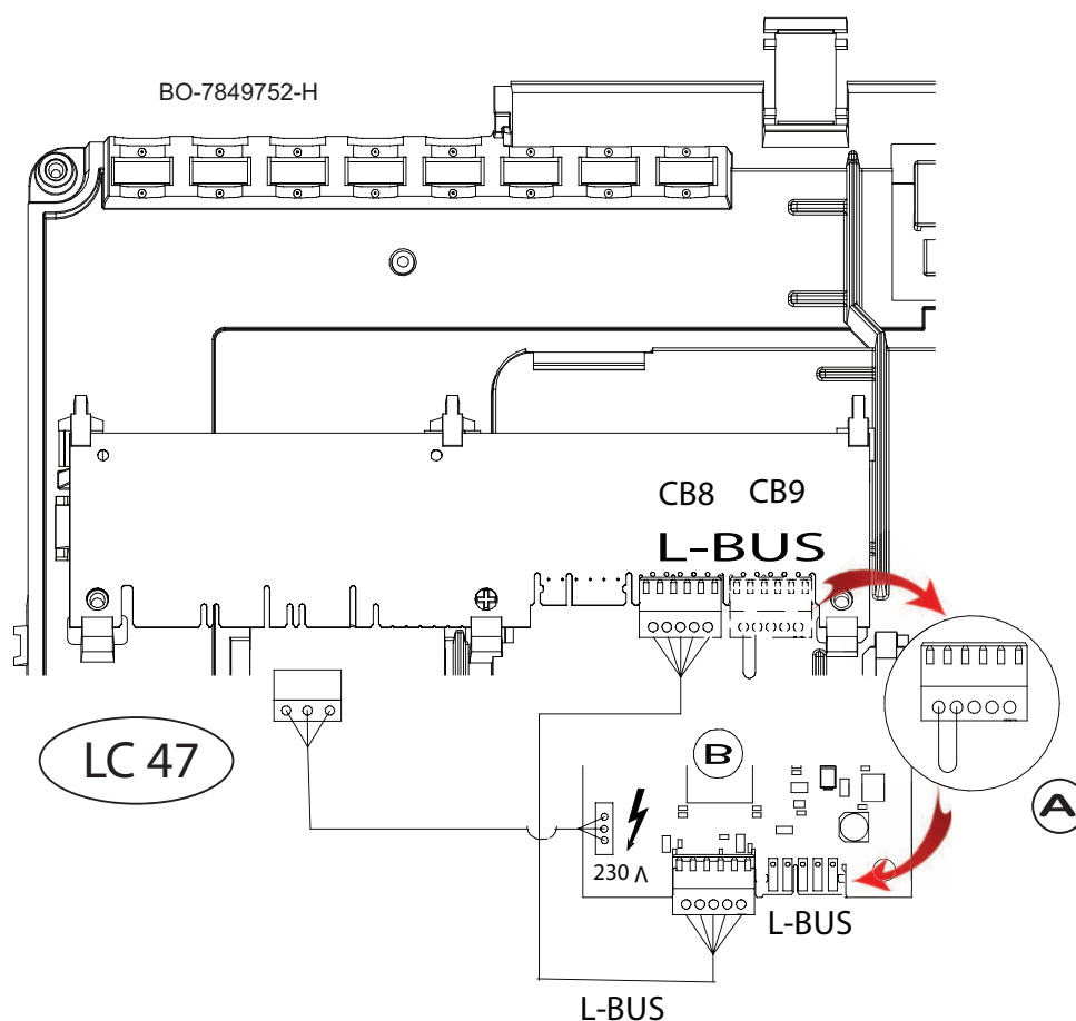
Fig.146 Collegamento scheda accessoria in caldaia
