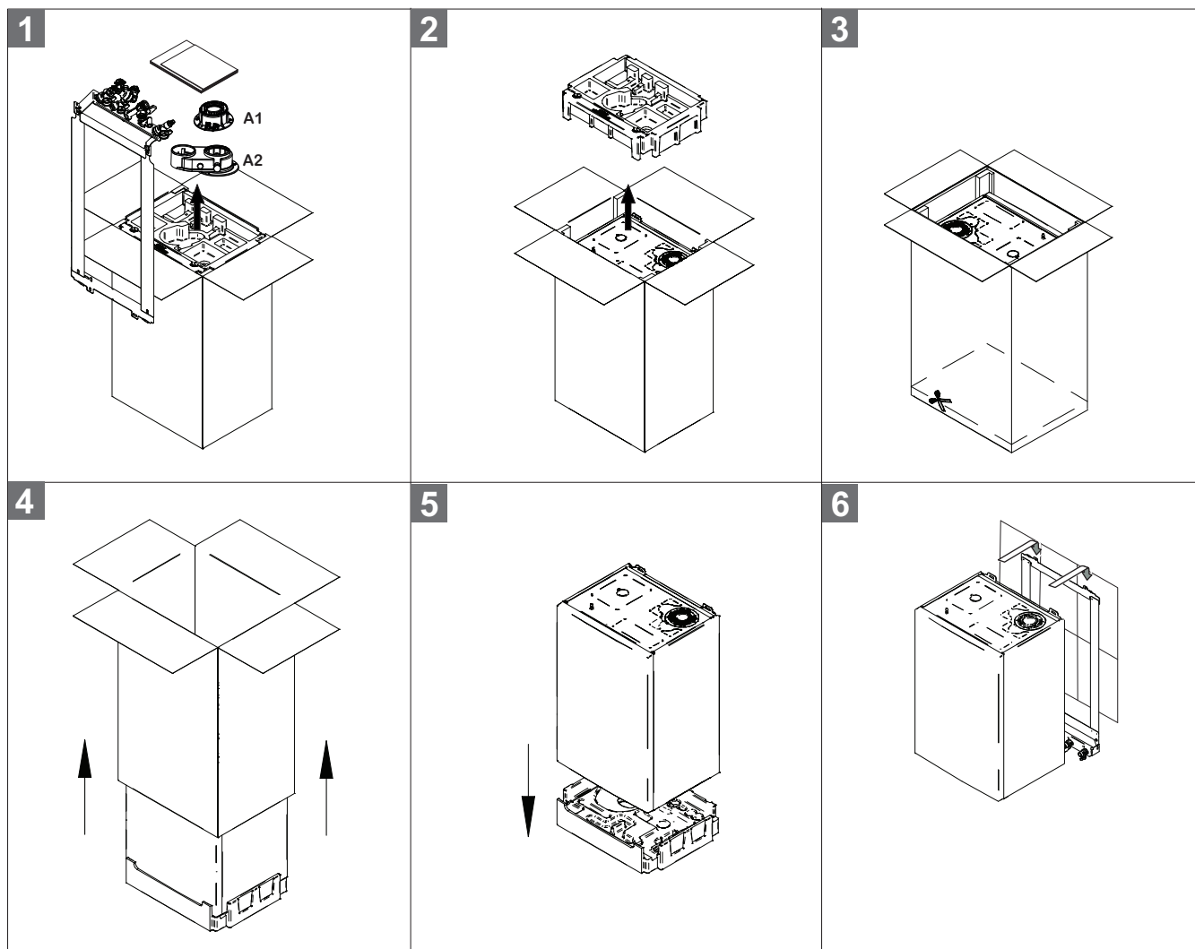
Fig.184 Procedimento de desembalamento
