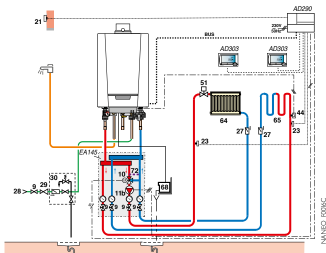
EMC-M... MI con 1 circuito diretto + 1 circuito impianto a pavimento con valvola miscelatrice (con modulo idraulico compatto - Collo EA 145), comandata da 2 comandi ambiente modulanti "OpenTherm" (via radio) + modulo di comando per 2 circuiti (collo AD 290)
