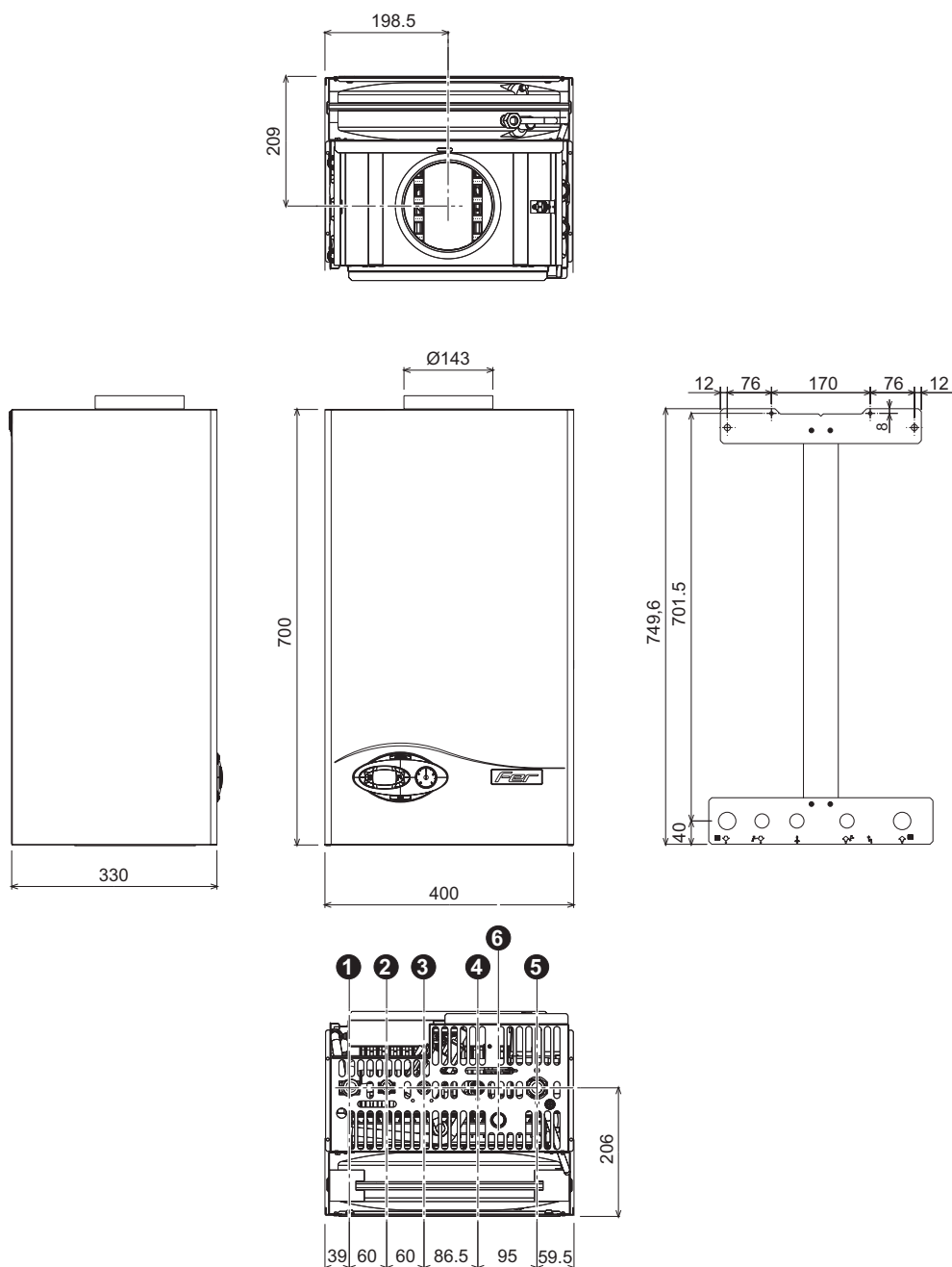
fig. 18 - Dimensioni e attacchi
