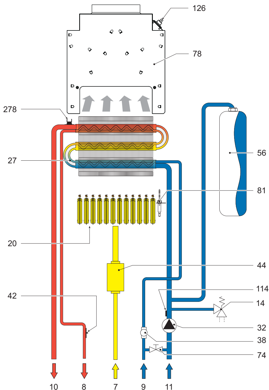
fig. 20 - Circuito idraulico
