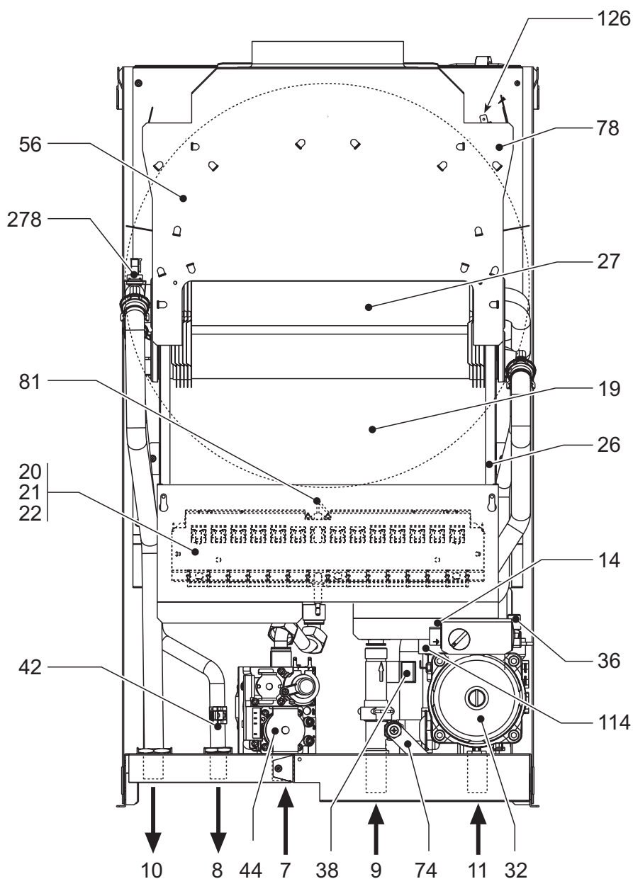
fig. 19 - Vista generale
