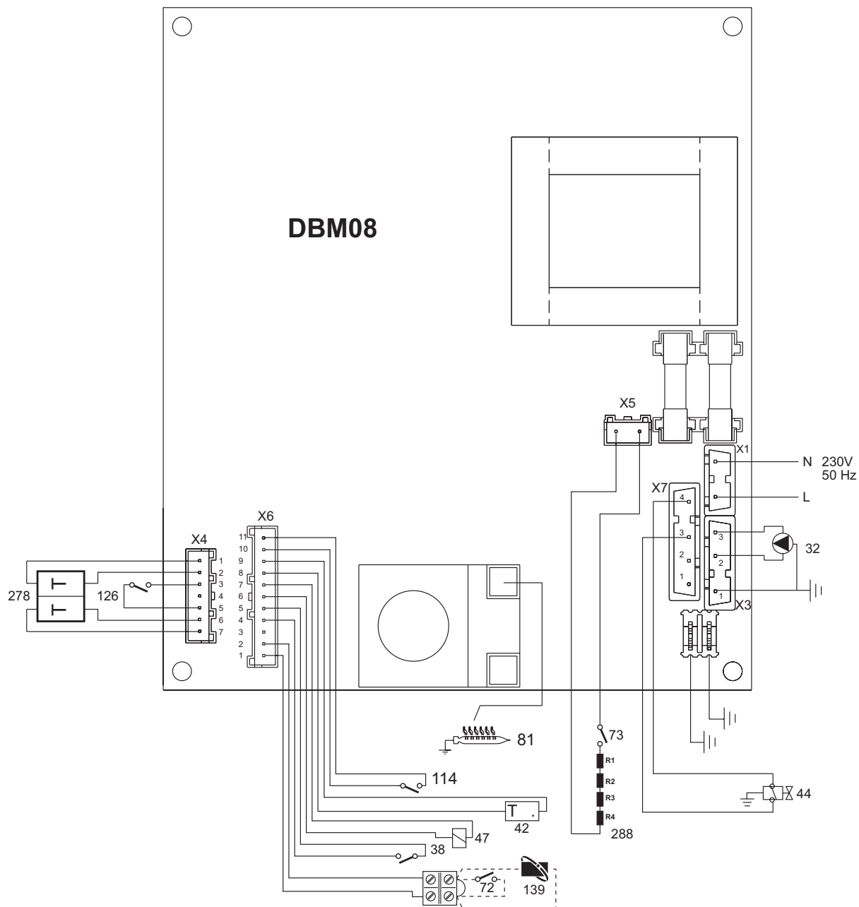
fig. 21 - Schema elettrico
