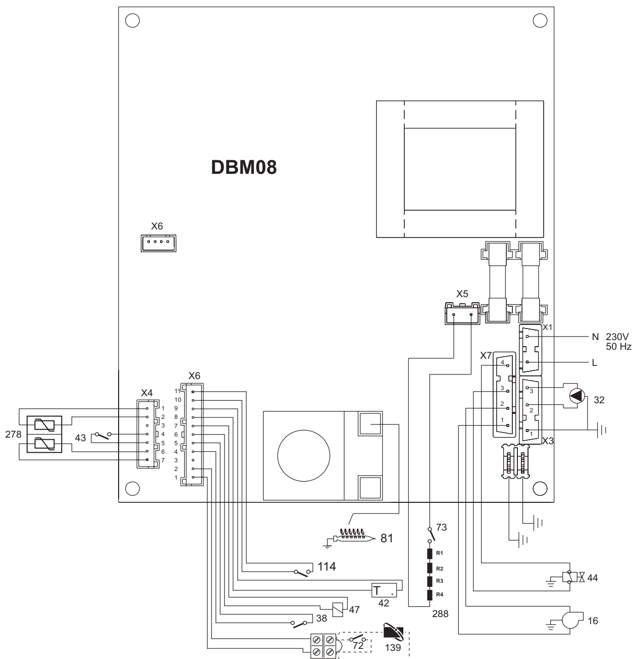
fig. 29 - Schema elettrico
