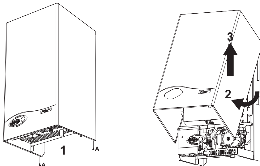
fig. 24 - Apertura mantello
