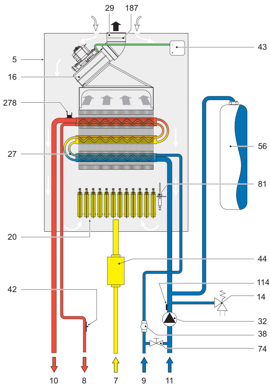
fig. 28 - Circuito idraulico
