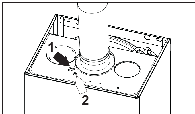
fig. 25 - Analisi fumi
