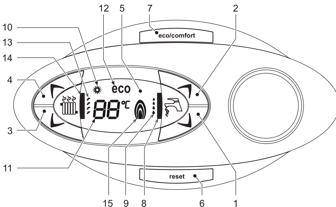
fig. 1 - Pannello di controllo
