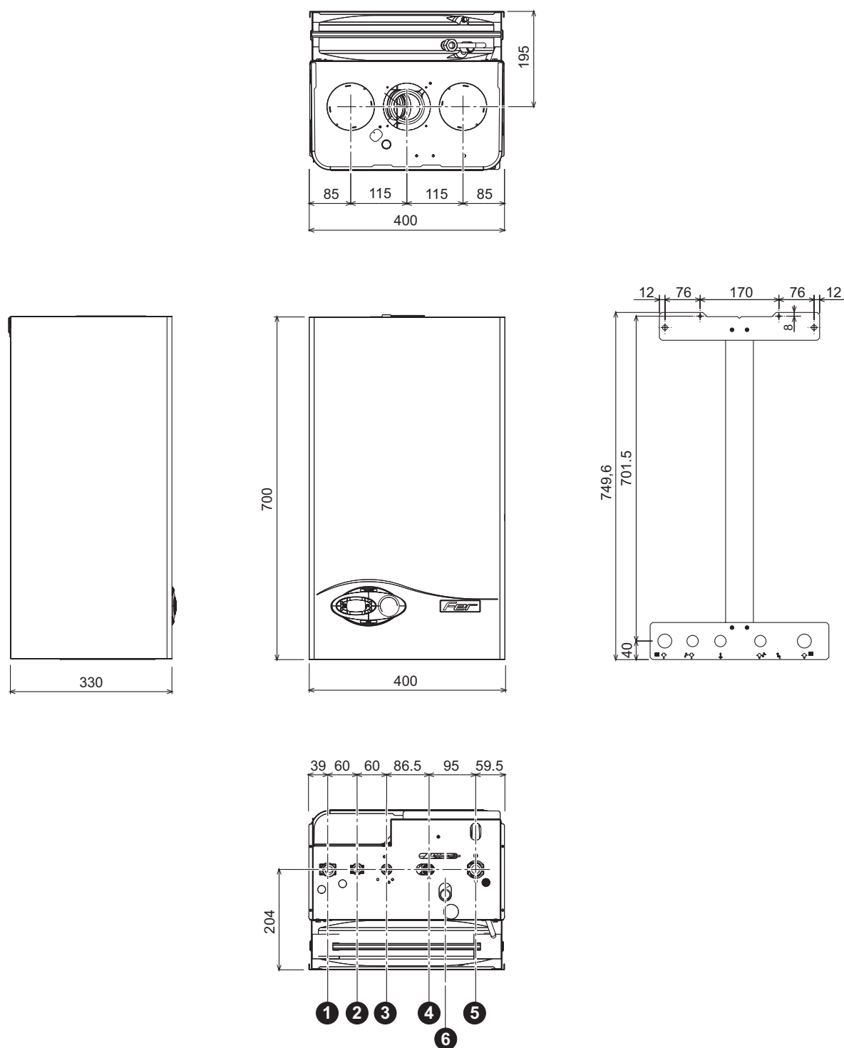
fig. 26 - Dimensioni e attacchi
