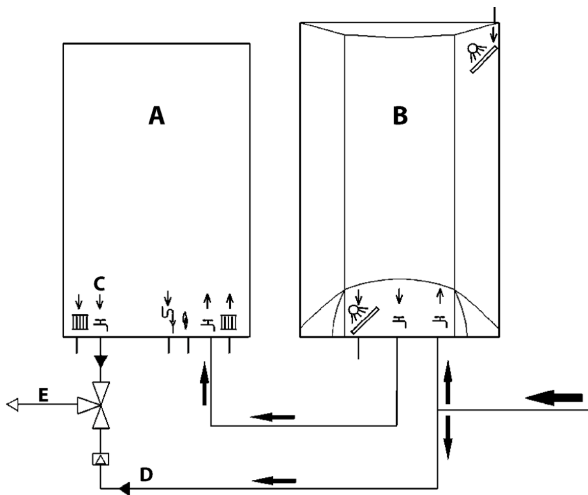
fig. 20 - Schema impianto solare
