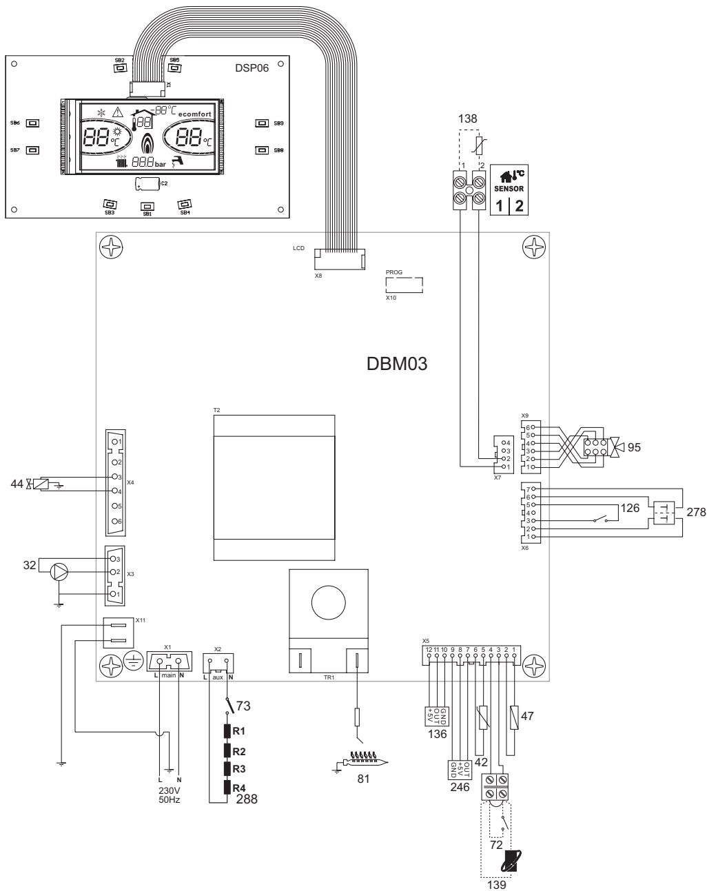
fig. 28 - Schema elettrico
