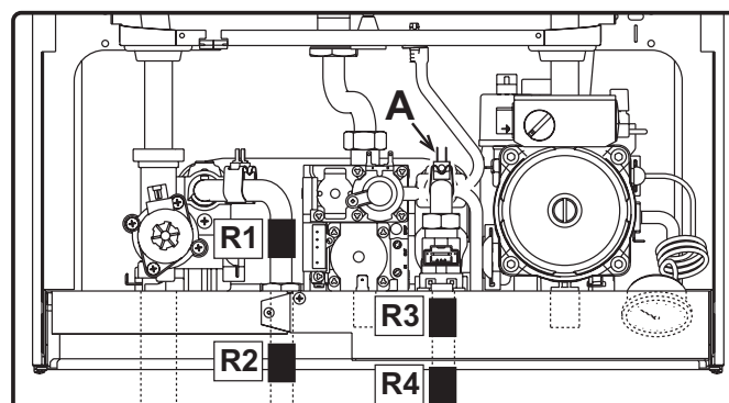
fig. 19 - Posizionamento riscaldatori e termostato antigelo
