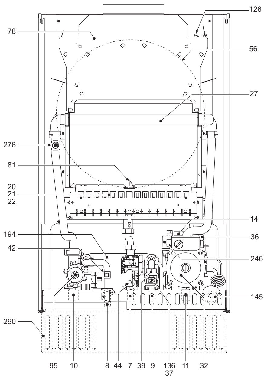
fig. 26 - Vista generale
