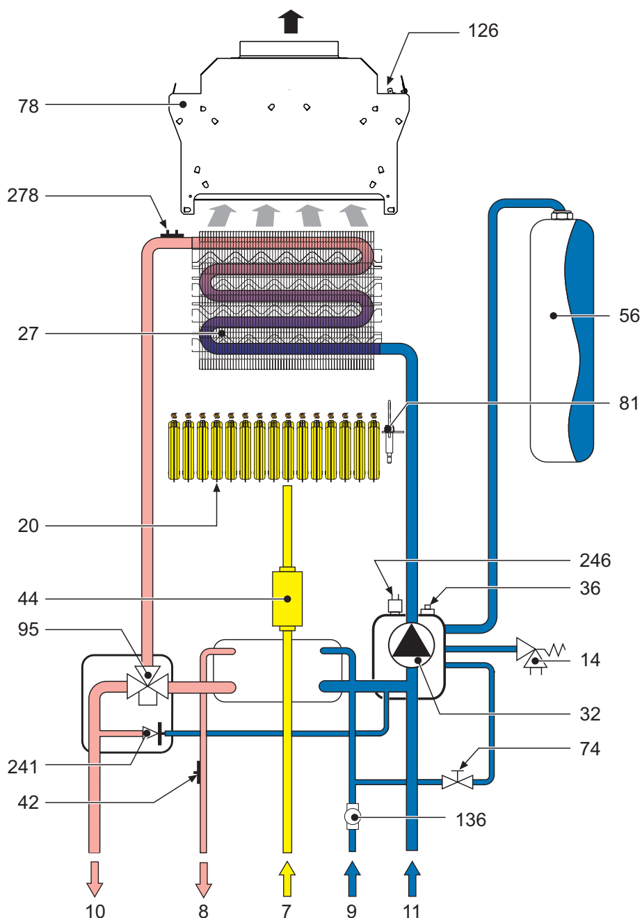
fig. 27 - Circuito idraulico
