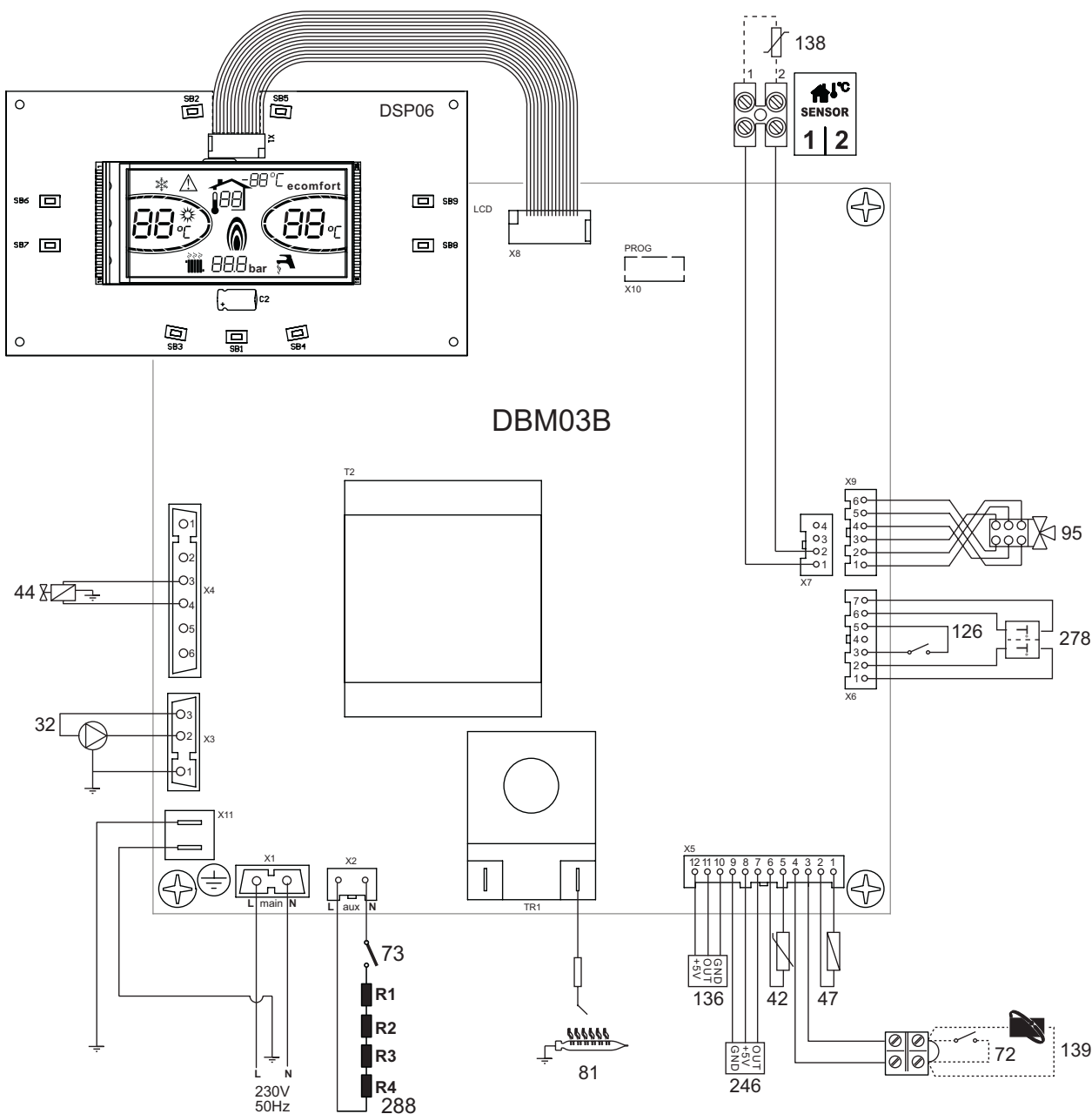
fig. 28 - Schema elettrico
