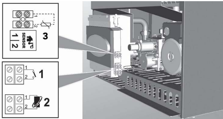
fig. 21 - Accesso alla morsettiera
