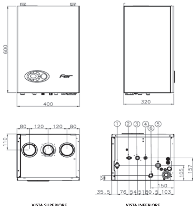
VISTA SUPERIORE
