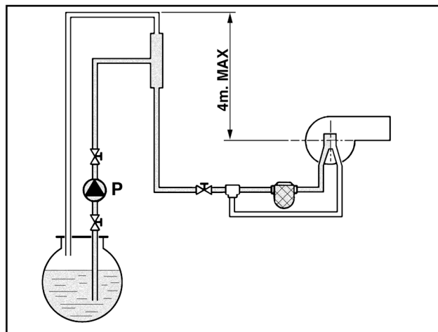
fig. 26 - Alimentation par anneau
