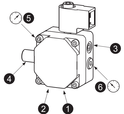
fig. 30 - Pompa DANFOSS
