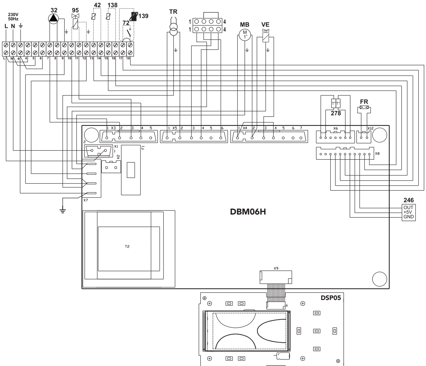
fig. 45 - Schakelschema
