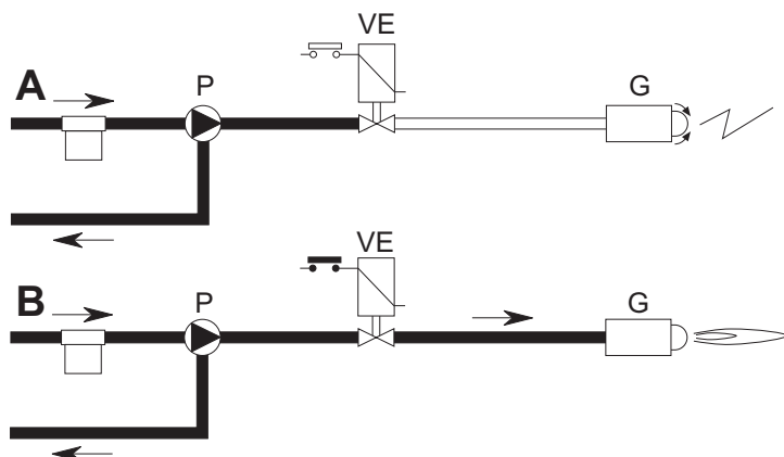
wygląd 34- Zapłon
