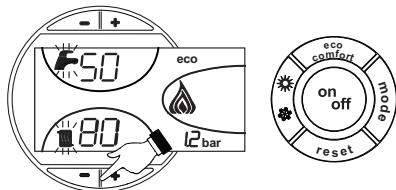
fig. 28 - Modo TEST
