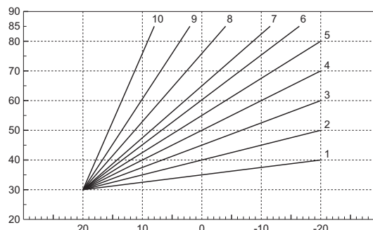
wygląd 13 - Krzywe kompensacji
