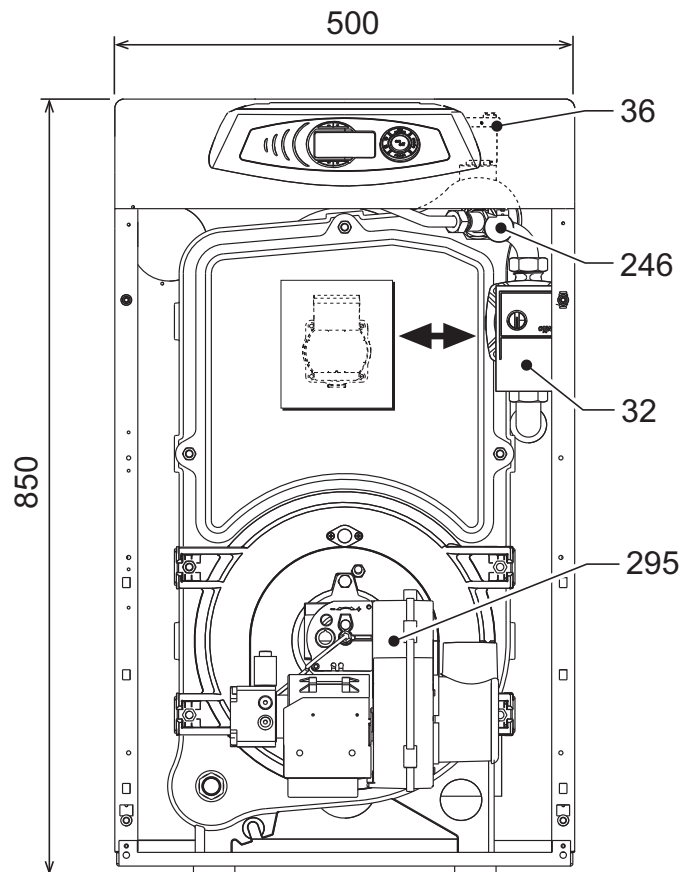
fig. 40- Dimensions raccords et composants principaux
