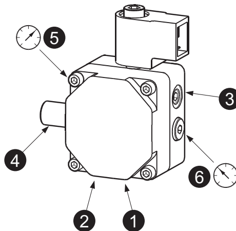
wygląd 30- Pompa DANFOSS
