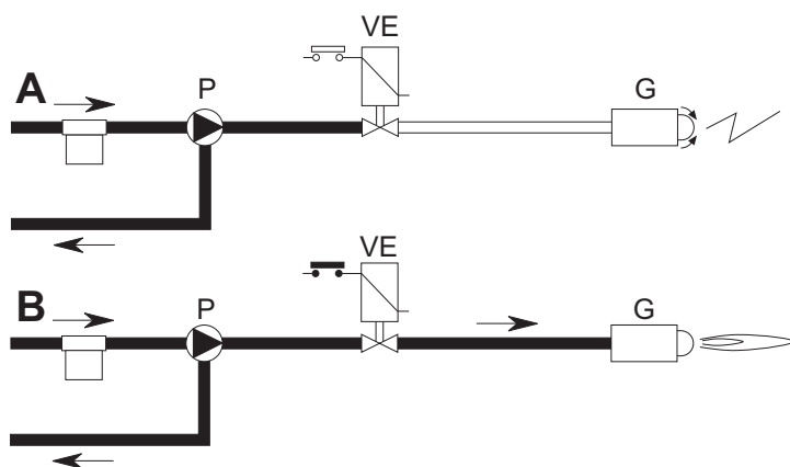
fig. 34 - Allumage
