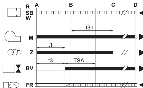
wygląd 35- Cykl urządzenia
