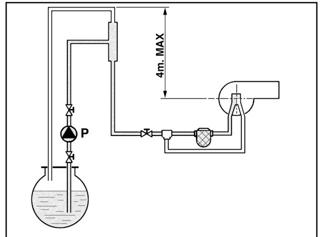
fig. 26 - Alimentación en anillo
