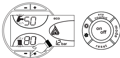
fig. 28 - TEST mode
