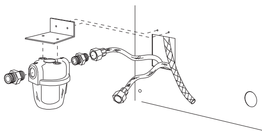
fig. 22 - Installation filtre combustible
