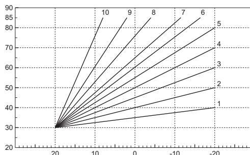
ΕΙΚ. 13 - Καμπύλες αντιστάθμισης
