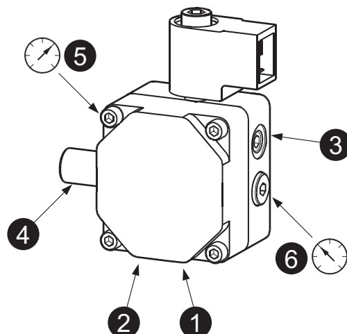
fig. 30- Pompe DANFOSS
