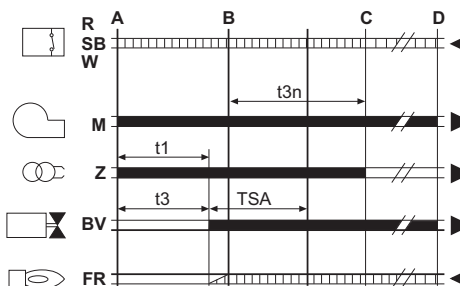
fig. 35 - Cycle de l'appareil
