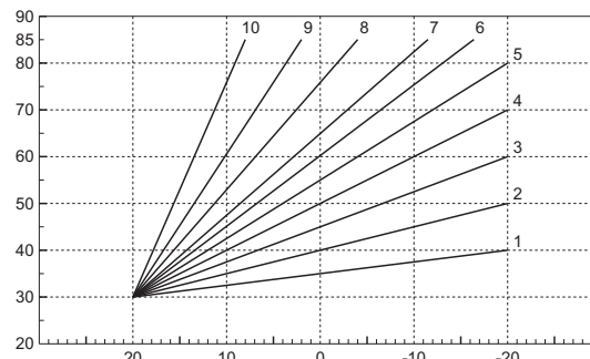
fig. 13 - Compensatiecurven
