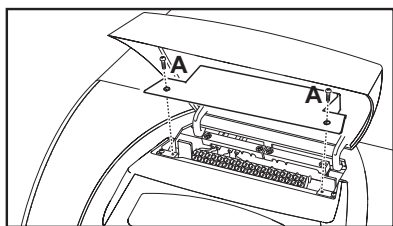
fig. 27 - Accès au bornier
