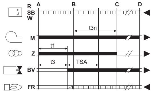
fig. 35 - Ciclo del aparato
