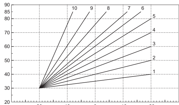
fig. 13 - Curvas de compensación
