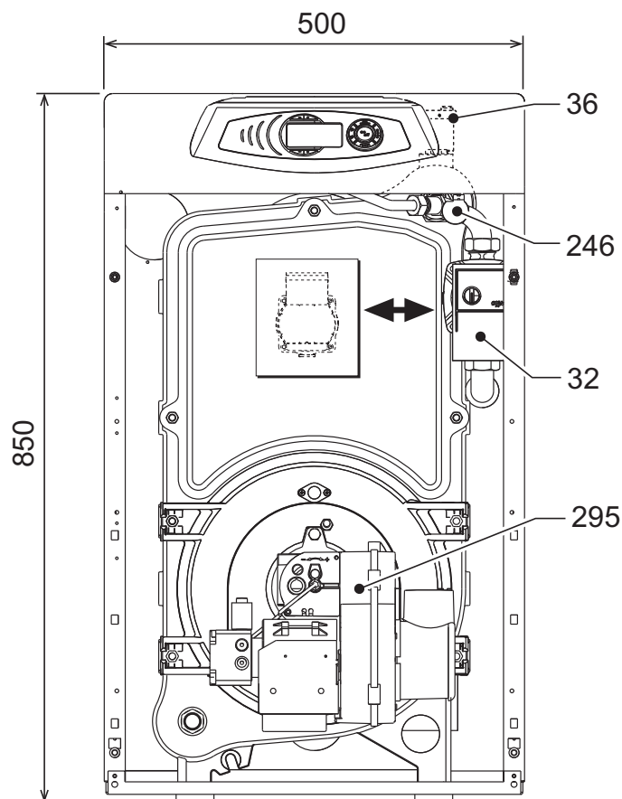
fig. 40- Dimensiones de conexiones y componentes principales
