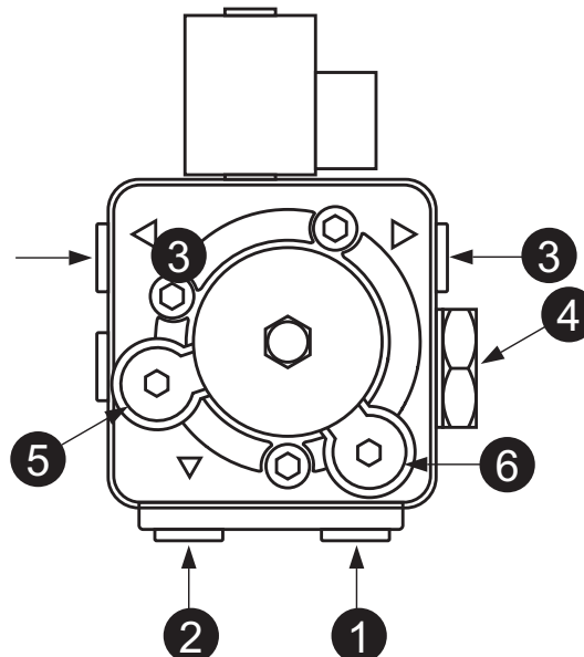
fig. 29- Pomp ITALPUMP
