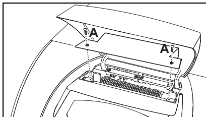
wygląd 27 - Dostęp do elektrycznej skrzynki zaciskowej
