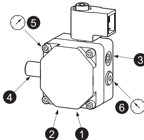
fig. 30- Pomp DANFOSS
