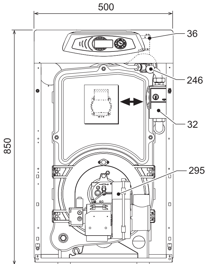
ΕΙΚ. 40- Διαστάσεις, συνδέσεις και κύρια εξαρτήματα
