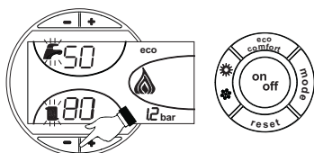
fig. 28 - Functie TEST
