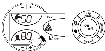
fig. 28 - Fonctionnement en mode TEST
