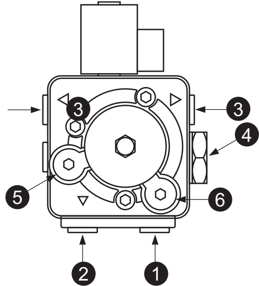
fig. 29 - Pompa ITALPUMP
