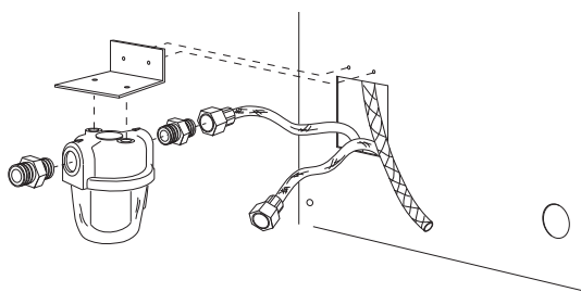
ΕΙΚ. 22 - Τοποθέτηση φίλτρου πετρελαίου
