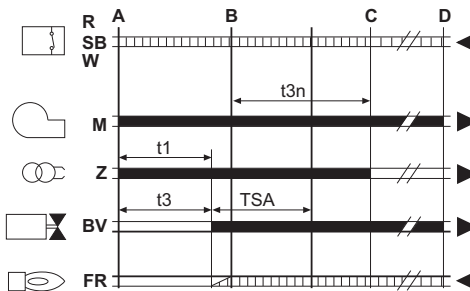
fig. 35 - Cyclus van het apparaat
