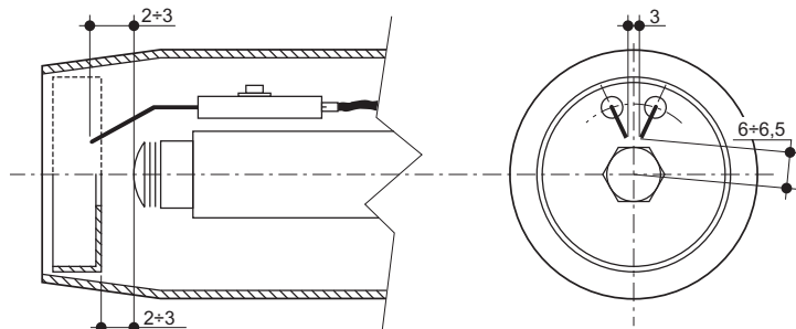
wygląd 33- Pozycja elektrod - deflektora
