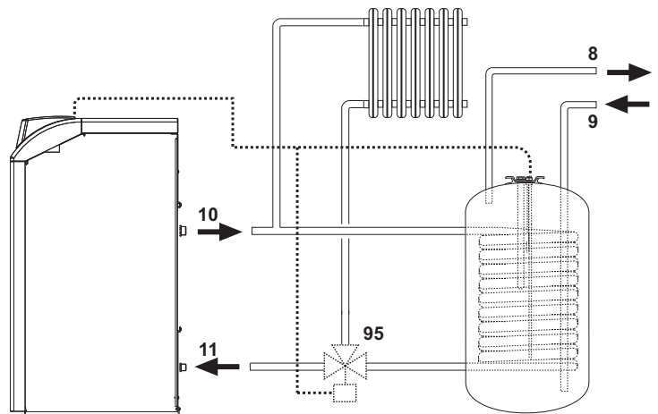
fig. 21 - Schema collegamento ad un bollitore esterno
