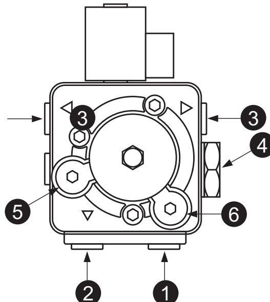
wygląd 29- Pompa ITALPUMP
