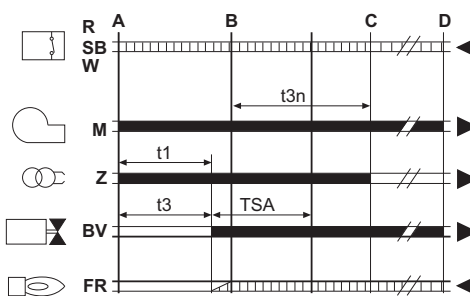
fig. 35 - Ciclo dell'apparecchiatura
