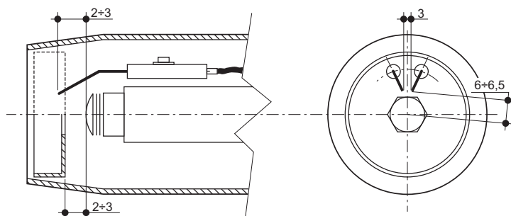
fig. 33 - Position des électrodes - déflecteur
