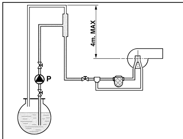
ΕΙΚ. 26 - Τροφοδοσία μέσω δακτυλίου
