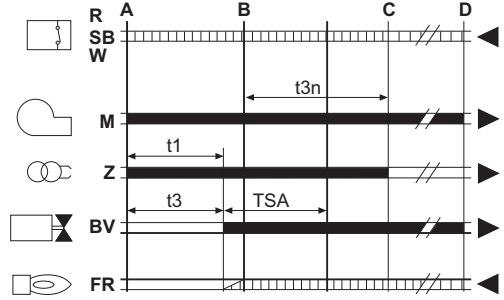
ΕΙΚ. 35 - Κύκλος συσκευής
