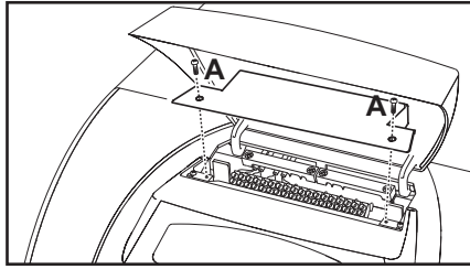
fig. 27 - Accesso alla morsetteria
