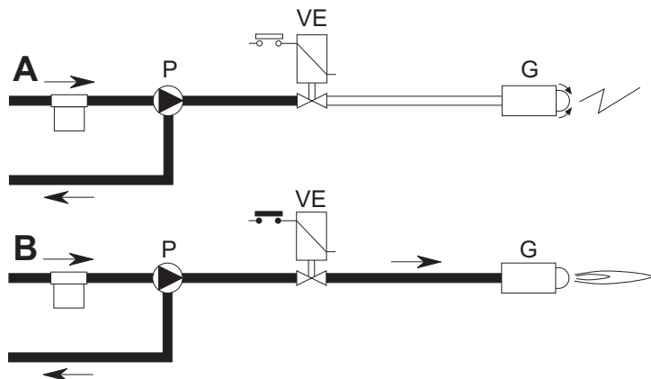
fig. 34 - Aanzetten
