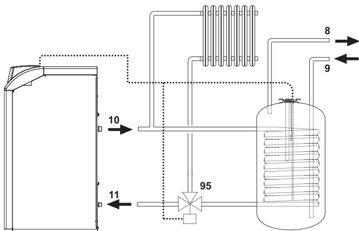
fig. 21 - Schéma de branchement à un ballon externe
