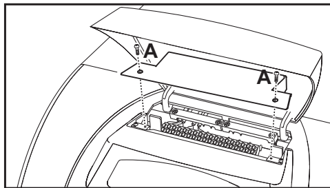
fig. 27 - Acceso a la regleta de conexiones
