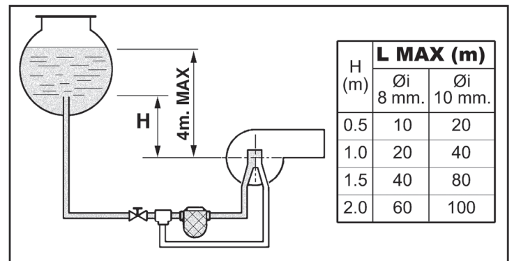
ΕΙΚ. 21 - Τροφοδοσία μέσω βαρύτητας
