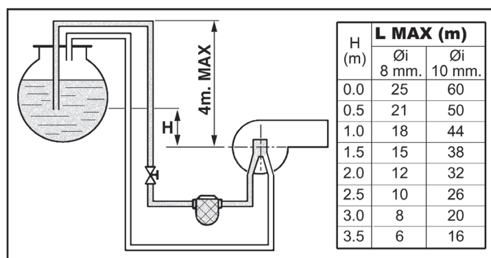
рис. 23 - Сифонная подача
