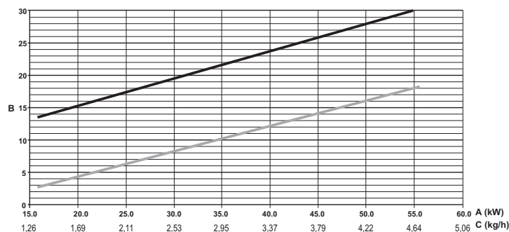
fig. 29 - Grafiek afstellingen brander SUN G6
