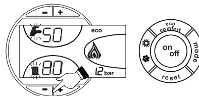
рис. 26 - Работа в режиме TEST
