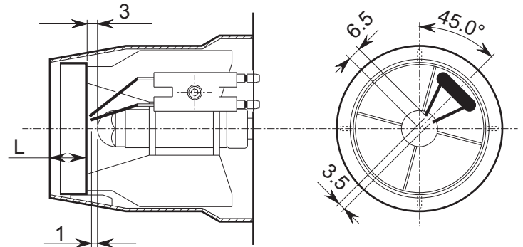
şek. 31 - Elektrot-deflektör/saptırıcı konumu
