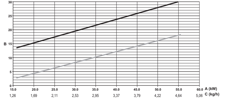
şek. 29 - Brülör ayarları grafiği SUN G6
