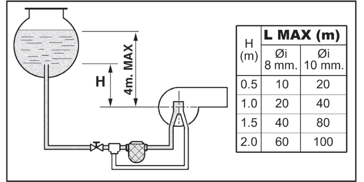
şek. 21 - Ağırlığı ile besleme
