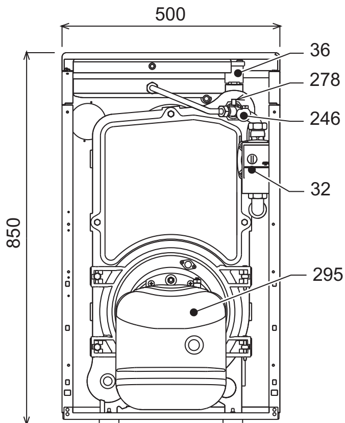
рис. 36 - Размеры, места подключений и основные компоненты
