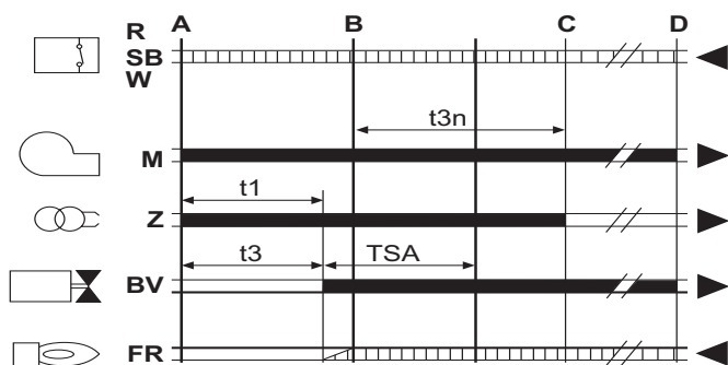
fig. 33 - Cyclus van het apparaat
