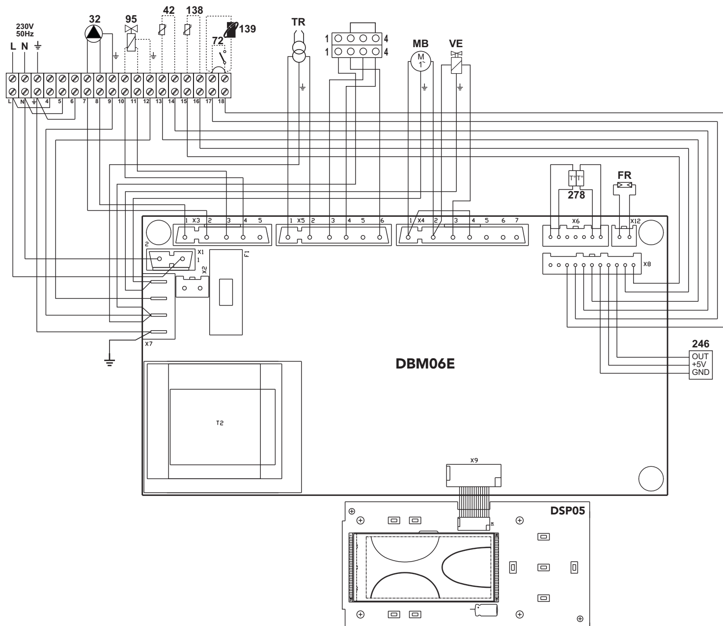
fig. 41 - Schéma électrique
