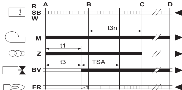
fig. 33 - Ciclo del aparato
