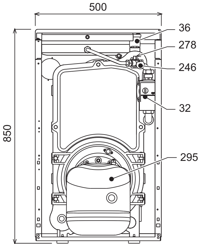
fig. 36 - Dimensiones de conexiones y componentes principales
