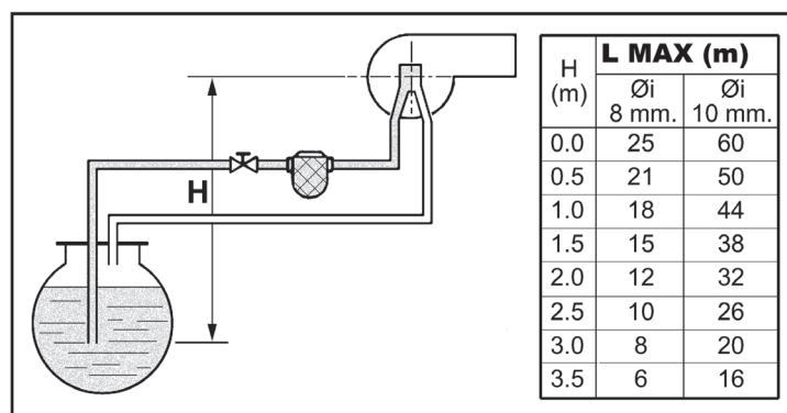
рис. 22 - Подача всасыванием
