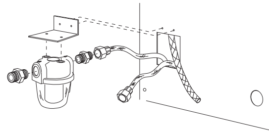
ΕΙΚ. 20 - Τοποθέτηση φίλτρου πετρελαίου
