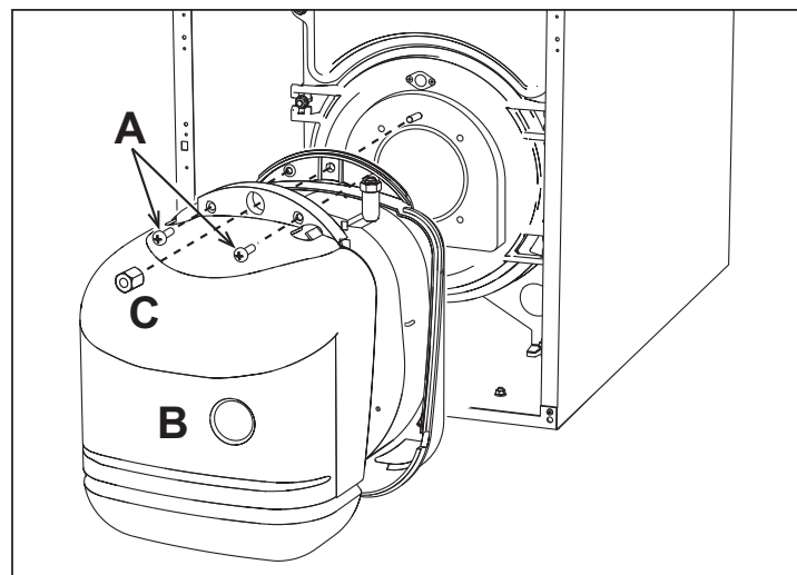
fig. 34 - Demontage van de brander
