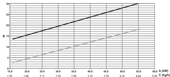
fig. 29 - Gráfico de regulaciones del quemador SUN G6
