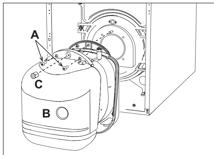
fig. 34 - Smontaggio bruciatore
