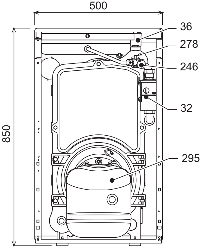
şek. 36 - Bağlantı boyutları ve ana bileşenler
