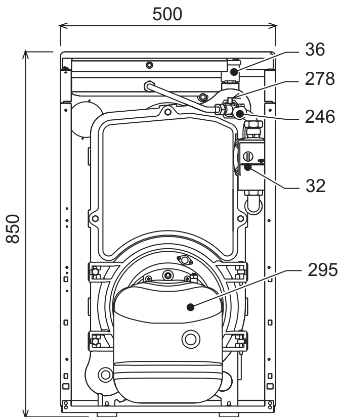
fig. 36 - Afmetingen aansluitingen en hoofdcomponenten
