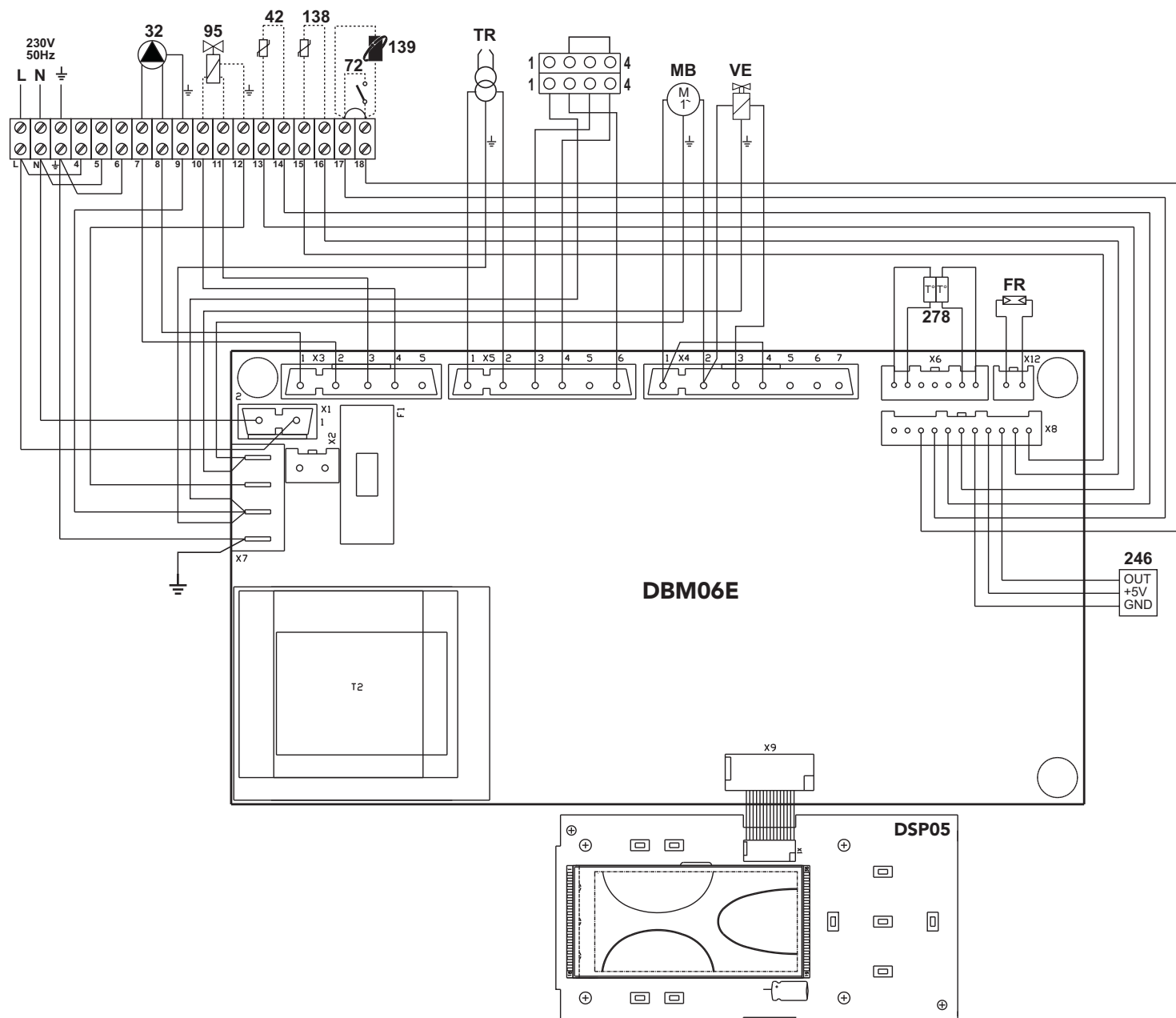
fig. 41 - Schakelschema
