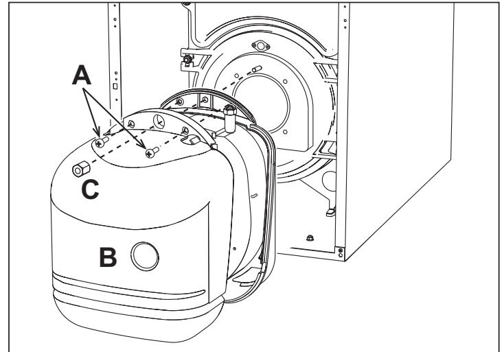
şek. 34 - Brülörün sökülmesi
