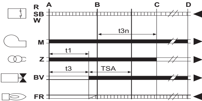
şek. 33 - Cihaz döngüsü
