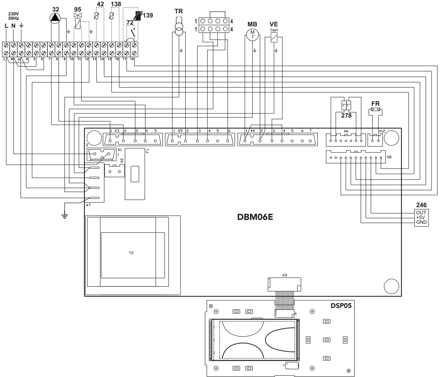
şek. 41 - Elektrik şeması
