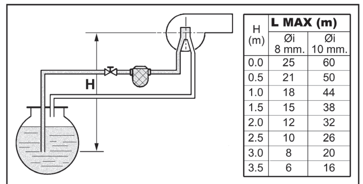
ΕΙΚ. 22 - Τροφοδοσία μέσω αναρρόφησης
