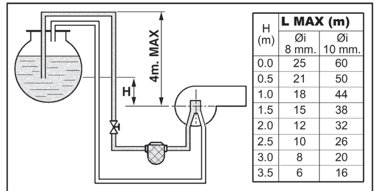
şek. 23 - Sifon yöntemiyle besleme
