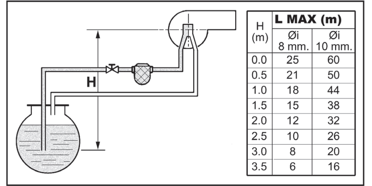
şek. 22 - Emiş yoluyla besleme
