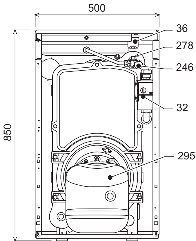
ΕΙΚ. 36 - Διαστάσεις, συνδέσεις και κύρια εξαρτήματα
