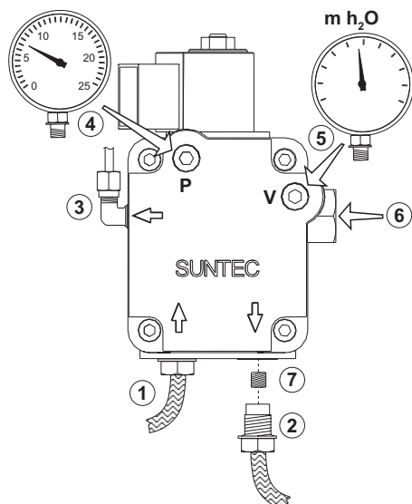
fig. 27 - Pomp SUNTEC
