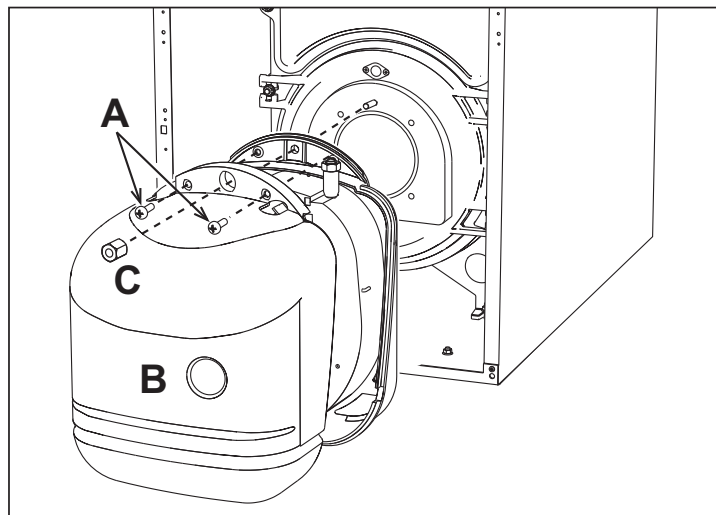
рис. 34 - Демонтаж горелки
