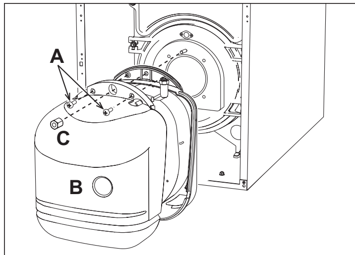
fig. 34 - Démontage du brûleur
