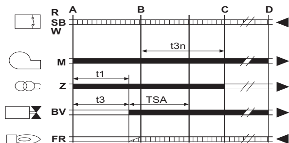
fig. 33 - Ciclo dell'apparecchiatura
