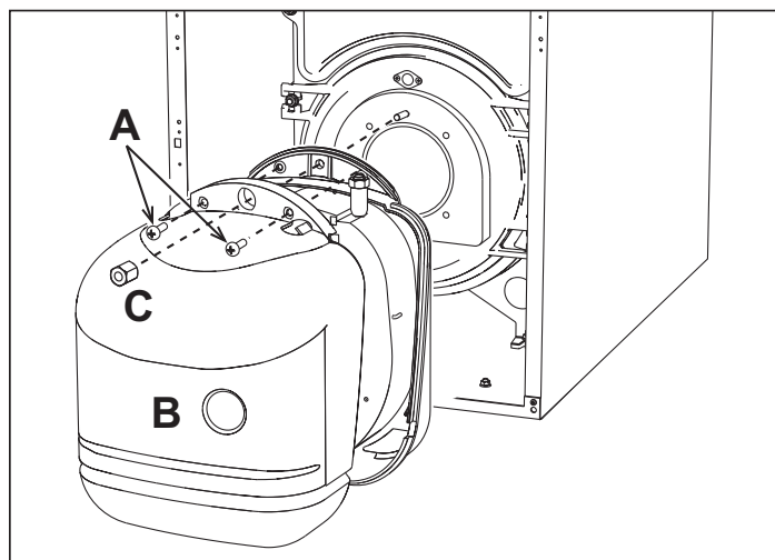
ΕΙΚ. 34 - Αποσυναρμολόγηση καυστήρα
