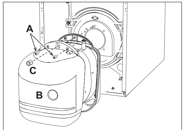
fig. 34 - Desmontaje del quemador
