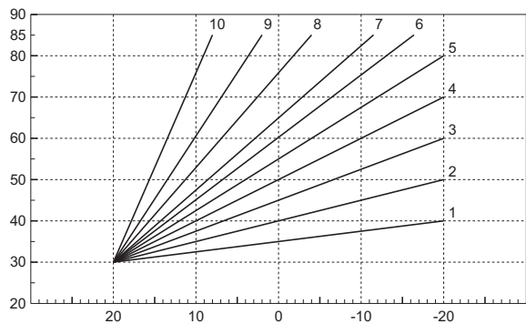
fig. 13 - Compensatiecurven
