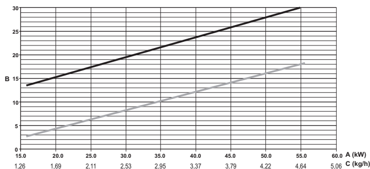
рис. 29 - График регулировки горелки SUN G6
