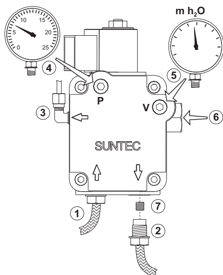
fig. 27 - SUNTEC pump
