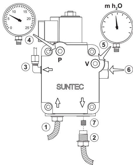
εικ. 27 - Αντλία SUNTEC
