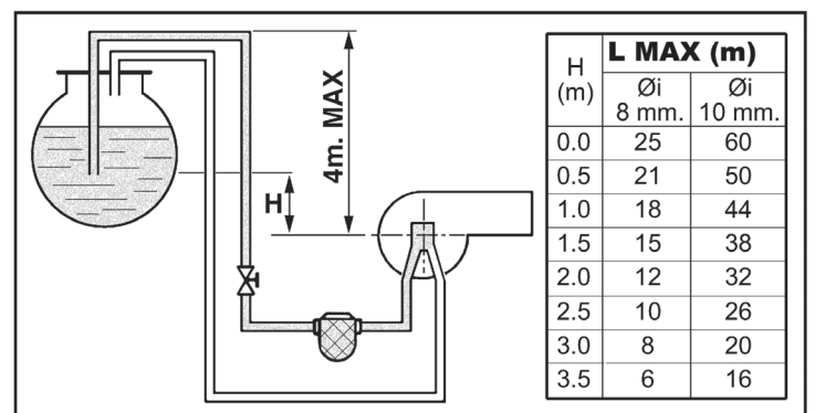
ΕΙΚ. 23 - Τροφοδοσία μέσω σιφονιού
