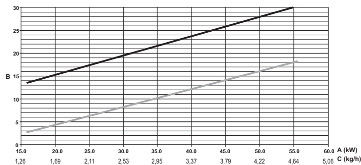
εικ. 29 - Γράφημα ρυθμίσεων καυστήρα SUN G6
