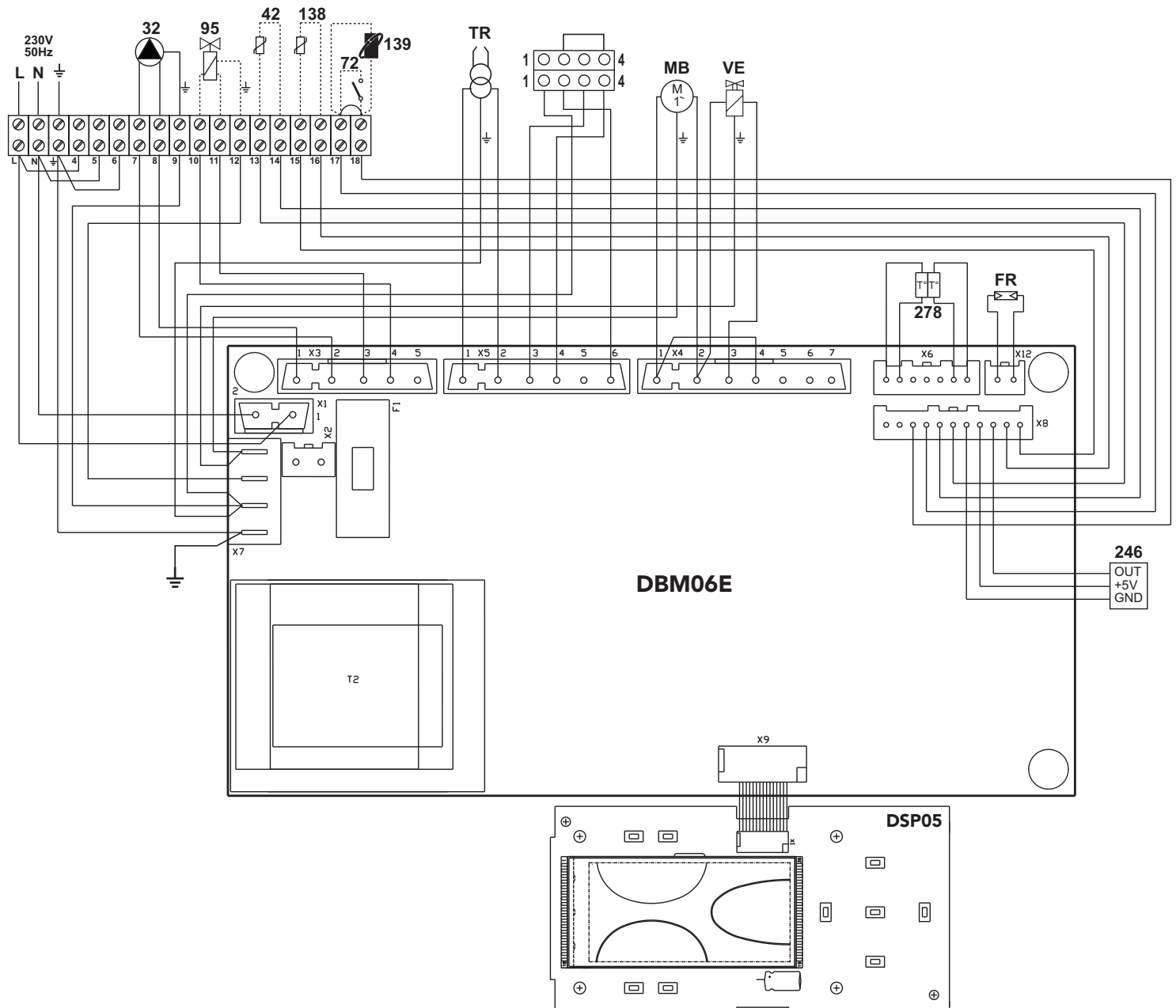
fig. 41 - Schema elettrico
