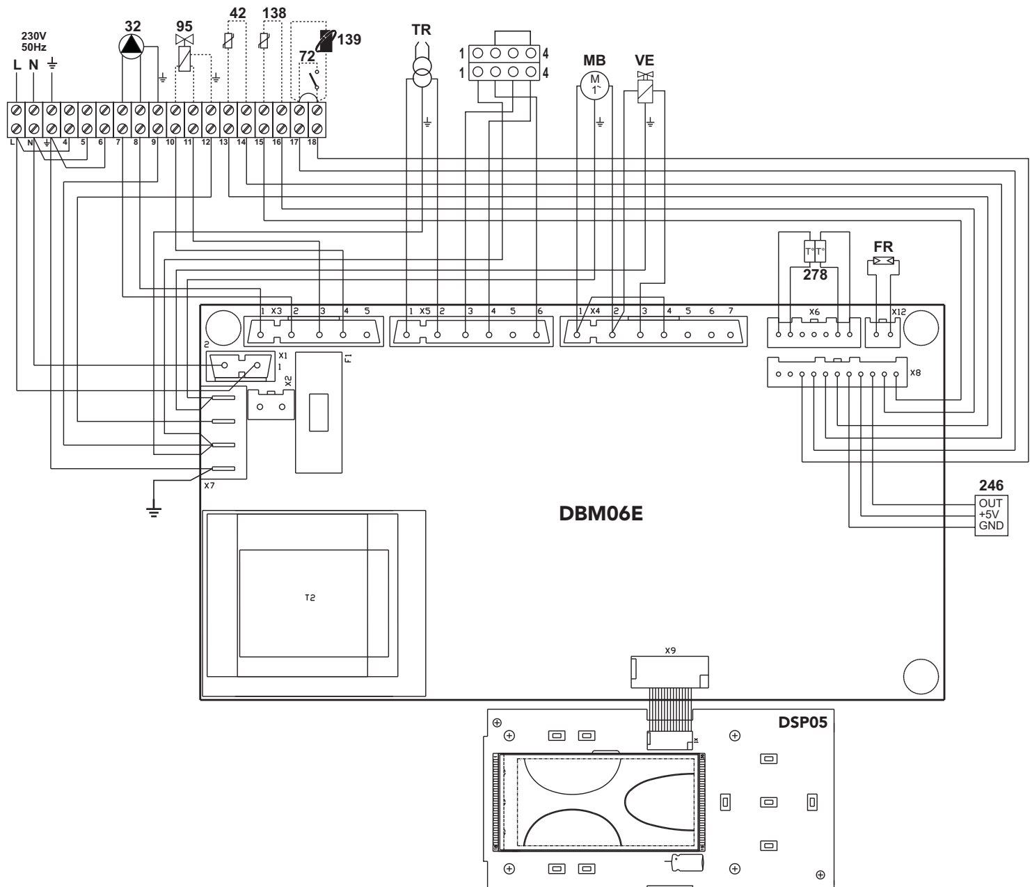
fig. 41 - Esquema eléctrico
