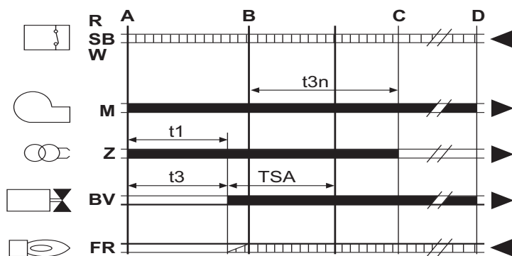
fig. 33 - Cycle de l'appareil
