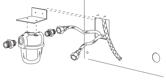
şek. 20 - Yakıt filtresinin takılması
