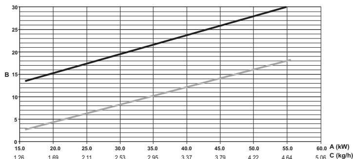
fig. 29 - Graphique réglages brûleur SUN G6
