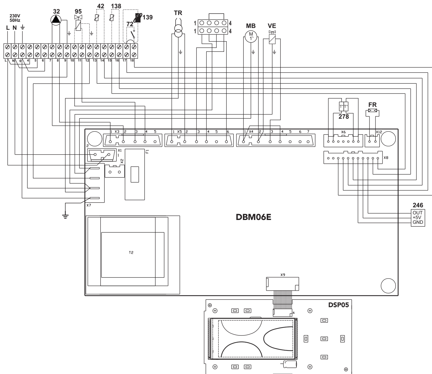
ΕΙΚ. 41 - Ηλεκτρολογικό διάγραμμα
