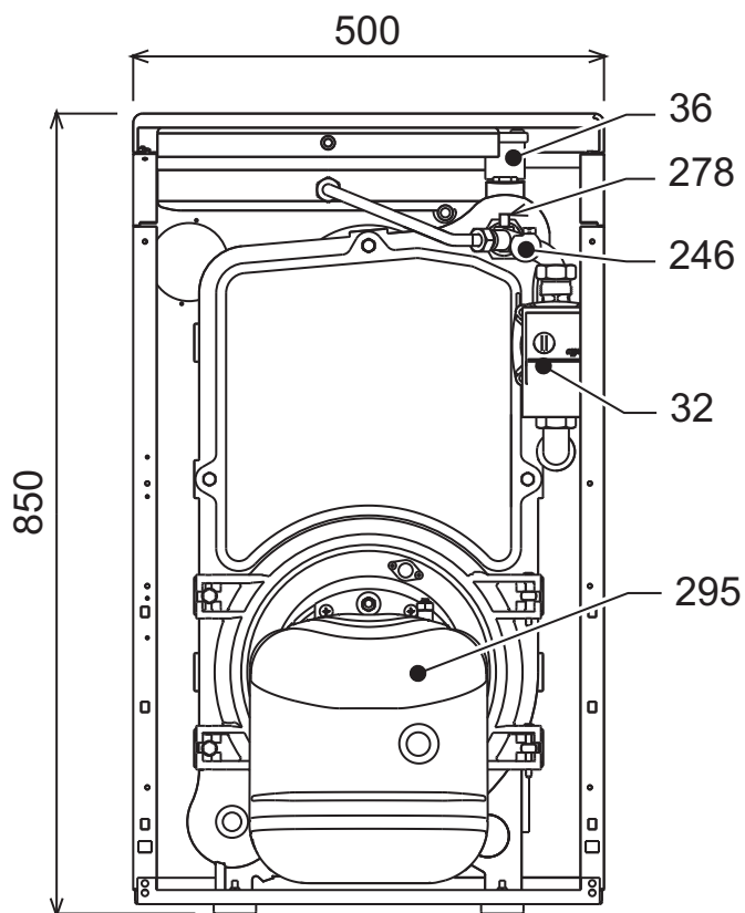
fig. 36 - Dimensions raccords et composants principaux
