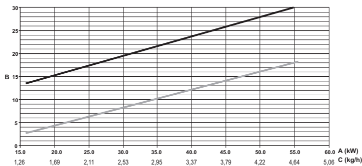
fig. 29 - Grafico regolazioni bruciatore SUN G6
