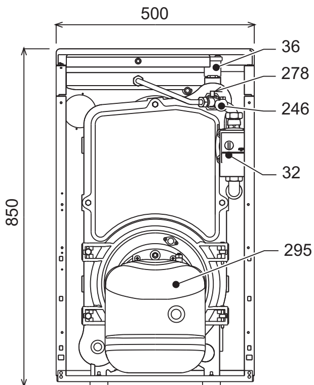
fig. 36 - Dimensionale attacchi e componenti principali
