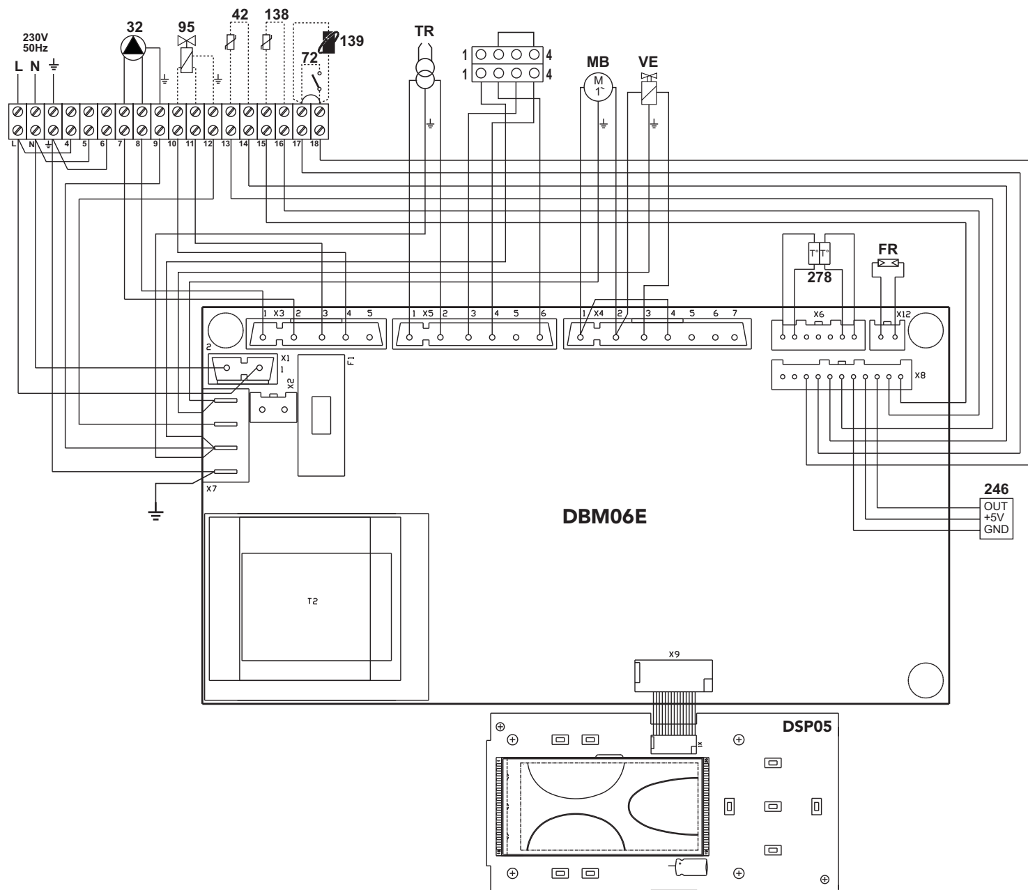
fig. 41 - Wiring diagram
