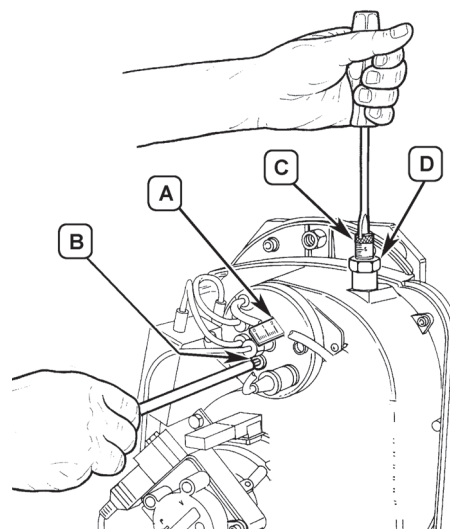
fig. 30 - Afstellen brander
