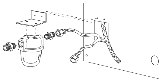
рис. 20 - Установка топливного фильтра
