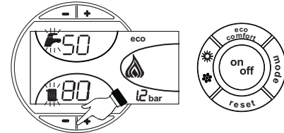
fig. 26 - Modalità TEST
