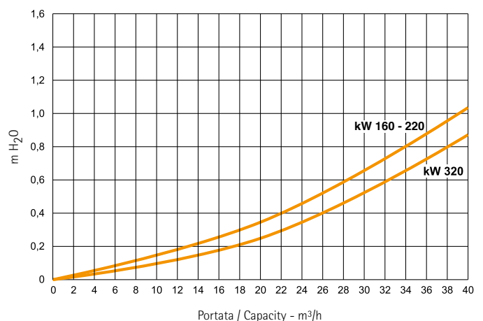
OPERA 160 - 220 - 320
