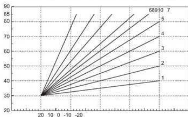
fig. 30 - Curve di compensazione
