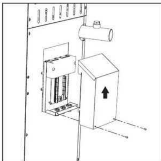
fig. 55- Bornier électrique
