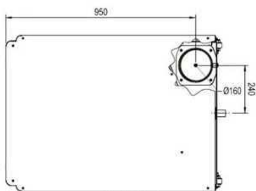
fig. 82- Haut
