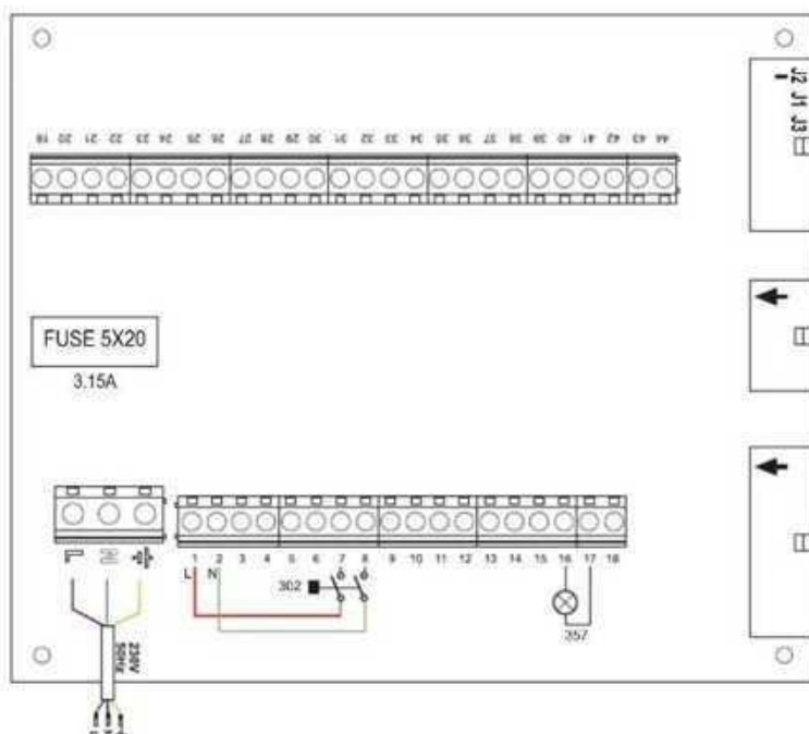
fig. 52- ESCLAVA
