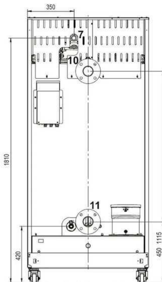
fig. 84 - Vista posteriore modello 320
