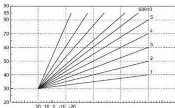
рис. 30- Компенсационные кривые
