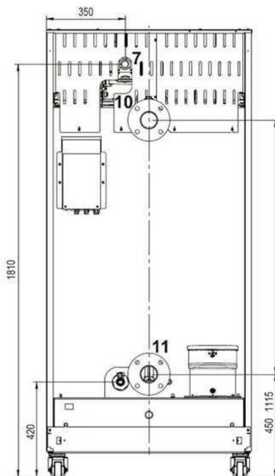
fig. 84- Vista posterior modelo 320
