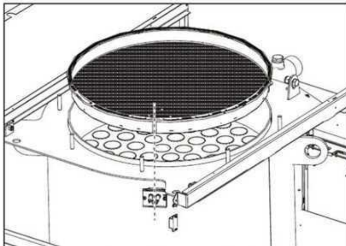
fig. 67 - Alineación del quemador
