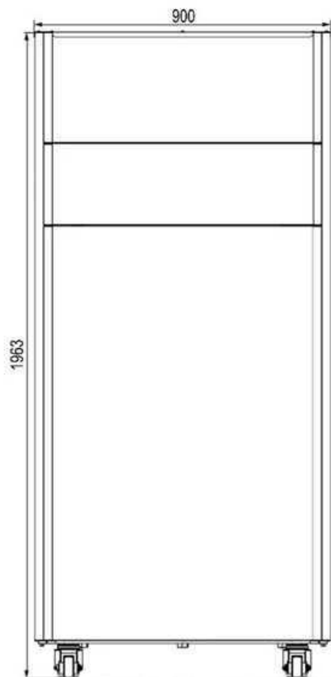
fig. 83- Vista frontal modelo 320
