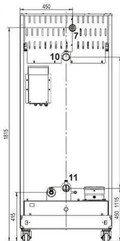
fig. 80- posterior 160
