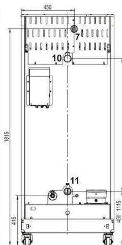
fig. 80- Arrière 160
