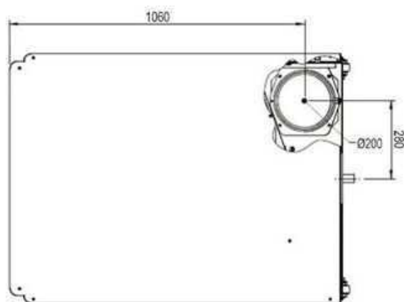
fig. 85- Vue du haut modèle 320
