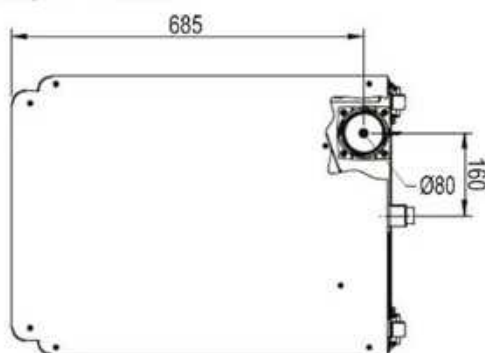
fig. 75 - Superiore
