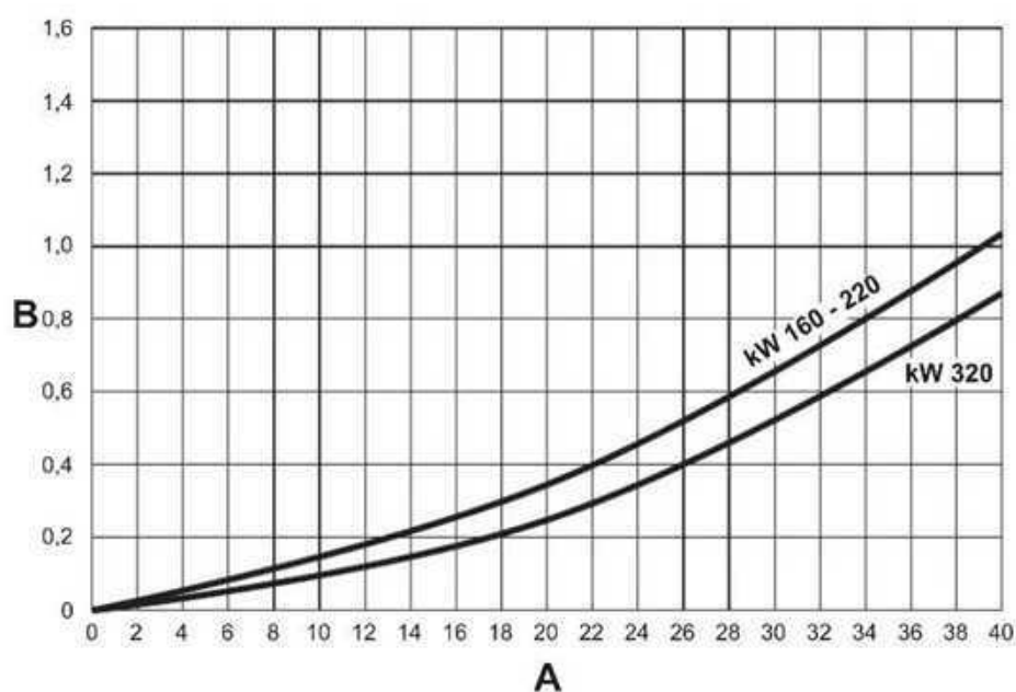
fig. 91 - Diagramma perdita di carico modelli 220, 320 e 450
