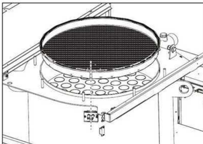
fig. 67 - Alignement du brûleur
