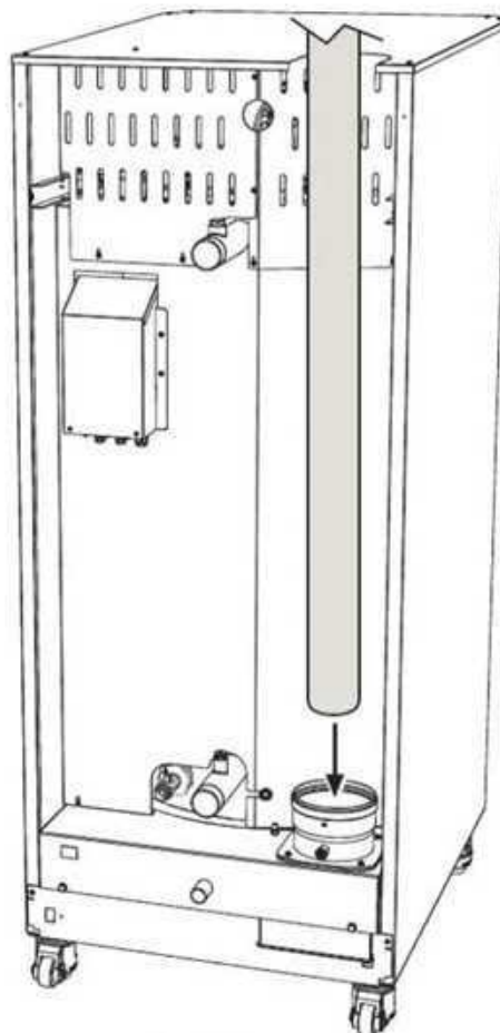
fig. 57- Fume outlet
