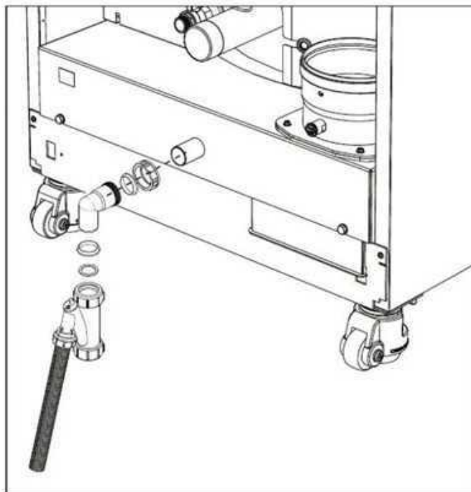
fig. 58 - Collegamento scarico condensa
