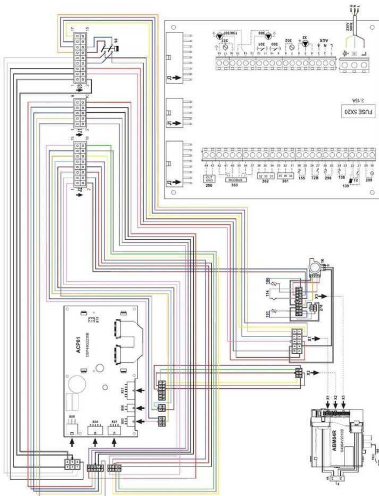
fig. 96- Schéma électrique OPERA 125 et 160
