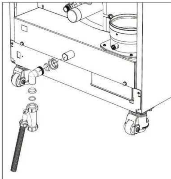
fig. 58- Conexión de la descarga de condensado
