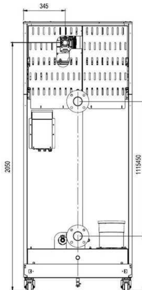
fig. 87 - Vista posteriore modello 450
