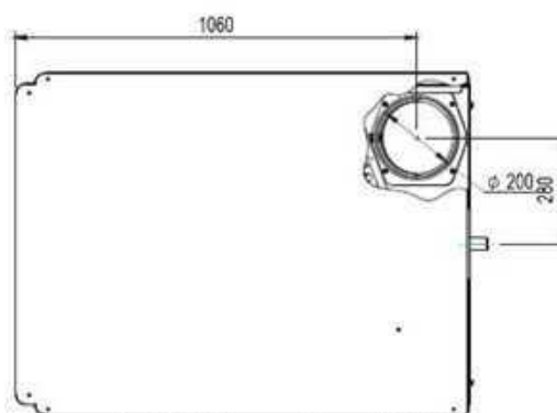
fig. 88- Vista superior modelo 450
