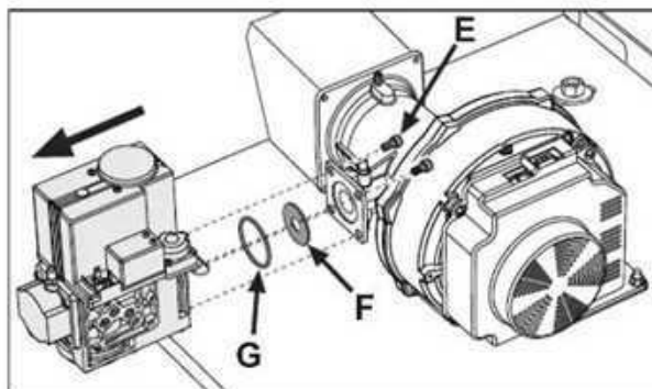
fig. 62- Modèle OPERA 320 et OPERA 450
