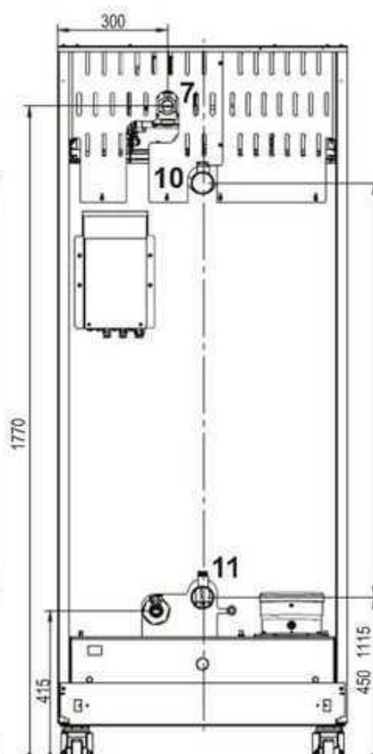
fig. 81- posterior 220
