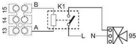
fig. 92 - Collegamento della valvola a 3 vie con 2 fili
