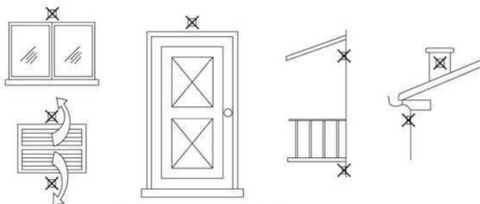
fig. 54- Posición desaconsejada de la sonda exterior
