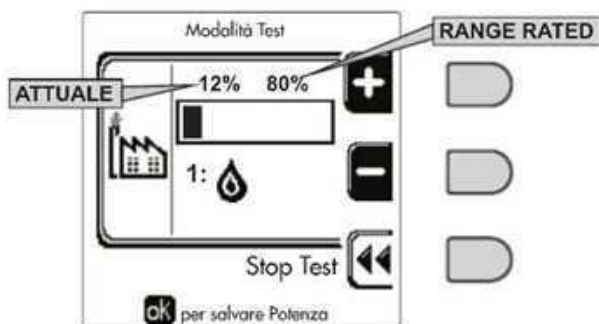
fig. 64 - Modalità TEST (esempio potenza riscaldamento = 80%)
