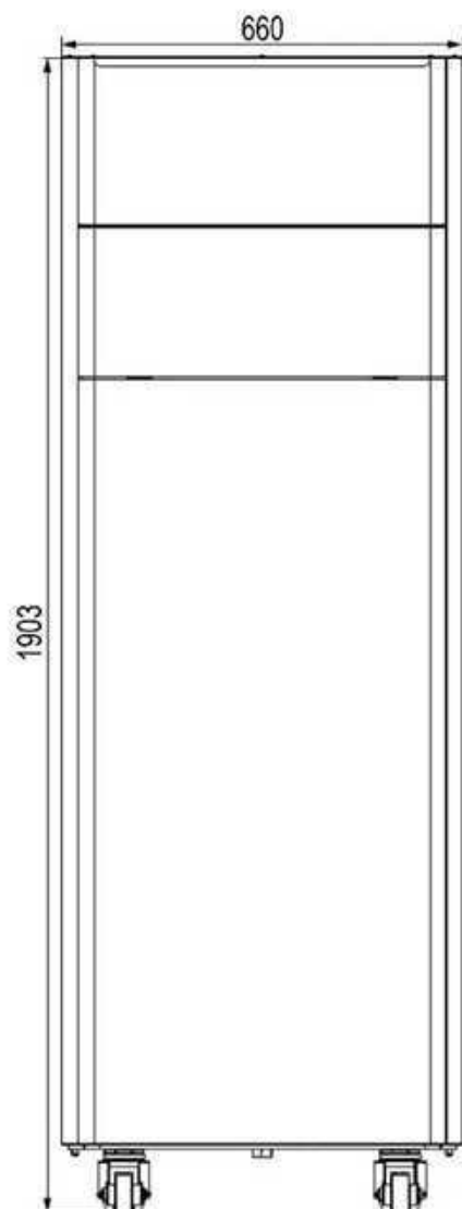
fig. 76 - anteriore fig. 77 - posteriore
