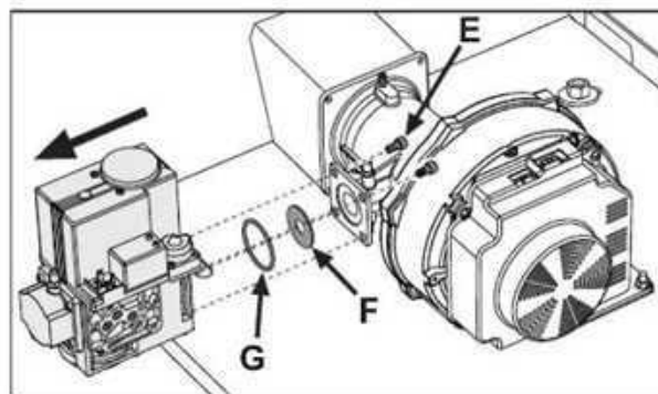
fig. 62- Modelo OPERA 320 y OPERA 450
