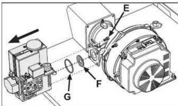
fig. 62 - Modello OPERA 320 e OPERA 450
