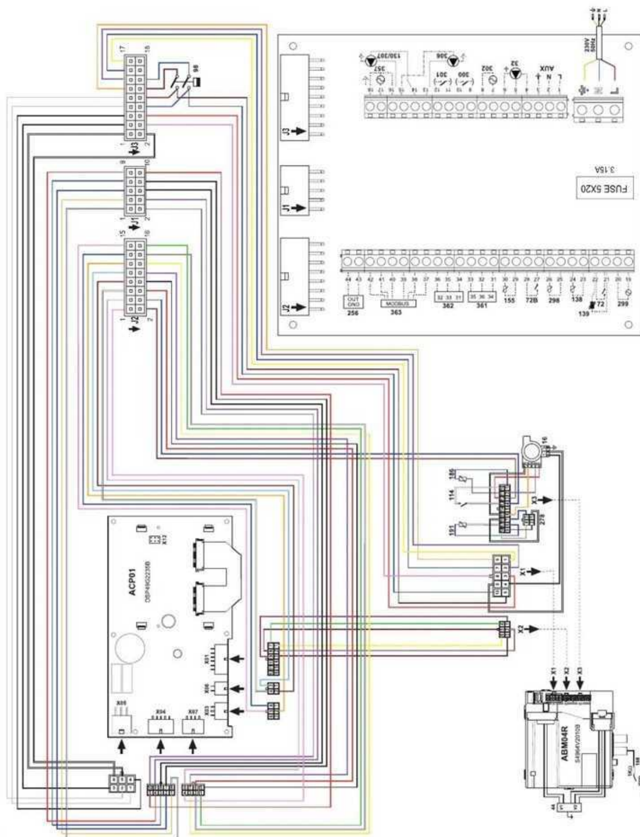
fig. 96- Esquema eléctrico OPERA 125 y 160
