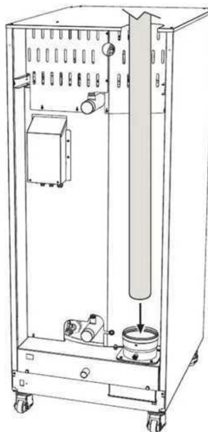
fig. 57 - Uscita fumi
