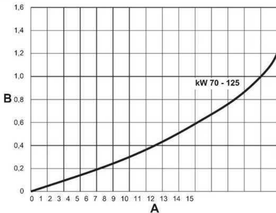
fig. 90 - Diagramma perdita di carico modelli 70 - 125
