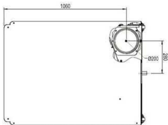
fig. 85- Vista superior modelo 320
