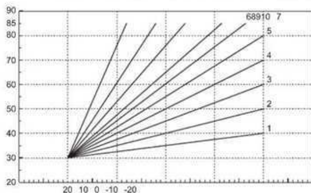
fig. 30- Courbes de compensation
