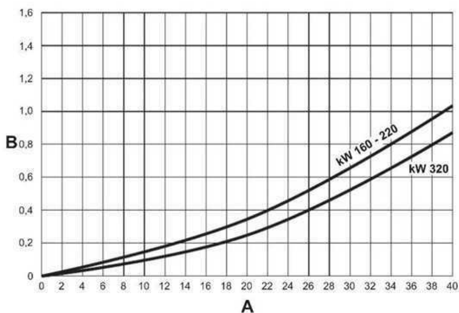
fig. 91 - Diagrama de pérdidas de carga modelos 220, 320 y 450
