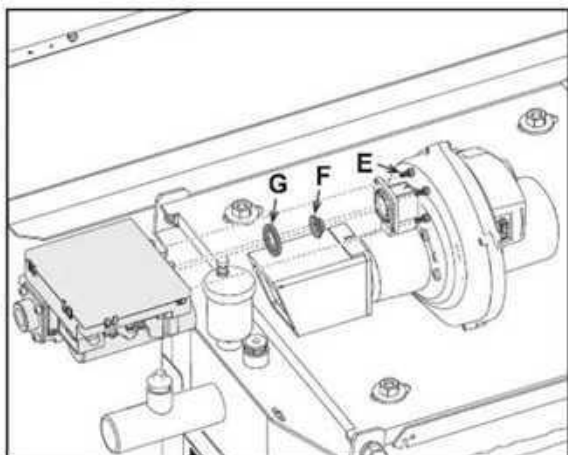
fig. 60- Modelo OPERA 125 y OPERA 160
