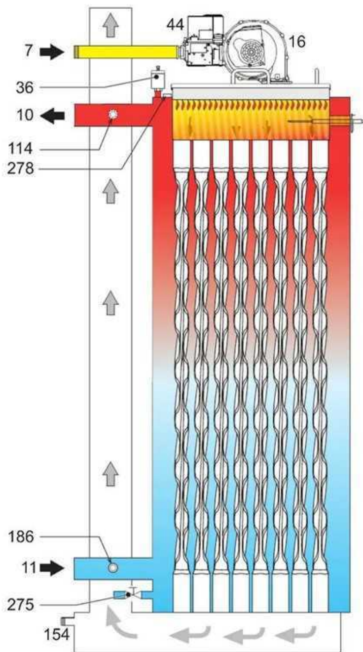
fig. 89- Circuit hydraulique
