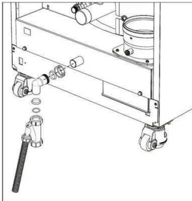
fig. 58- Raccordement de l'évacuation des condensats
