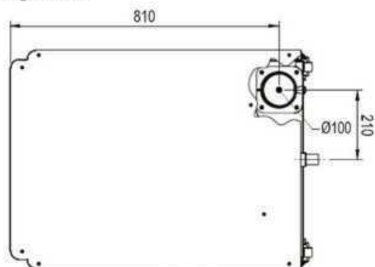
fig. 78- top
