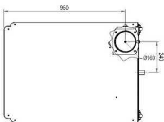
fig. 82 - superiore
