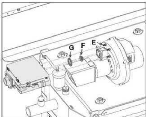
fig. 60- Modèle OPERA 125 et OPERA 160
