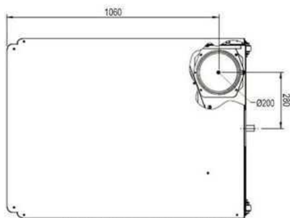
fig. 85 - Vista superiore modello 320
