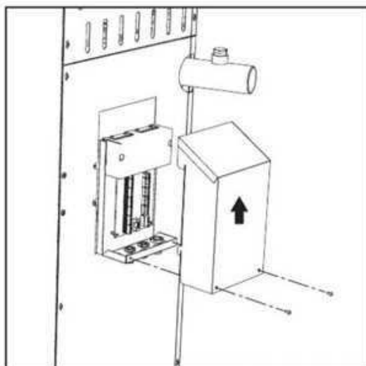
fig. 55- Regleta eléctrica
