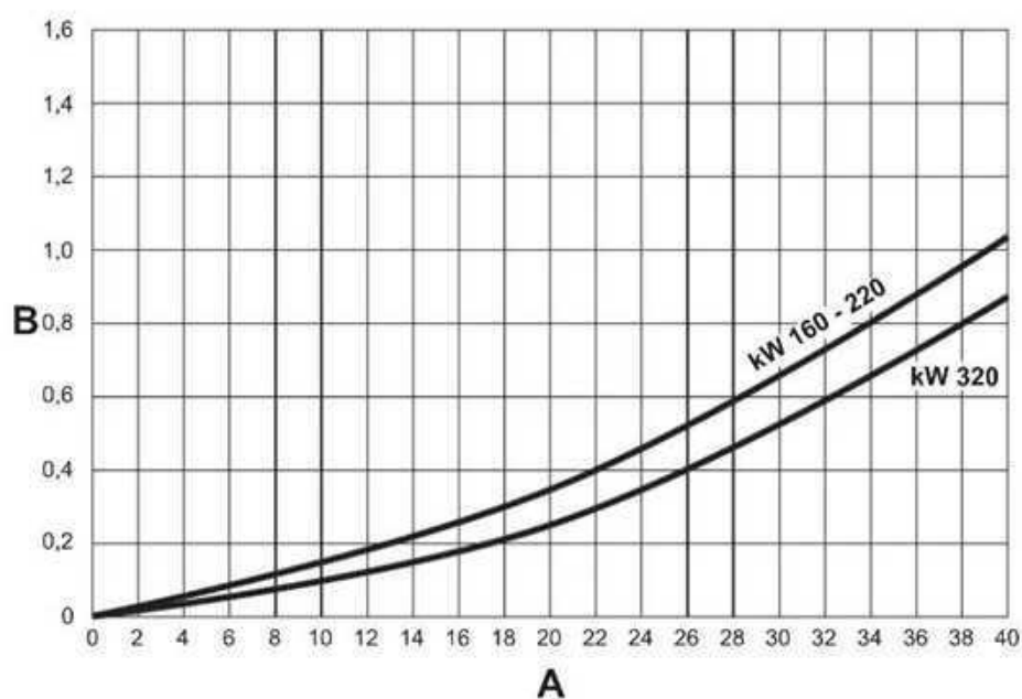
fig. 91 - Diagramme perte de charge modèles 220, 320 et 450
