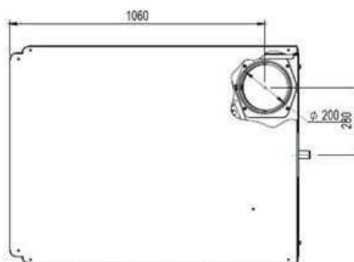
fig. 88- Vue du haut modèle 450
