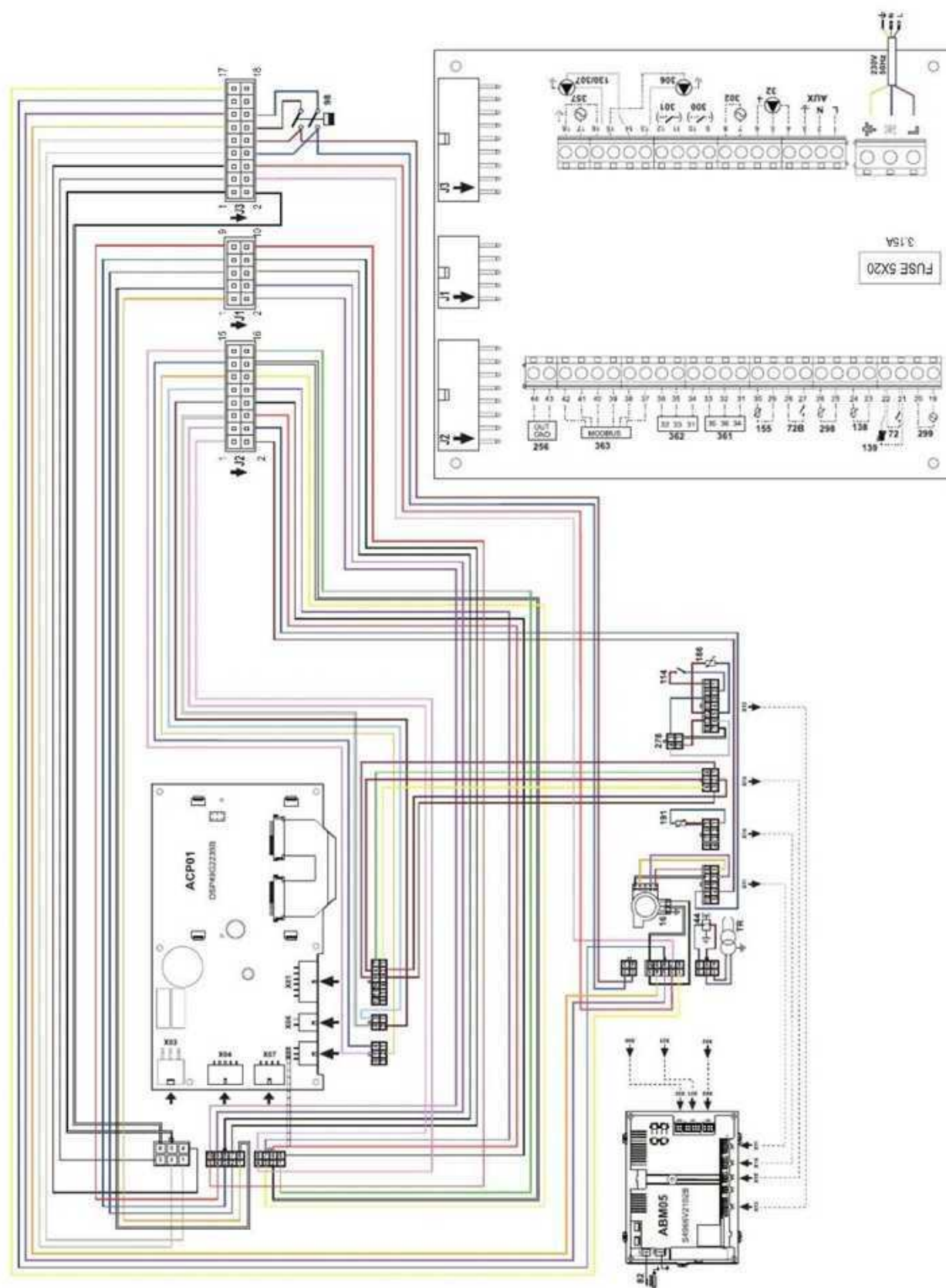
fig. 97 - Schema elettrico OPERA 220/320 e OPERA 450
