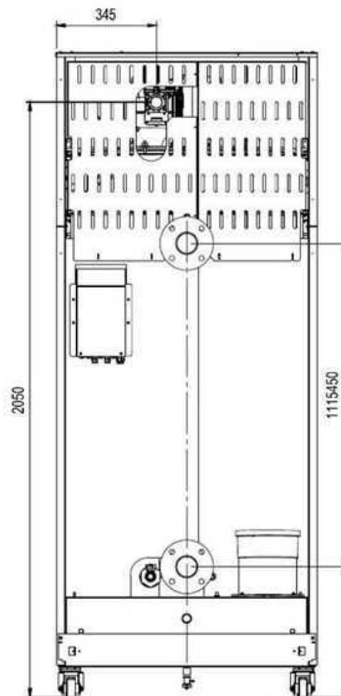
fig. 87- Vue arrière modèle 450
