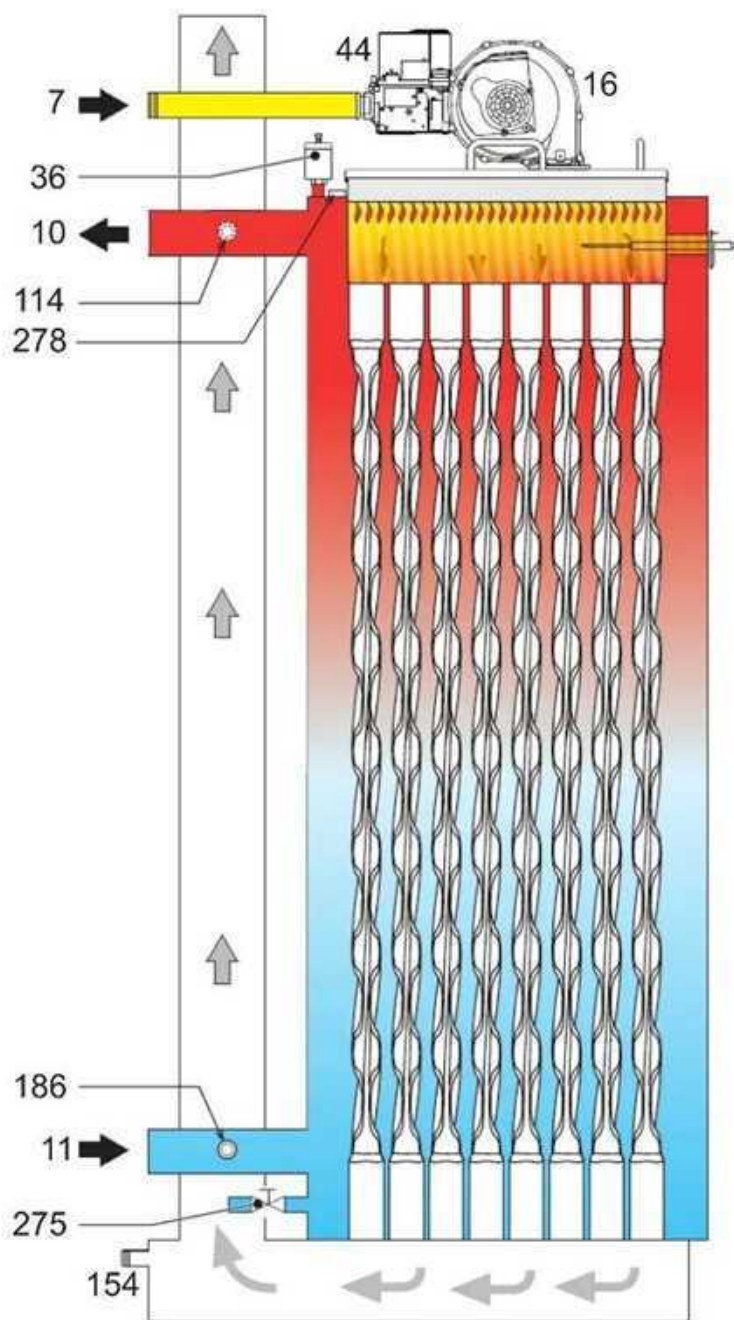
fig. 89 - Circuito idraulico
