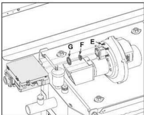
fig. 60 - Modello OPERA 125 e OPERA 160
