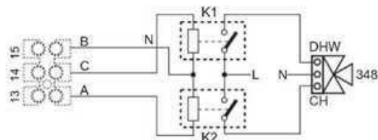
fig. 93- Conexión de la válvula de 3 vías con 3 hilos
