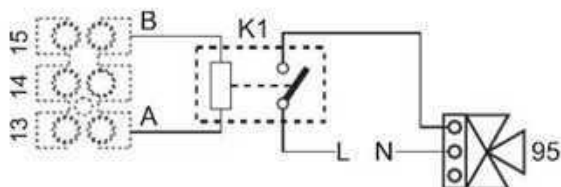
fig. 92- Raccordement de la vanne 3 voies à 2 fils
