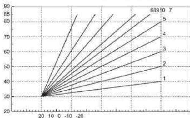
fig. 30- Curvas de compensación
