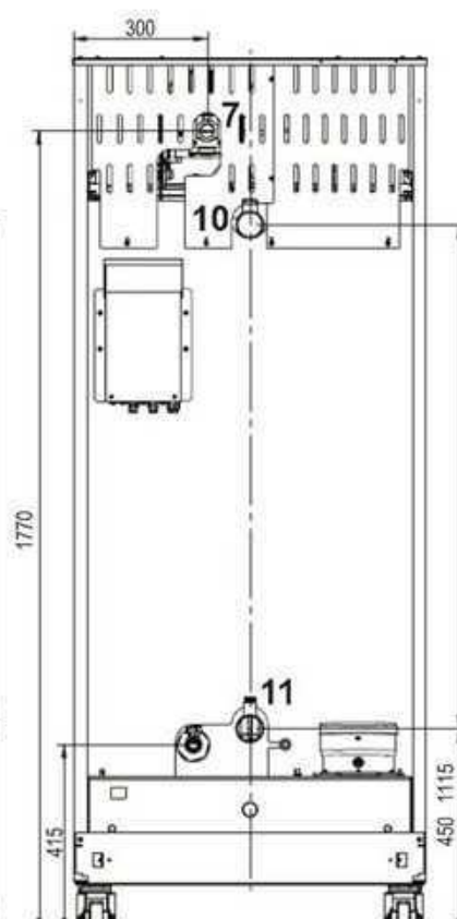
fig. 81- Arrière 220
