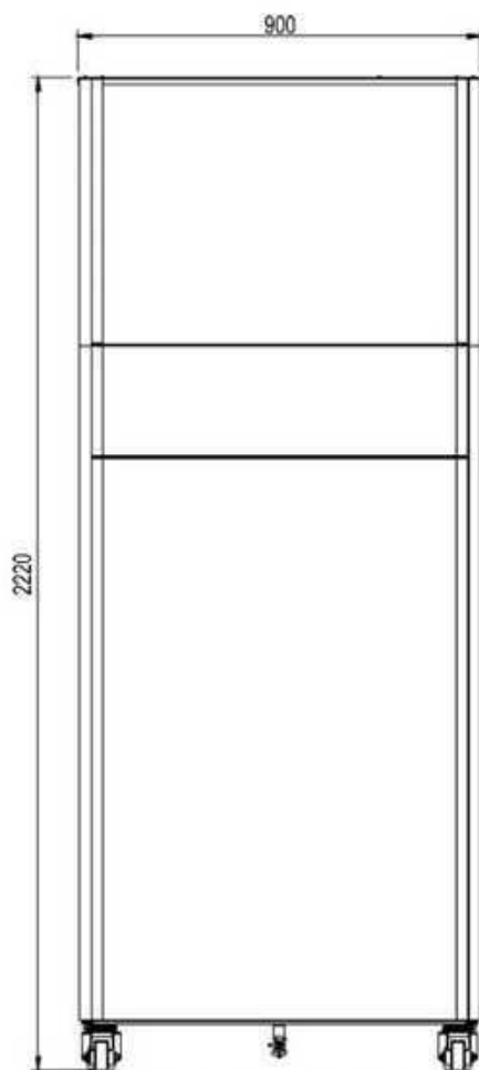
fig. 86- Vue de face modèle 450
