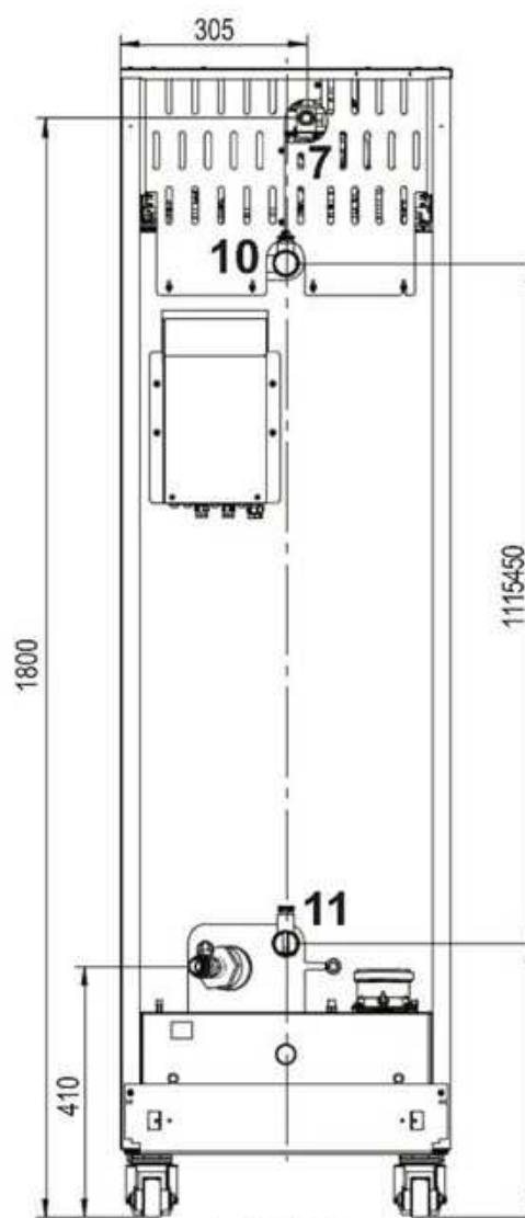
fig. 74- Rear
