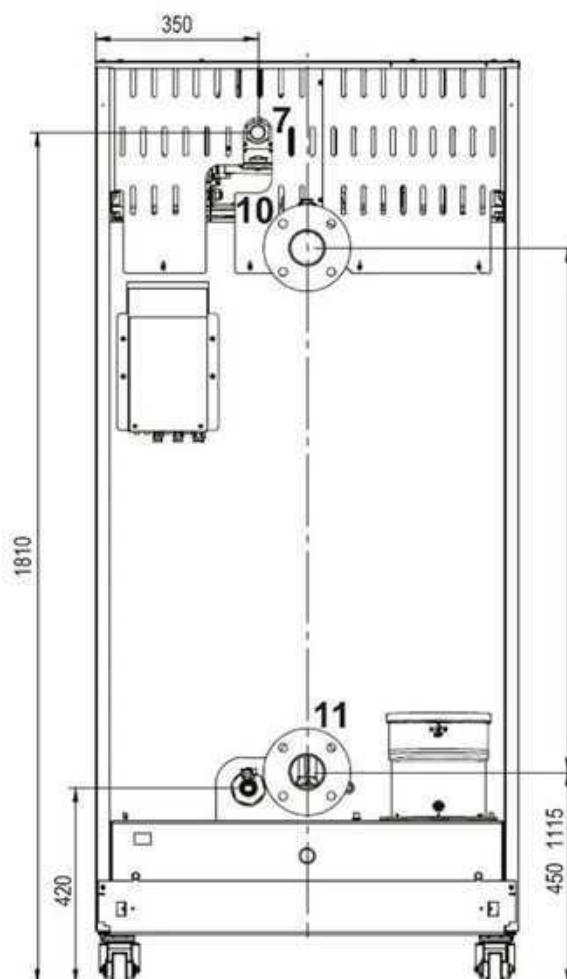
fig. 84- Vue arrière modèle 320
