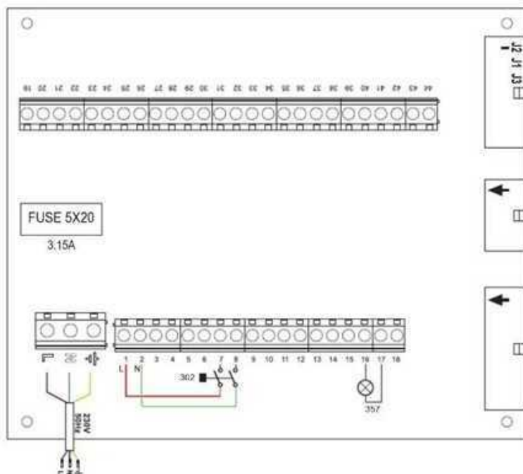
fig. 52- SLAVE
