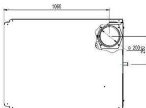
fig. 88 - Vista superiore modello 450
