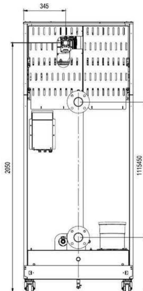
fig. 87- Vista posterior modelo 450
