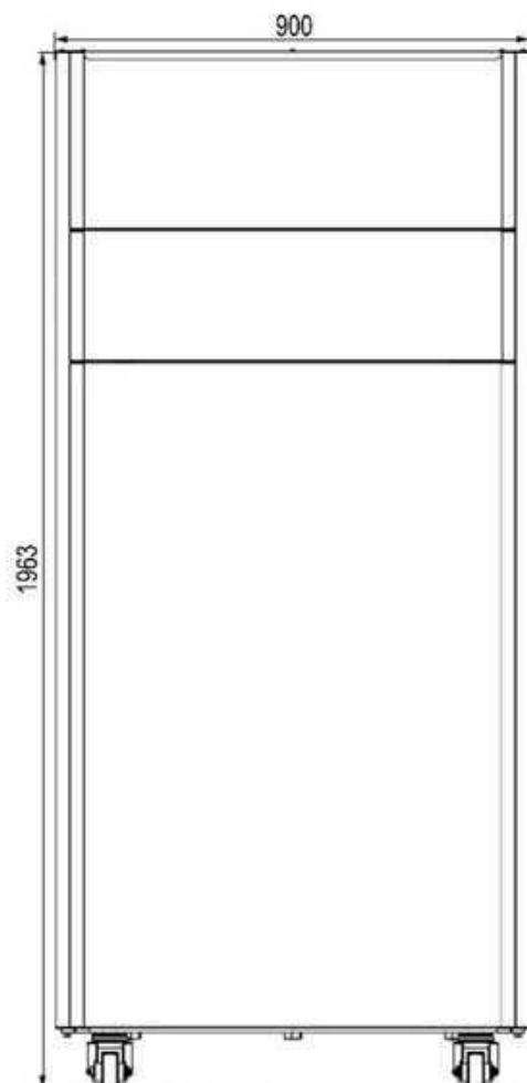
fig. 83- Vue de face modèle 320
