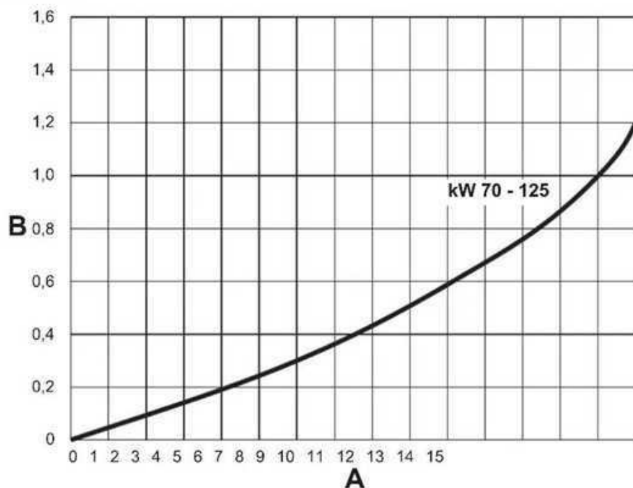
fig. 90 - Diagrama de pérdidas de carga modelos 70 - 125
