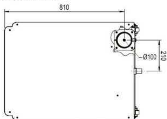
fig. 78- superior
