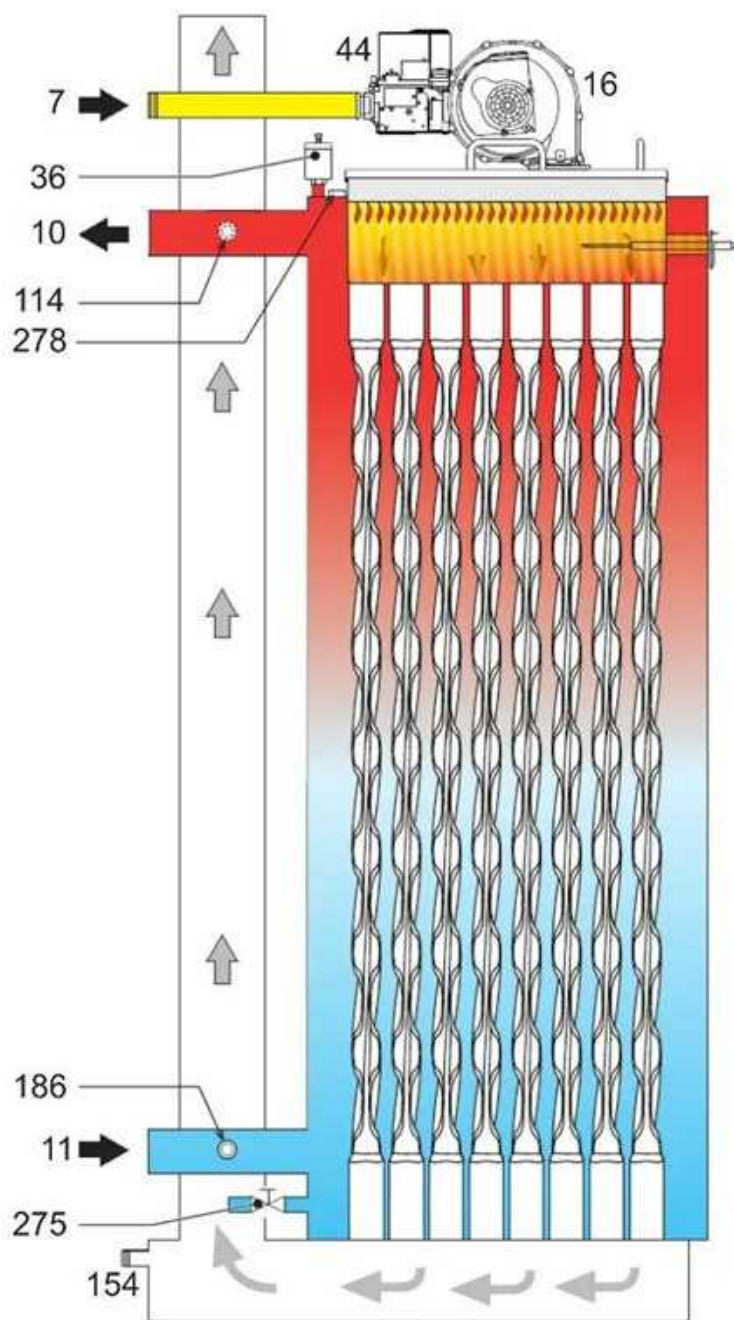
fig. 89- Circuito hidráulico
