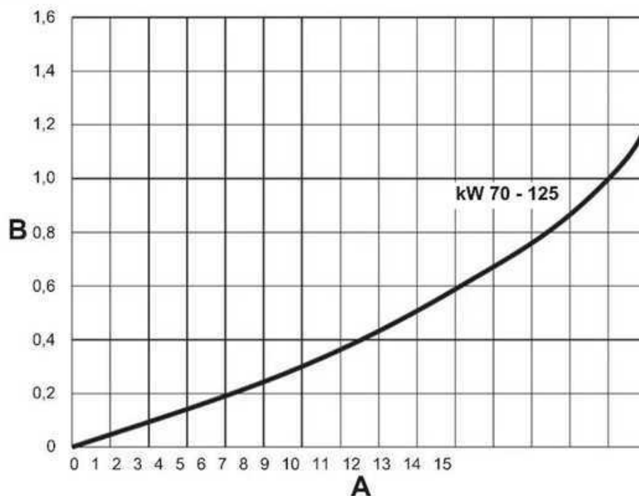
fig. 90 - Diagramme perte de charge modèles 70 - 125
