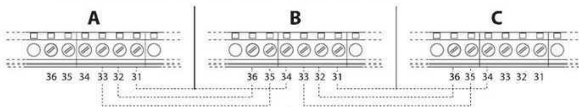
fig. 56- Raccordement en cascade
