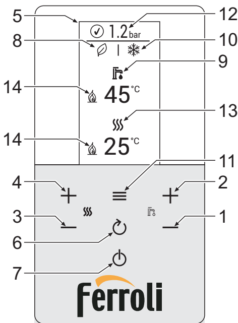
εικ. 1- Πίνακας χειριστηρίων
