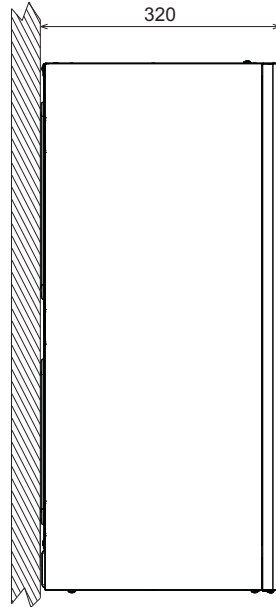
fig. 59- Vista lateral
