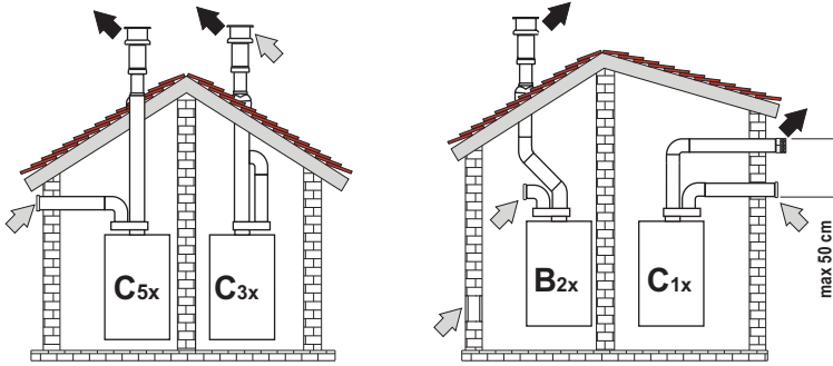
fig. 32 - Esempi di collegamento con tubi separati (⇨ = Aria / ⇩ = Fumi)
