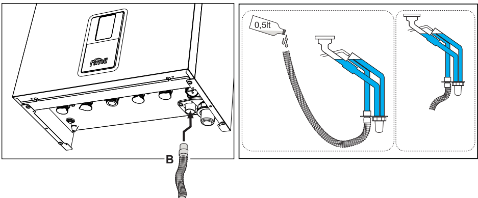
fig. 37- Conexión de la descarga de condensado
