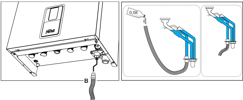
wygląd 37- Podłączenie spustu kondensatu
