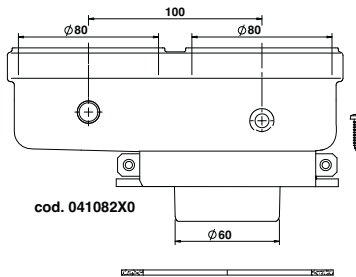
fig. 33- Accesorio inicial para conductos separados
