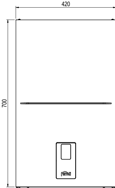
fig. 58- Vista frontal
