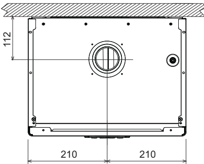
fig. 60 - Vista dall'alto
