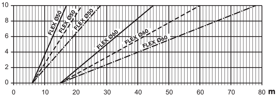
wygląd 35- Wykres wyboru parametrów przewodu spalinowego
