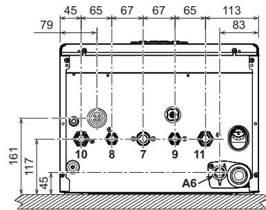
fig. 61- Vista inferior
