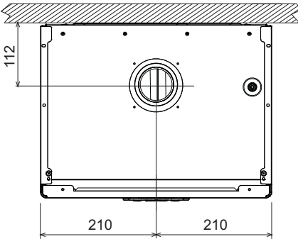
fig. 60- Vista superior
