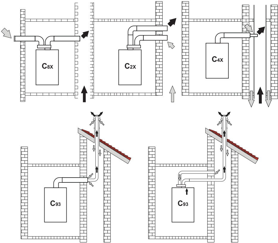
εικ. 36 Παραδείγματα σύνδεσης σε καπνοδόχους (⇐ = Αέρας / ⇨ = Καυσαέρια)
