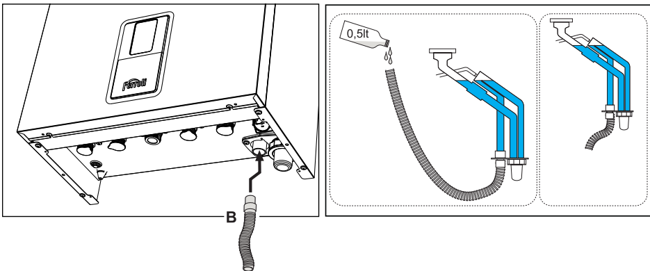
fig. 37- Racordarea evacuării condensului
