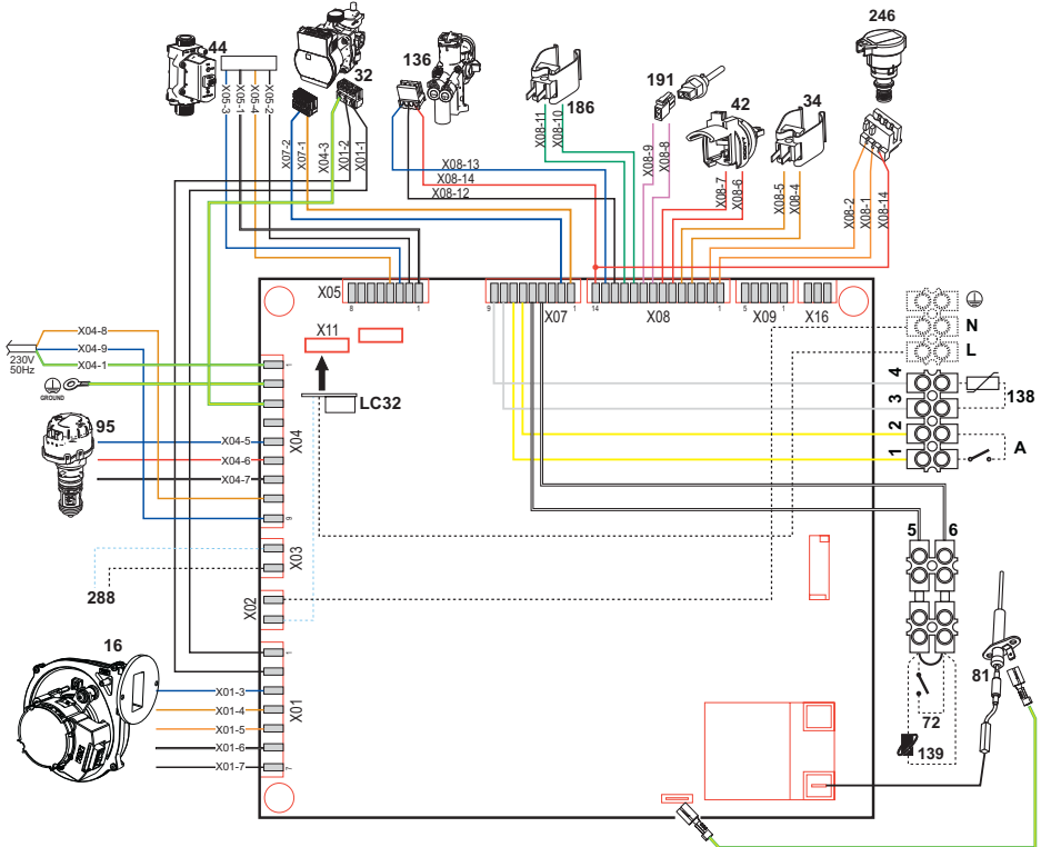
fig. 67- Wiring diagram
