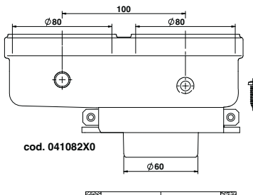
wygląd 33- Człon początkowy do montażu oddzielnych przewodów
