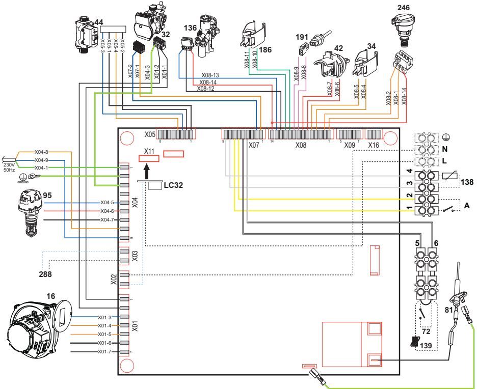
fig. 67- Schema electrică
