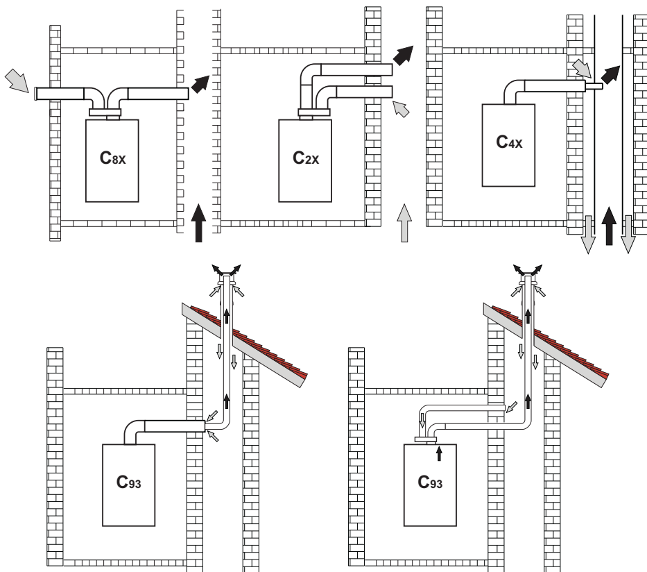
wygląd 36- Przykłady podłączenia do przewodów zbiorczych (⇐ = Powietrze / ➡ = Spaliny)
