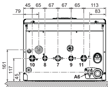
εικ. 61- Άνοψη
