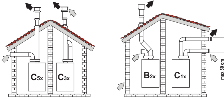
fig. 32- Ejemplos de conexión con tubos separados (— = aire / — = humos)
