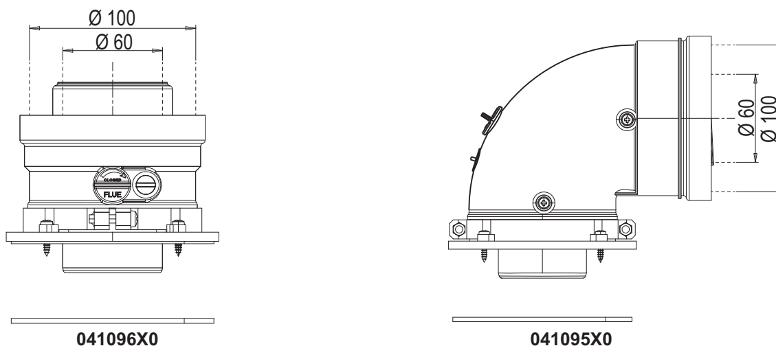
fig. 15- Accesorii de pornire pentru conducte coaxiale
