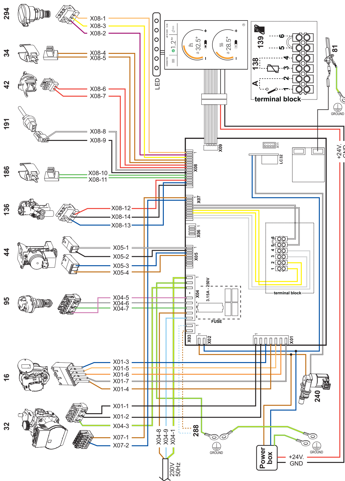
fig. 46- Esquema eléctrico
