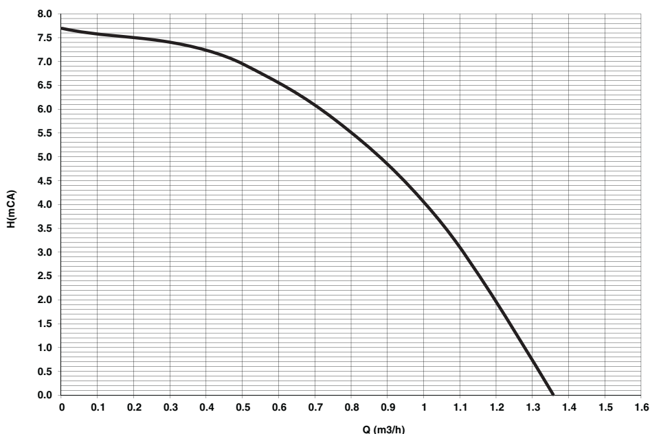
wygląd 45- Wysokość podnoszenia dostępna dla układu
