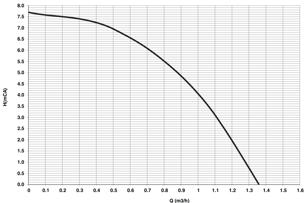
fig. 45 - Prevalenza residua disponibile all'impianto
