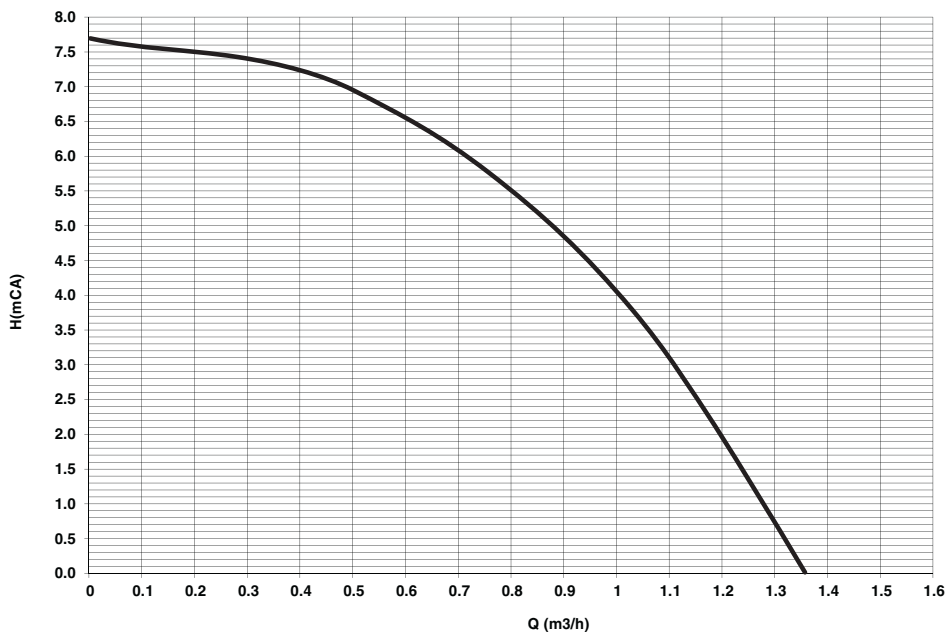
fig. 45- Înălțime de pompare reziduală disponibilă în instalație
