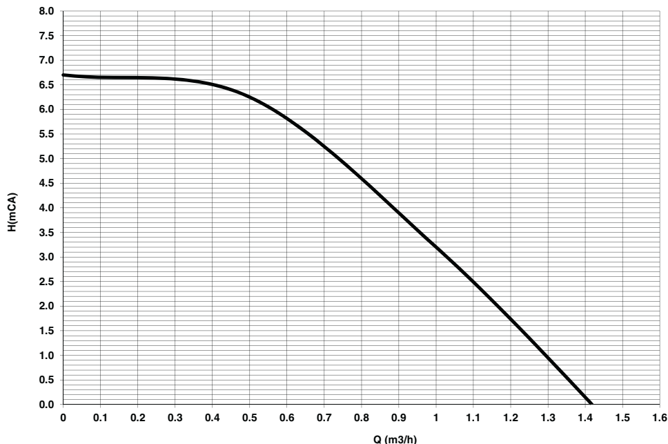
fig. 44 - Prevalenza residua disponibile all'impianto
