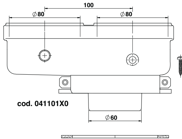
fig. 17- Accesorio inicial para conductos separados
