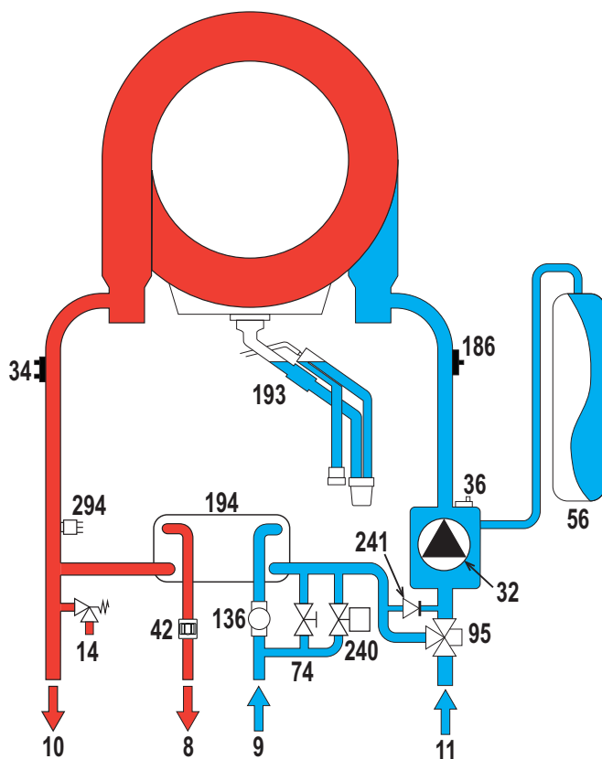
fig. 43- Circuitul hidraulic
