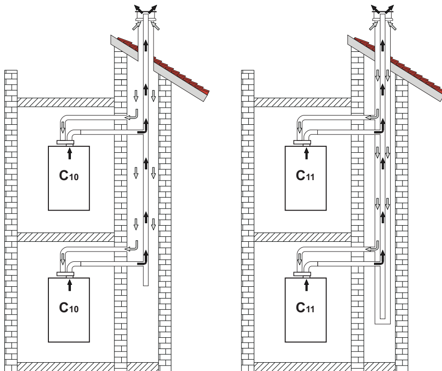
wygląd 21- Przykłady połączeń systemu C10 i C11 (⇨ = Powietrze / ⇨ = Spaliny)
