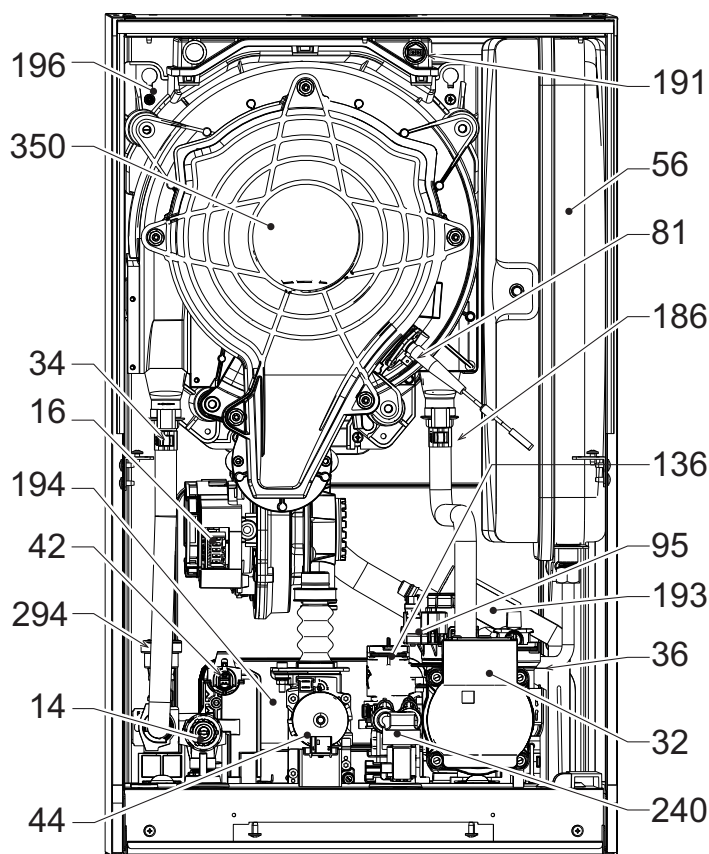
wygląd 42- Widok ogólny
