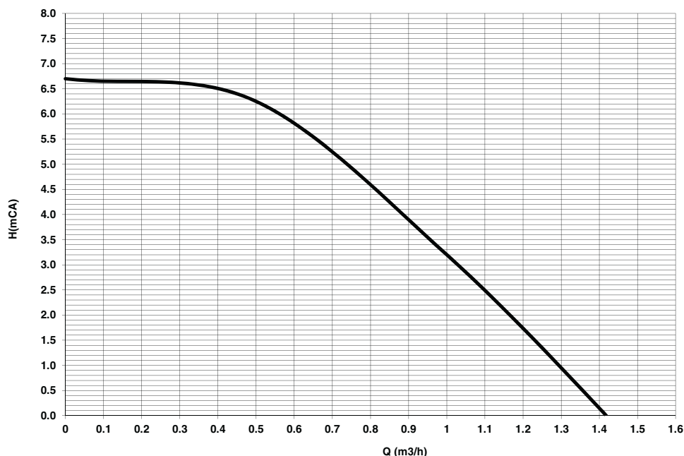
fig. 44- Carga hidrostática residual disponible en la instalación
