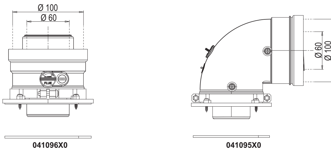
fig. 15 - Accessori di partenza per condotti coassiali
