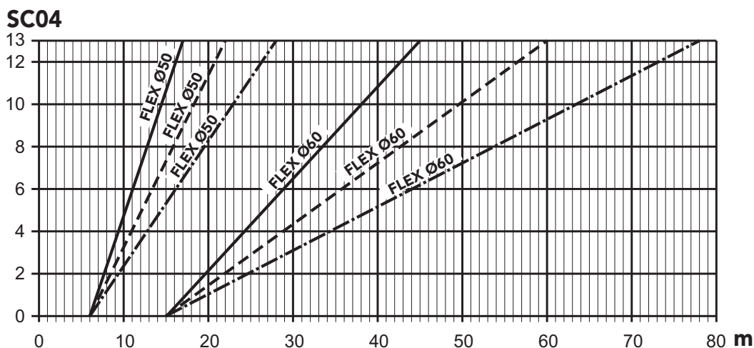
fig. 19- Grafic pentru alegerea parametrului pentru horn
