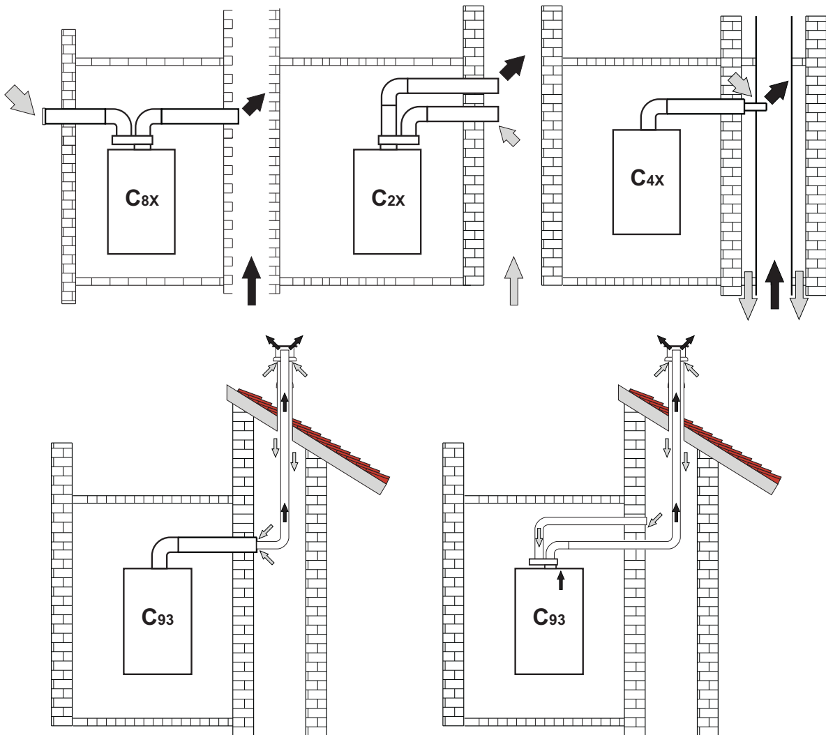
fig. 20- Ejemplos de conexión a chimeneas (⇨ = aire / ⇨ = humos)
