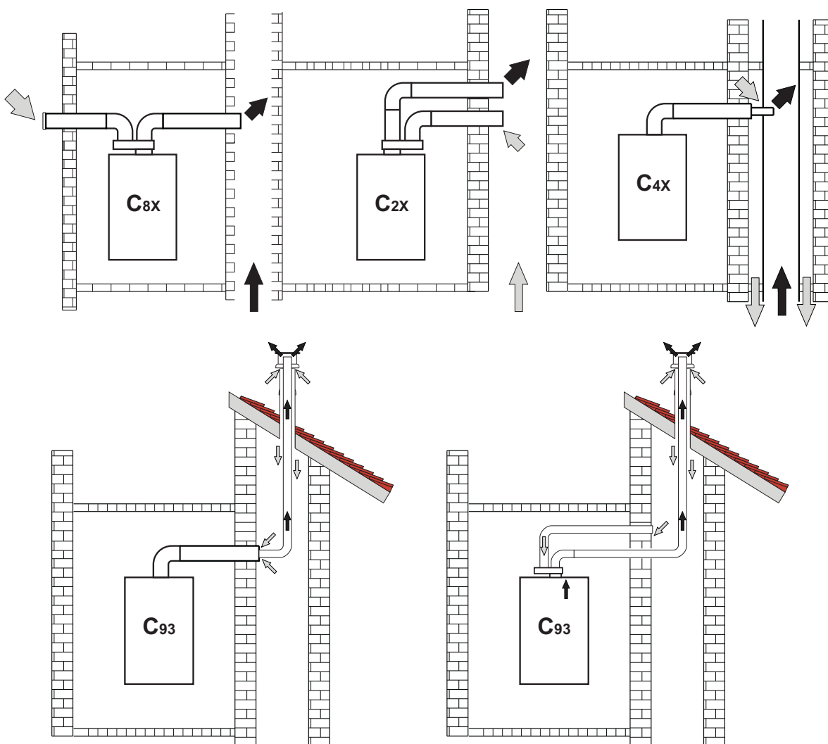
fig. 20 - Esempi di collegamento a canne fumarie (⇨ = Aria / ⇨ = Fumi)
