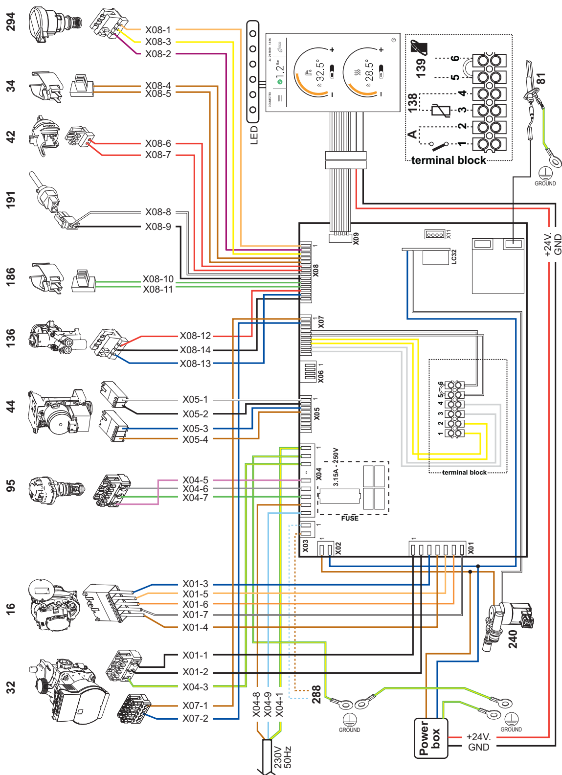
wygląd 46- Schemat instalacji elektrycznej
