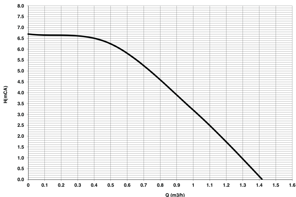
wygląd 44- Wysokość podnoszenia dostępna dla układu
