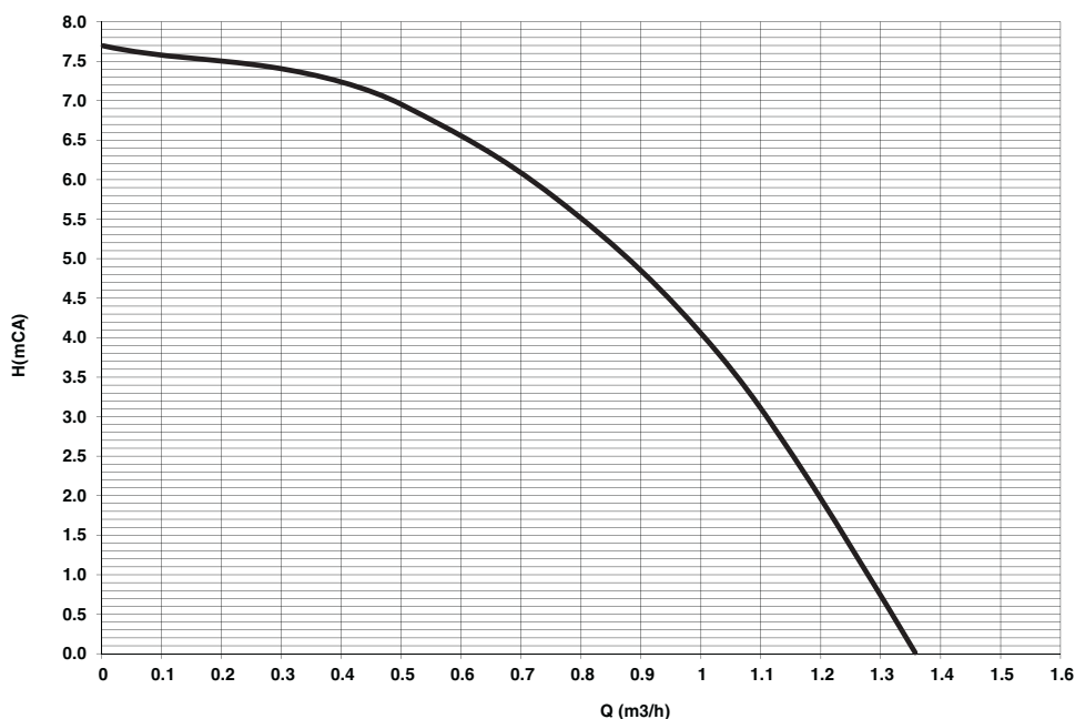
fig. 45- Carga hidrostática residual disponible en la instalación
