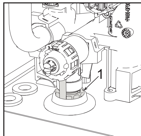
fig. 10- Supapă de siguranță cu robinete de golire
