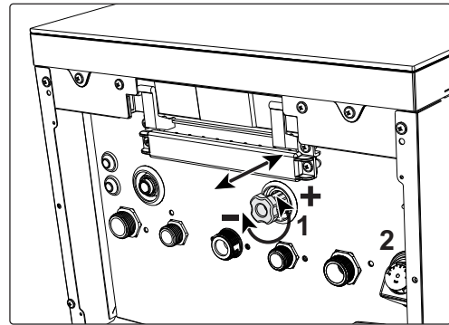
fig. 9- Buton de umplere
