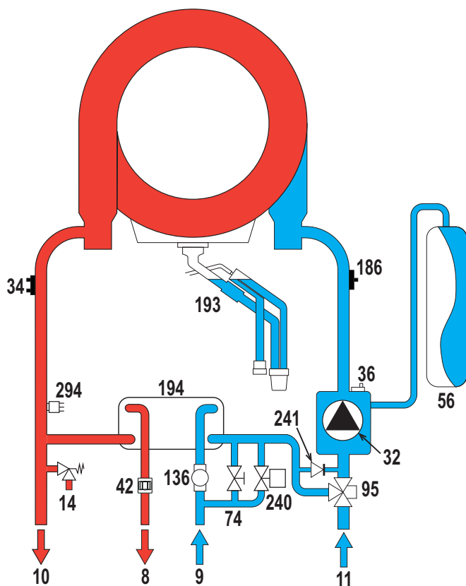
fig. 43- Circuito de agua
