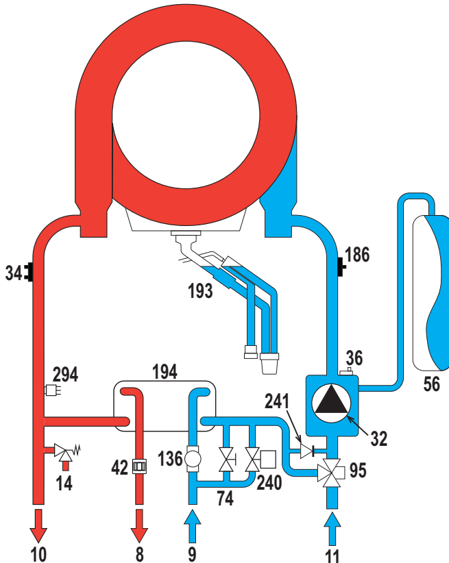
fig. 43 - Circuito idraulico
