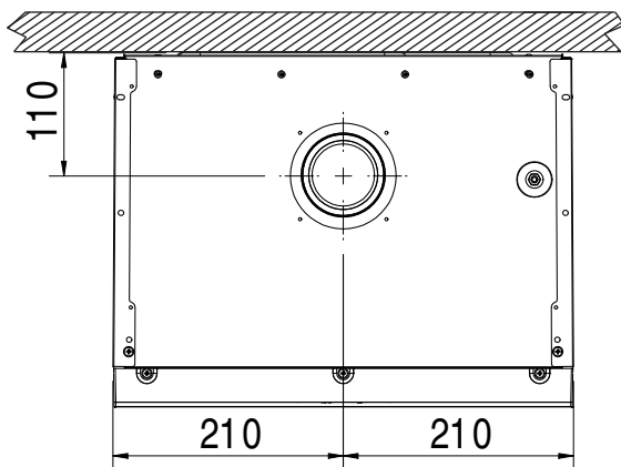
fig. 37 - Vista dall'alto
