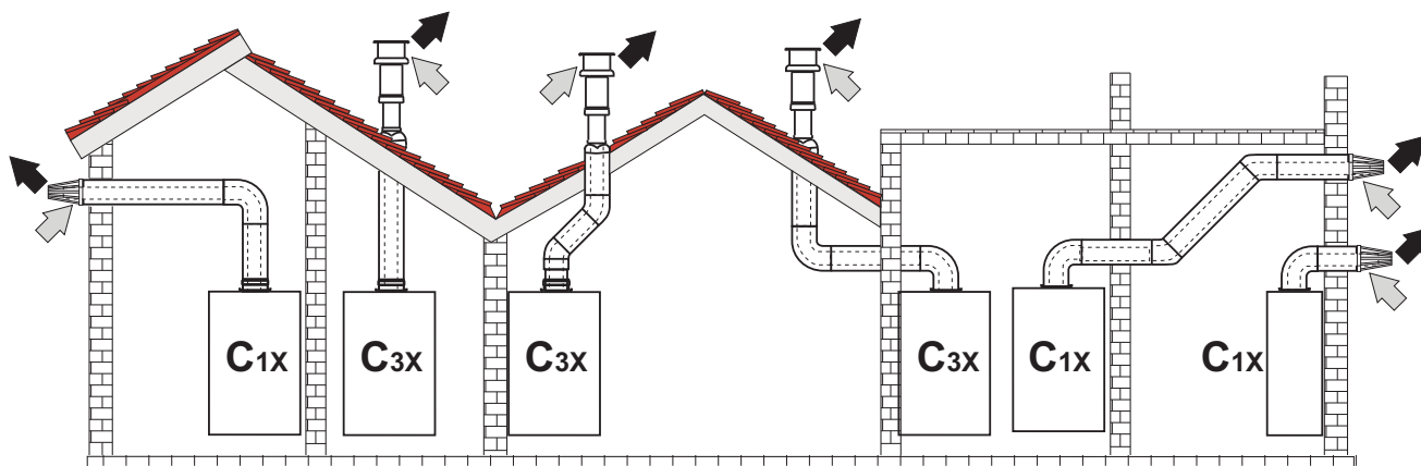
wygląd 14- Przykłady połączenia przewodami współosiowymi (⇨ = Powietrze / ⇨ = Spaliny)
