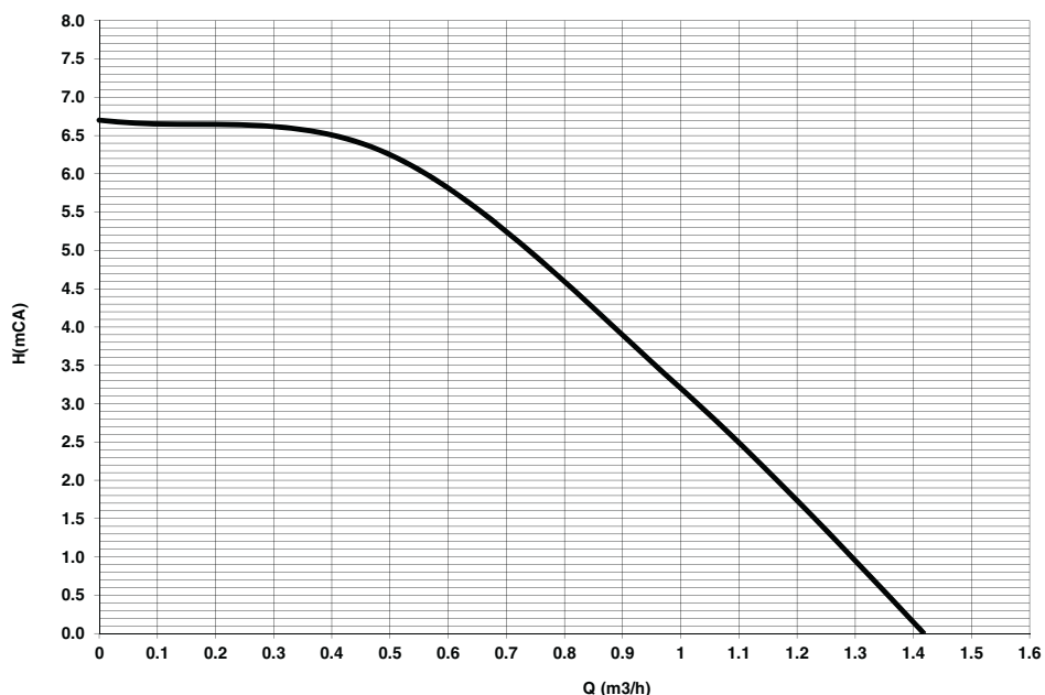
fig. 44- Înălțime de pompare reziduală disponibilă în instalație
