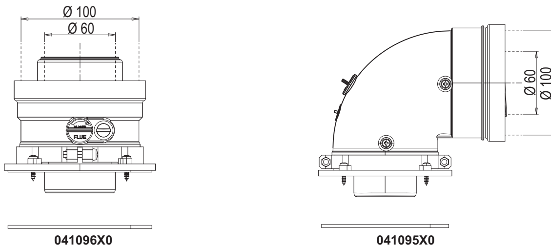
fig. 15- Accesorios iniciales para conductos coaxiales
