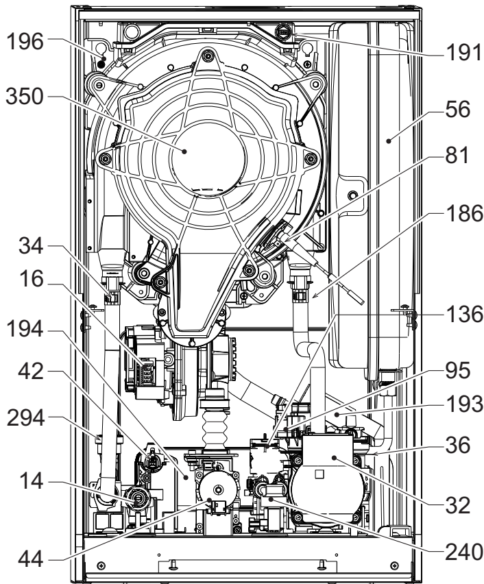
fig. 42 - Vista generale
