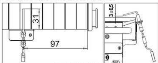
fig. 23- Posición del electrodo
