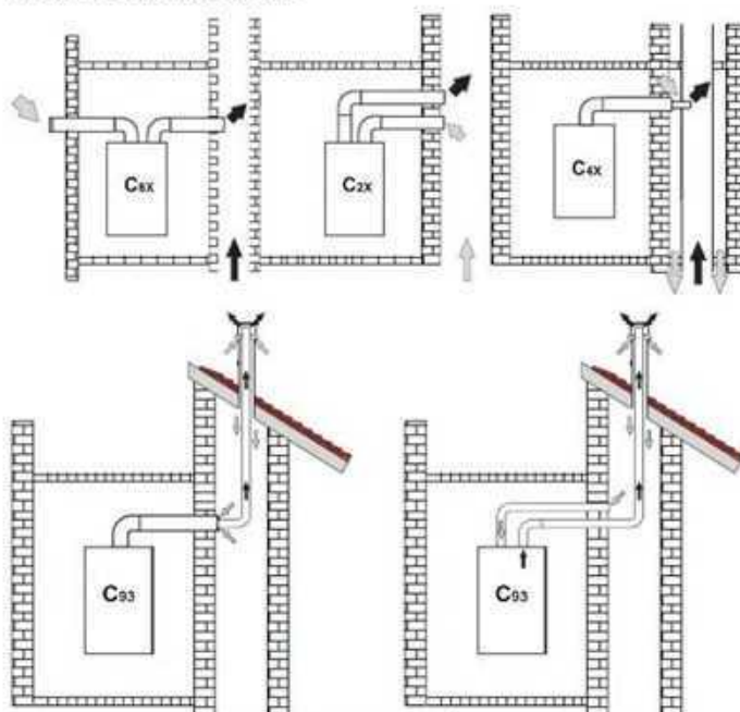
fig. 19 - Exemple de racordare la hornuri (A = Aer / = Gaze arse)
