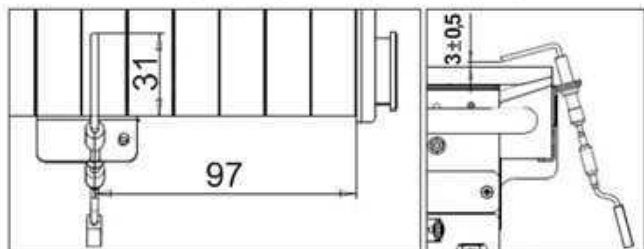
fig. 23- Poziționare electrod
