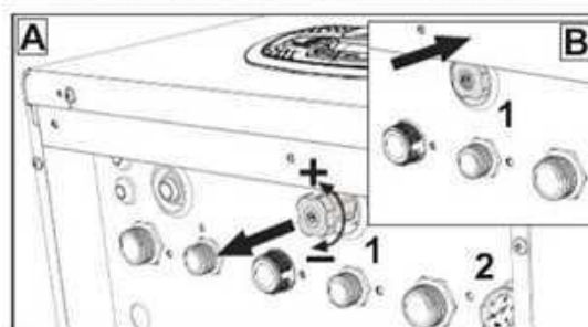
εικ. 8- Διακόπτης πλήρωσης
