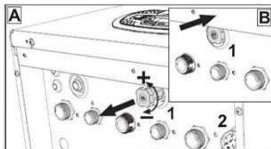
wygląd 8 - Pokrętło napełniania
