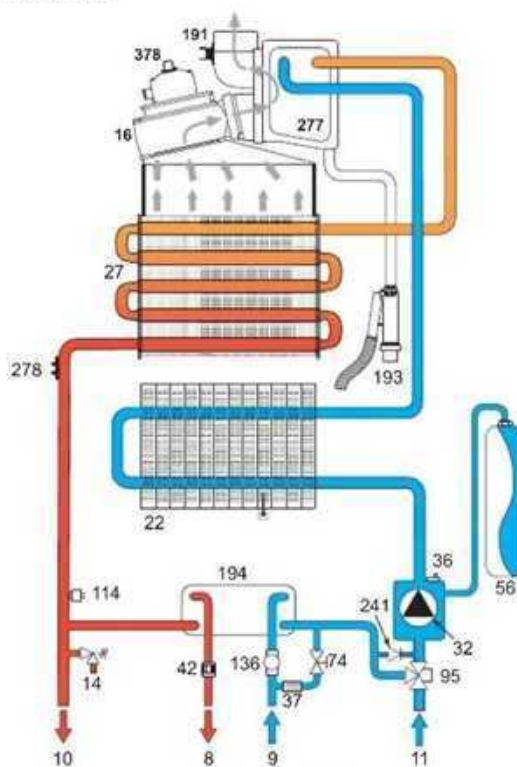
fig. 30- Circuitul de încălzire
