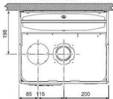
fig. 26 - Vista dall'alto
