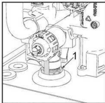
wygląd 9 - Zawór bezpieczeństwa z kurkiem spustowym
