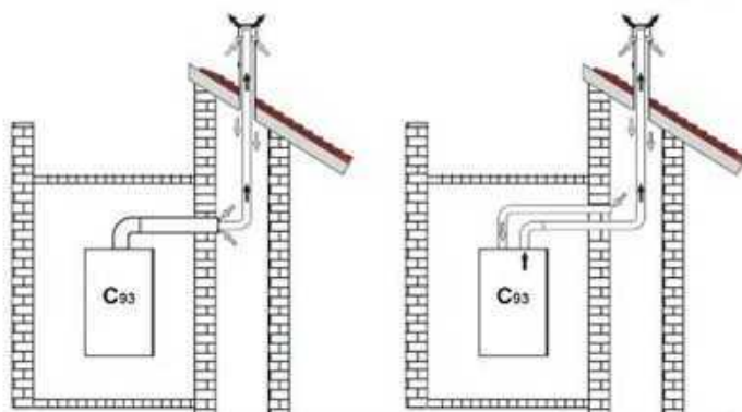
wygląd 19 - Przykłady podłączenia do kanałów dymowych (→ = Powietrze / → = Spaliny)
