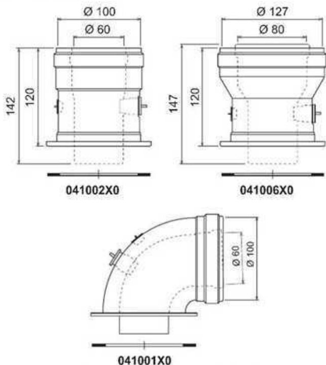
fig. 14 - Accesorii de pornire pentru conducte coaxiale
