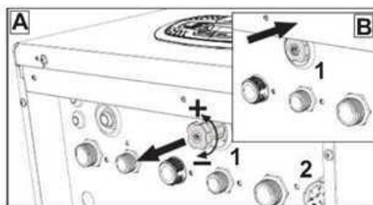
fig. 8 - Manopola di carico
