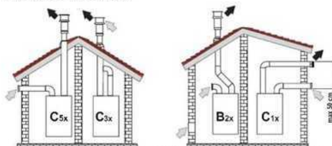
wygląd 15 - Przykłady połączenia oddzielnymi rurami ( = Powietrze / = Spaliny)
