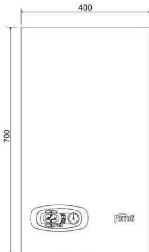
fig. 24 - Vista frontale
