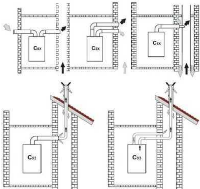
εικ. 19 Παραδείγματα σύνδεσης σε καπνοδόχους (↗ = Αέρας / ↘ = Κausaeria)
