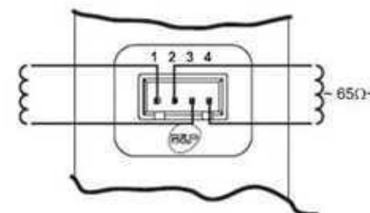
fig. 21 - Conexiune valvă gaz
