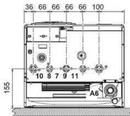
fig. 27- Vedere de jos
