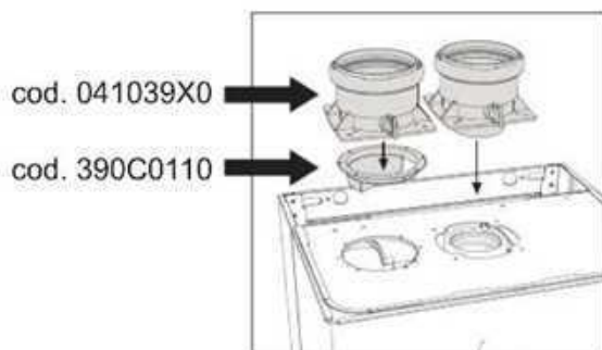
fig. 18 - Accesoriu de pornire pentru conducte separate
