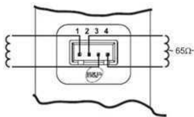
εικ. 21 - Σύνδεση βαλβίδας αερίου
