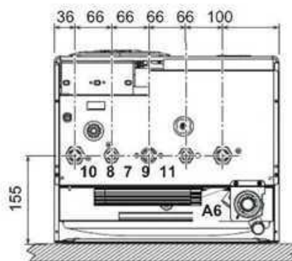
fig. 27- Vista inferior
