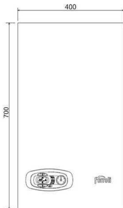
fig. 24- Vista frontal
