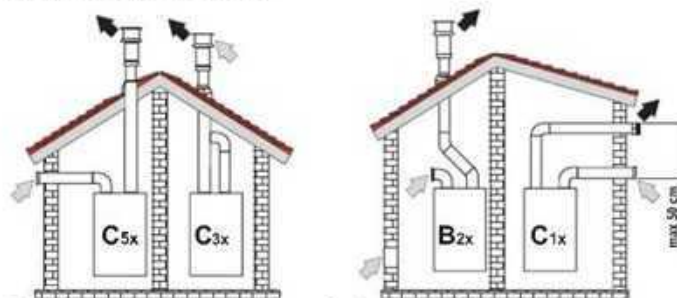
fig. 15 - Exemple de racordare cu conducte separate ( = Aer / = Gaze arse)
