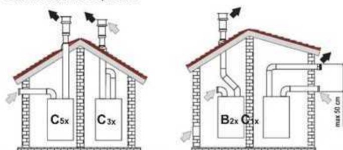
fig. 15 - Ejemplos de conexión con tubos separados (→ = aire / → = humos)
