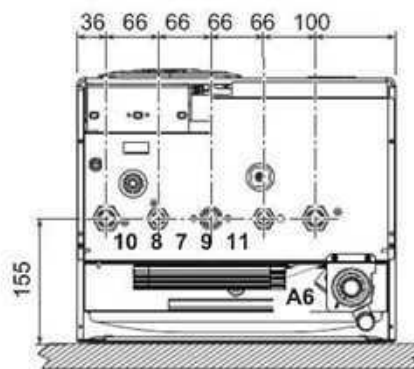
wygląd 27- Widok od dołu
