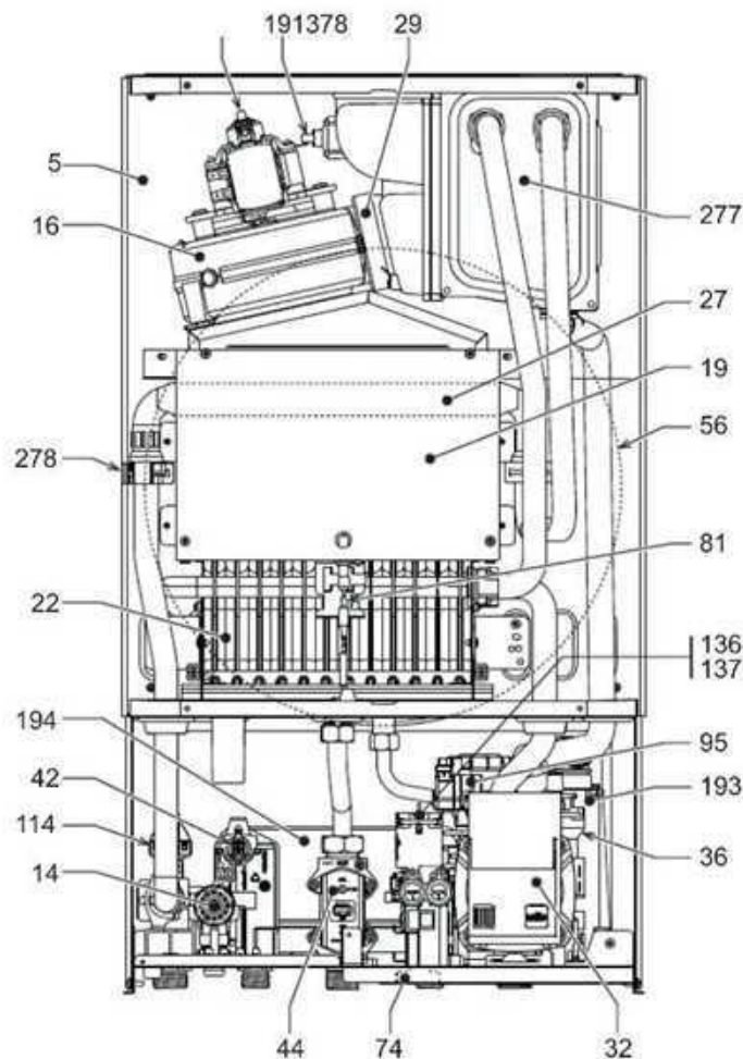
fig. 29- Vedere generală
