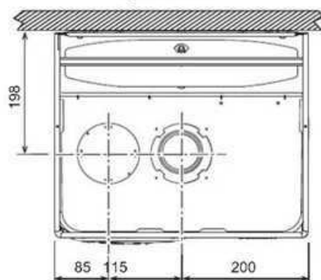
fig. 26- Vista superior
