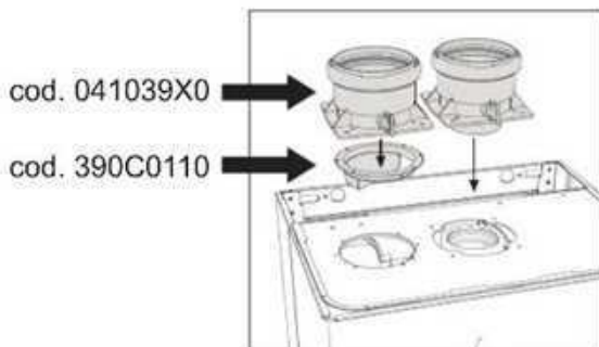
fig. 18 - Accessorio di partenza per condotti separati
