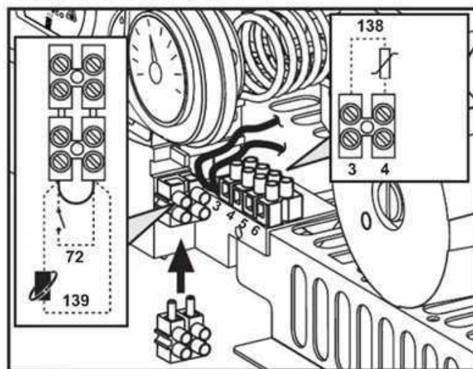
ΕΙΚ. 10- Πρόσβαση στην πλακέτα ακροδεκτών
