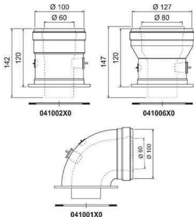
fig. 14 - Accesorios iniciales para conductos coaxiales
