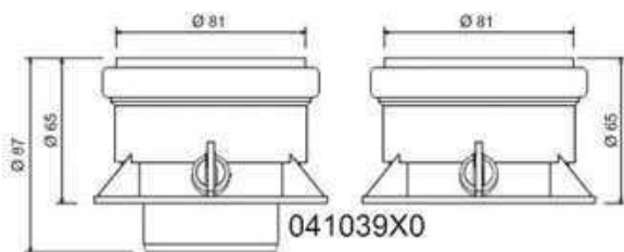
wygląd 18- Akcesoria wyjściowe do przewodów oddzielnych
