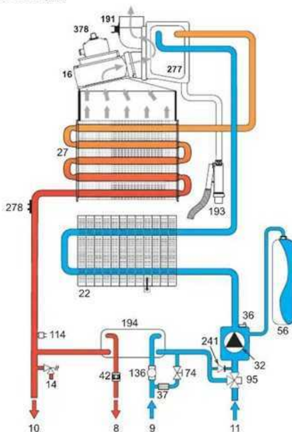
fig. 30- Circuito de calefacción
