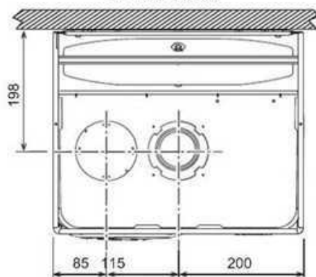
ΕΙΚ. 26 - Κάτωψη
