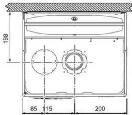
fig. 26- Vedere de sus
