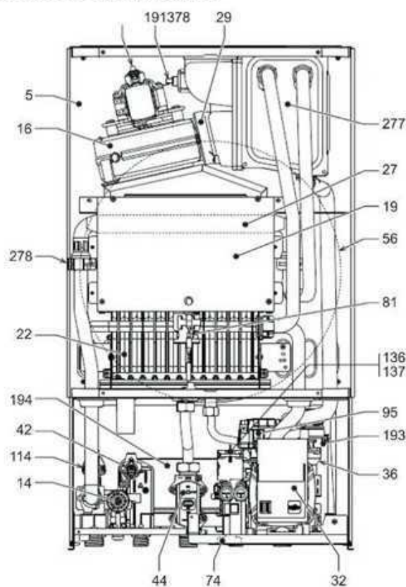
fig. 29 - Vista generale
