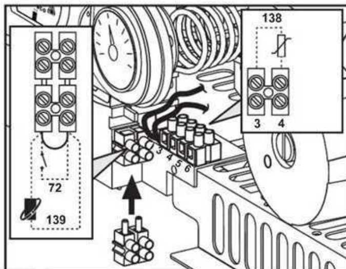
wygląd 10-Dostęp do elektrycznej listwy zaciskowej
