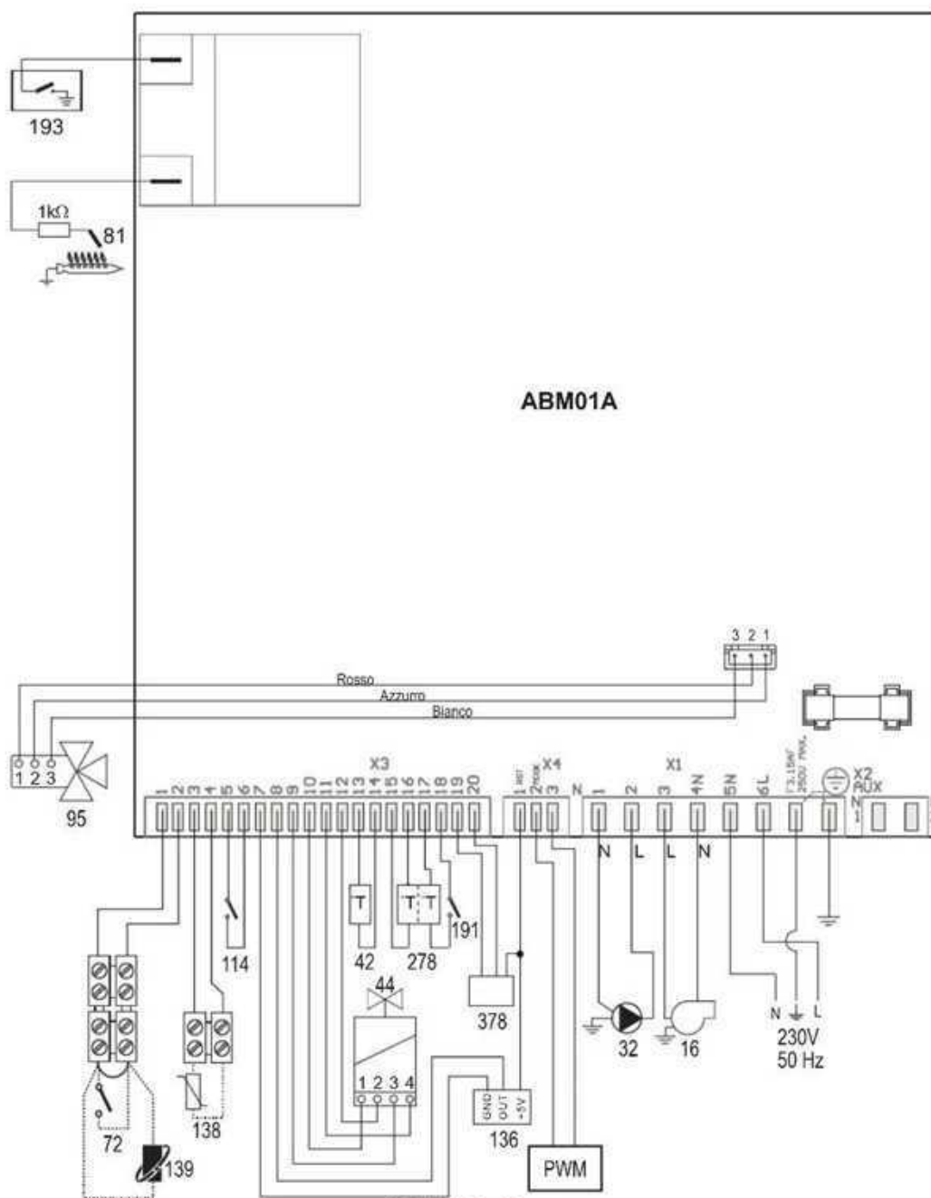
fig. 31- Wiring diagram
