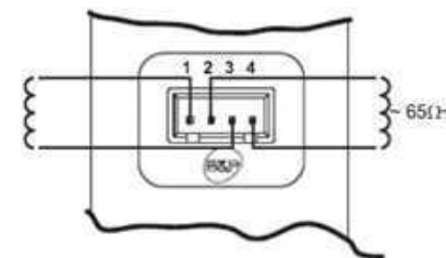
fig. 21 - Connessione valvola gas
