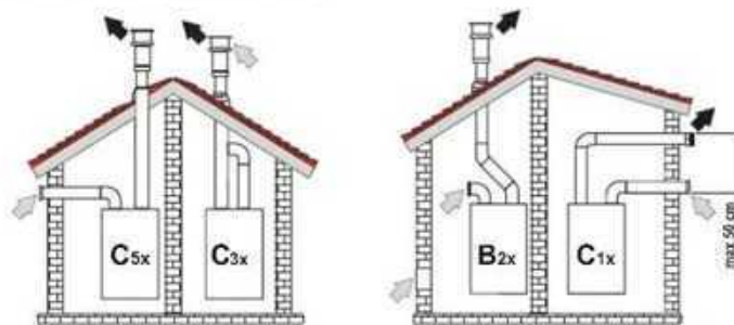
ΕΙΚ. 15 - Παραδείγματα σύνδεσης με ξεχωριστούς σωλήνες (→ = Αέρας / ← = Καυσαέρια)
