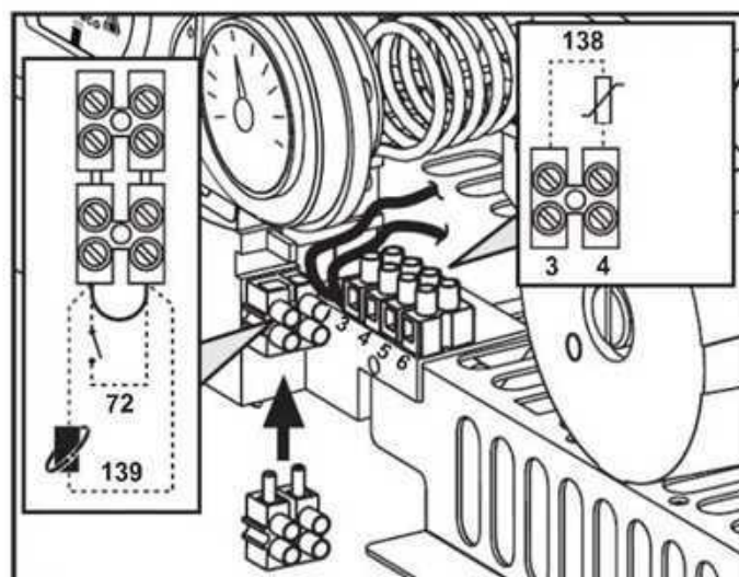
fig. 10- Accesul la panoul de borne
