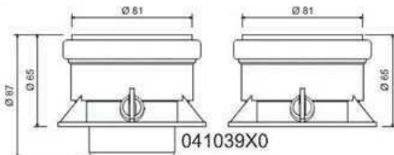
εικ. 18 - Εξάρτημα σύνδεσης για ξεχωριστούς αγωγούς
