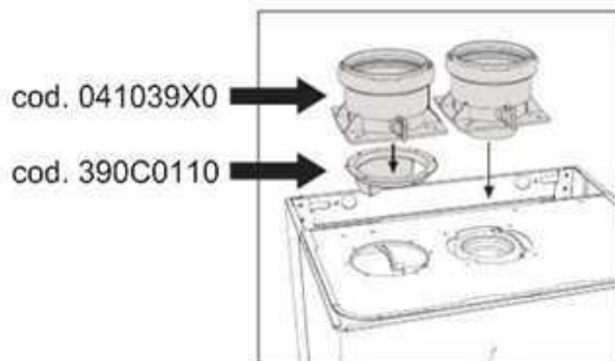
εικ. 18 - Εξάρτημα σύνδεσης για ξεχωριστούς αγωγούς
