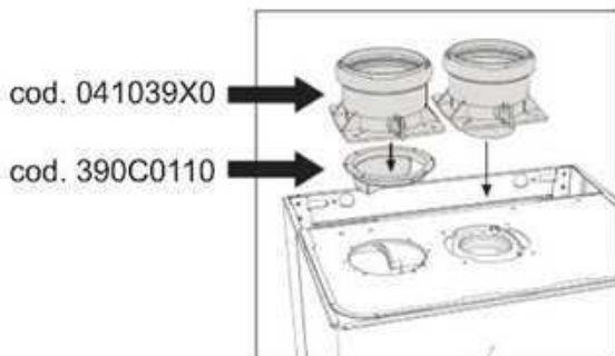
wygląd 18- Akcesoria wyjściowe do przewodów oddzielnych
