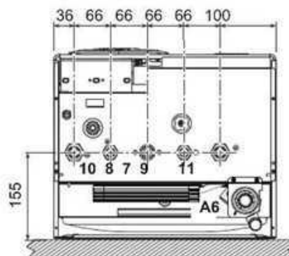
ΕΙΚ. 27- Άνοψη
