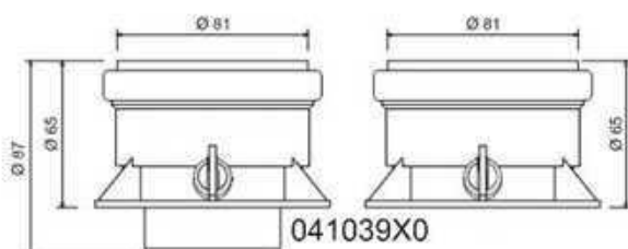
fig. 18 - Accesoriu de pornire pentru conducte separate
