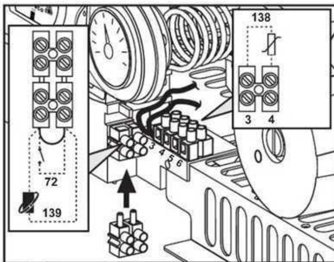
fig. 10 - Accesso alla morsettiere
