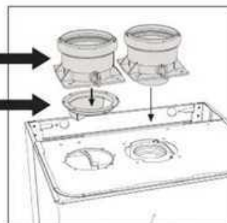
fig. 18 - Accesorio inicial para conductos separados
