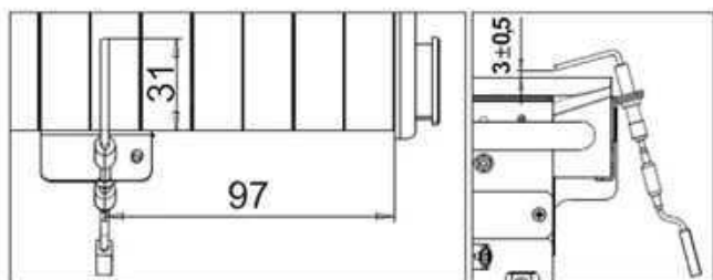
εικ. 23- Τοποθέτηση ηλεκτροδίου
