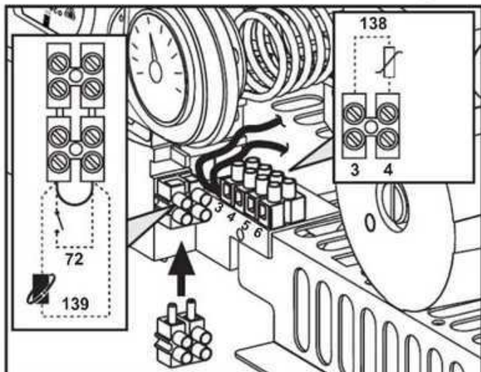
fig. 10- Acceso a la caja de conexiones
