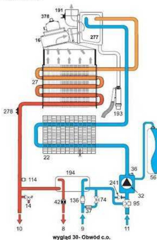
wygląd 30- Obwód c.o.
