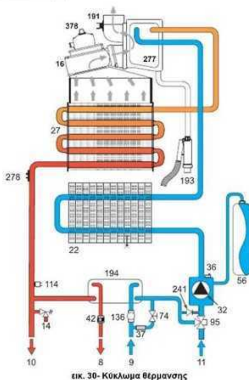
ΕΙΚ. 30- Κύκλωμα θέρμανσης
