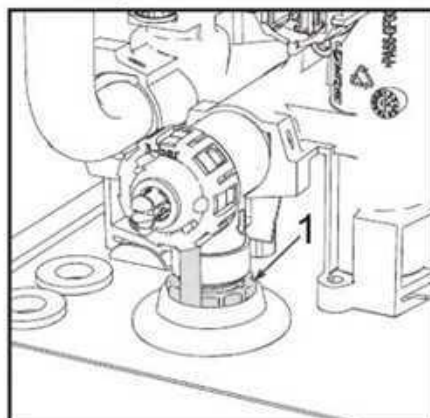
fig. 9 - Válvula de seguridad con grifo de descarga
