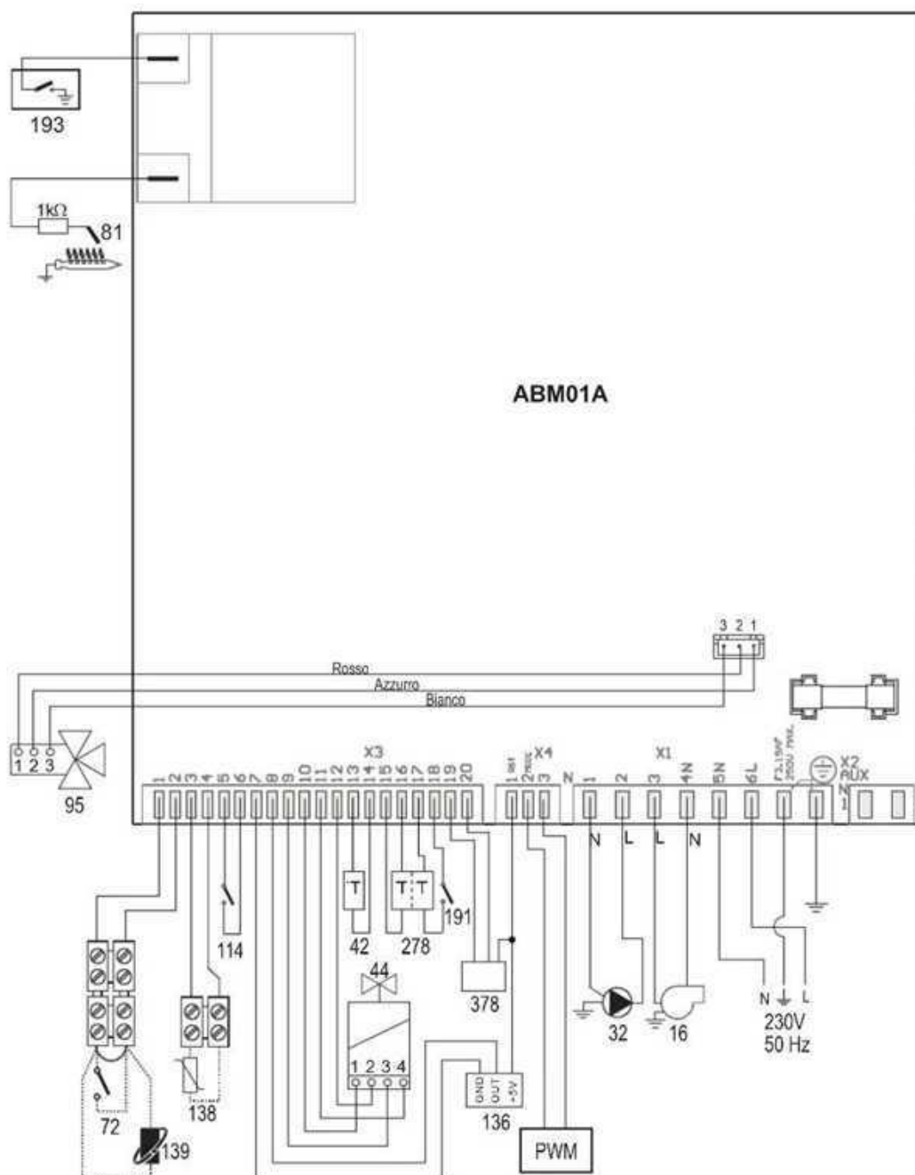
fig. 32 - Schema elettrico
