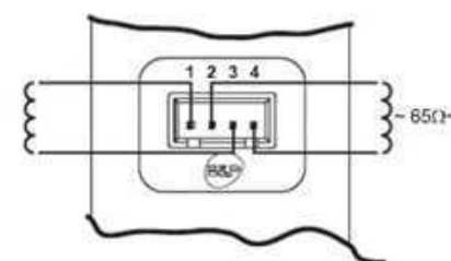
wygląd 21- Podłączenie zaworu gazowego
