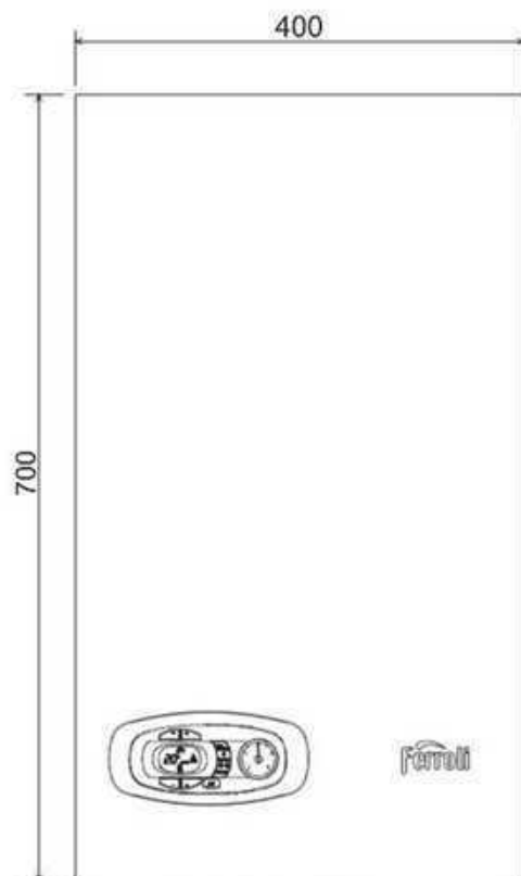
wygląd 24- Widok z przodu
