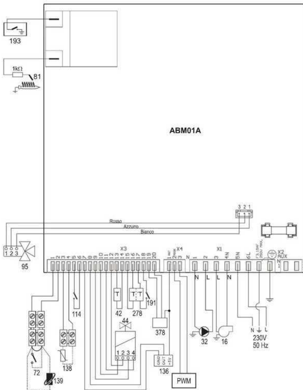
fig. 31- Esquema eléctrico
