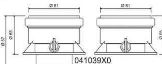
fig. 18 - Accesorio inicial para conductos separados
