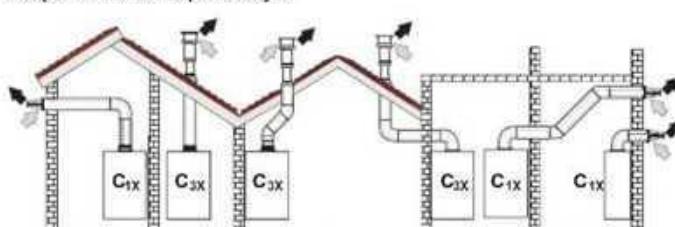
wygląd 12- Przykłady połączenia przewodami współosiowymi (→ = Powietrze / → = Spaliny)
