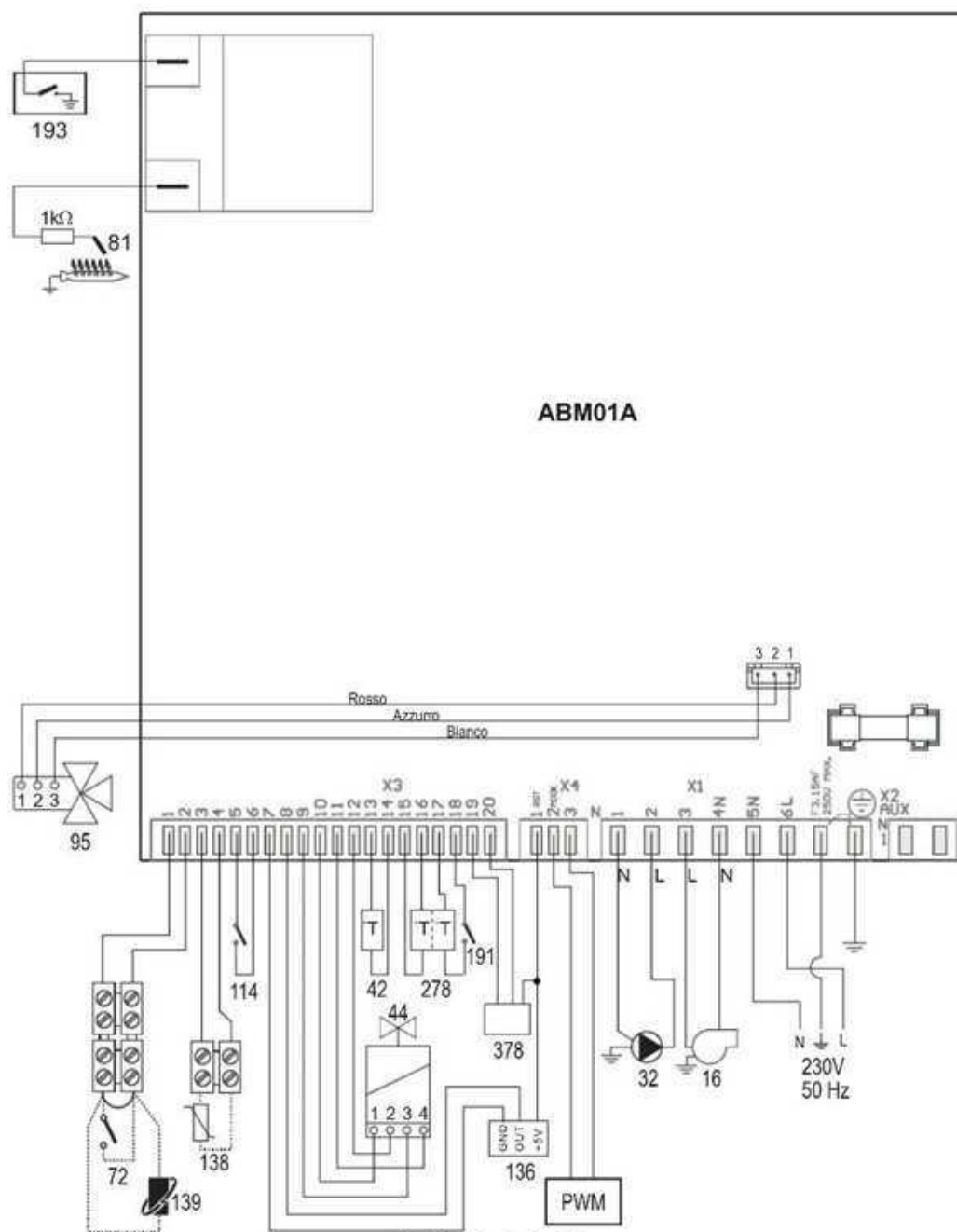
fig. 31- Schemă electrică
