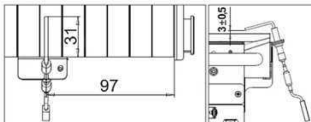
fig. 23 - Posizionamento elettrodo
