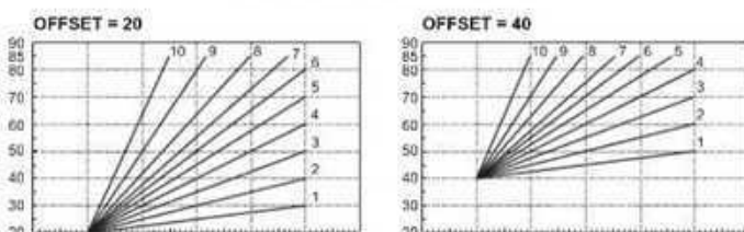
εικ. 7 - Παράδειγμα παράλληλης μετατόπισης των καμπυλών αντιστάθμισης
