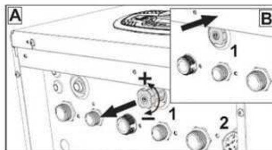
fig. 8 - Buton de umplere
