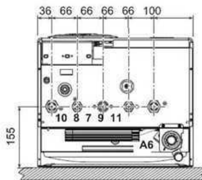
fig. 27 - Vista dal basso
