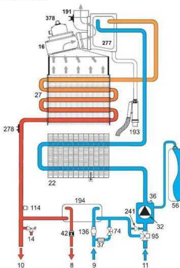
fig. 30 - Circuito riscaldamento
