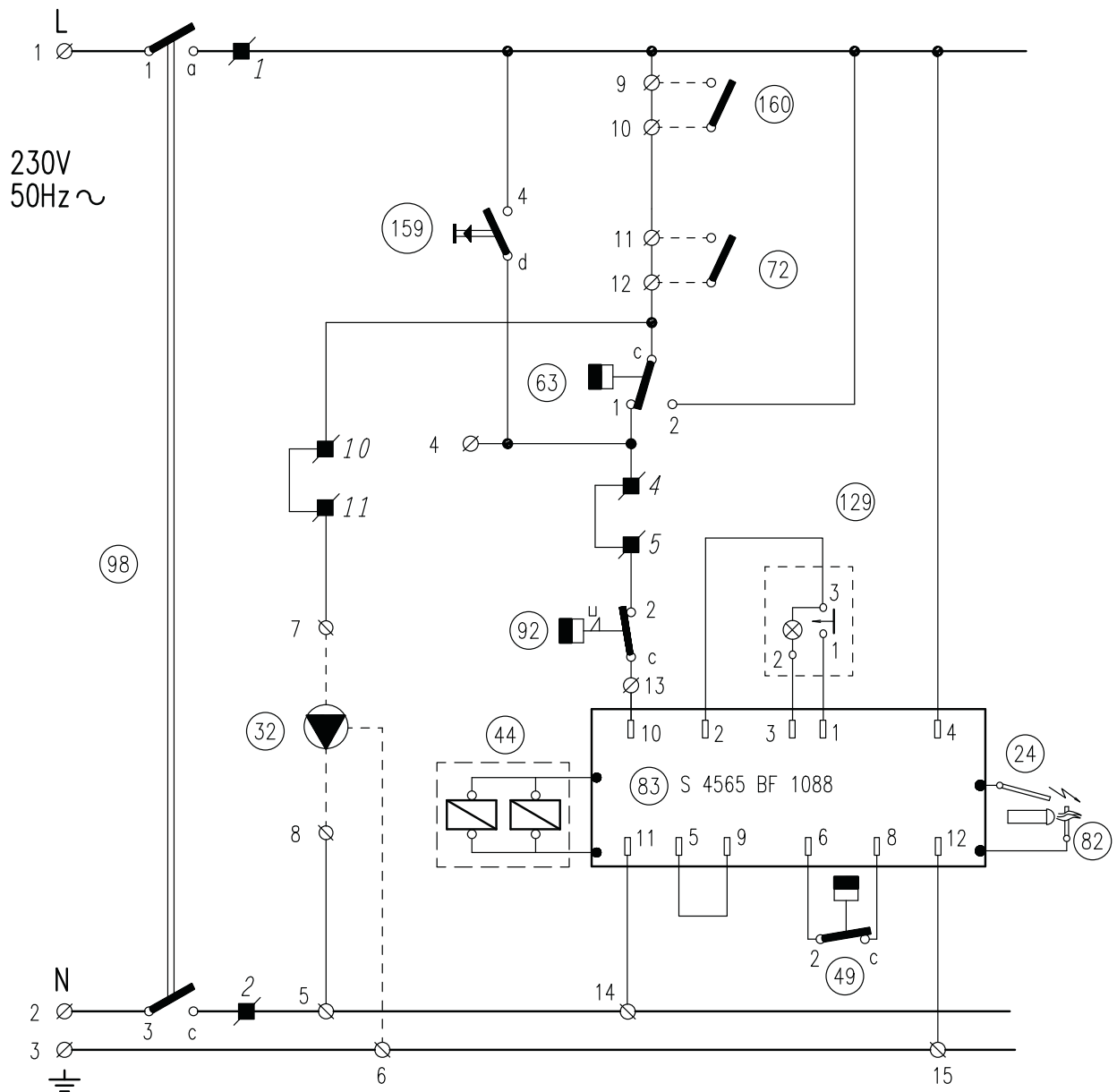
fig. 14 - Schema elettrico di principio
