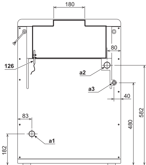
řek. 11 - Arkadan görünüm
