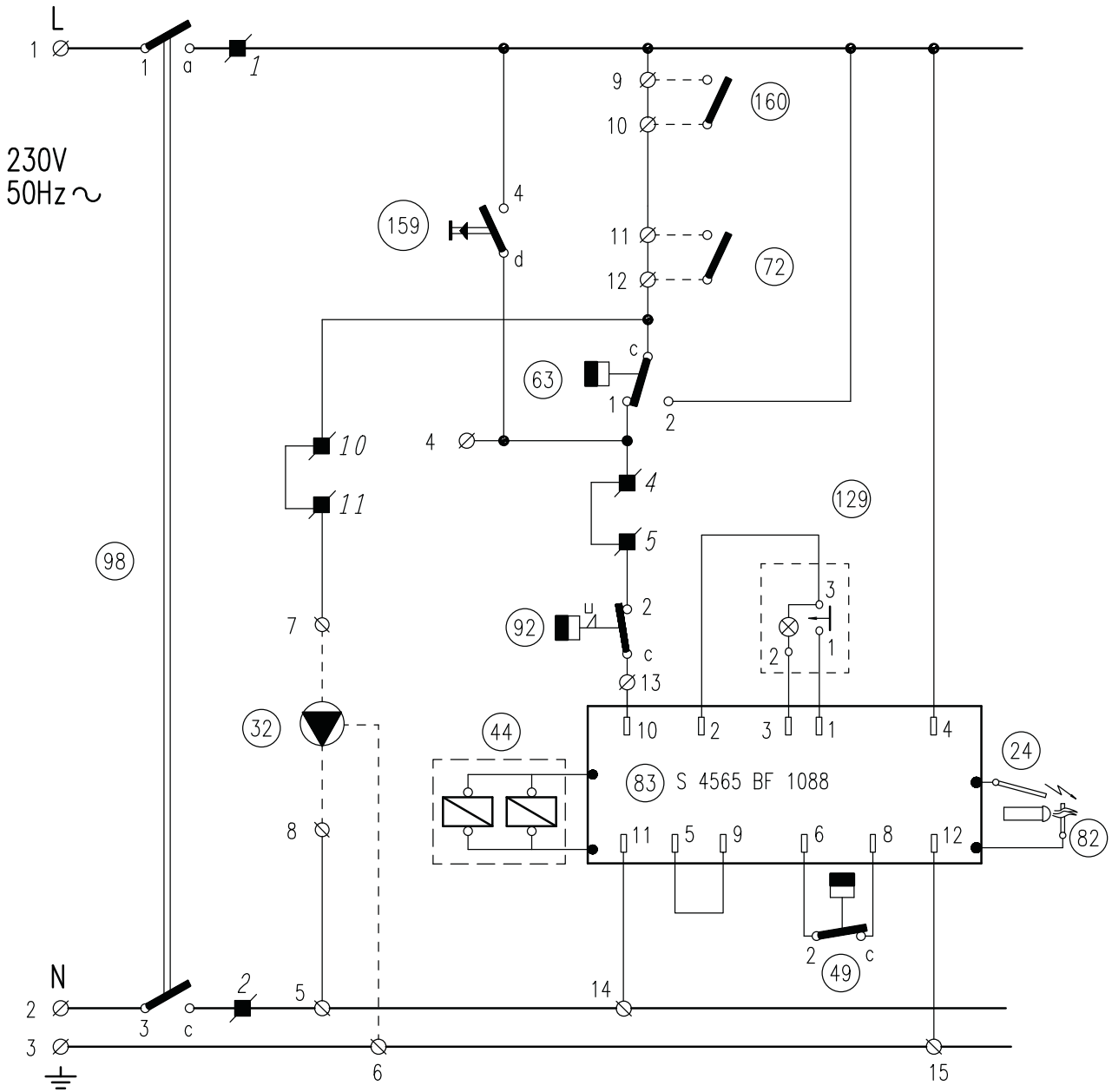
şek. 14 - Elektrik prensip şeması
