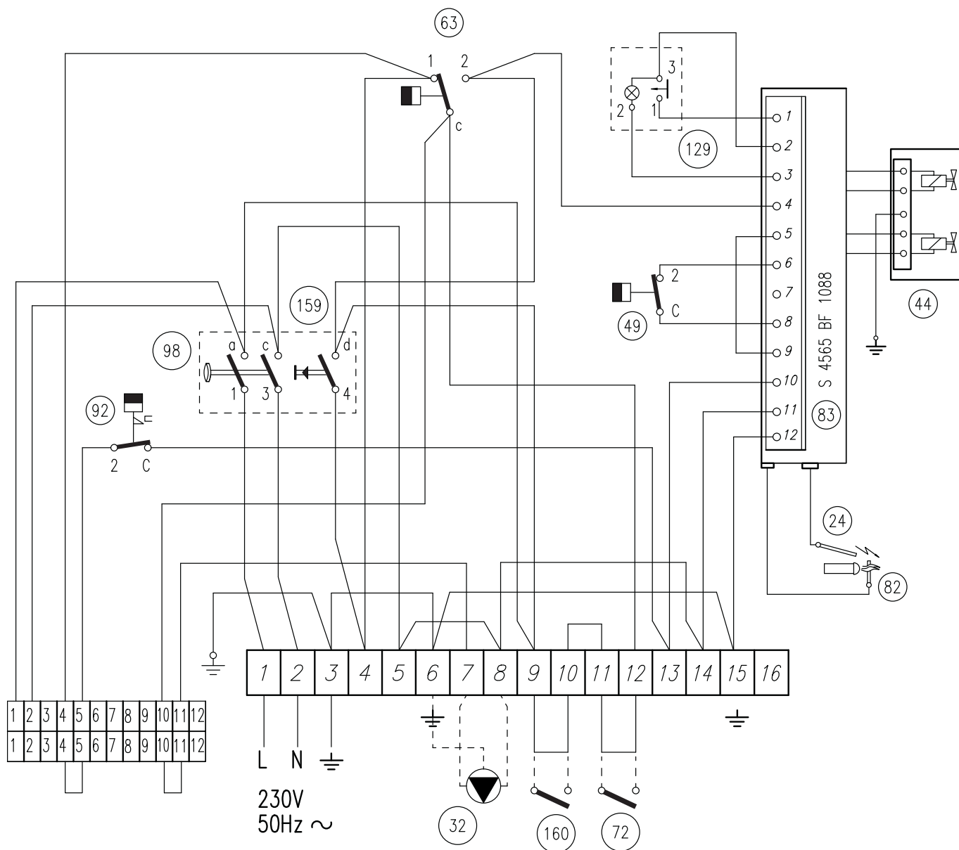
fig. 15 - Esquema eléctrico de conexión
