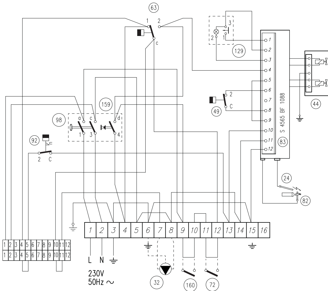
fig. 15 - Schéma électrique de raccordement
