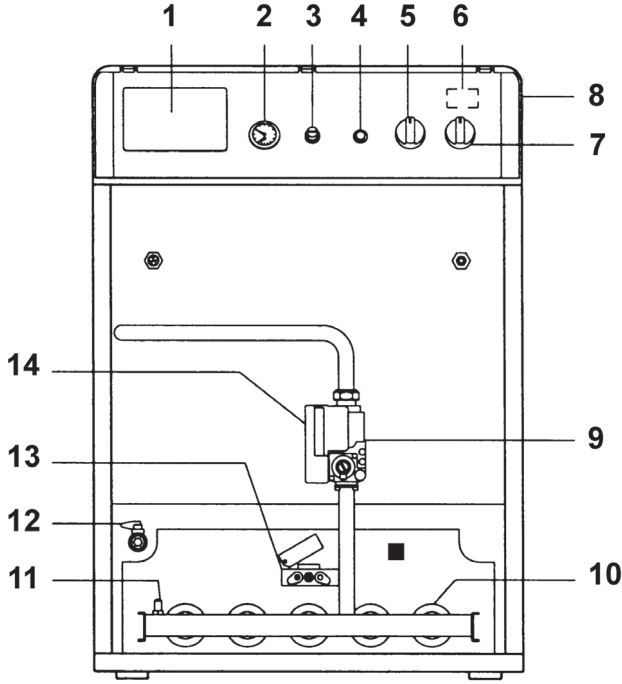
şek. 12 - Genel görünüm
