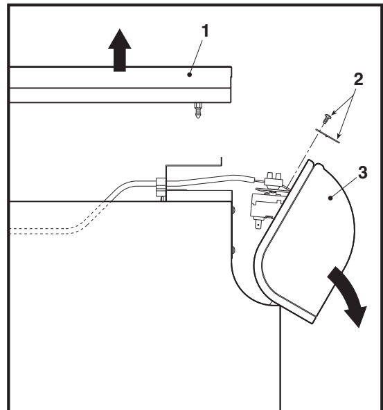
fig. 2 - Ouverture panneau de commande
