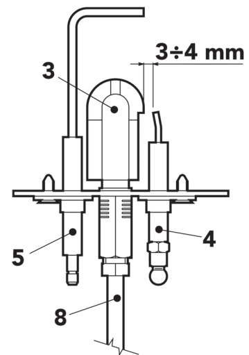
fig. 8 - Bruciatore pilota
