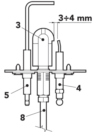
şek. 8 - Pilot brülör
