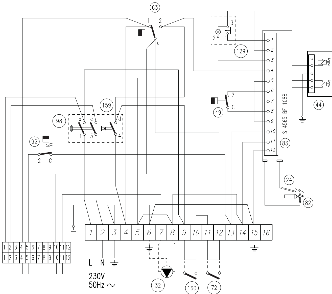
fig. 15 - Schema elettrico di allacciamento
