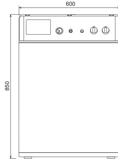
fig. 9 - Vista frontale
