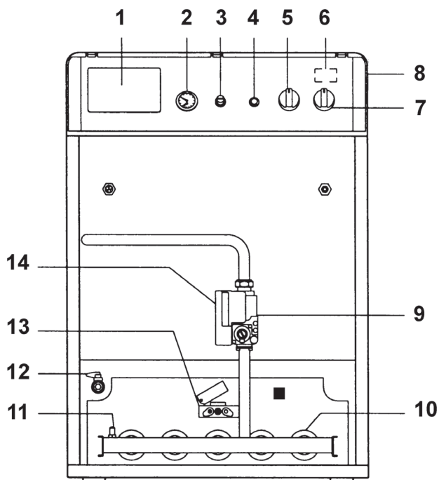
fig. 12 - Vista general
