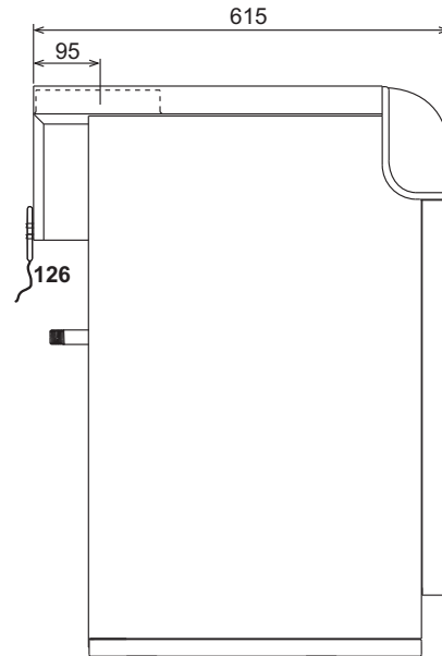
fig. 10 - Vista laterale
