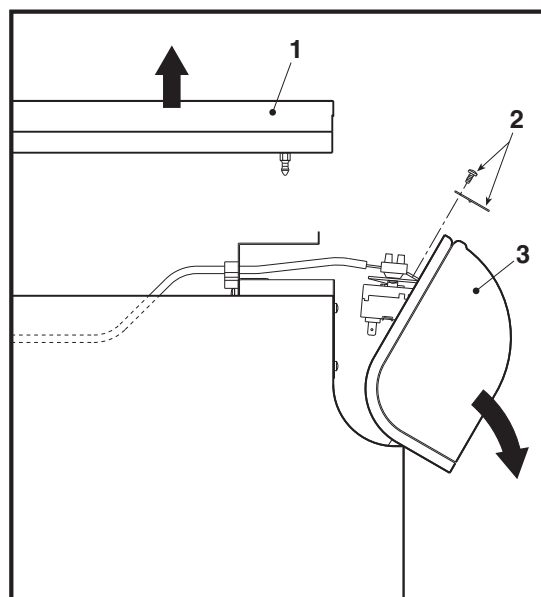
fig. 2 - Apertura cruscotto
