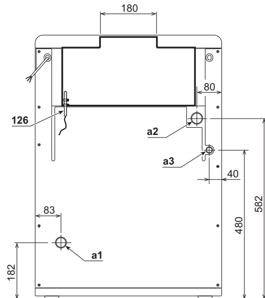
fig. 11 - Vista posteriore
