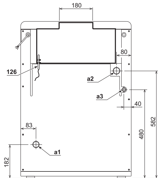
fig. 11 - Vista posterior
