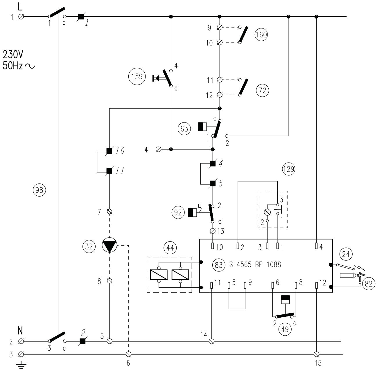
fig. 14 - Schéma électrique de base
