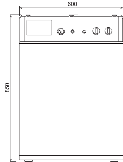
fig. 9 - Vue avant
