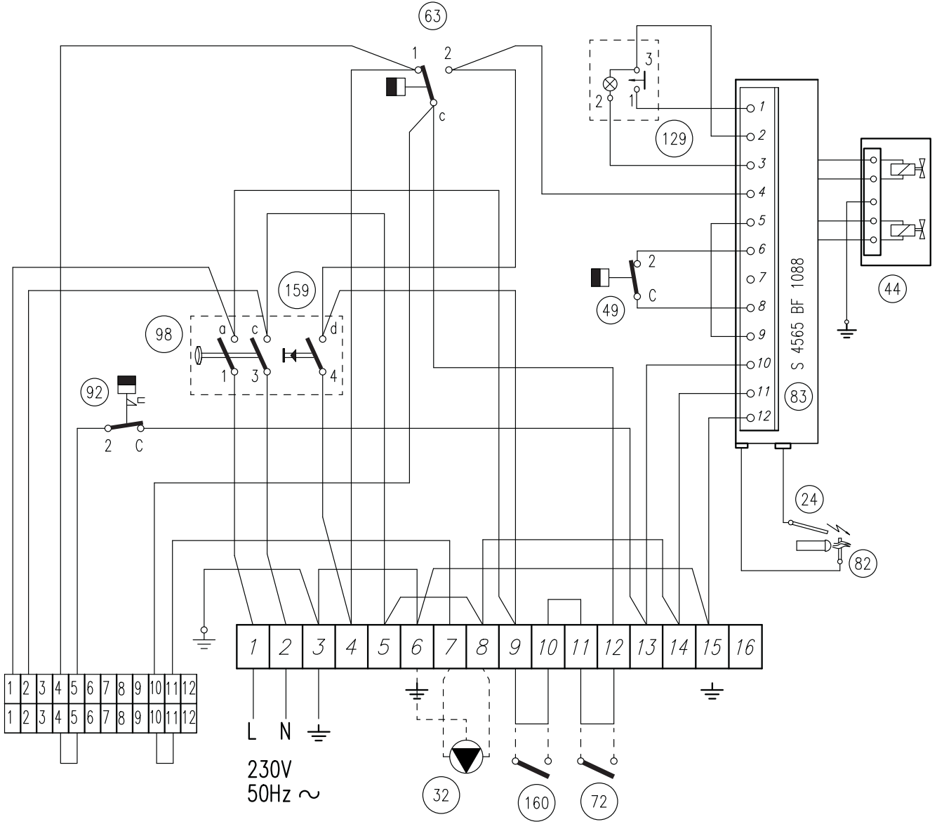
şek. 15 - Elektrik bağlantı şeması
