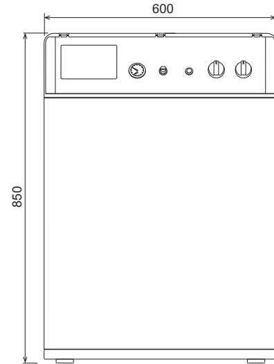
fig. 9 - Vista frontal
