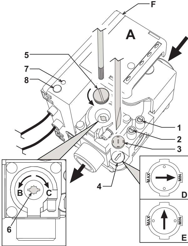
şek. 3 - Basıncın ayarlanması
