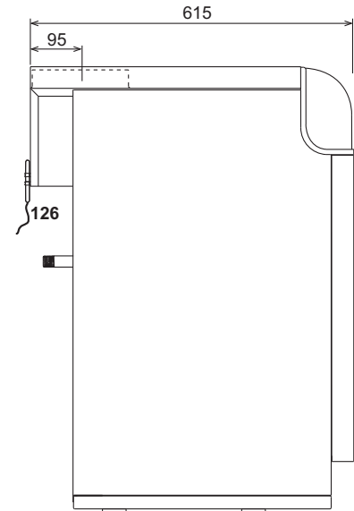
fig. 10 - Vista lateral
