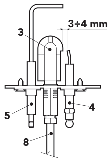
fig. 8 - Brûleur pilote
