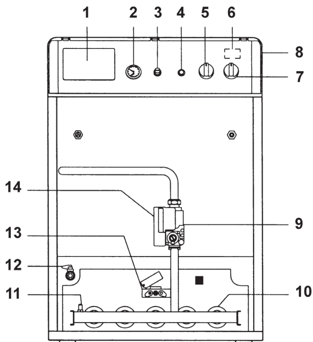
fig. 12 1.4 Vue générale
