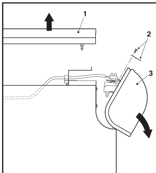
fig. 2 - Apertura del panel de mandos
