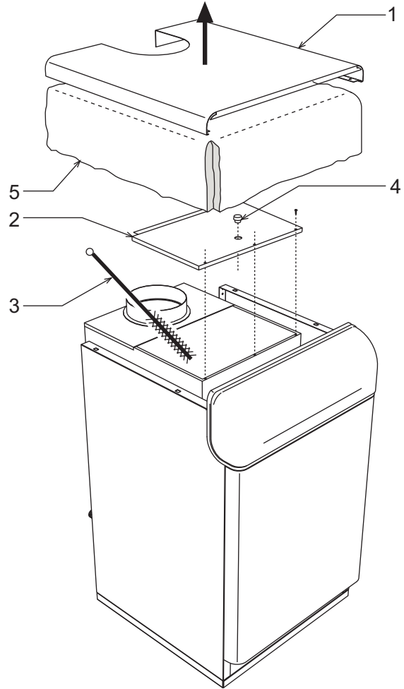
fig. 5 - Nettoyage de la chaudière
