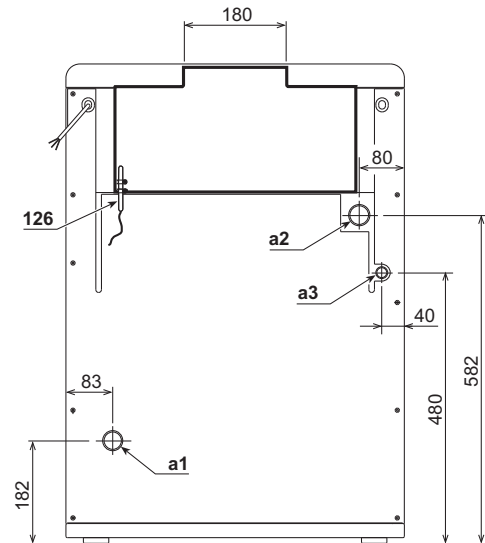
fig. 11 - Vue arrière
