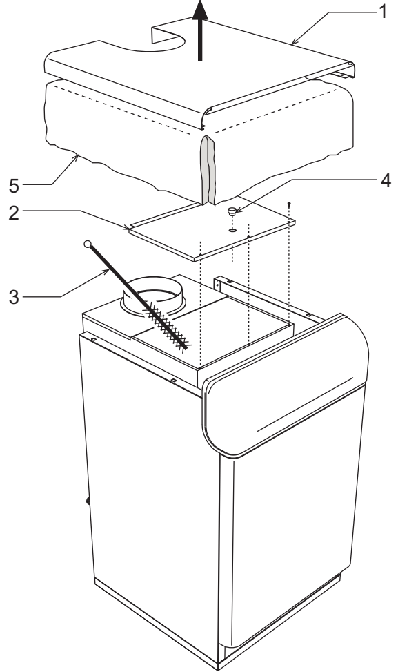
şek. 5 - Kombinin temizlenmesi
