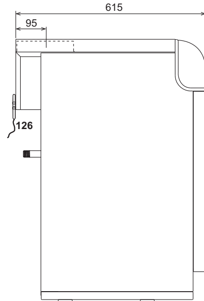
fig. 10 - Vue latérale
