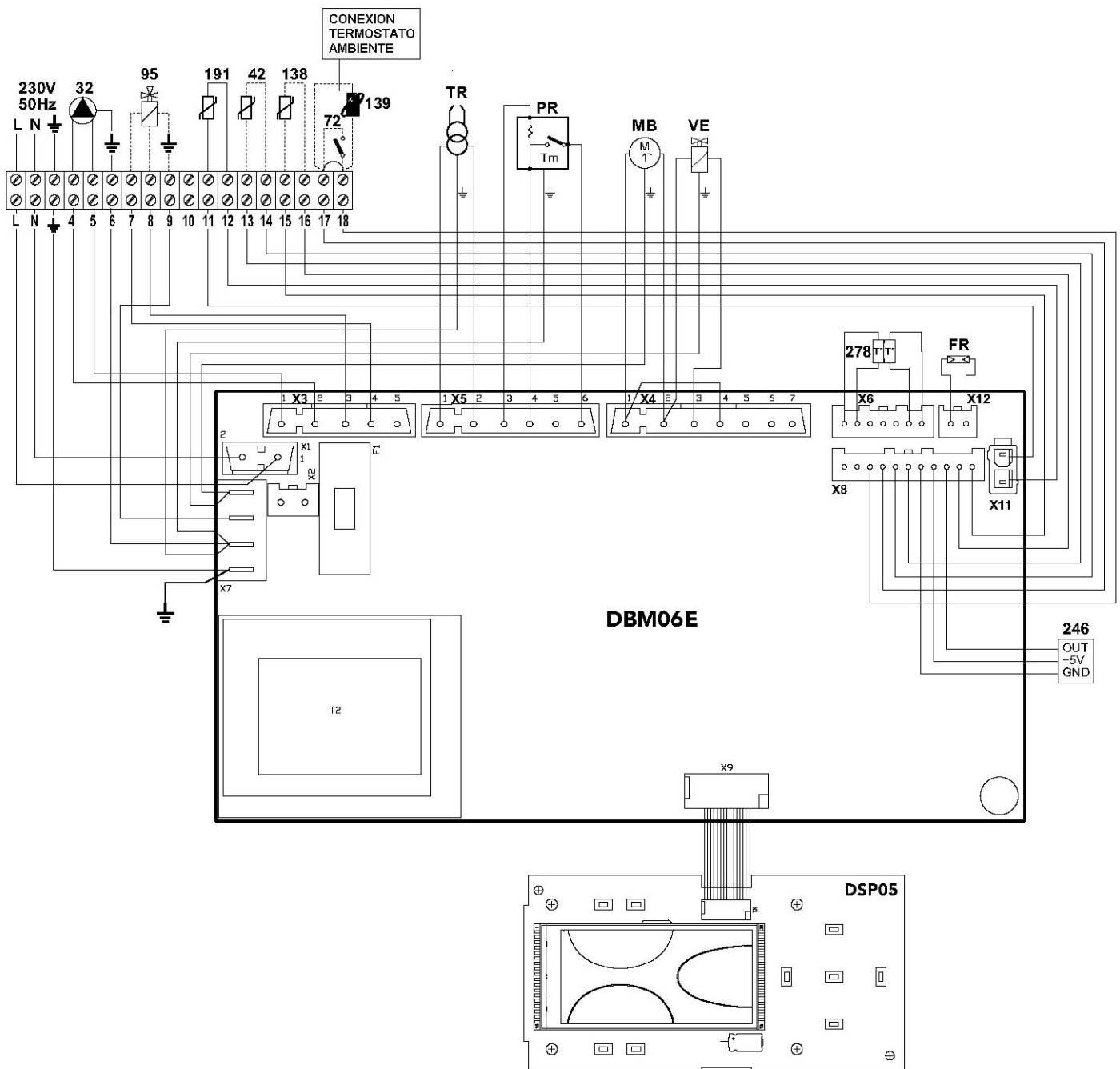
fig.45 – Schema elettrico
