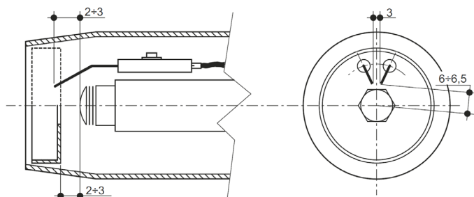
fig.32 - Posizione elettrodi - deflettore
