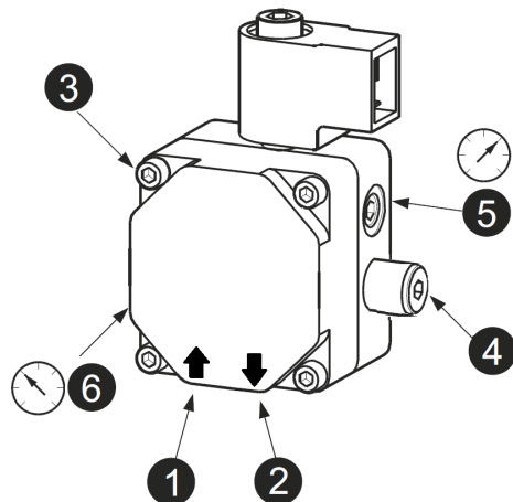
fig.29 - Pompa DANFOSS
