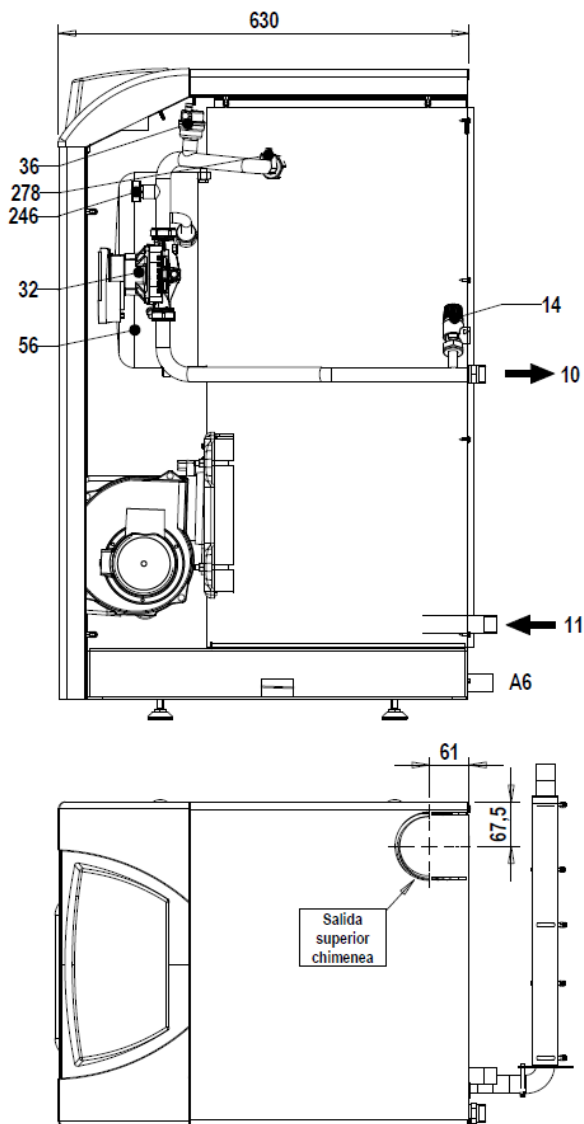
fig.40 - Vista laterale e superiore
