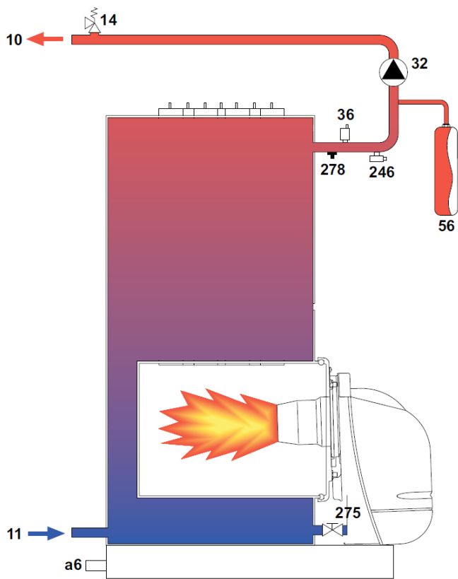
fig.42 – Circuito idraulico
