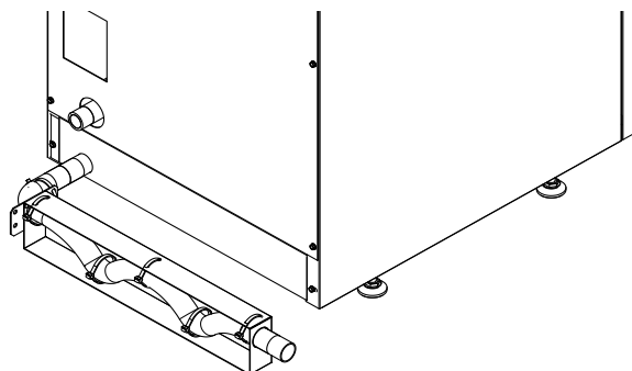
fig.26 – Scarico condensa
