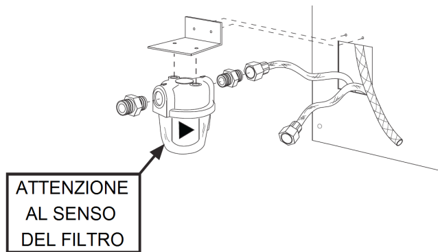
fig.21 - Installazione filtro combustibile
