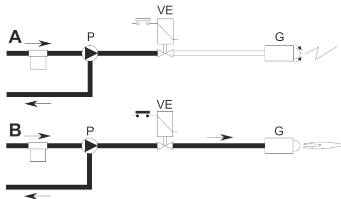
fig.33 - Avviamento
