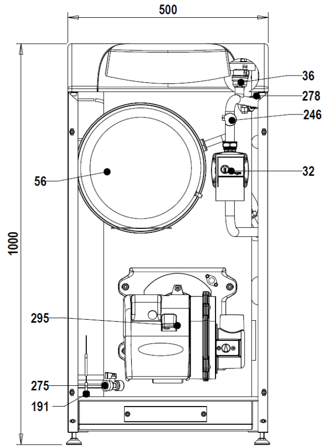
fig.41 - Vista frontale
