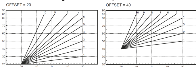
fig.15 - Esempio di spostamento parallelo delle curve di compensazione
