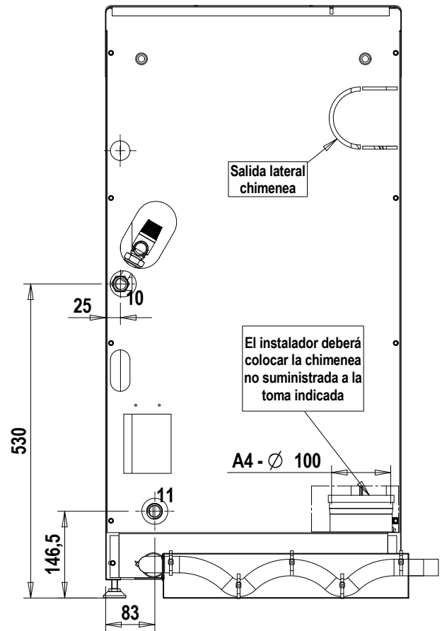
fig. 40 - Vista posteriore
