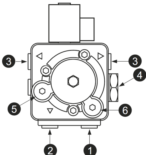
fig.28 - Pompa ITALPUMP
