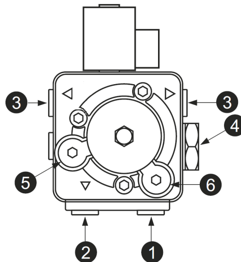
fig.26 - Pompa ITALPUMP
