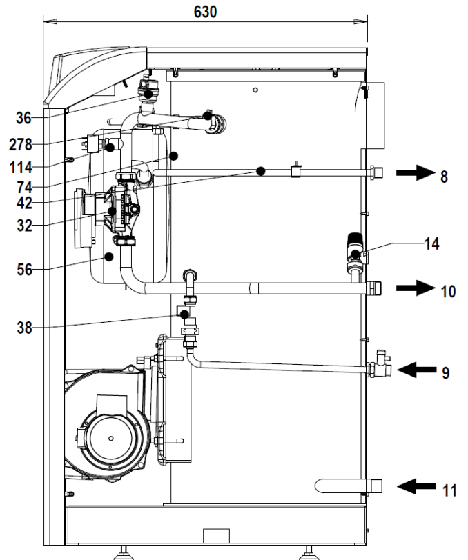
fig.38 - Vista laterale
