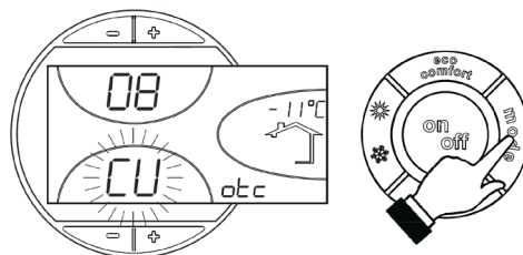
fig.12 - Curva di compensazione
