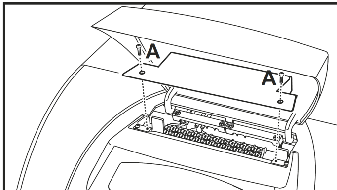
fig.24 – Accesso alla morsetteria
