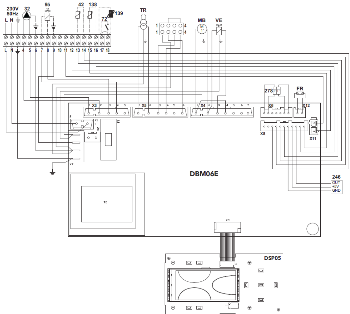
fig.43 - Schema elettrico
