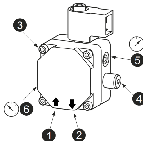
fig.27 - Pompa DANFOSS
