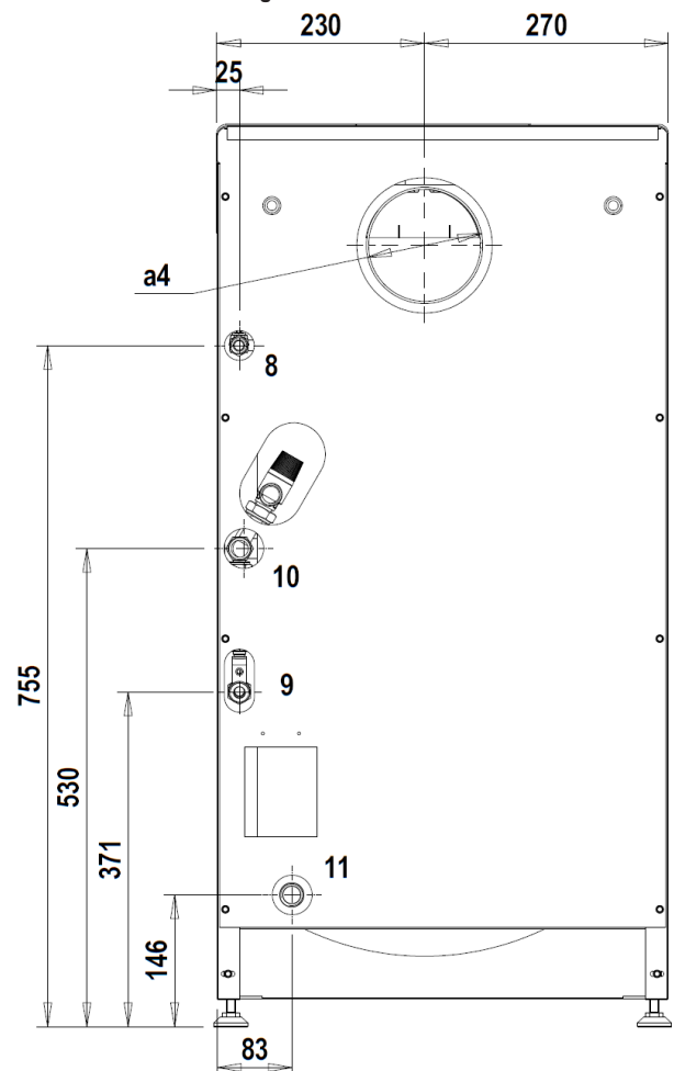
fig.39 - Vista posteriore
