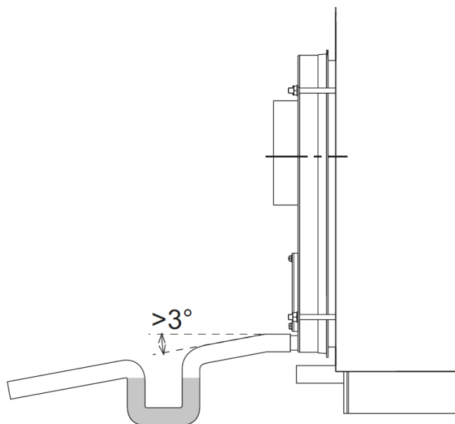
fig. 8 - Condensate discharge
