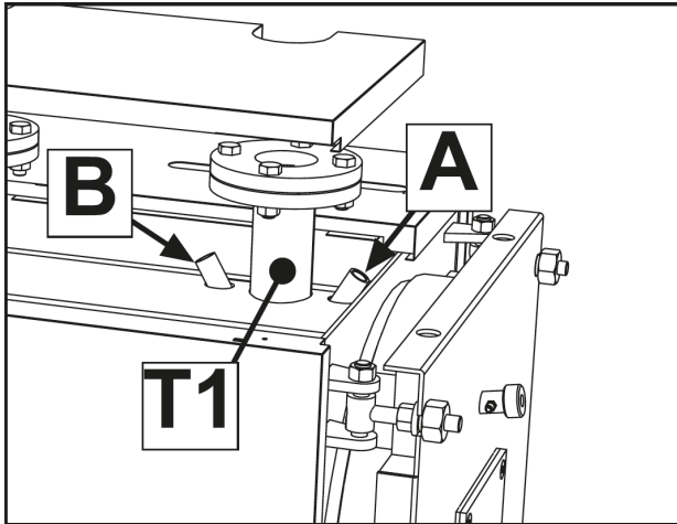
fig. 15 - Alojamiento sondas y bulbos
