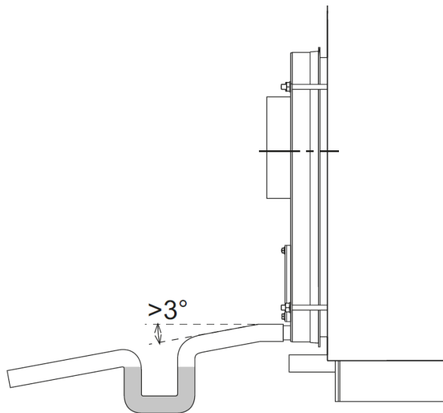
fig. 8 - Scarico condensa
