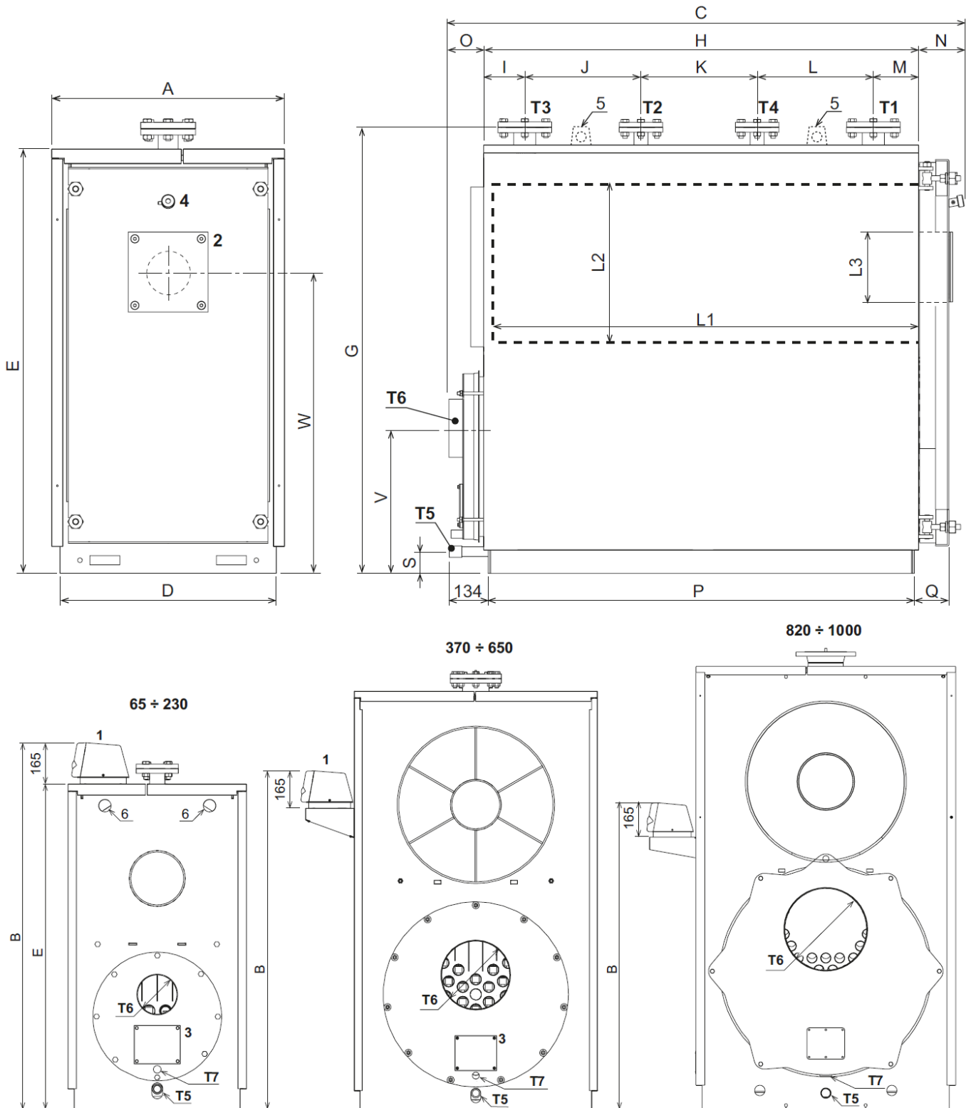
fig. 2 - Medidas y conexiones
