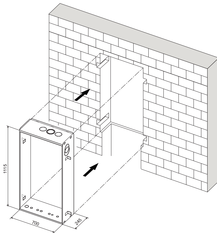
fig. 16 - Fissaggio dell'involucro alla parete
