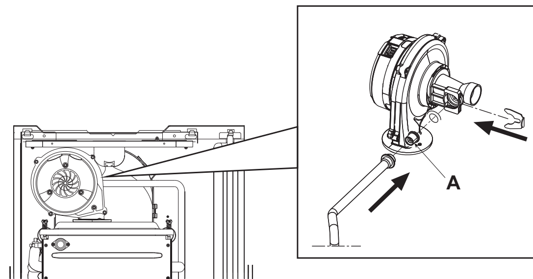
fig. 28 - Sostituzione ugello gas
