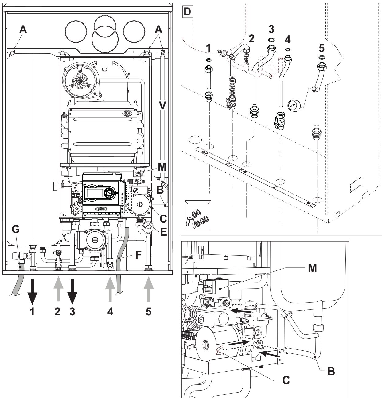
fig. 18 - Collegamento attacchi idraulici e gas / Kit tubi attacchi
