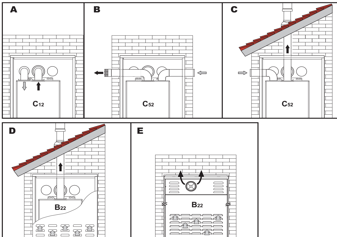
fig. 23 - Esempi di collegamento con tubi separati (⇨ = Aria / ⇨ = Fumi)
