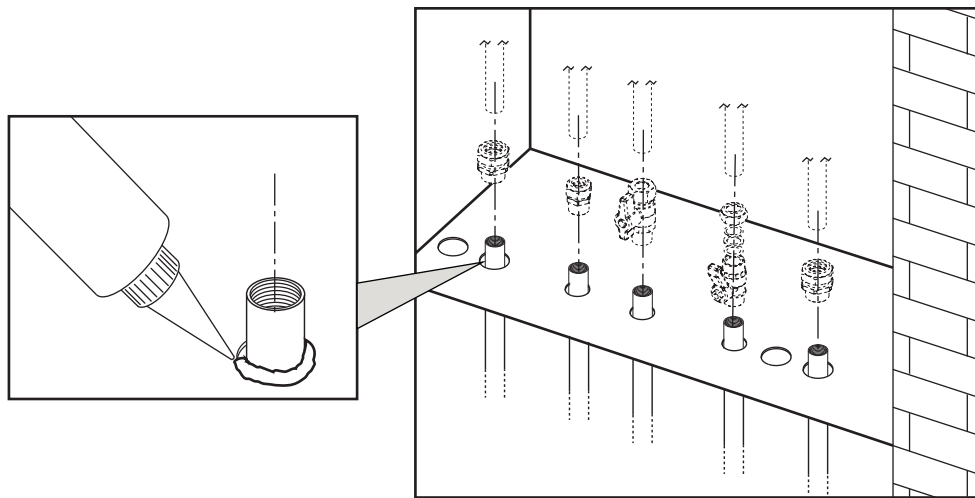
fig. 19 - Sigillatura involucro
