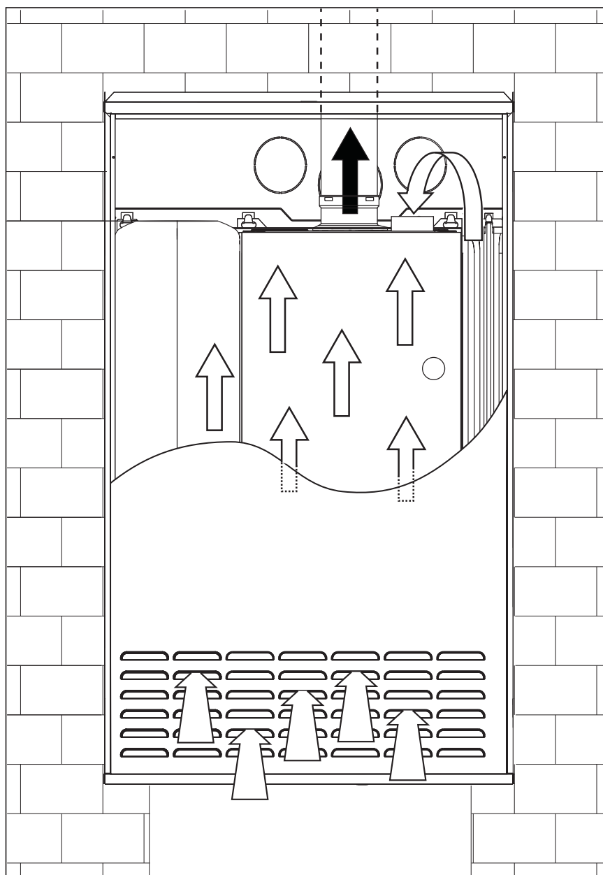
fig. 25 - Prelievo aria
