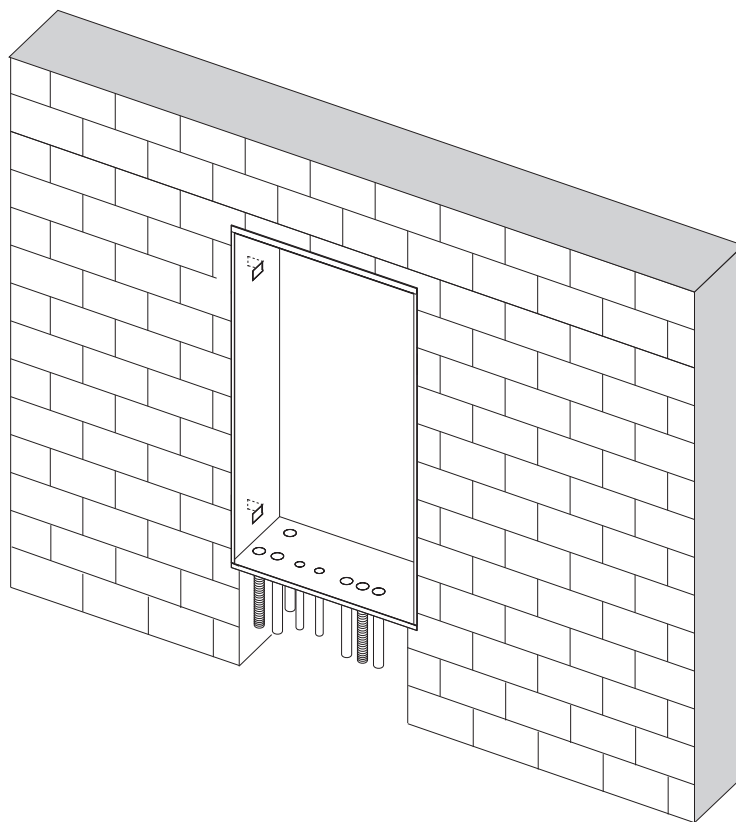
fig. 17 - Allacciamenti all'involucro
