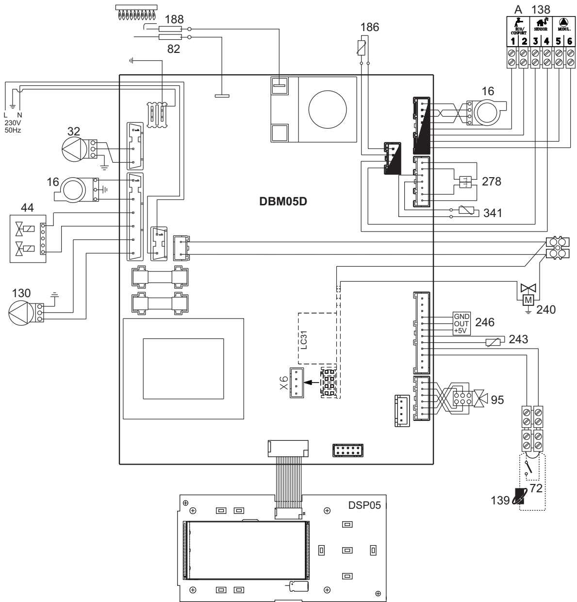
fig. 36 - Schema elettrico
