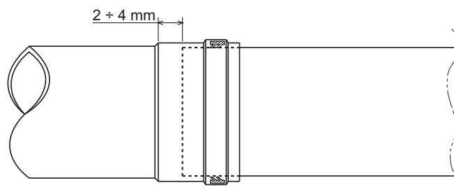
fig. 20 - Dilatazione
