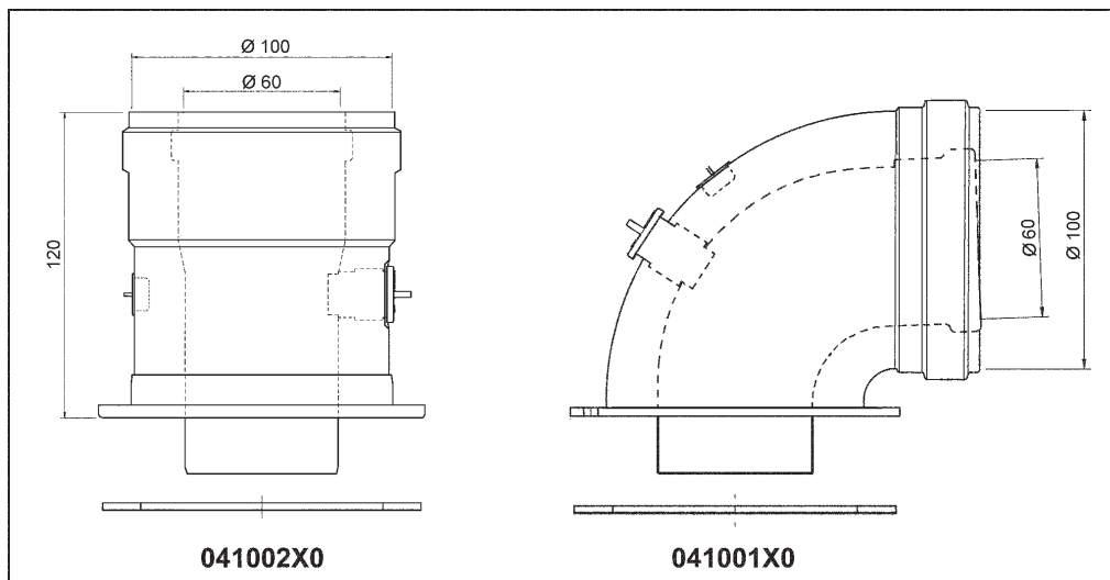
fig. 22 - Accessori di partenza per condotti coassiali
