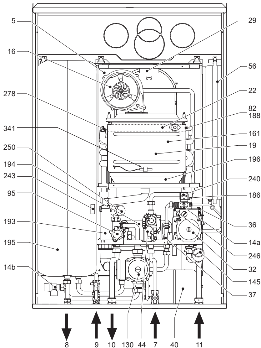
fig. 33 - Vista generale
