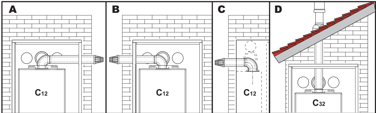
fig. 21 - Esempi di collegamento con tubi coassiali
