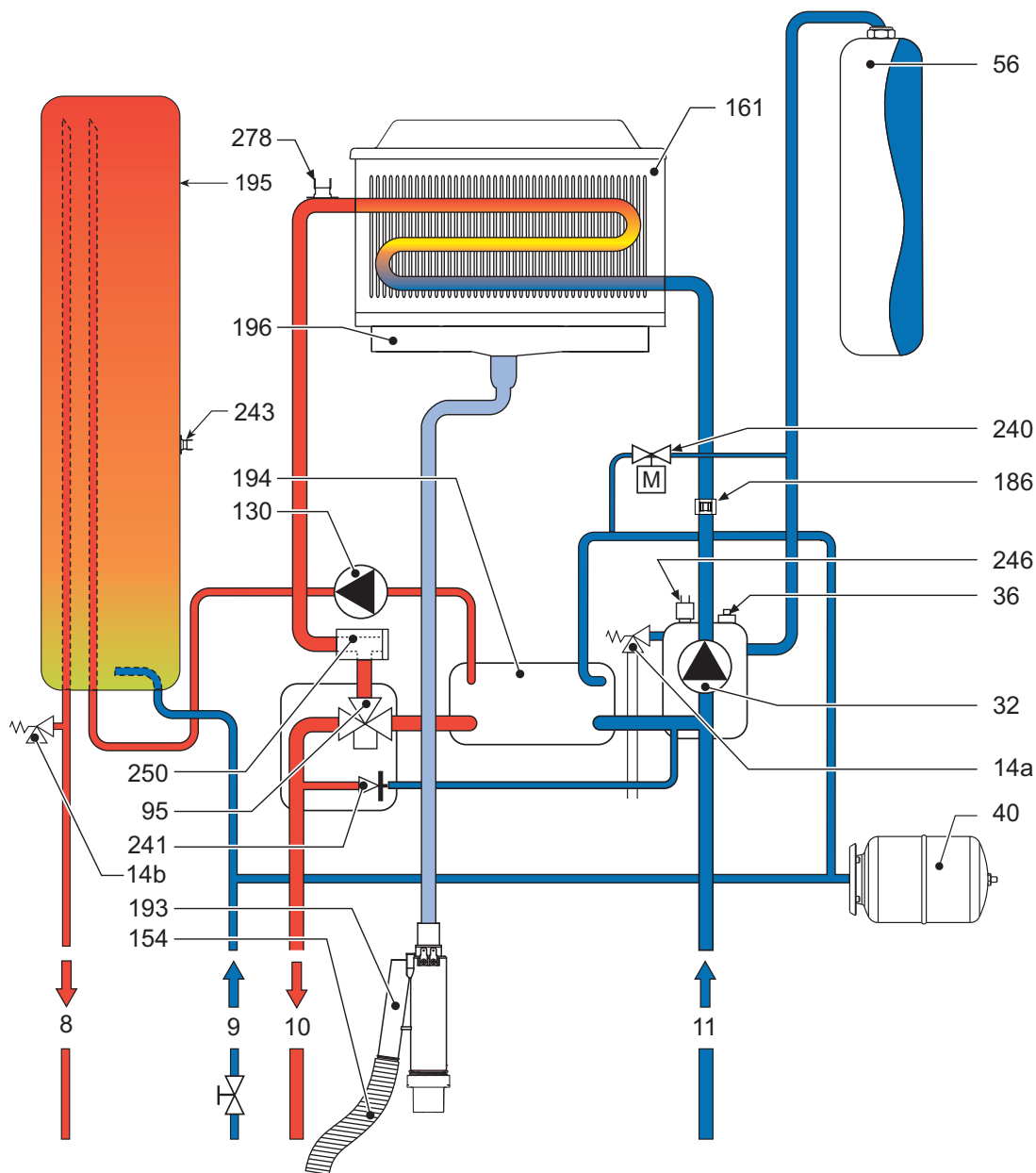
fig. 34 - Circuito idraulico
