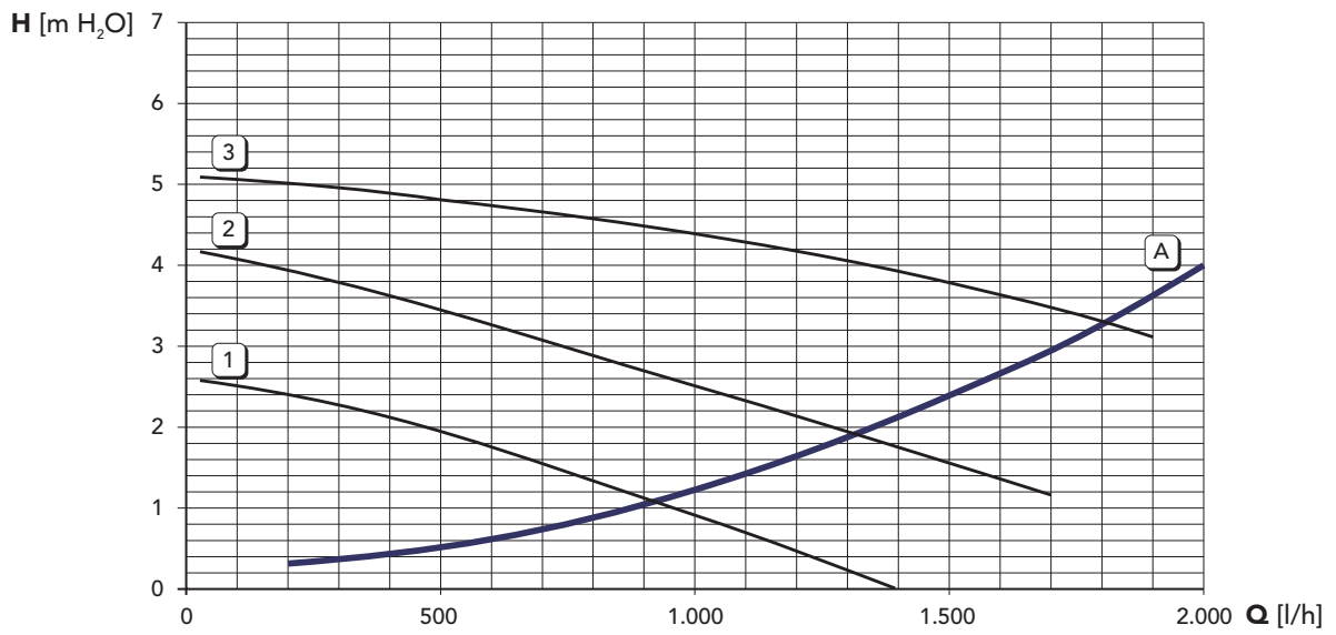
fig. 35 - Perdita di carico/prevalenza circolatori
