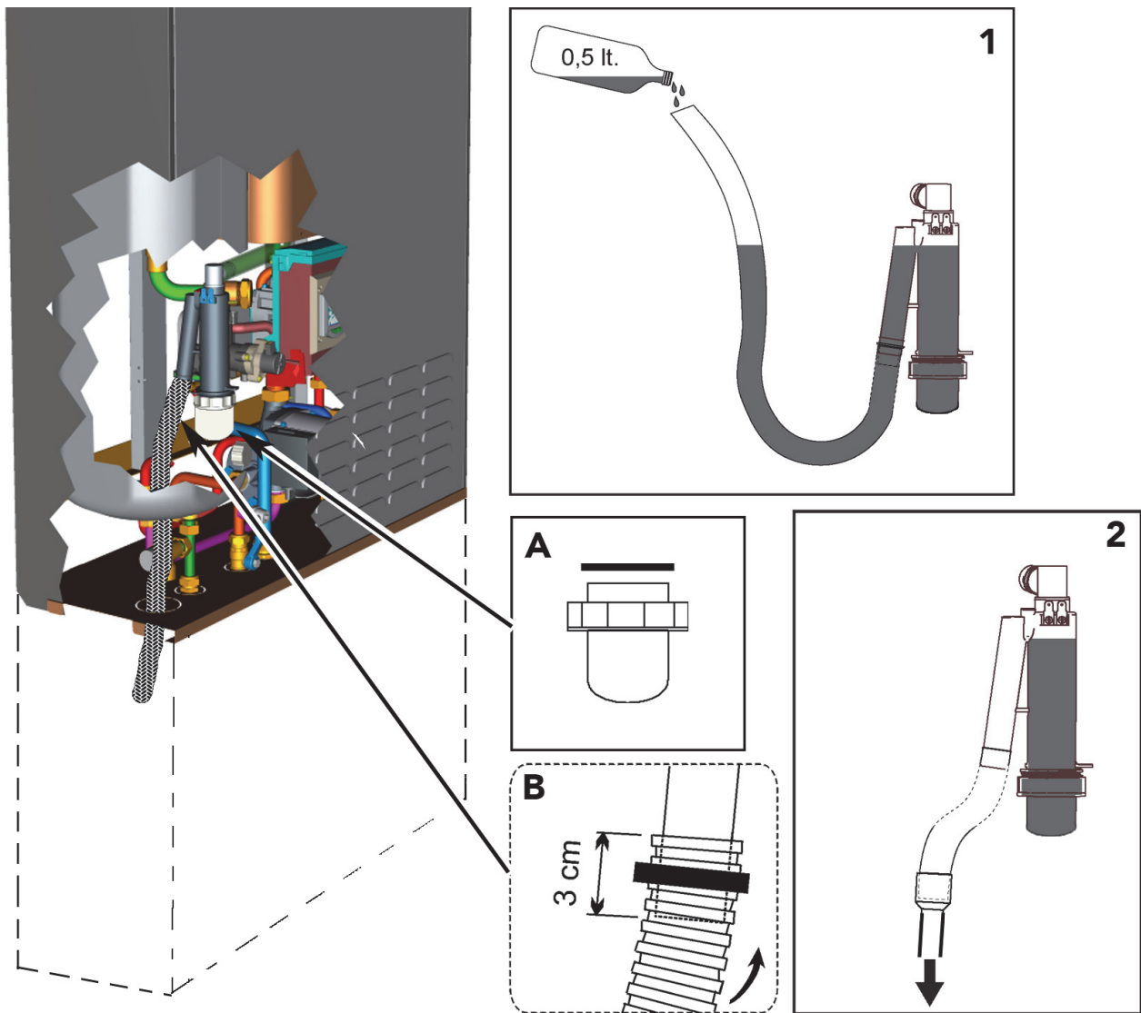
fig. 27 - Scarico condensa
