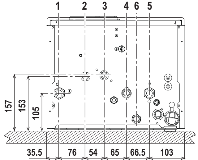
şek. 13 - Su bağlantıları
