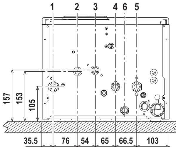
fig. 13 - Racorduri hidraulice
