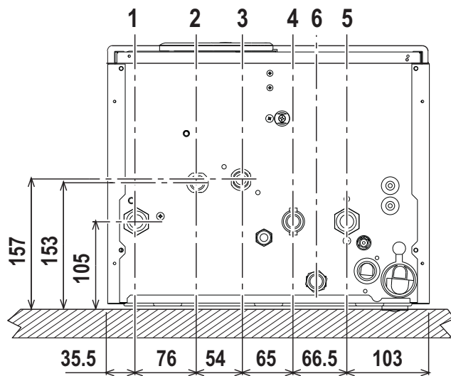
fig. 13 - Attacchi idraulici
