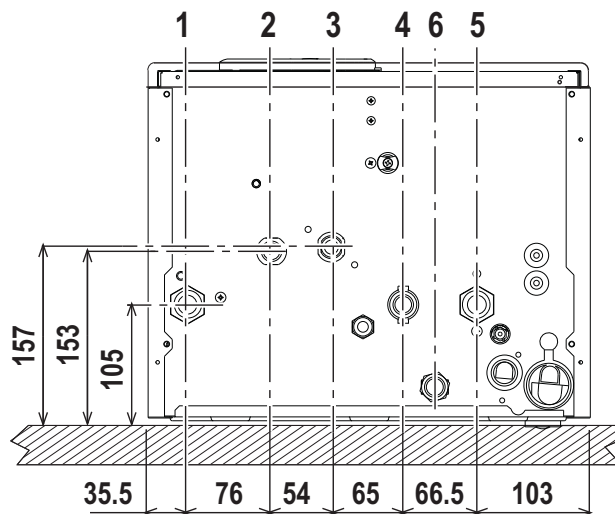
fig. 13 - Conexiones hidráulicas
