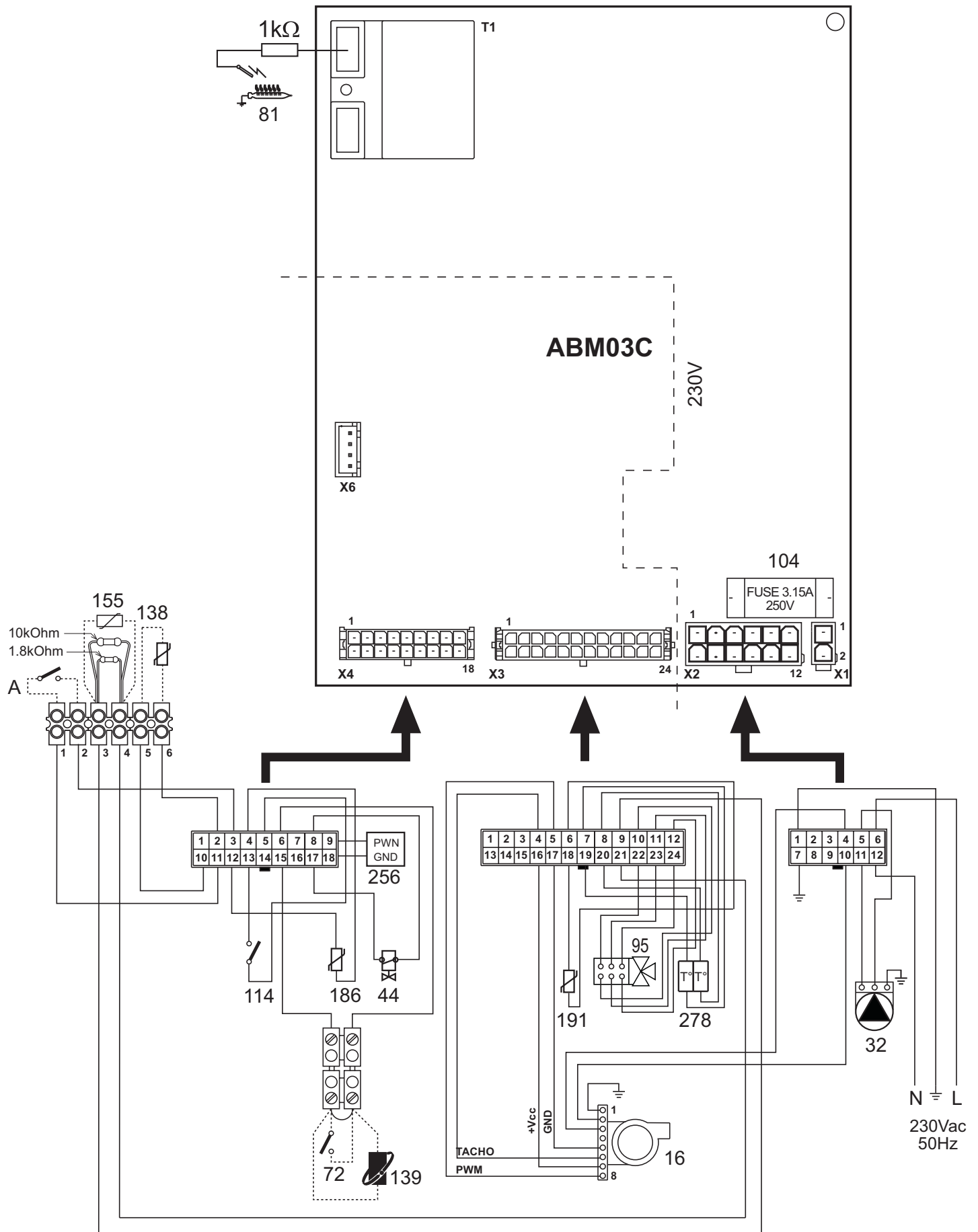
fig. 31 - Schéma électrique
