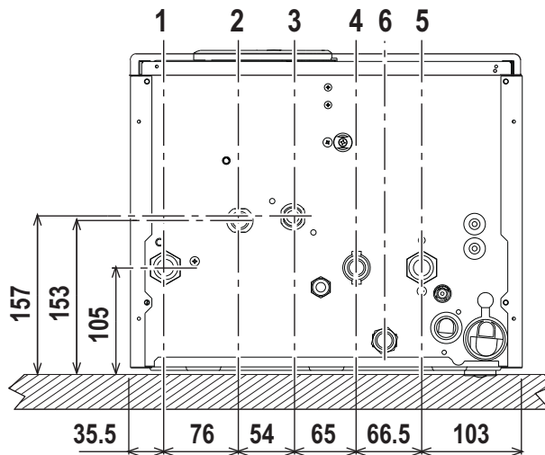
мал. 13 - Водопровідні штуцери
