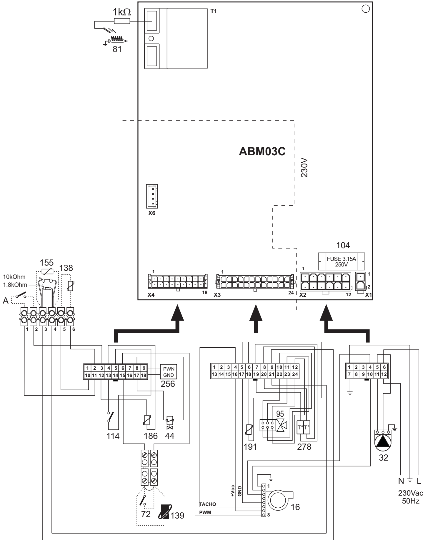
рис. 31 - Электрическая схема
