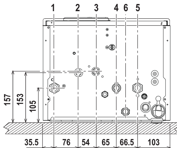
рис. 13 - Гидравлические штуцеры
