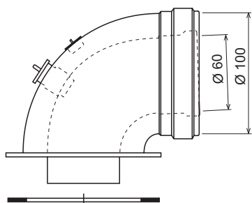
fig. 17 - Accesorii de pornire pentru conducte coaxiale
