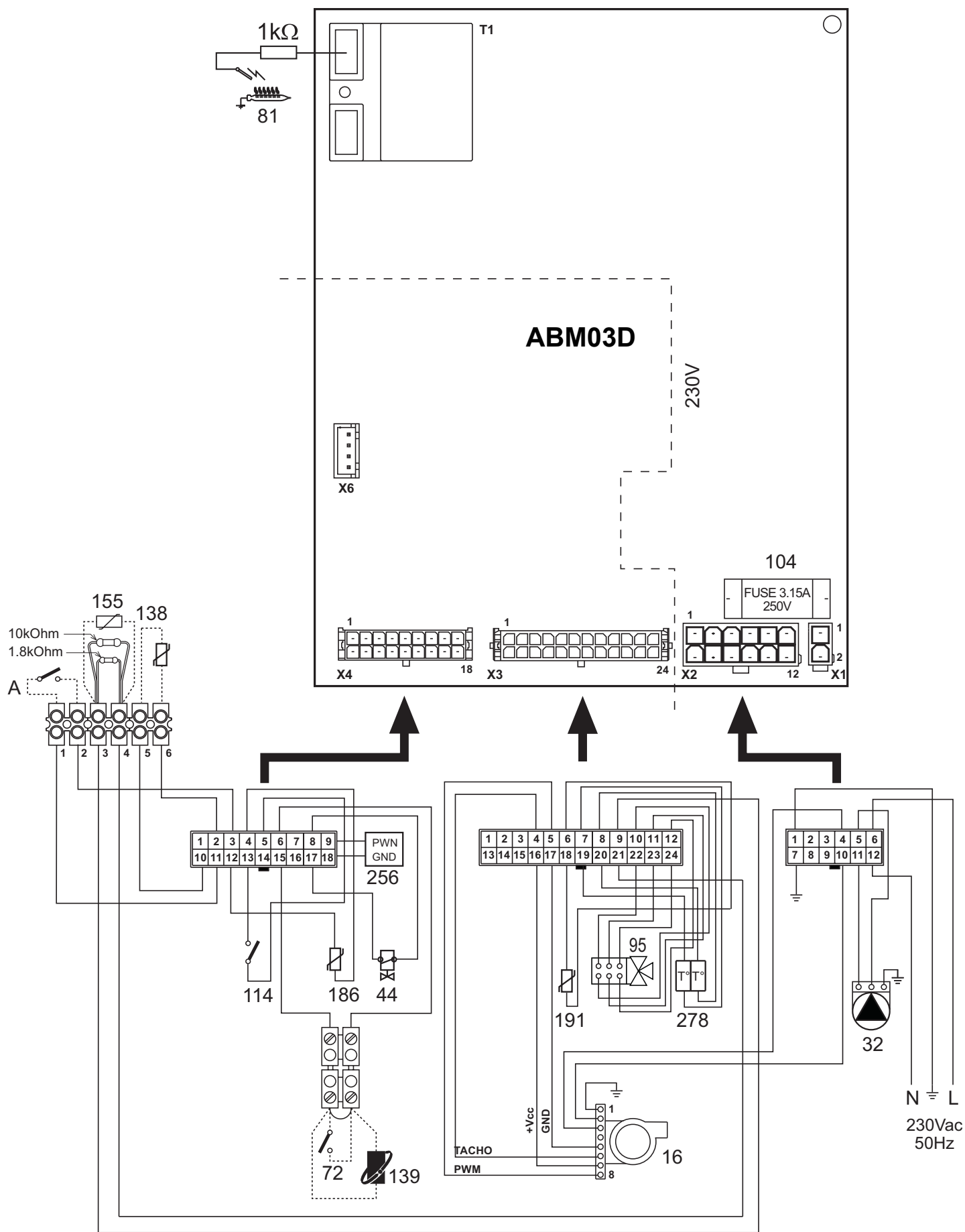
fig. 31 - Schemă electrică
