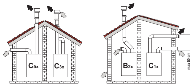
мал. 18 - Приклад підключення за допомогою відокремлених труб (→ = Повітря / → = Відпрацьовані газів)
