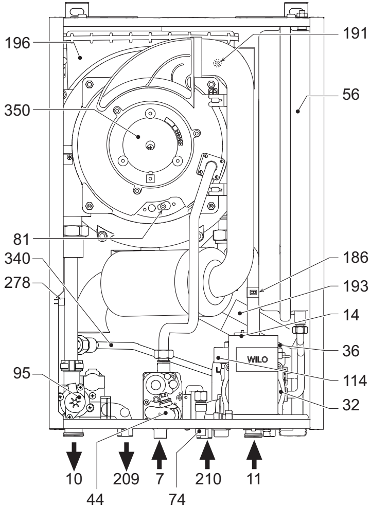
рис. 27 - Общий вид
