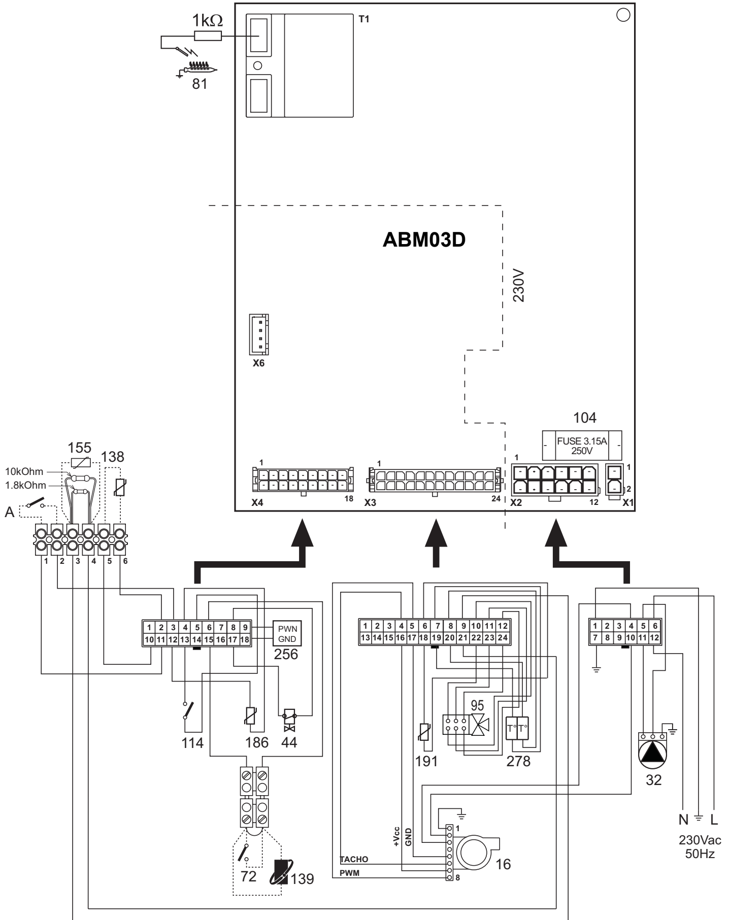
fig. 31 - Schema elettrico
