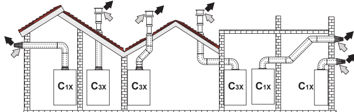
мал. 16 - Приклад підключення за допомогою співісних (коаксіальних) труб (→ = Повітря / → = Відпрацьовані газів)
