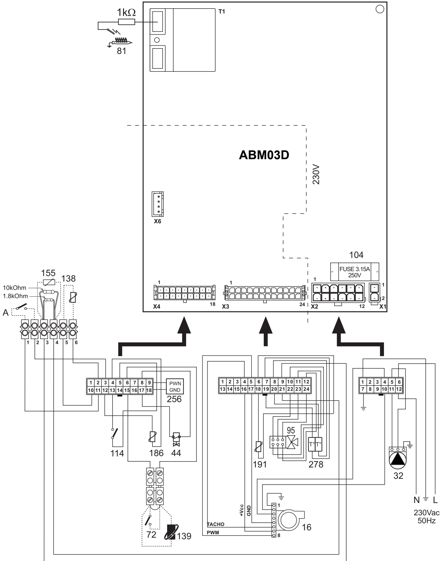
fig. 31 - Schéma électrique
