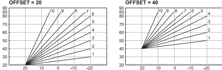
şek. 11 - Kompensasyon eğrilerinin paralel hareketi için örnek
