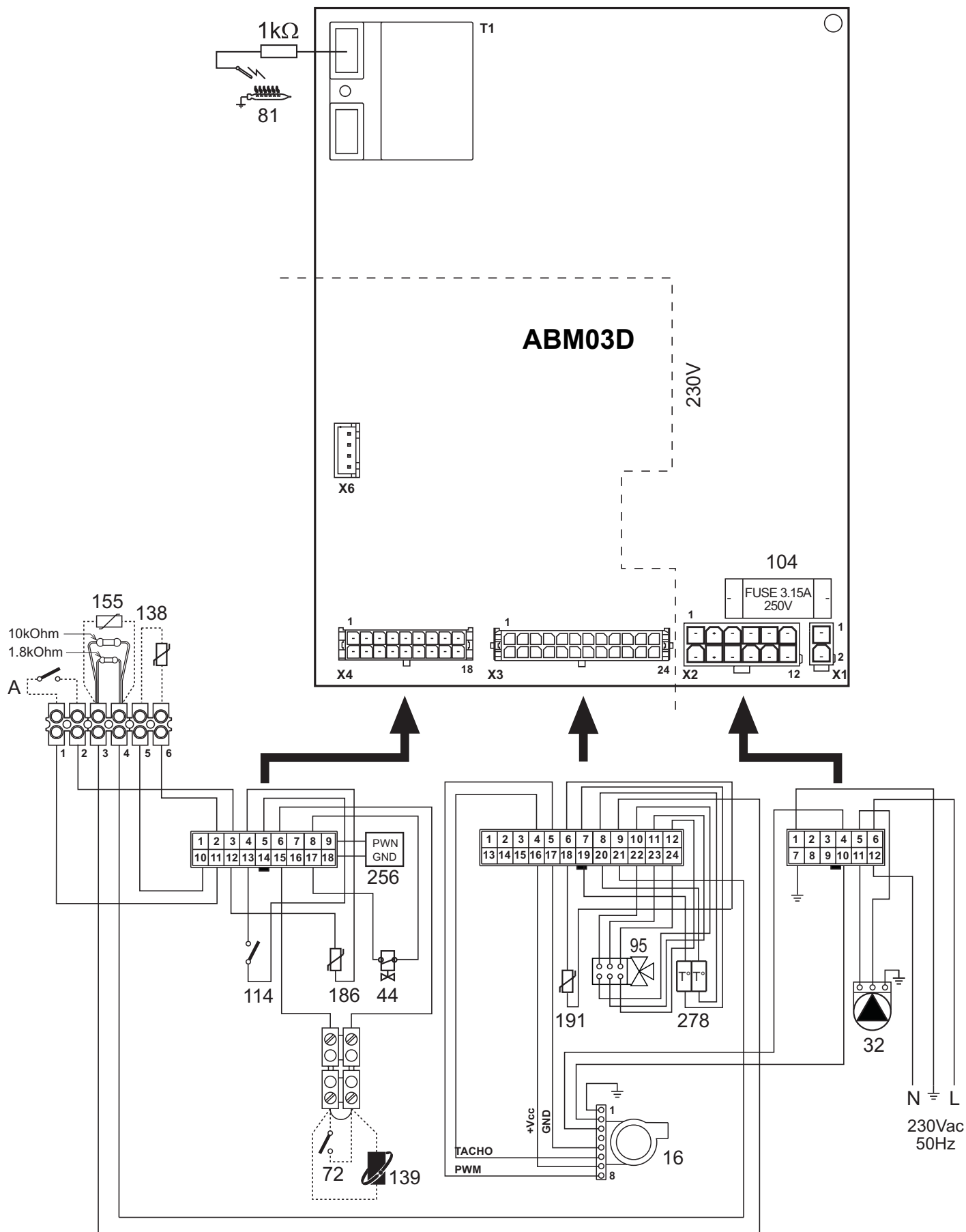
fig. 31 - Wiring diagram
