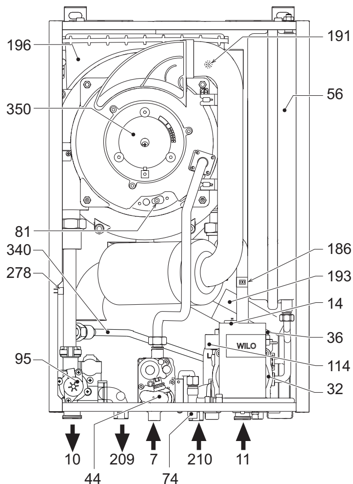
fig. 27 - Vista generale
