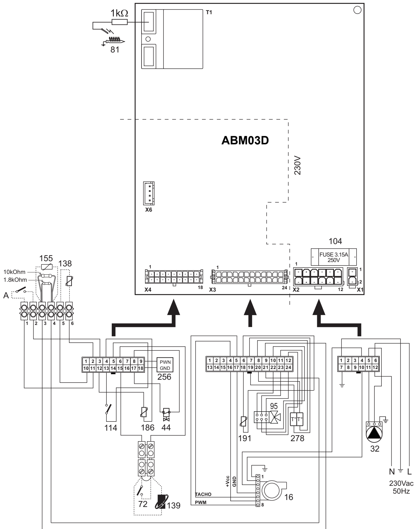
fig. 31 - Esquema eléctrico
