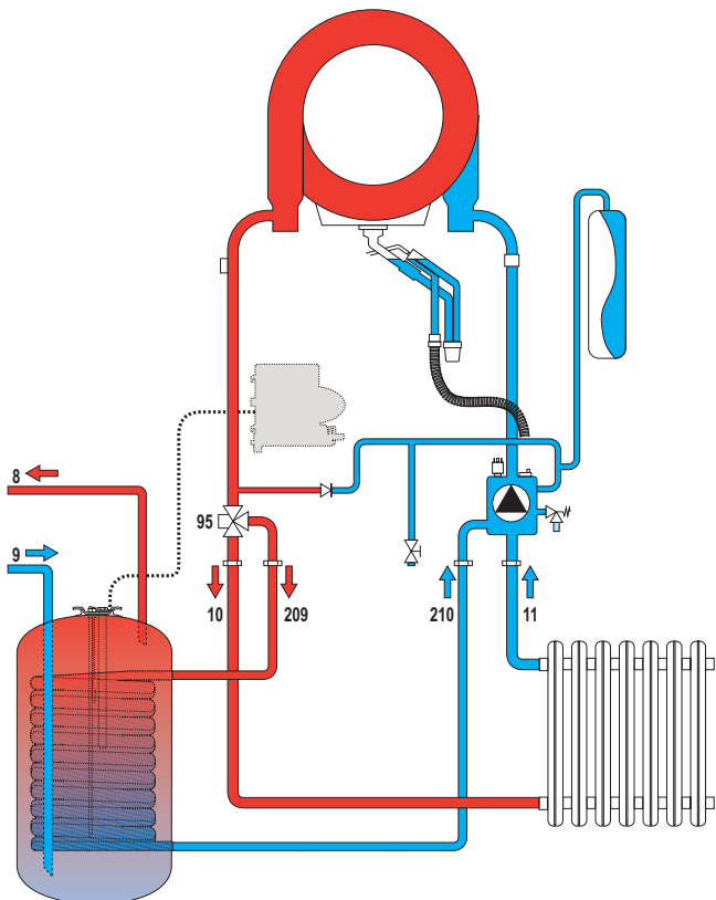
мал. 14 - Система підключення до зовнішнього бойлера
