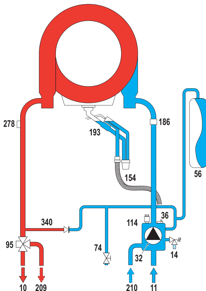
fig. 28 - Circuito idraulico
