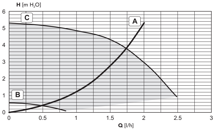
мал. 30 Втрати напору / напір циркуляційних насосів
