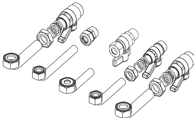
fig. 18 - Kit idraulico
