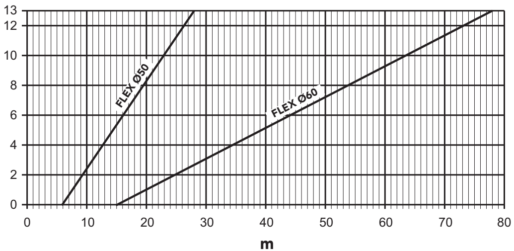
fig. 26- Chart for flue parameter choice
