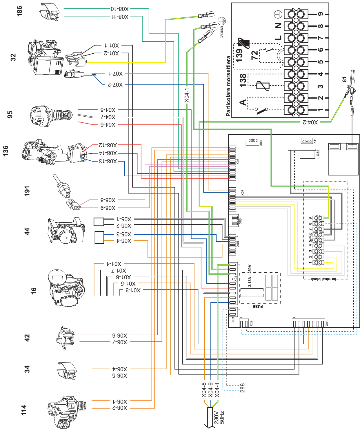
fig. 62- Esquema eléctrico
