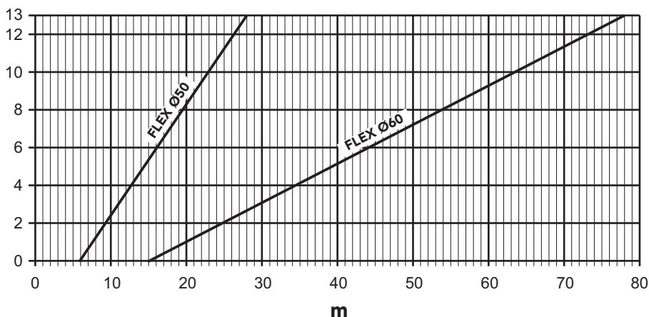
fig. 26 - Grafico per scelta parametro camino
