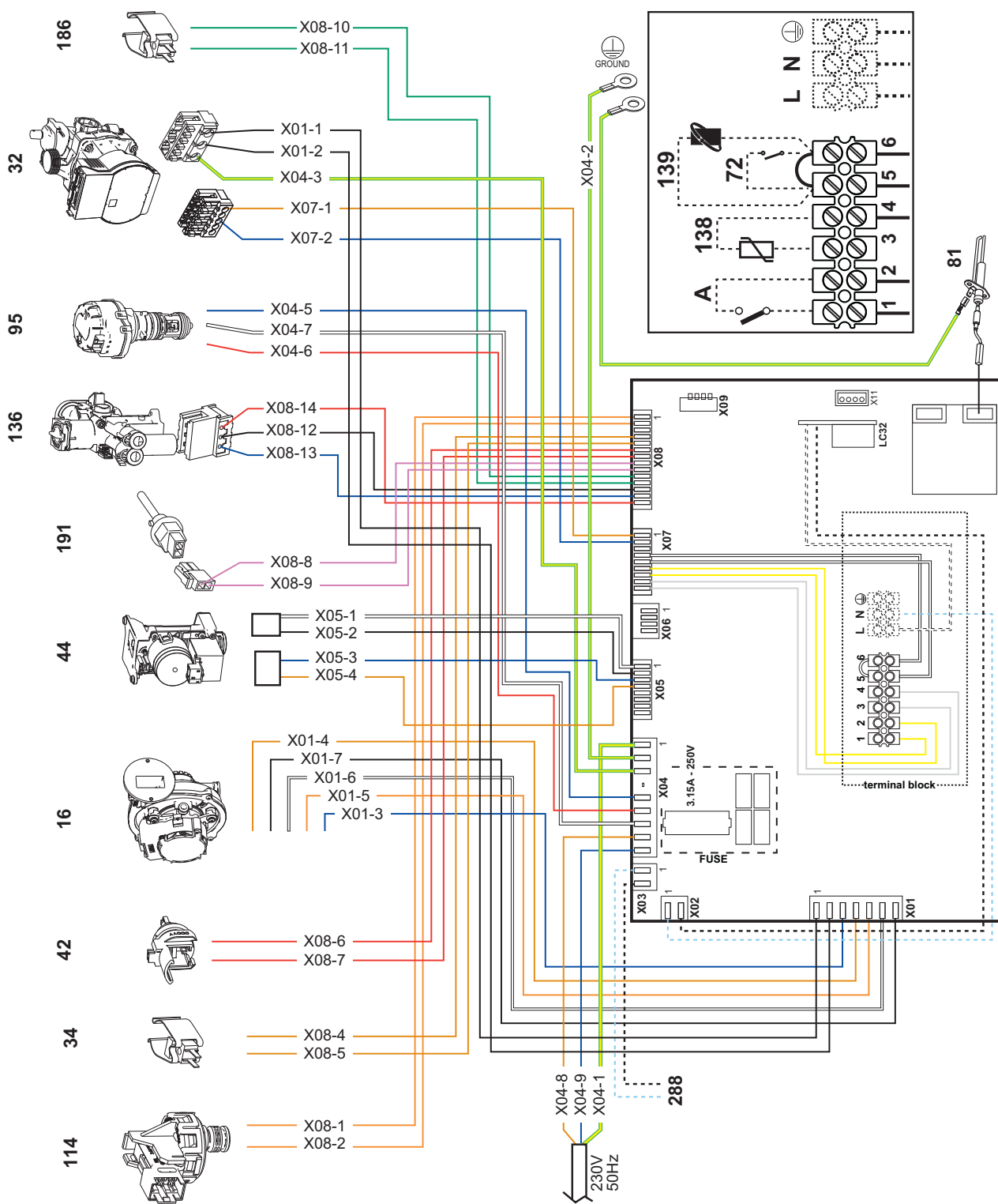
fig. 63- Esquema eléctrico
