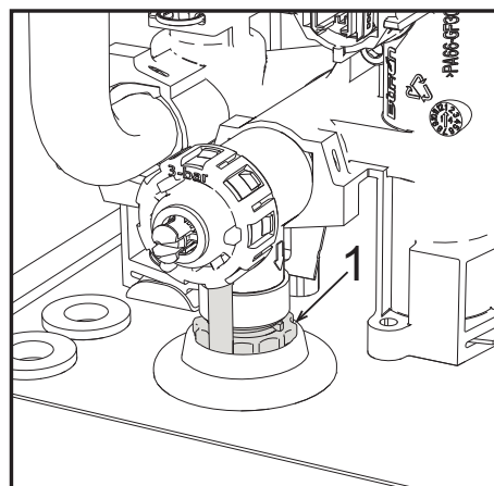
ΕΙΚ. 17- Βαλβίδα ασφαλείας με στρόφιγγα εκκένωσης
