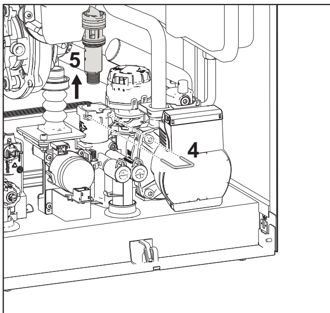
fig. 48- Caudalímetro
