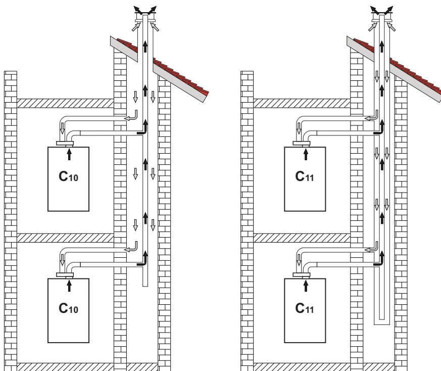
εικ. 28- Παραδείγματα σύνδεσης συστήματος C10 και C11 (⇨ = Αέρας / ⇨ = Καυσαέρια)
