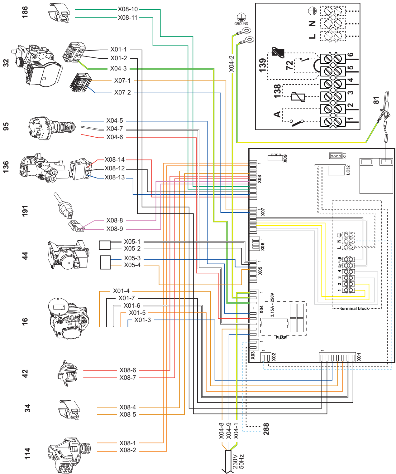
fig. 63 - Schema elettrico
