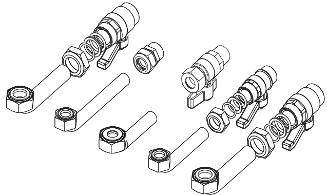
fig. 18 - Kit idraulico
