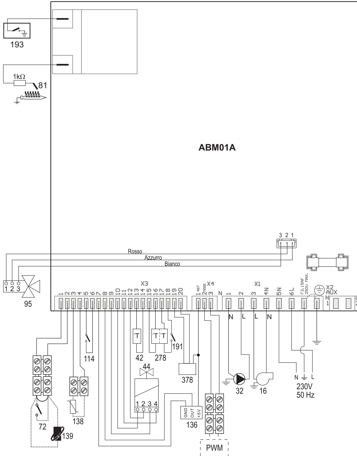
fig. 28- Schemă electrică
