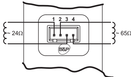
wygląd 18- Podłączenie zaworu gazowego
