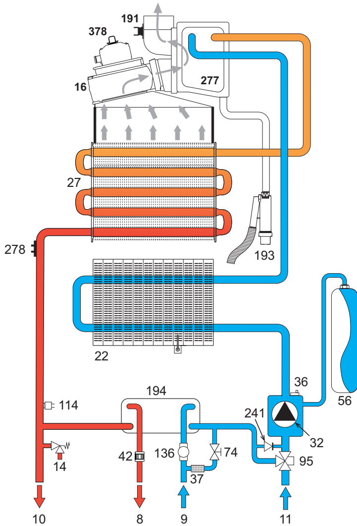
fig. 27 - Circuito riscaldamento
