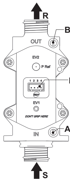
fig. 17 - Válvula del gas
