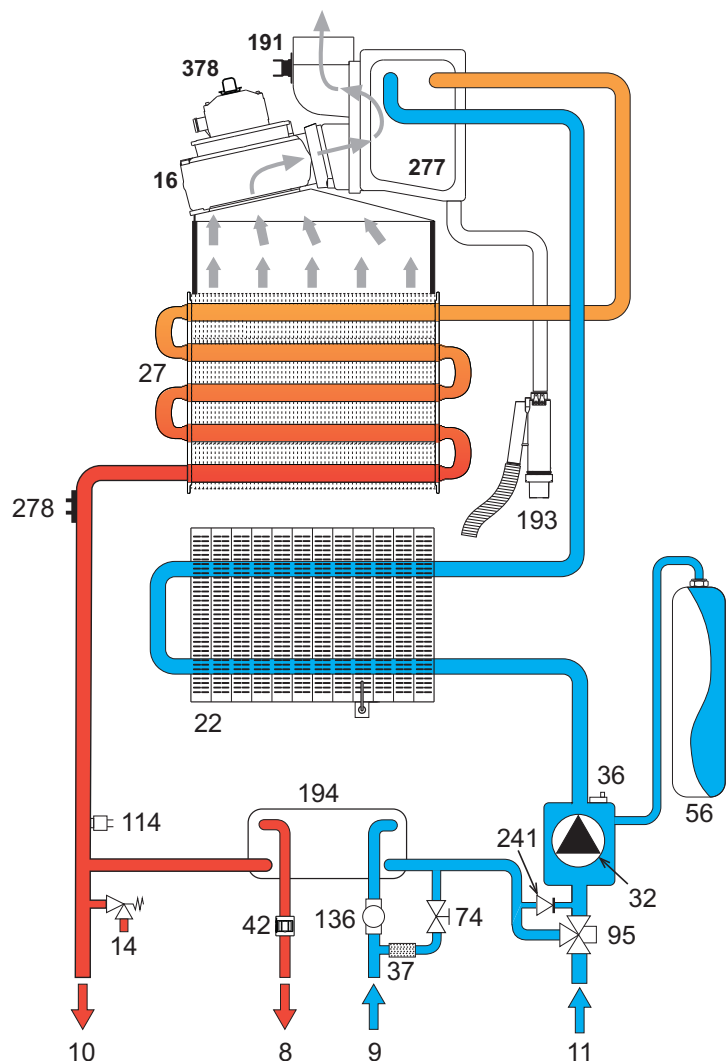
ΕΙΚ. 27- Κύκλωμα θέρμανσης
