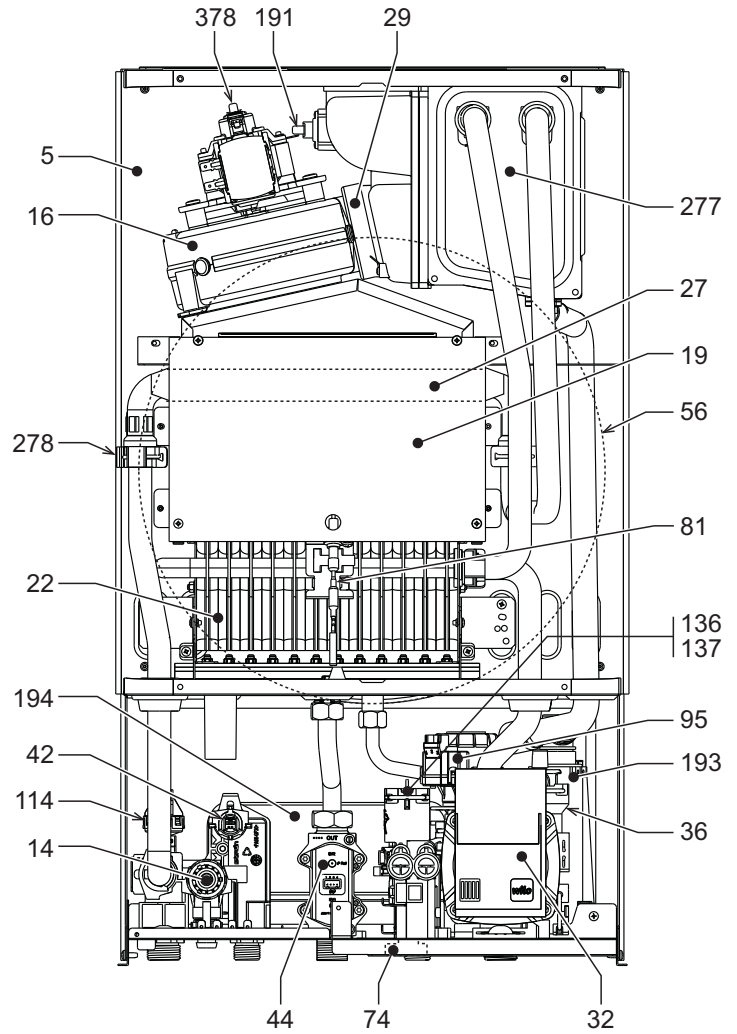
fig. 26- Vedere generală
