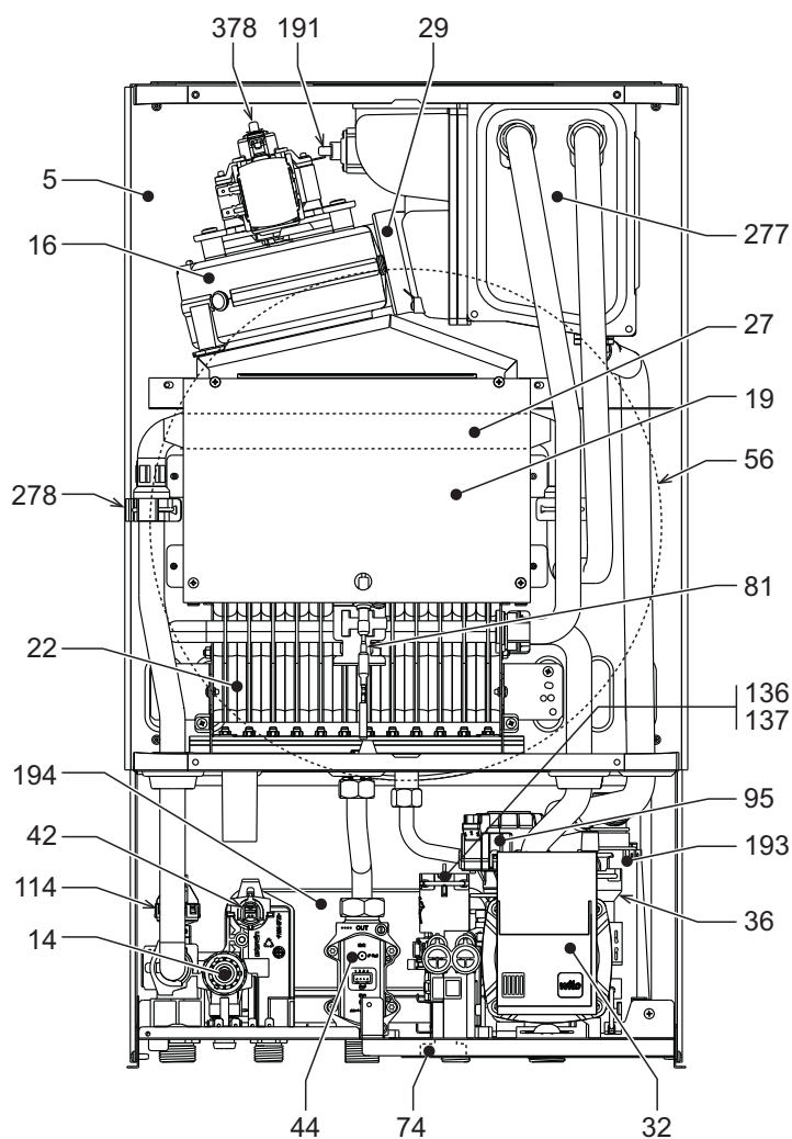
fig. 26- Vista general
