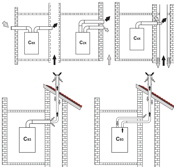
ΕΙΚ. 16 Παραδείγματα σύνδεσης σε κεντρικές καπνοδόχους (⇨ = Αέρας / ⇩ = Καυσαέρια)
