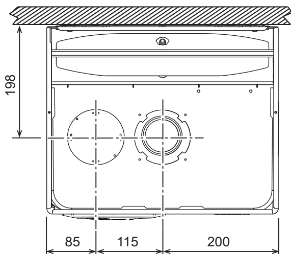
wygląd 23- Widok z góry
