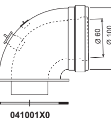
ΕΙΚ. 13 - Εξαρτήματα σύνδεσης για ομοαξονικούς αγωγούς
