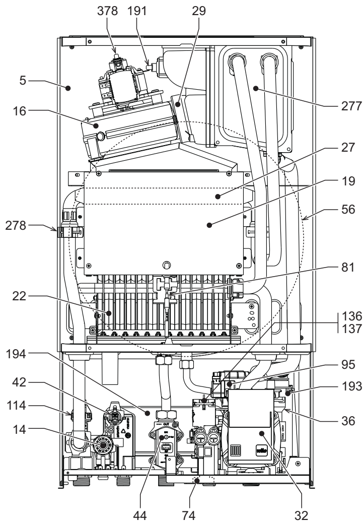
fig. 26 - Vista generale
