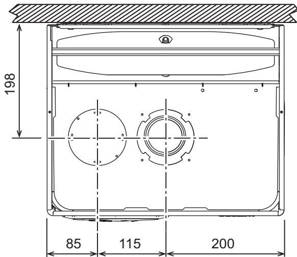
fig. 23- Vista superior
