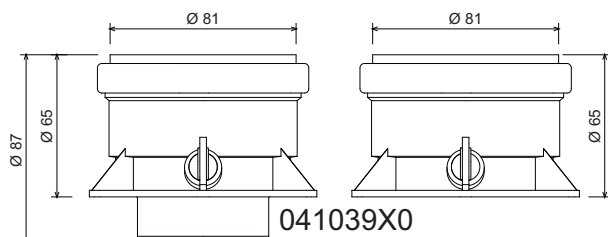
fig. 15 - Accessorio di partenza per condotti separati
