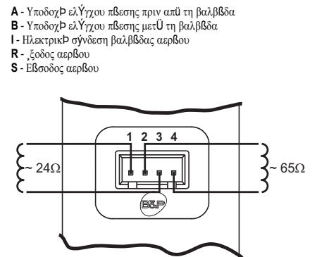
άεε. 18 - Σύνδεση βαλβίδας αερίου
