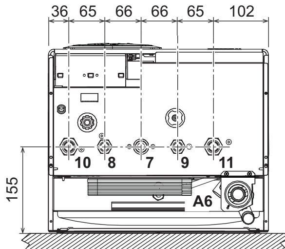
fig. 24- Vista inferior
