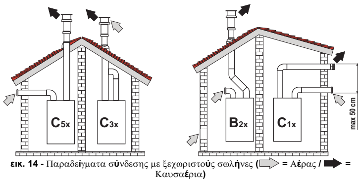
ΕΙΚ. 14 - Παραδείγματα σύνδεσης με ξεχωριστούς σωλήνες (⇨ = Αέρας / ⇩ = Καυσαέρια)
