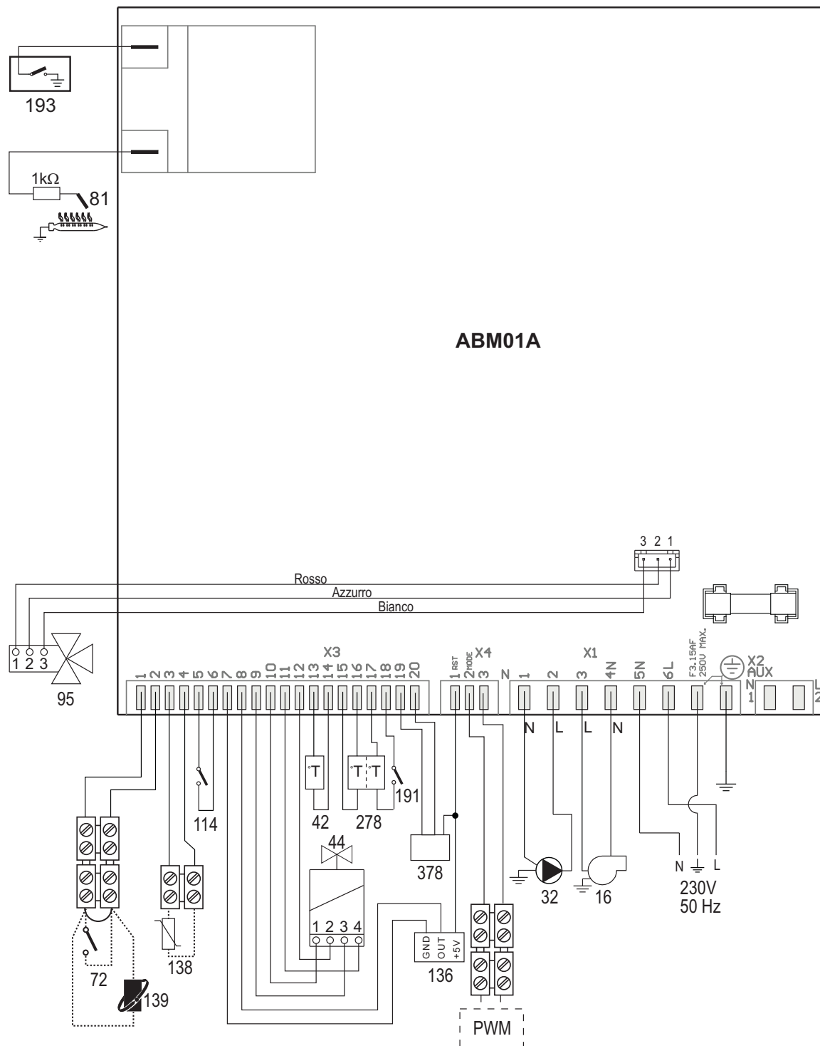
fig. 28- Esquema elèctrico
