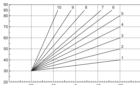
ΕΙΚ. 6 - Καμπύλες αντιστάθμισης
