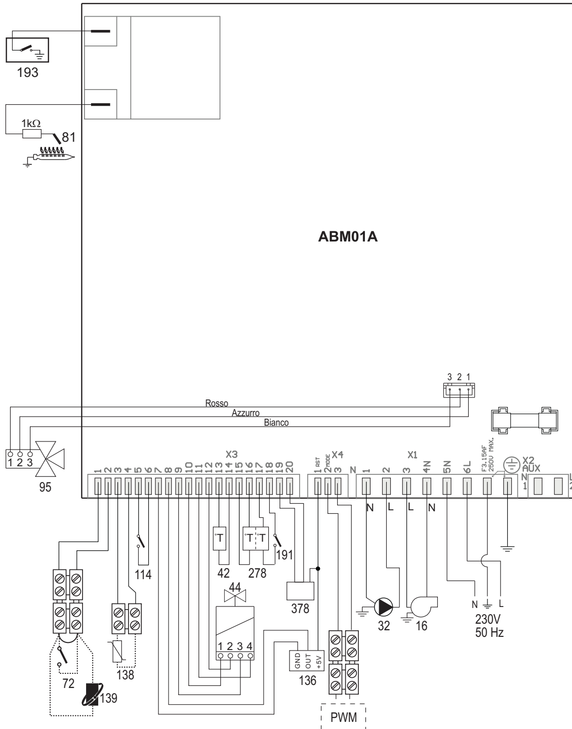
fig. 28 - Schema elettrico
