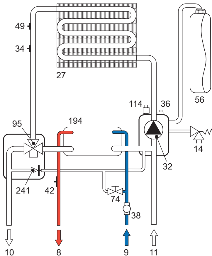
рис. 14 - Контур ГВС
