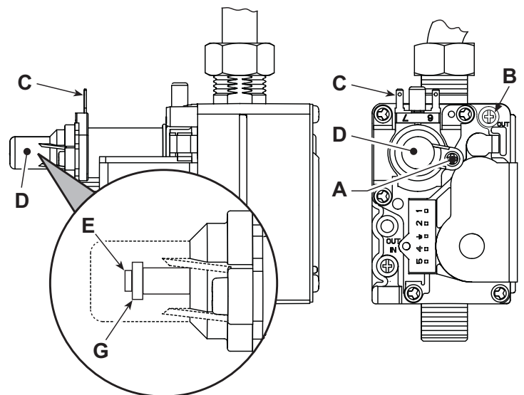
fig. 6 - Válvula del gas
