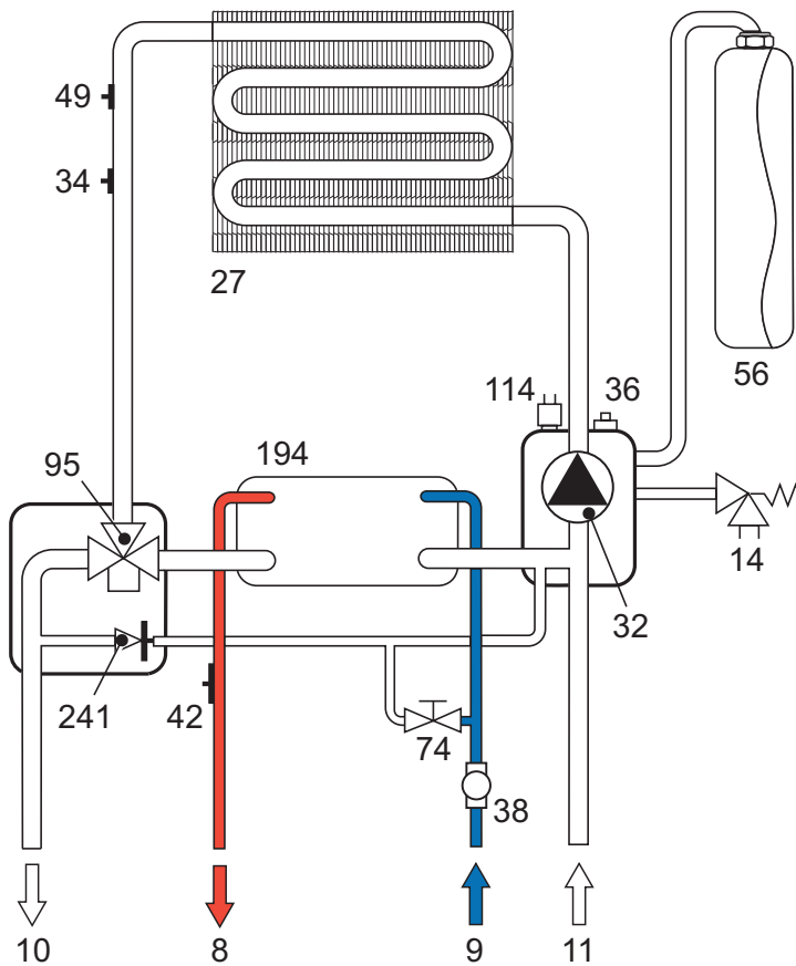
fig. 14 - Circuito de agua sanitaria
