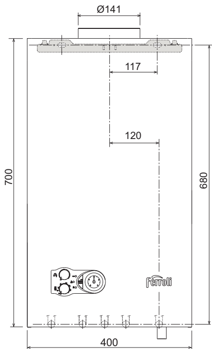
рис. 8 - Вид спереди
