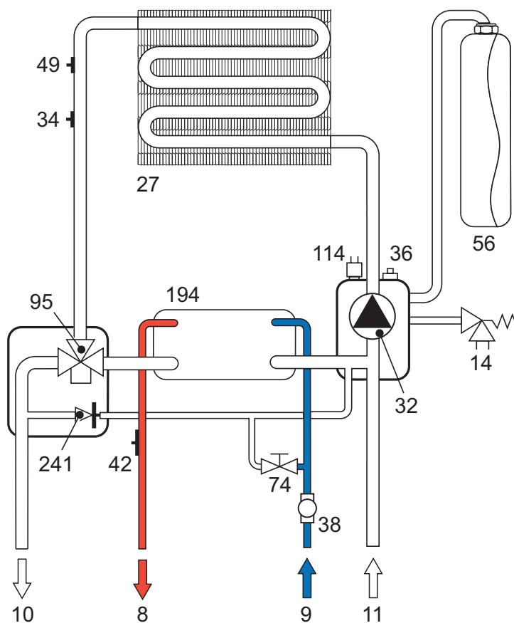
fig. 14 - Circuit sanitaire
