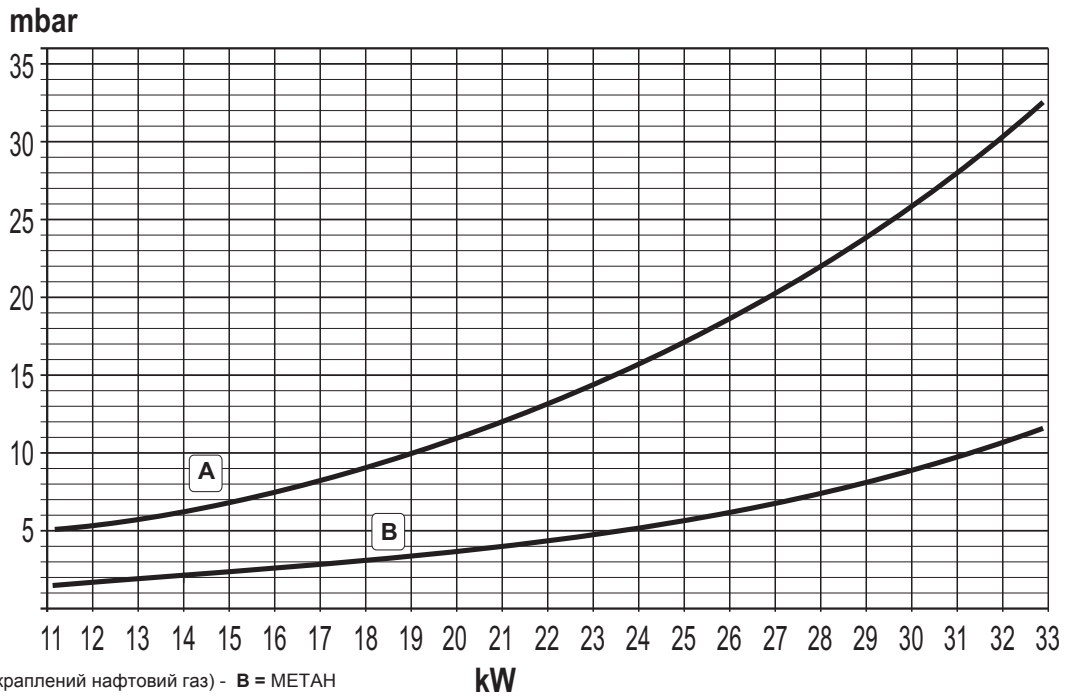
Втрати напору / тиску циркуляційних насосів
