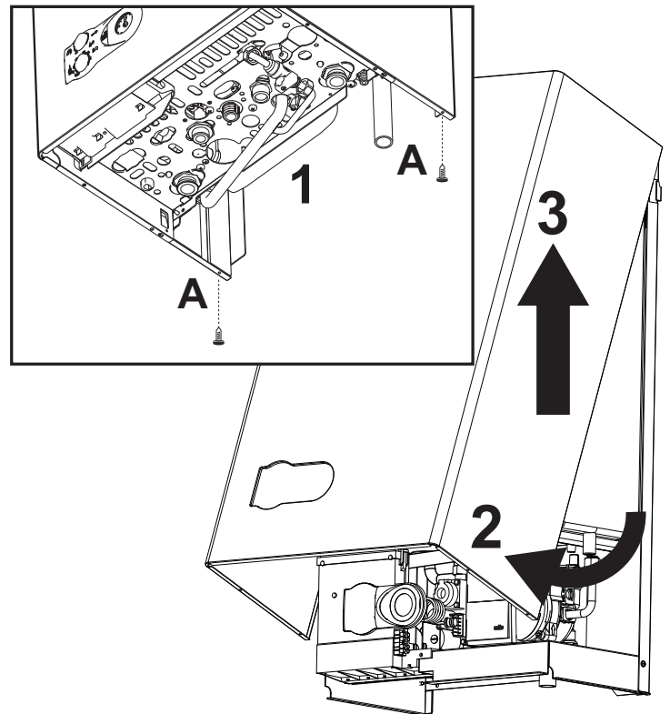
fig. 7 - Apertura mantello
