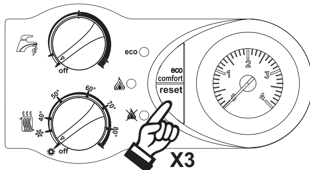
fig. 5 - TEST mode
