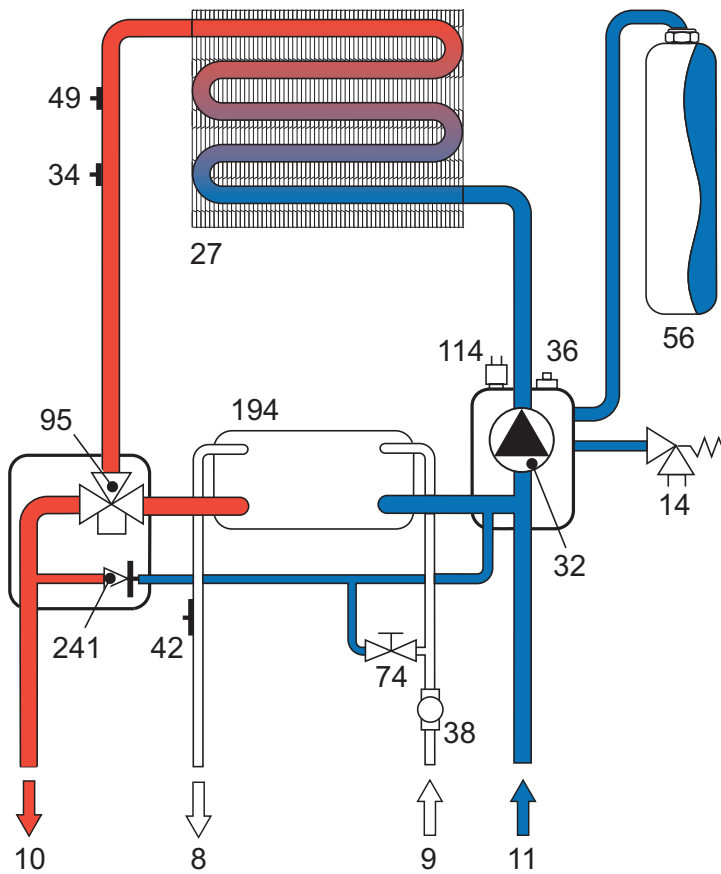
fig. 13 - Circuito Riscaldamento
