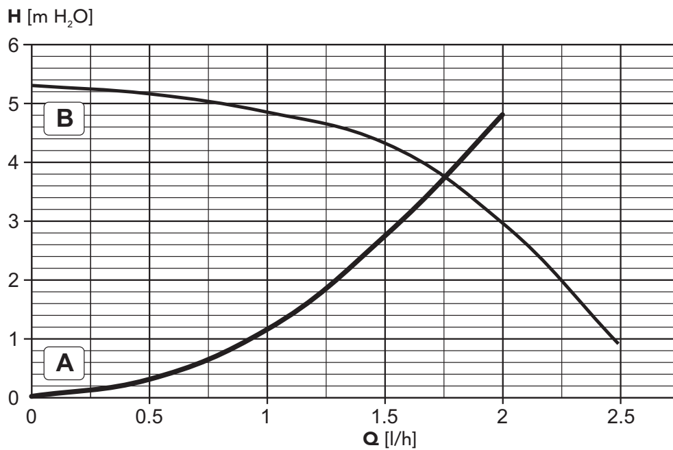
A = Спад потужності котла - B = Швидкість циркуляційного насосу
