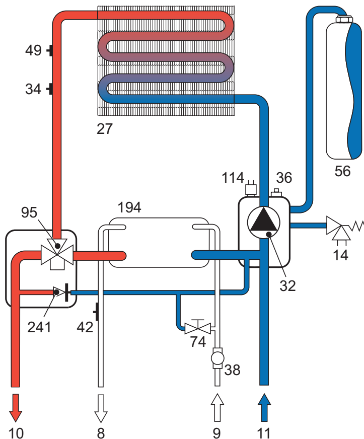
fig. 13 - Circuit chauffage
