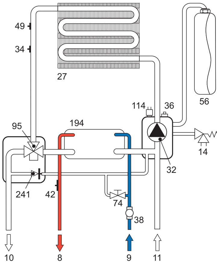
fig. 14 - Circuito Sanitario
