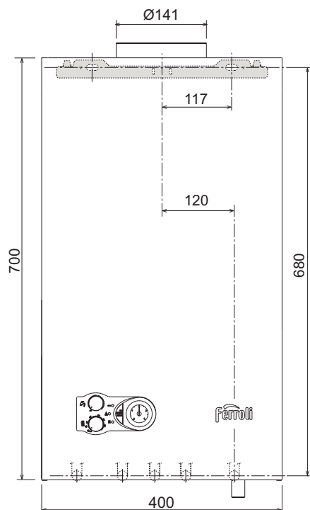
fig. 8 - Vue avant
