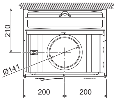
fig. 9 - Vista dall'alto
