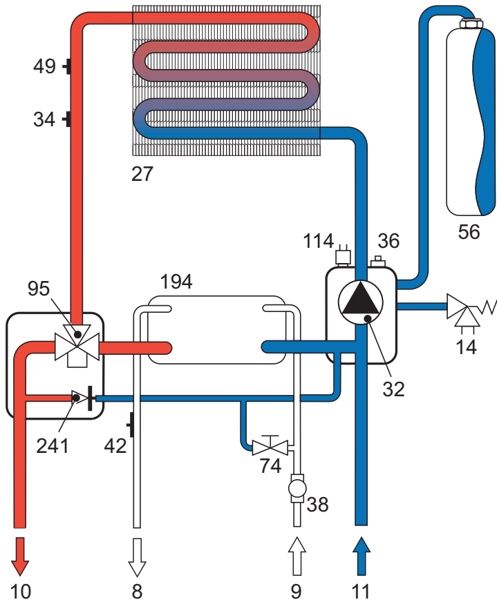
fig. 13 - Circuito de calefacción
