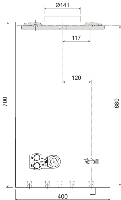
fig. 8 - Vedere frontală
