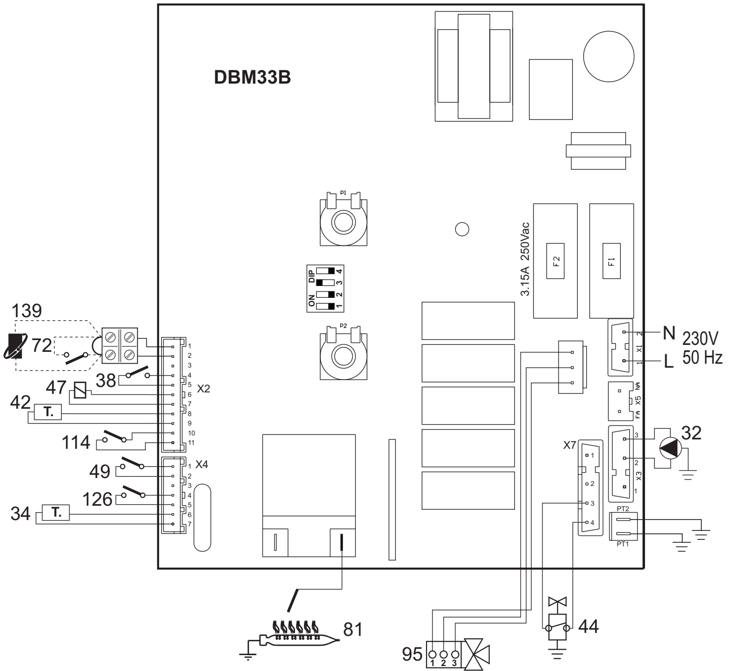
fig. 15 - Schema elettrico
