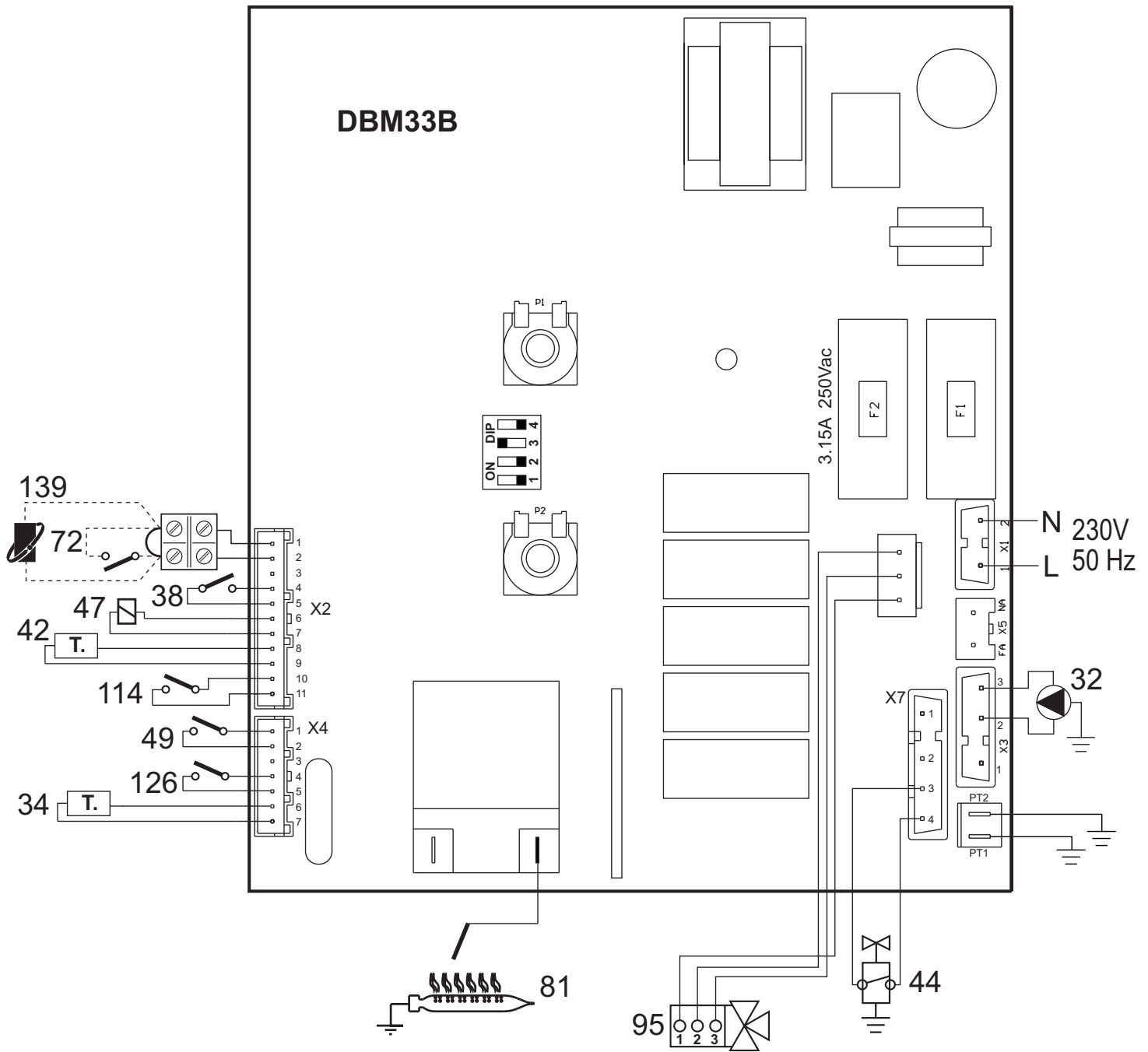
рис. 15 - Электрическая схема
