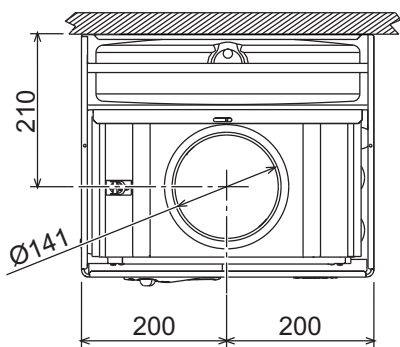
рис. 9 - Вид сверху
