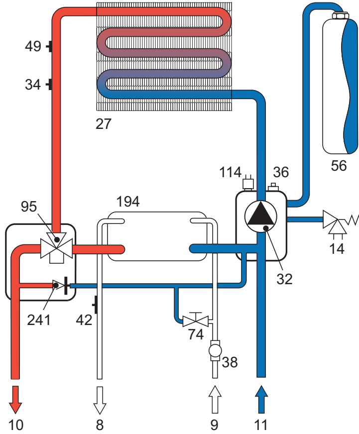
şek. 13 - Isıtma Devresi
