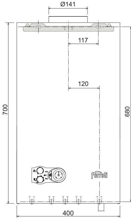
fig. 8 - Vista frontale
