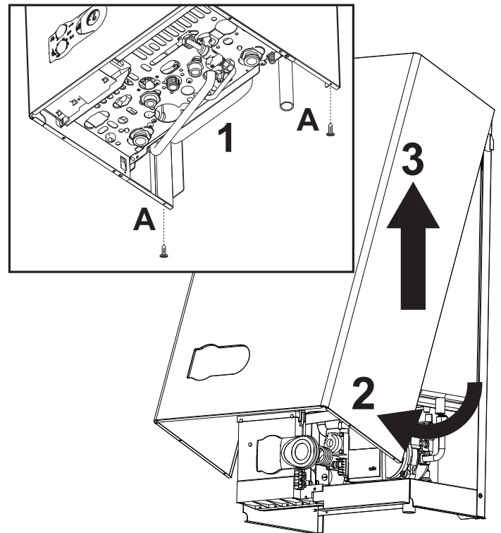
мал. 7 - Зняття обшивки
