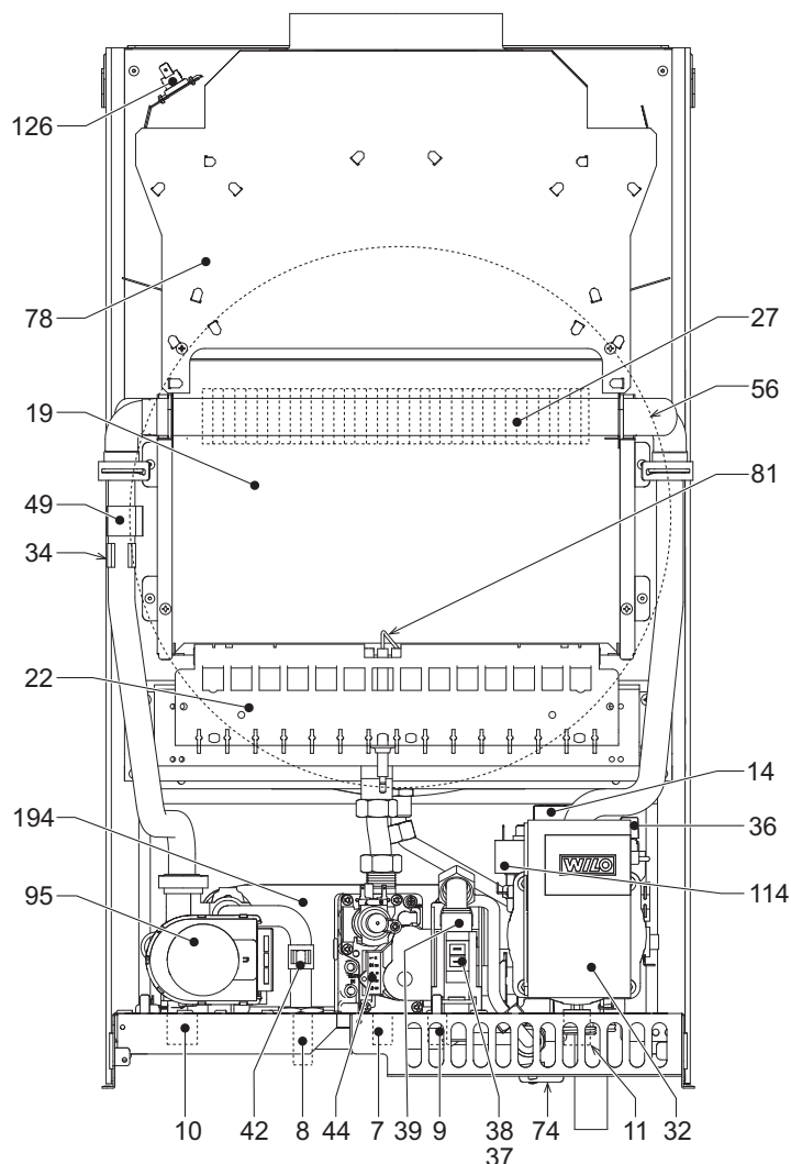
fig. 12 - Vista general
