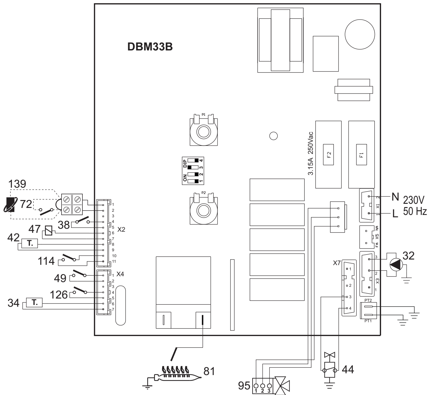
fig. 15 - Esquema eléctrico
