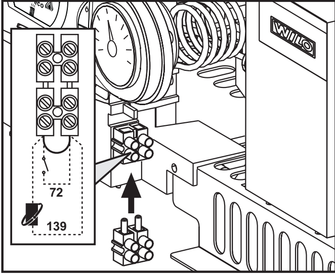
şek. 4 - Terminal kutusuna erişim
