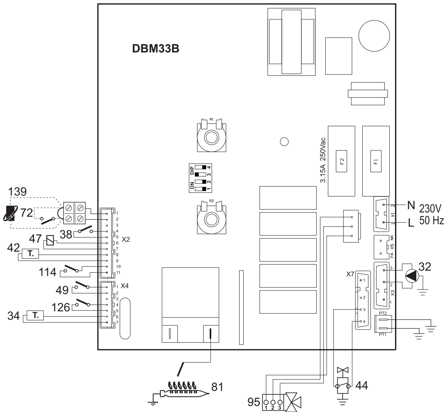
fig. 15 - Wiring diagram
