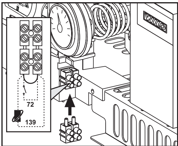
рис. 4 - Доступ к клеммной коробке
