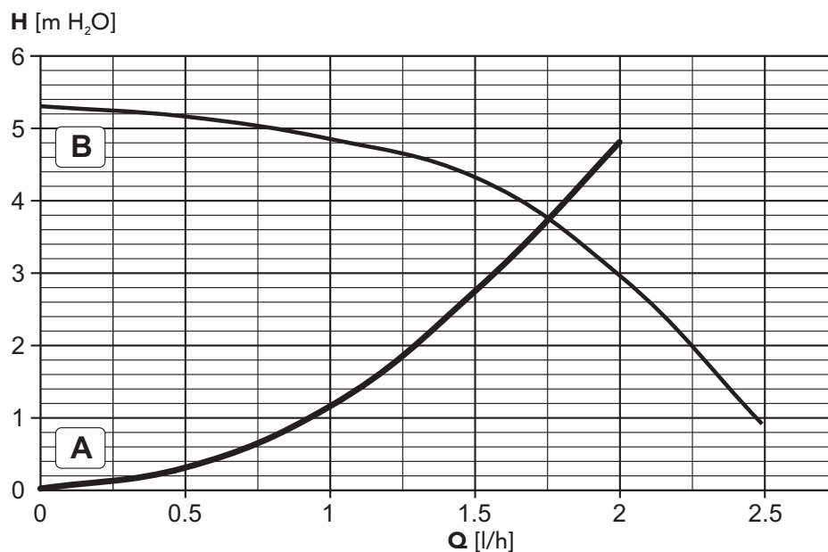
Perdite di carico / prevalenza circolatori
