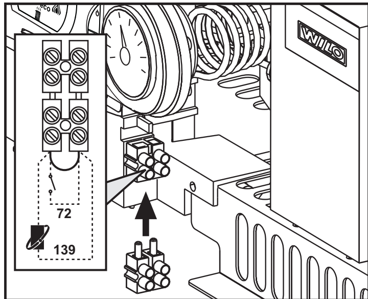
fig. 4 - Accesso alla morsettiera
