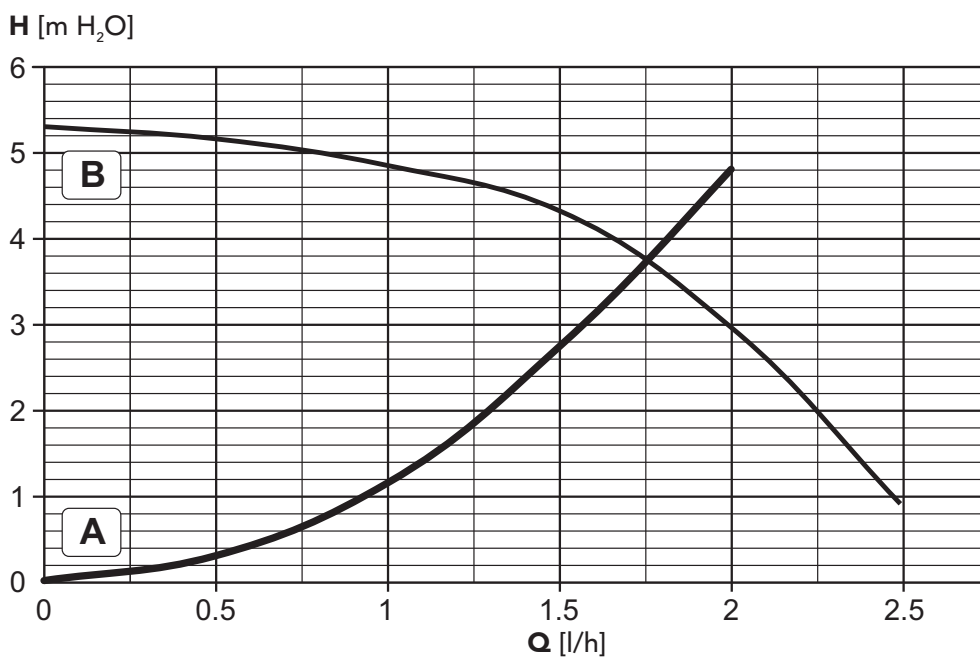
Потери нагрузки/напора циркуляционных насосов
