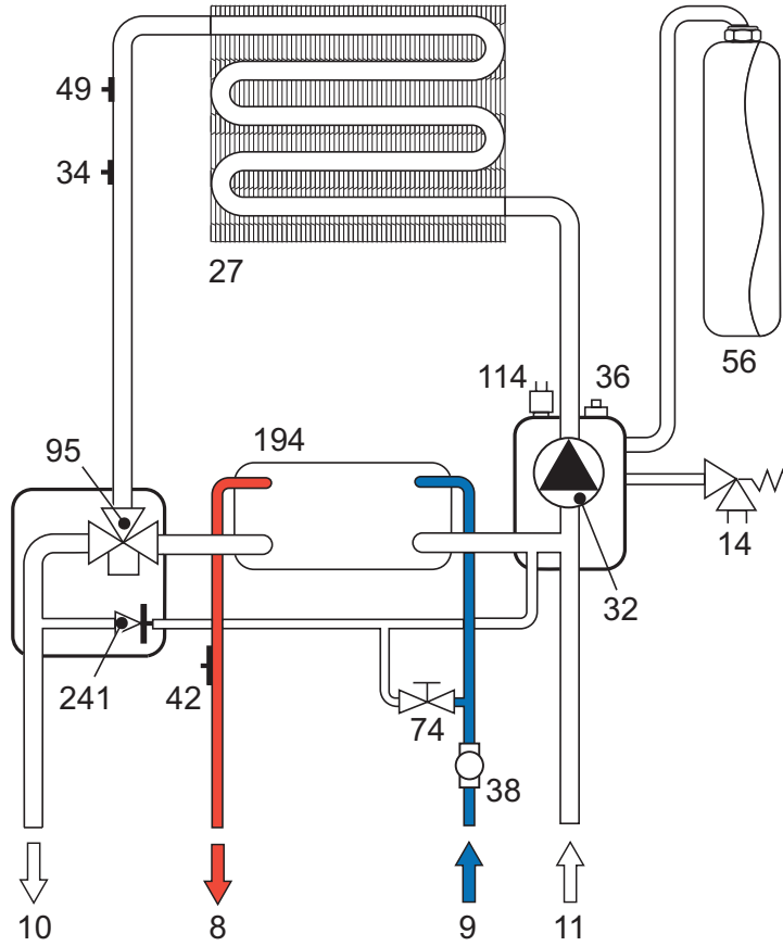
şek. 14 - Sıhhi Su Devresi
