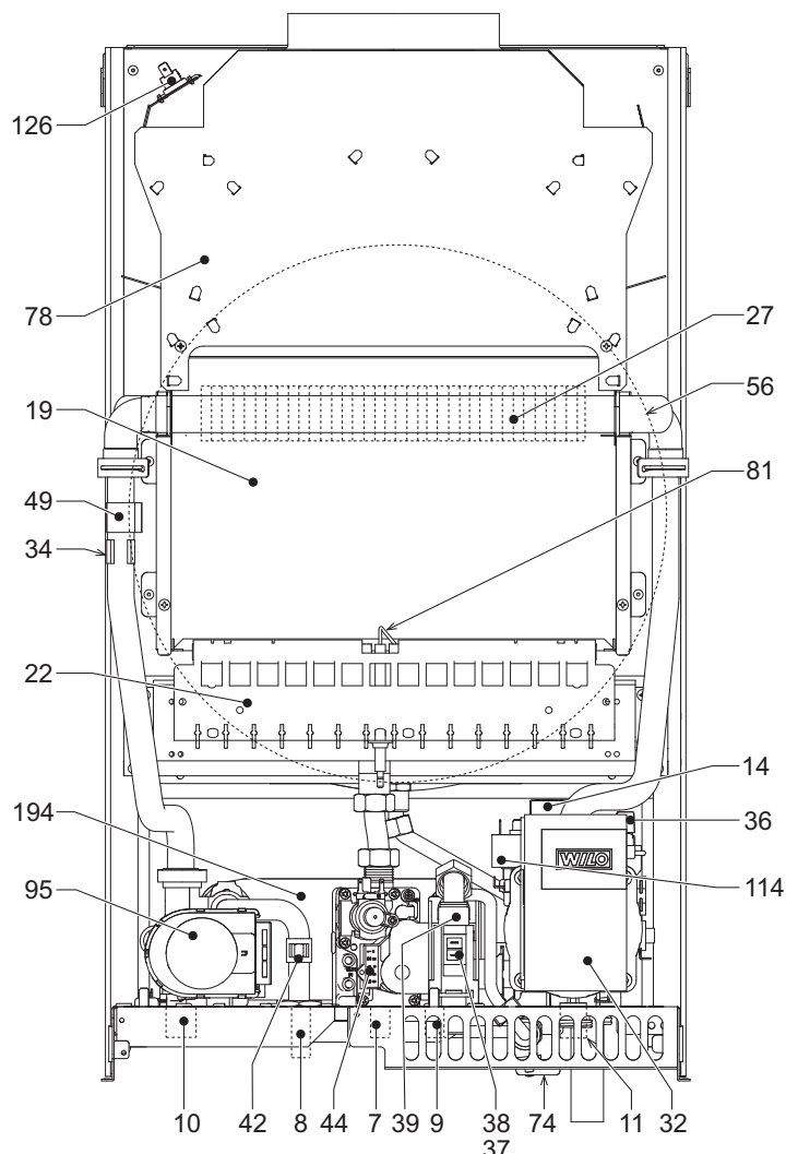
рис. 12 - Общий вид
