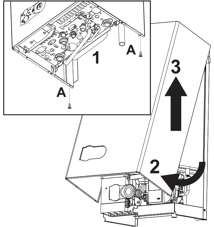
şek. 7 - Muhafazanın/kasanın açılması
