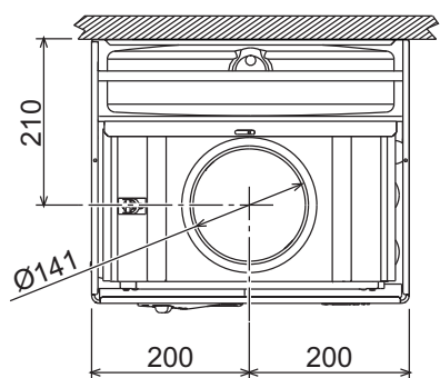
fig. 9 - Vista superior
