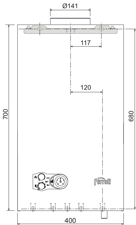
fig. 8 - Vista frontal
