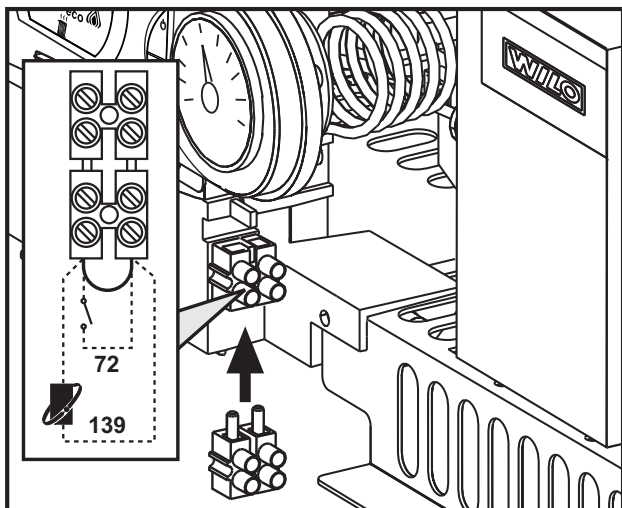
мал. 4 - Доступ до клемної коробки
