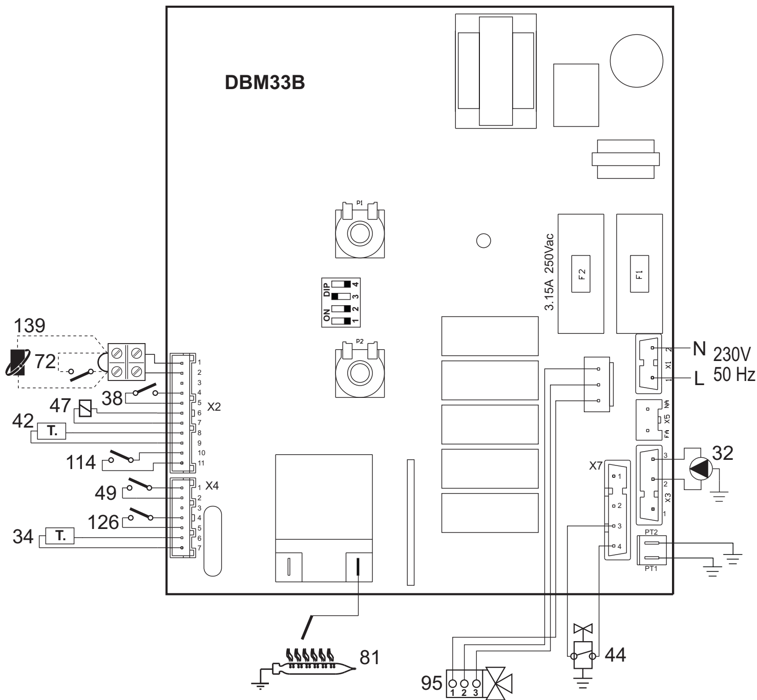
fig. 15 - Schemă electrică
