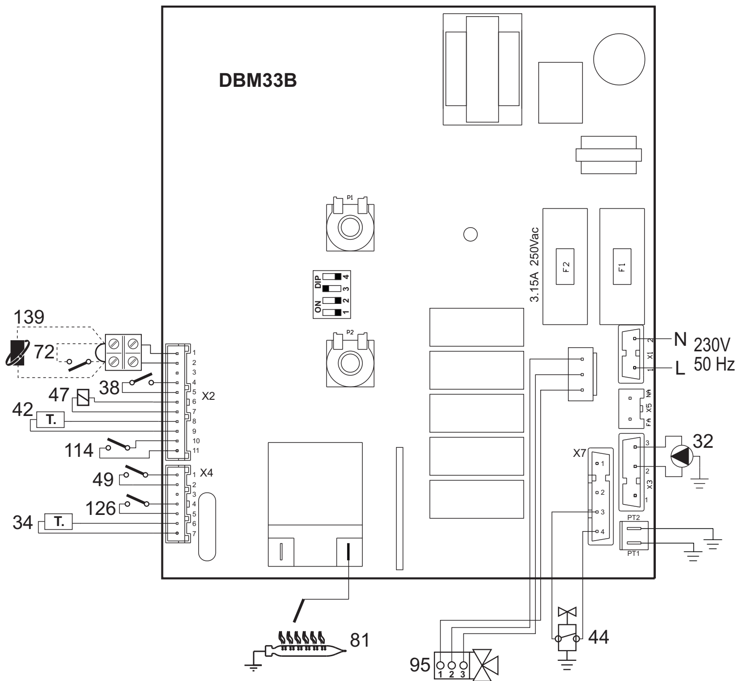
fig. 15 - Schéma électrique
