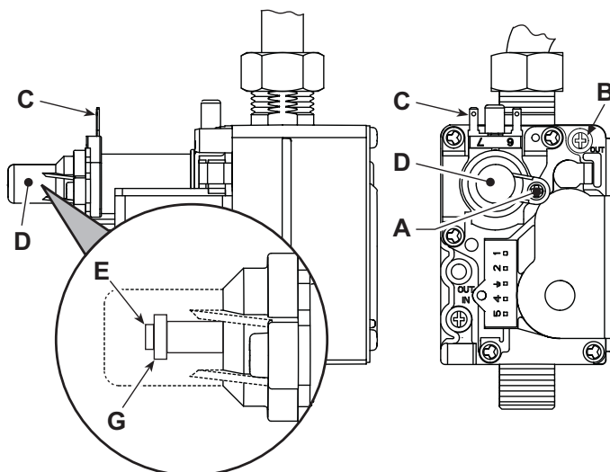
рис. 6 - Газовый клапан
