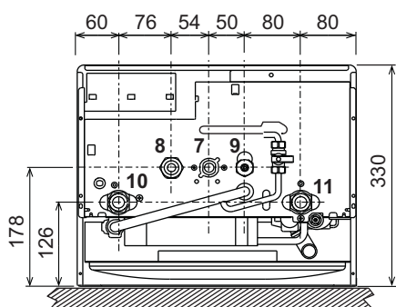
fig. 10 - Vista inferior
