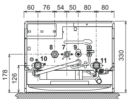
рис. 10 - Вид снизу
