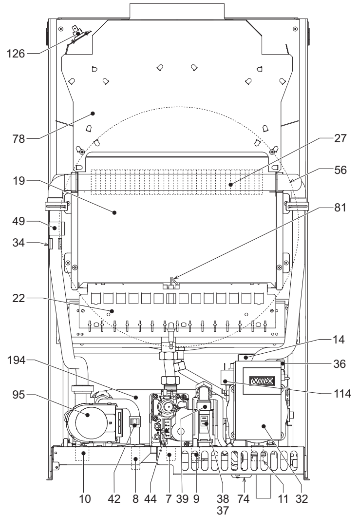
fig. 12 - Vista generale
